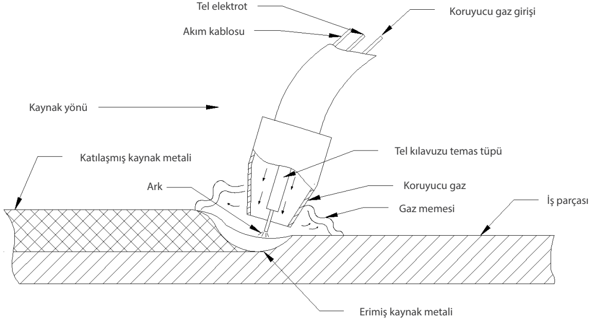
GörSEL 12.31: Kaynak konumlarının parça üzerine etkileri
