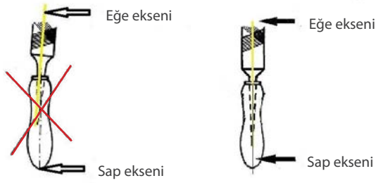
Görsel 3.6: Eğelere sap takma yöntemleri
