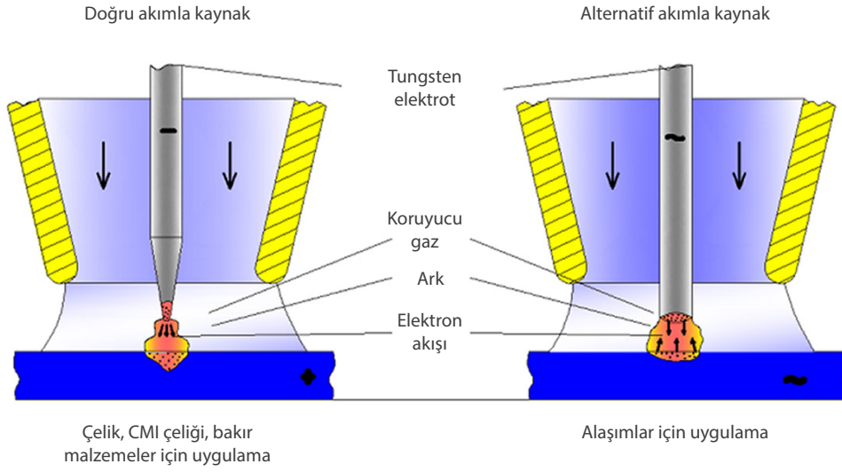
Görsel 13.9: Arkın ateşlenmesi
