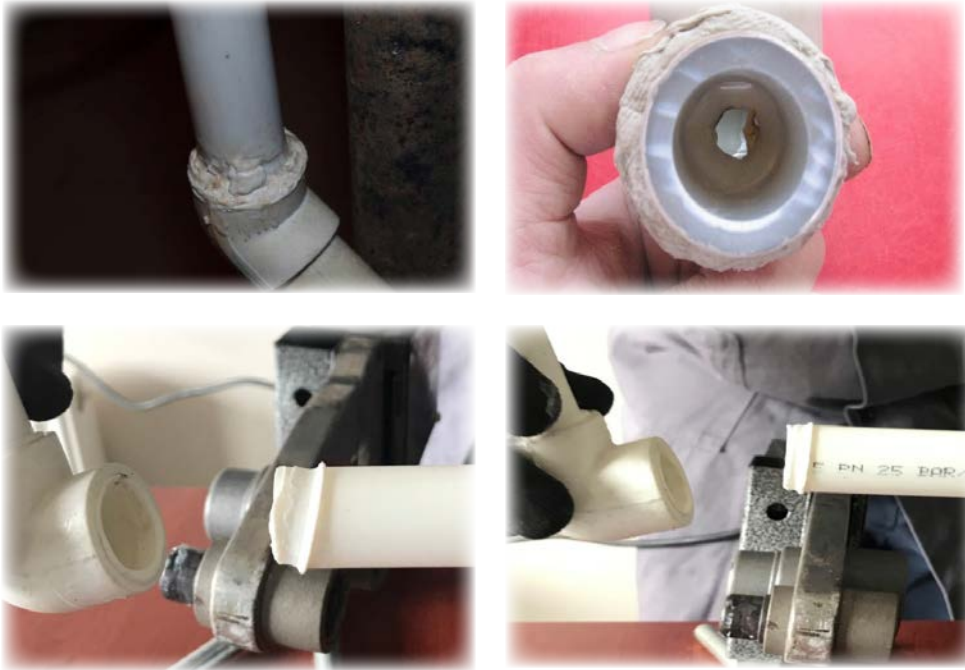
Görsel 5.8: PPRC boru kaynak işleminde yapılan hatalar
