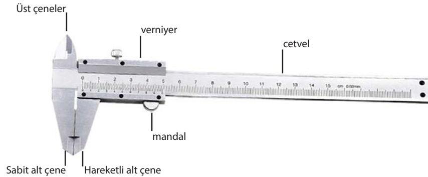
Görsel 2.6: Kumpas
