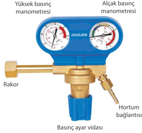
Görsel 8.4: Oksijen basınç düşürücüsü
