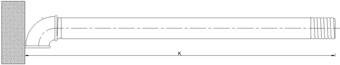
Görsel 4.29: Uçtan sırta ölçü alma
