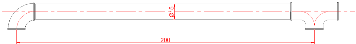
Görsel 4.35: Fittings sıkılmış boru ölçüsü
