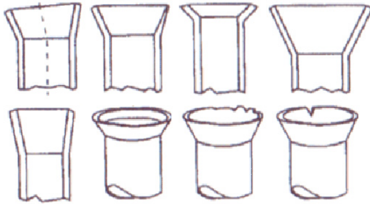
Görsel 6.15: Hatalı havşa örnekleri
