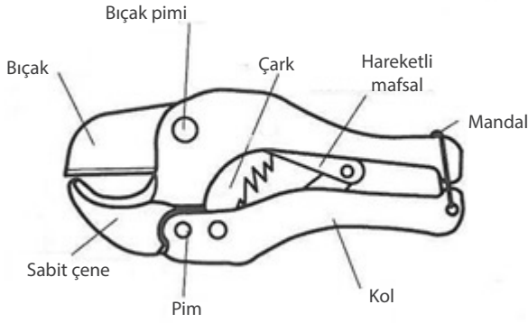
Görsel 5.2: Polipropilen boru kesme makası
