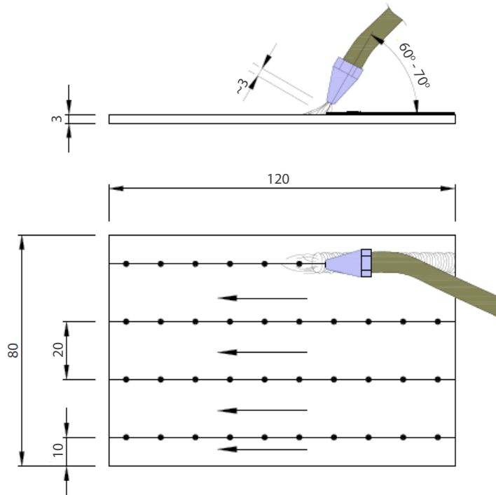
Görsel 9.3: Kaynak uygulaması
