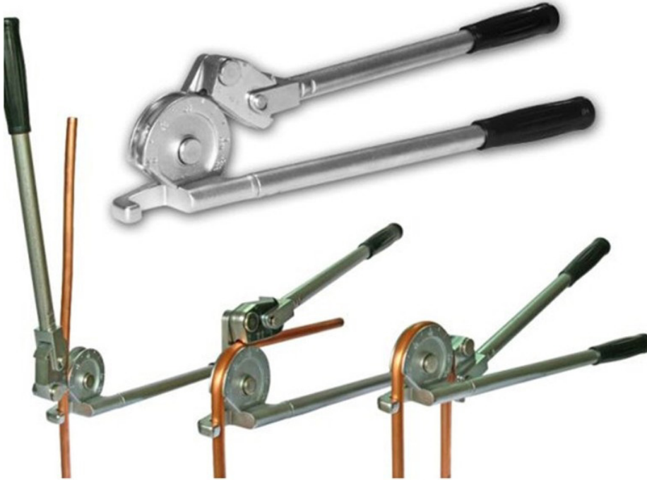
Görsel 6.21: Bakır boru bükme şekilleri
