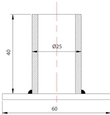
Görsel 12.24: Kaynak yapılacak metalin ve borunun ölçüsü
