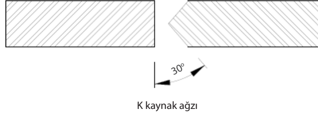
Görsel 9.1: Kaynak ağızı çeşitleri
