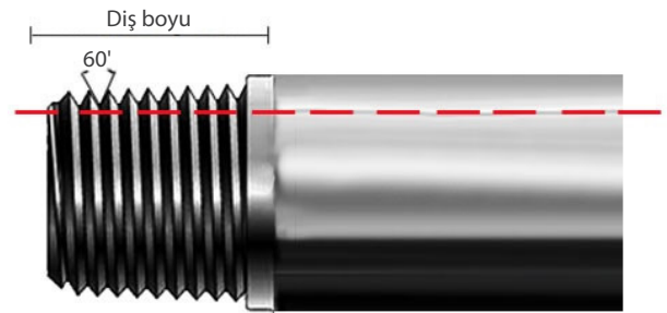
Görsel 4.11: Çelik boru vida bölümleri
