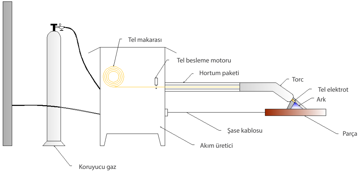
Görsel 12.2: MIG-MAG kaynak donanımları
