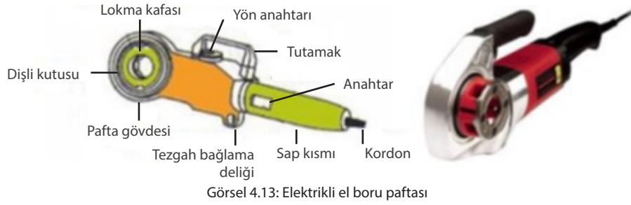
Görsel 4.13: Elektrikli el boru paftası
