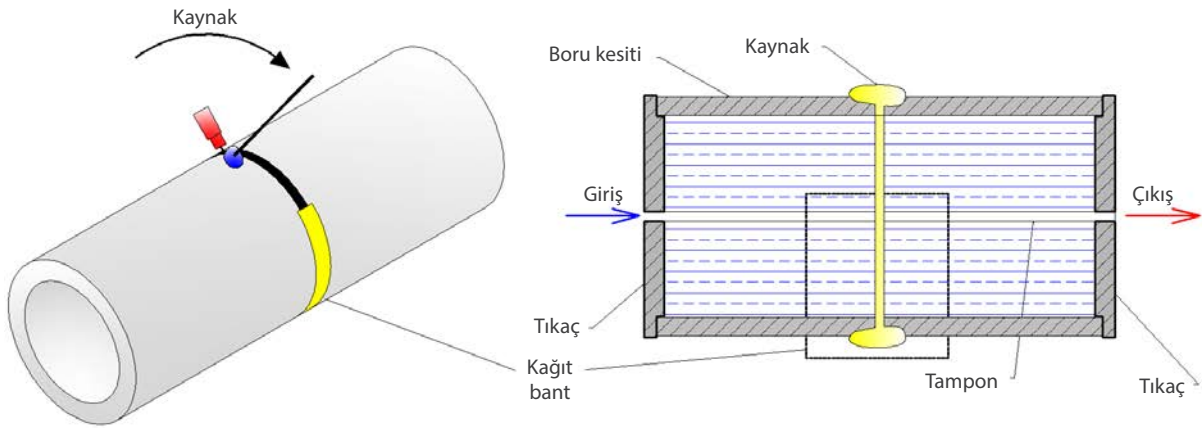
Görsel 13.13: Tampon gaz kullanılarak yapılan boru kaynağı
