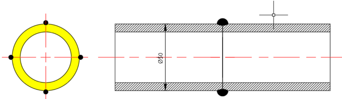
Görsel 11.8: Puntalama işlemi
