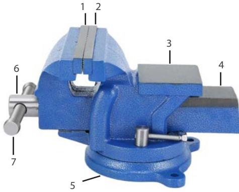
Görsel 3.1: Tesviyeci mengenesi ve kısımları
