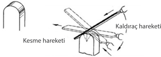
Görsel 3.16: Dışa kavisli yüzeylerin eğelenmesi
