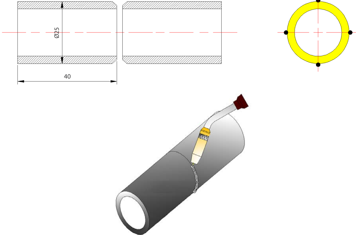
Görsel 12.32: Kaynak yapılacak borunun ölçüsü
