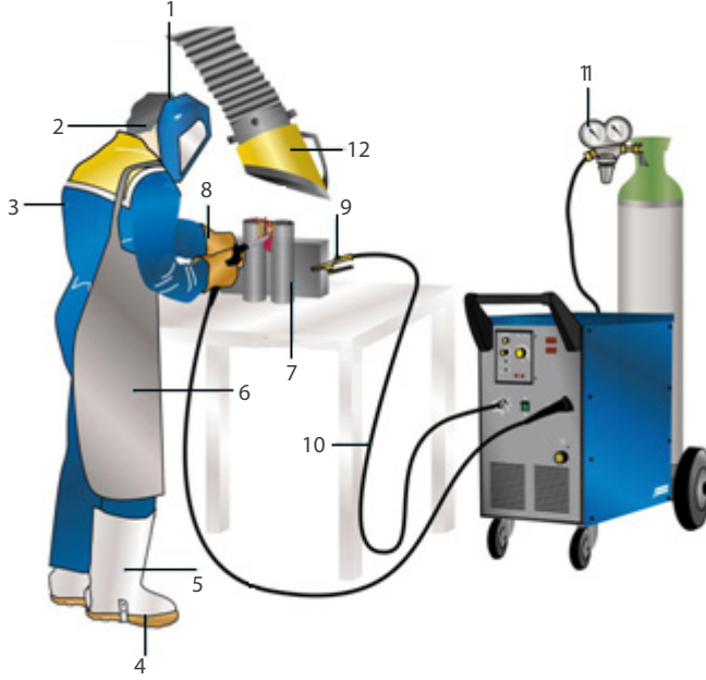
Görsel 13.16: TIG kaynağında güvenlik ekipmanı
