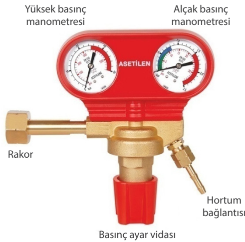
Görsel 8.3: Asetilen basınç düşürücüsü
