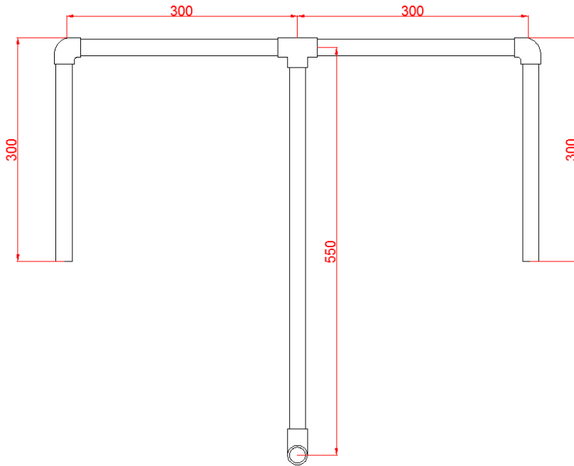
Görsel 5.10: Polipropilen boru kaynak bağlantısı
