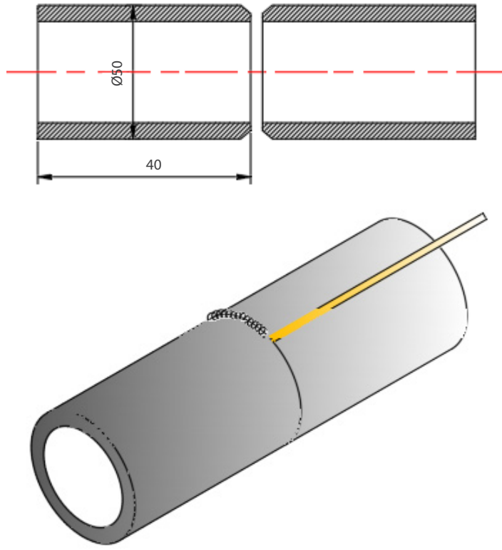
Görsel 11.9: Kaynak işlemi
