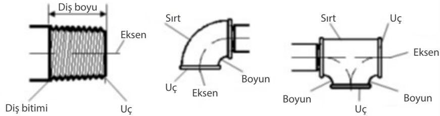
Görsel 4.26: Boru üzerinde ölçü alma terimleri
