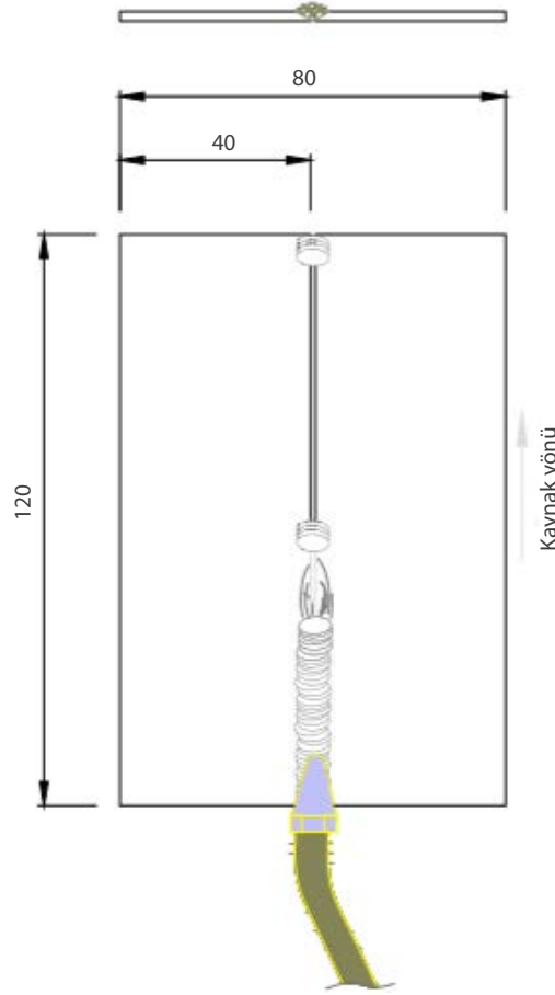
Görsel 9.10: Kaynak uygulaması
