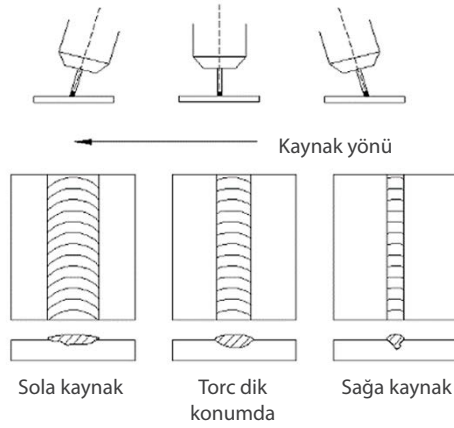
Görsel 12.29: Kaynak konumlarının parça üzerine etkileri
