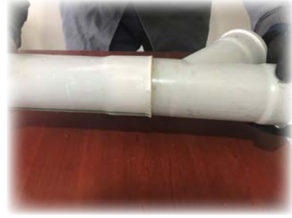
Görsel 5.21: Muf açılmış boruyu birleştirme
