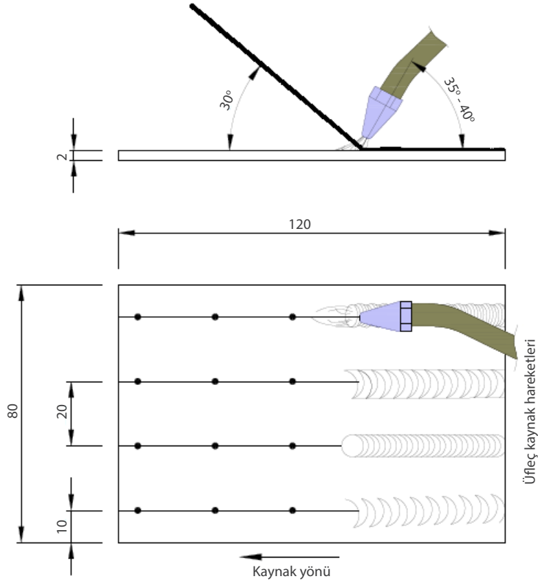
Görsel 9.5: Kaynak uygulaması
