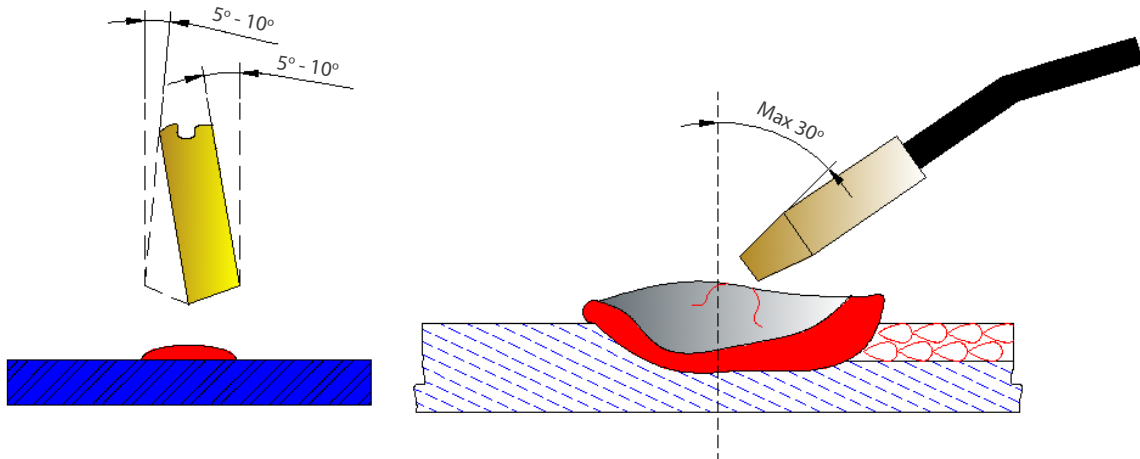
Görsel 12.14: Torcun iş parçasına göre konumu
