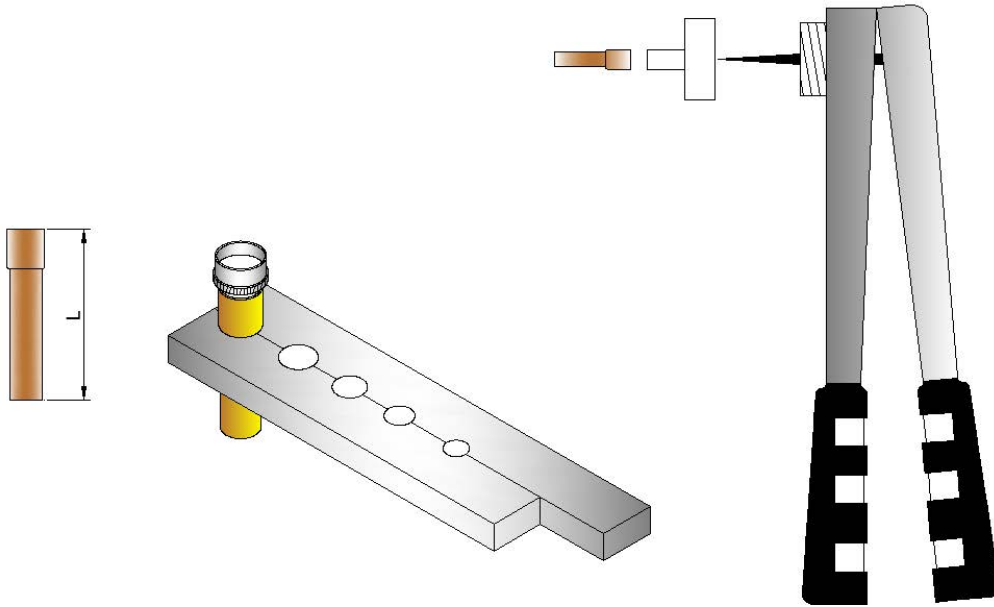
Görsel 7.2: Muf açım yöntemleri
