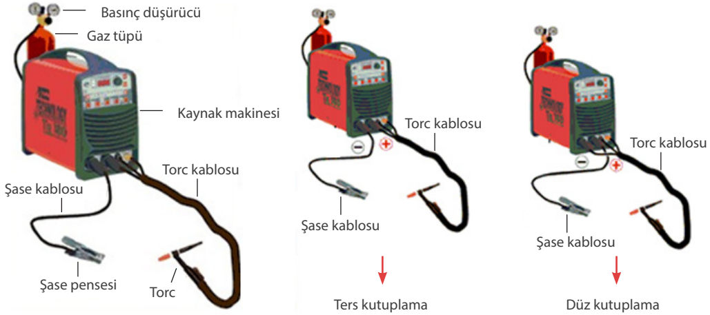
Görsel 13.6: TIG kaynak makinesi kutuplama
