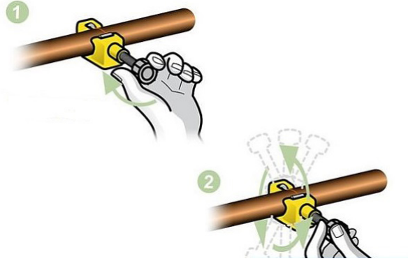
Görsel 6.5: Bakır boru makası ile boru kesme işlemi
