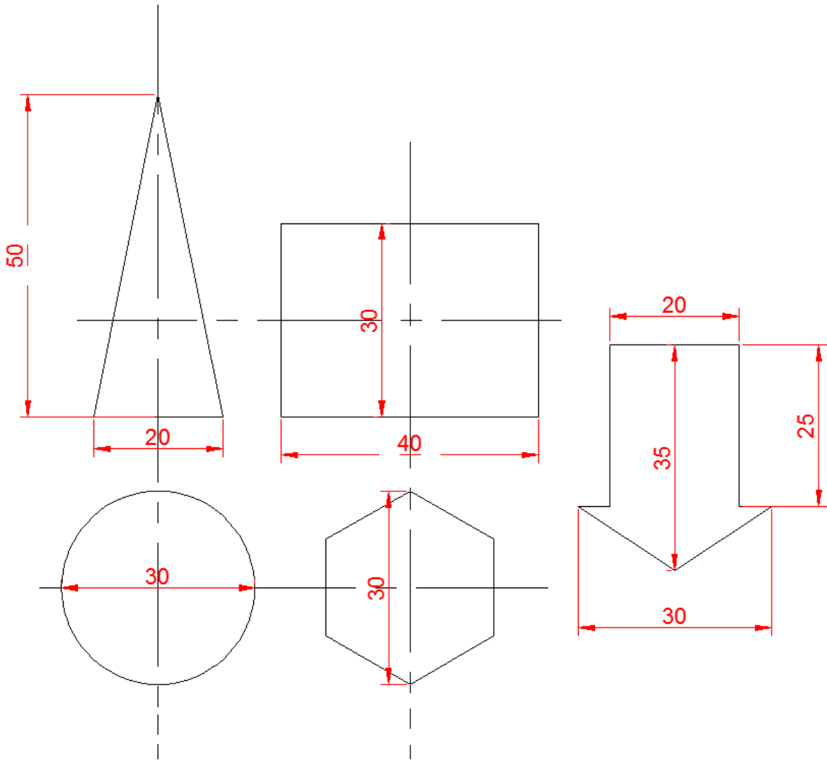
Görsel 2.28: Sac üzerine markalama çizimleri
