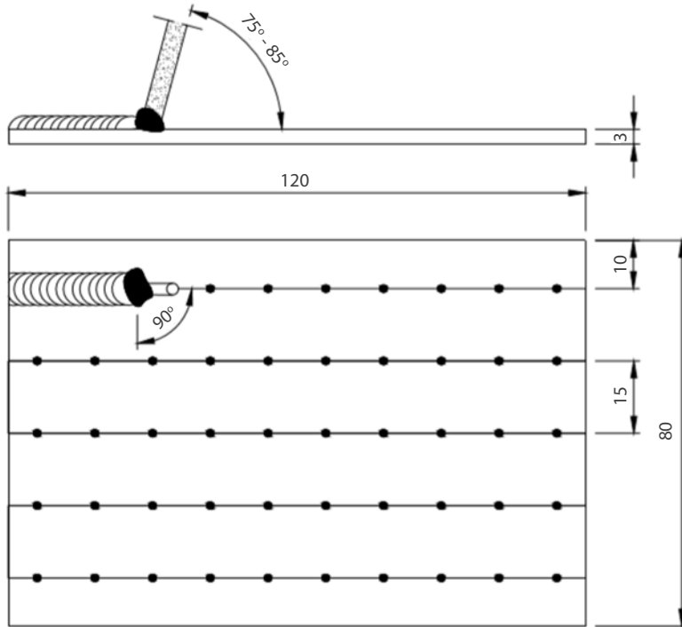
Görsel 11.4: Kaynak işlemi
