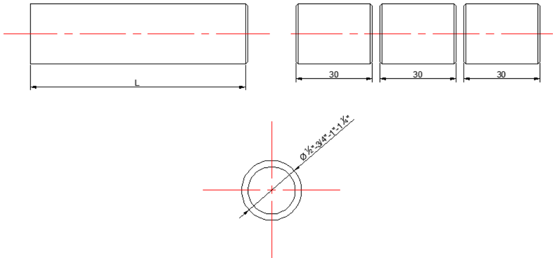
Görsel 4.10: Kesilecek boru ölçüleri
