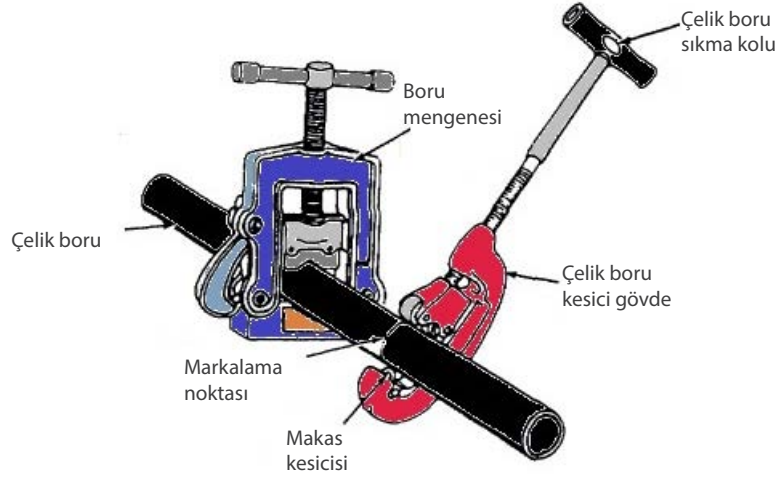
Görsel 4.6: Boru kesici ile kesme yönü
