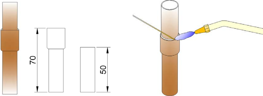
Görsel 7.9: Bakır borulara sert lehimleme
