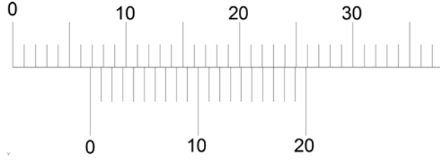
Görsel 2.14: Çeşitli hassasiyetteki kumpas örnekleri
