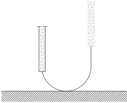
Vurarak ark başlatma
