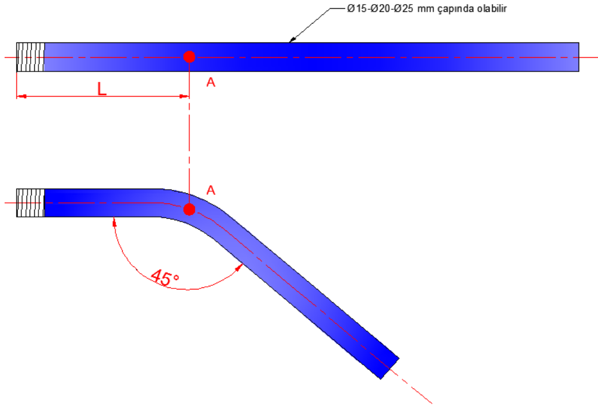
Görsel 4.42: 45° bükülmüş çelik boru ölçüleri
