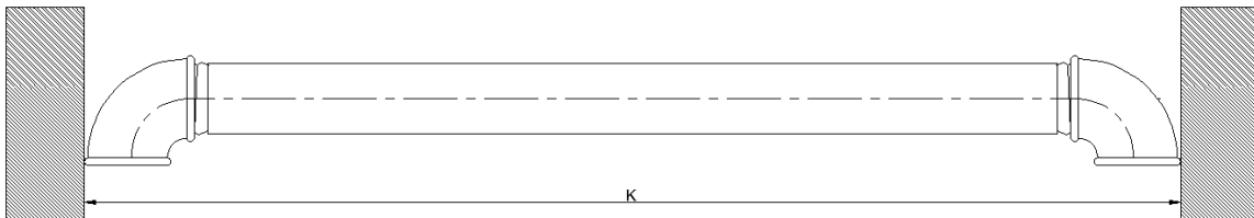
Görsel 4.31: Sırttan sırta ölçü alma
