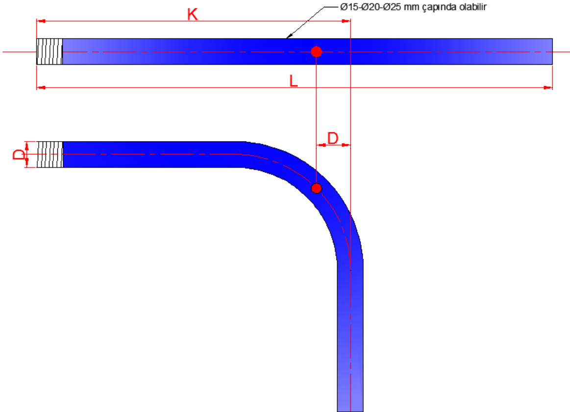
Görsel 4.41: 90° bükülmüş çelik boru ölçüleri
