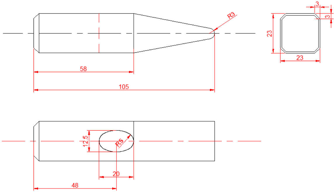
Görsel 3.17: Tesviyeci çekici ölçüleri
