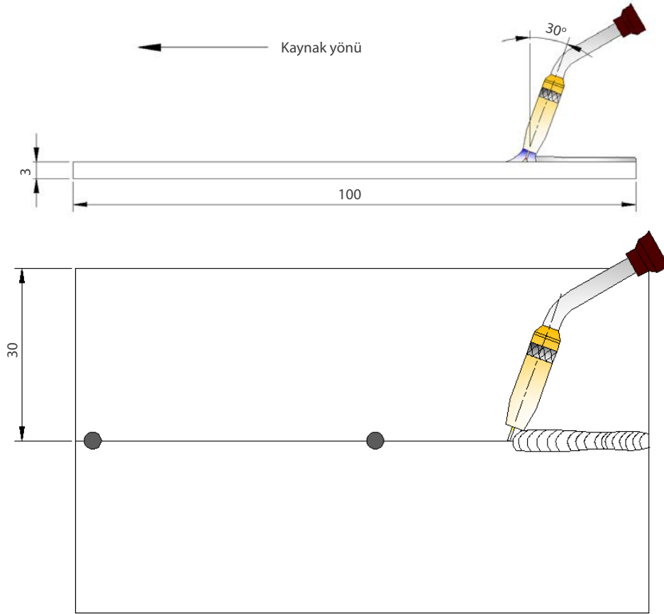
Görsel 12.19: Kaynak yapılacak metalin ölçüsü ve kaynak yönü
