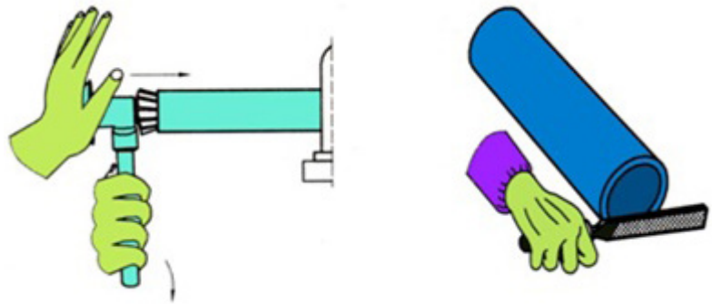
Görsel 13.15: Çapak temizleme
