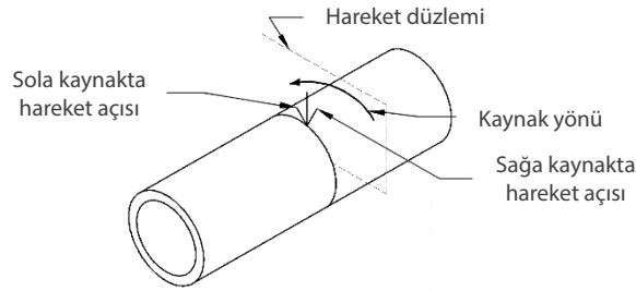
Görsel 12.28: Hareket düzlemi üzerinde çalışma açısı
