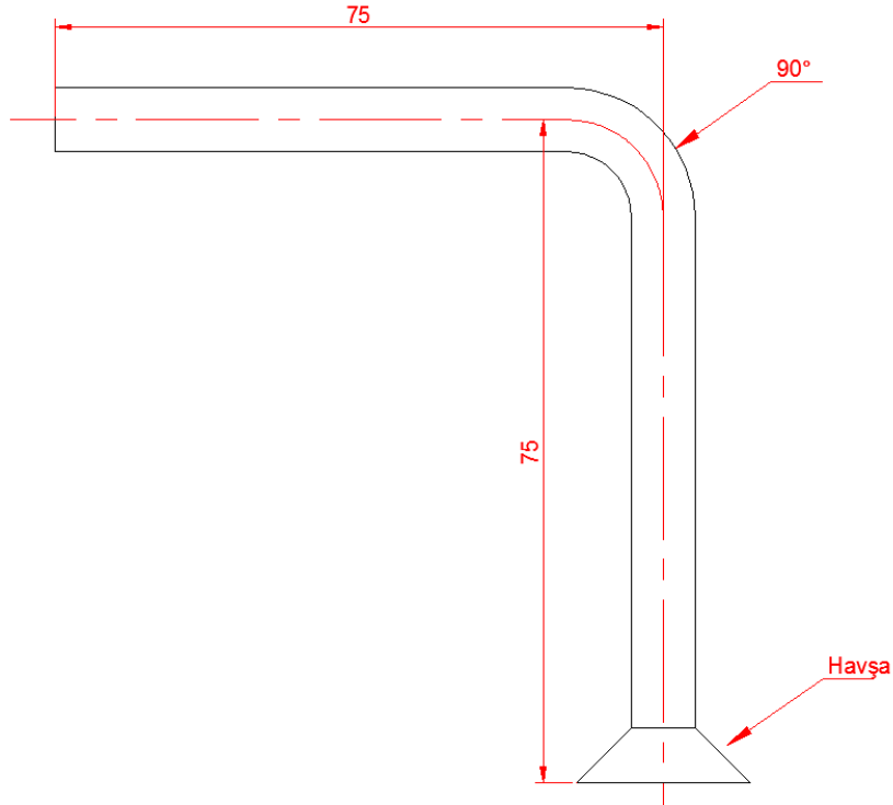
Görsel 6.23: Bakır boru birleştirme çizimi
