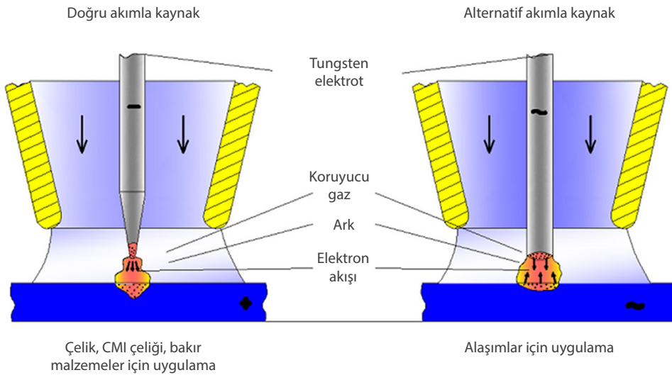
Görsel 13.22: Malzeme cinsine göre elektrodun ucu ve akımın seçimi
