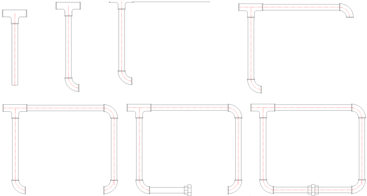
Görsel 4.36: Kare bağlantı ölçüleri ve işlem sıralaması
