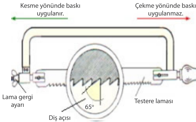
Görsel 4.2: Testere laması takma yönü
