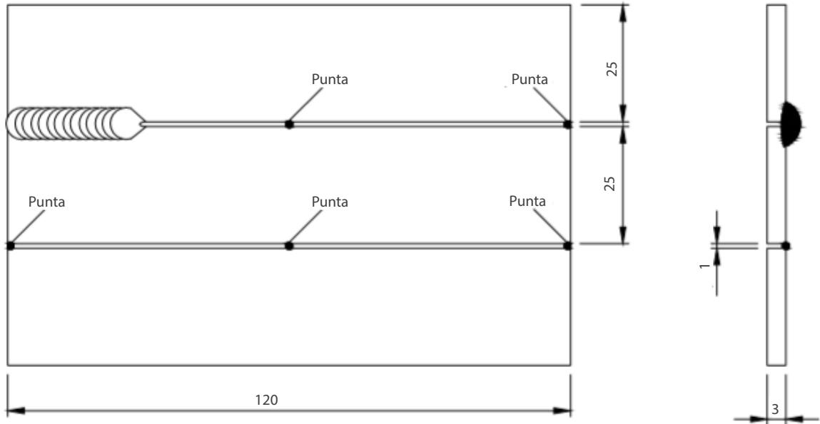
Görsel 11.5: Kaynak işlemi
