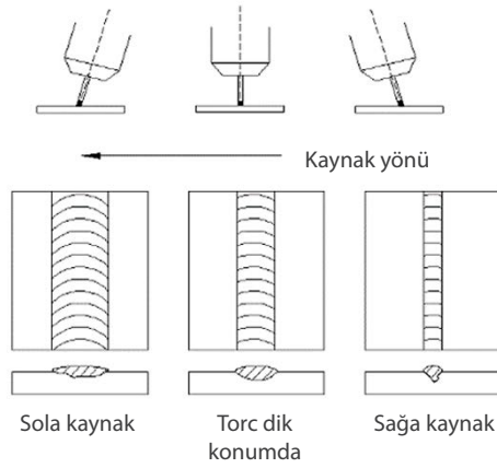
Görsel 12.15: Kaynak konumlarının parça üzerine etkileri
