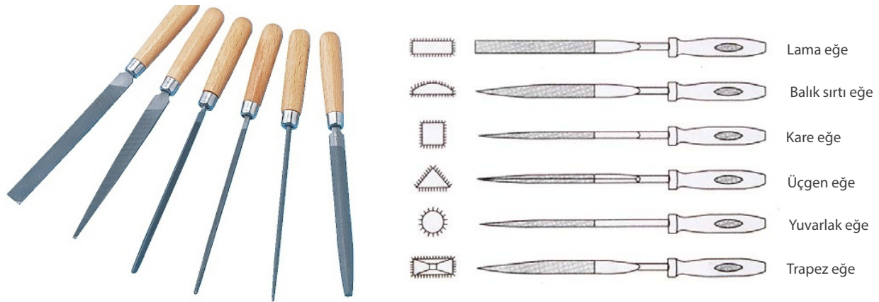
Görsel 3.4: Eğe çeşitleri
