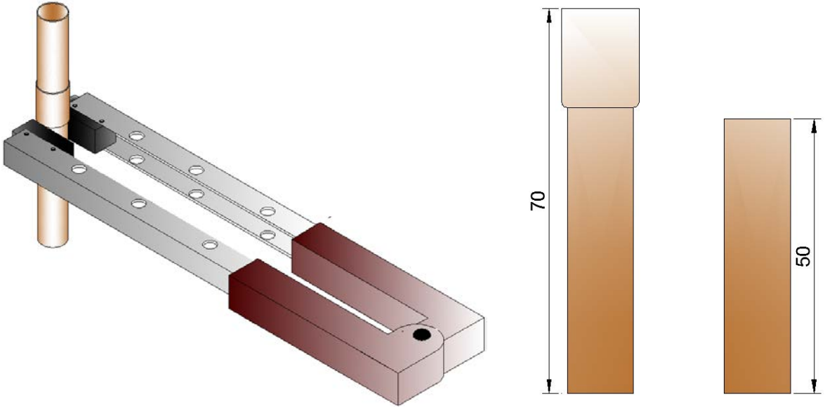
Görsel 7.6: Bakır borulara yumuşak lehimleme
