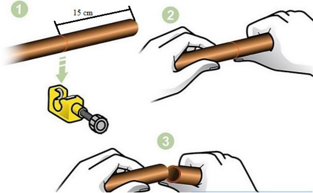
Görsel 6.7: Bakır boru kesme işlemi
