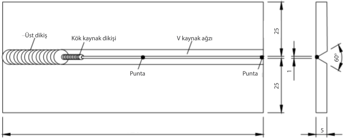
Görsel 11.6: Kaynak işlemi
