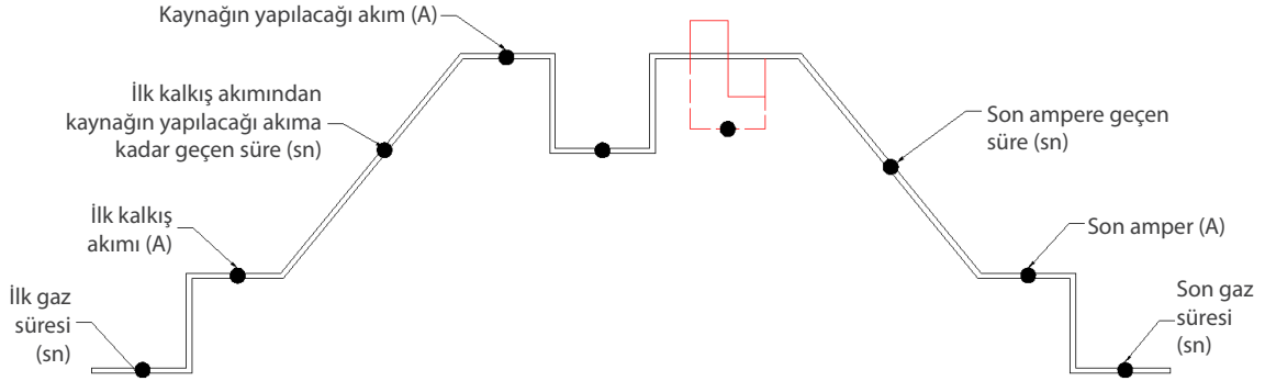
Görsel 13.12: TIG kaynak makinesi parametre şeması
