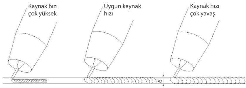
Görsel 12.30: Kaynak konumlarının parça üzerine etkileri
