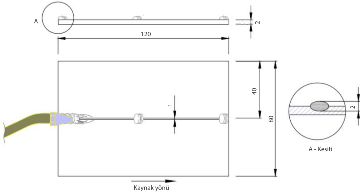
Görsel 9.7: Kaynak uygulaması
