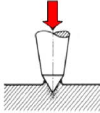
Görsel 2.24: İş parçasına nokta vurma işlemi ve bıraktığı iz
