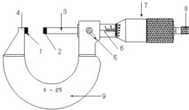
Görsel 2.13: Mikrometre gövde ve yapısı
