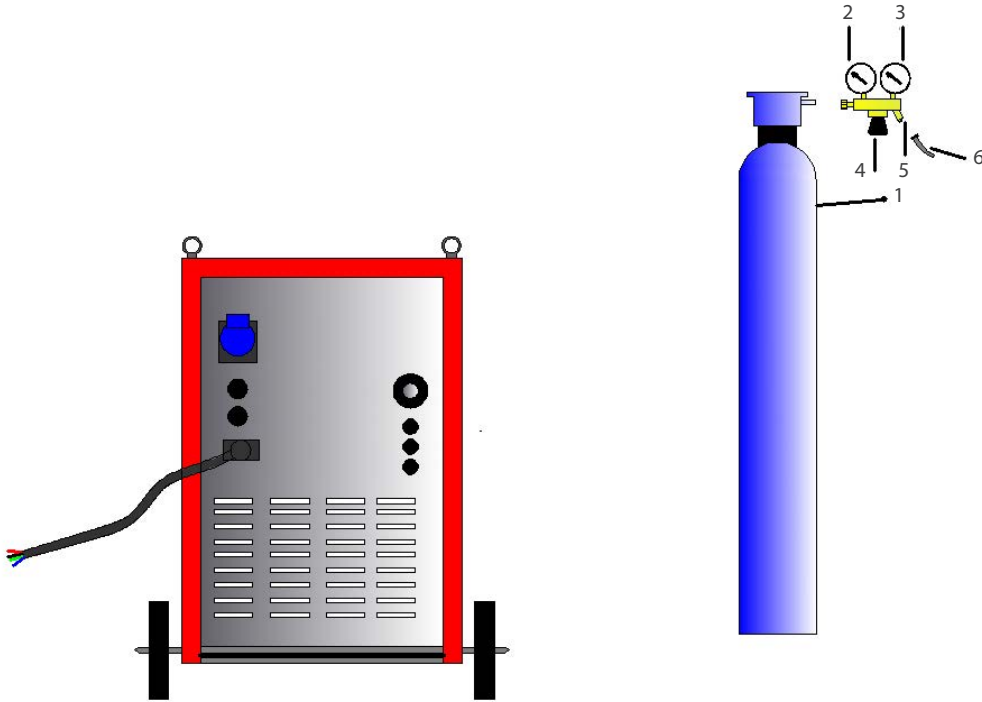
Görsel 12.12: Regülatör bağlantısı
