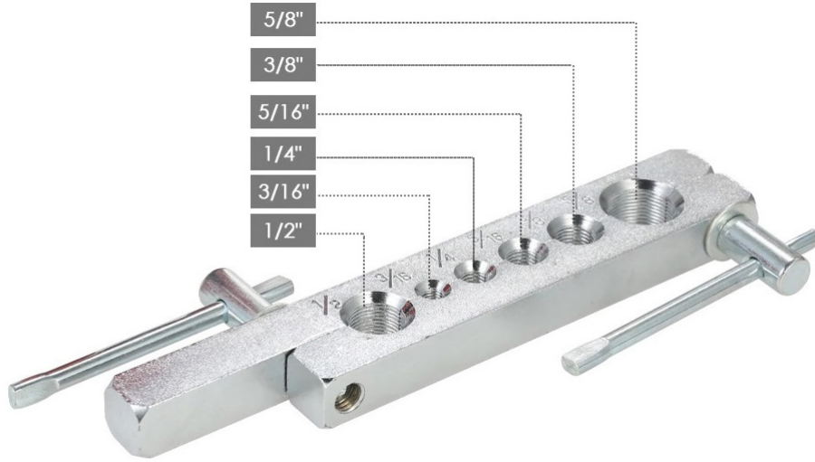
Görsel 6.17: Havşa mengesine uygun boru çapları
