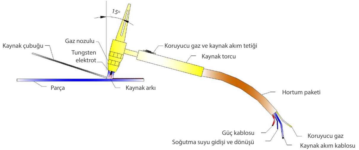
Görsel 13.1: TIG kaynak torcu kısımları
