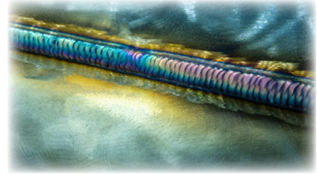
Görsel 13.20: Kaynak dikiş örneği
