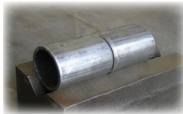
Görsel 12.26: Boruların puntalanmasında kullanılan V yatakları
