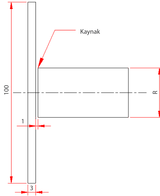
Görsel 12.22: Parçanın kaynağına hazırlanması
