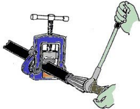
Görsel 4.8: Rayba ile çapak temizleme
