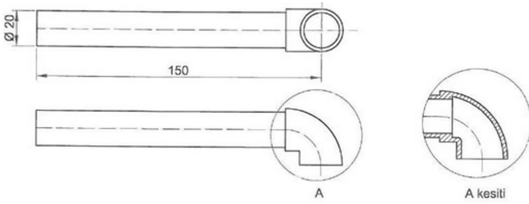
Görsel 5.9: Polipropilen boru kaynak işlemi için boru kesiti
