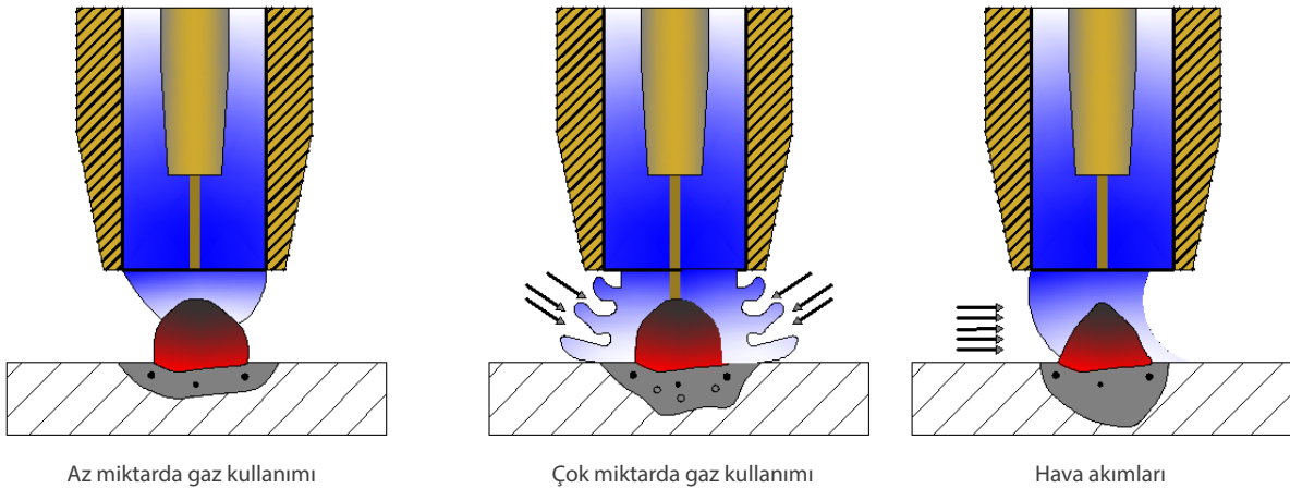
Görsel 12.18: Kaynak hatası oluşum sebepleri
