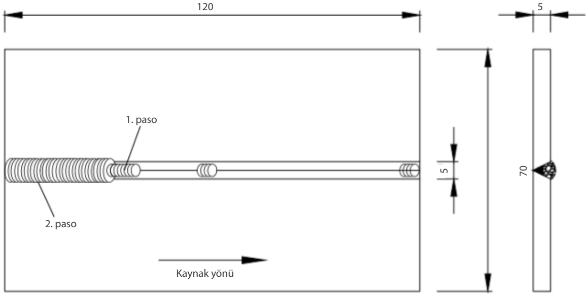
Görsel 9.8: Kaynak uygulaması
