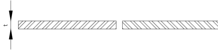
Kaynak ağzı açılmadan yapılan küt ek kaynaklı birleştirme
