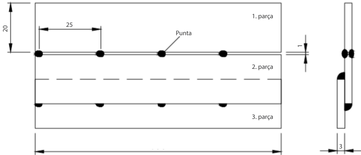
Görsel 11.3: Puntalama işlemi
