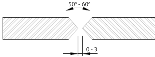
Çift taraflı açılmış X kaynak ağzı
