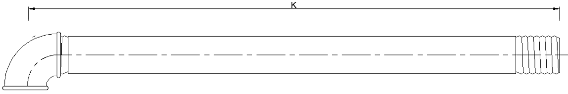
Görsel 4.28: Eksenden uca ölçü alma
