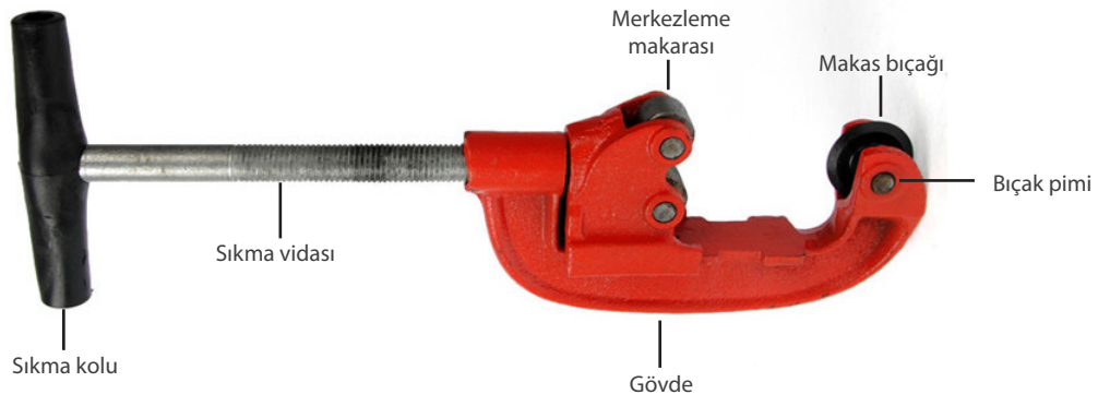
Görsel 4.5: Boru kesici kısımları
