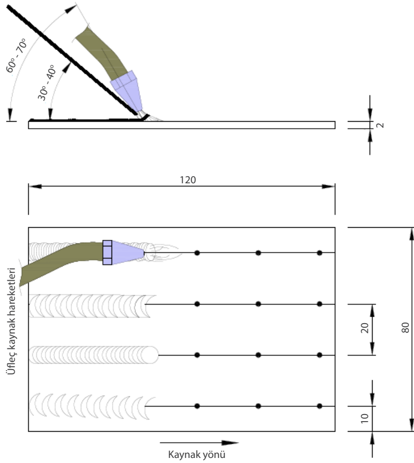
Görsel 9.6: Kaynak uygulaması
