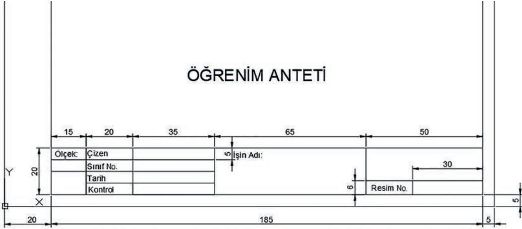
Görsel 2.14: Antet çizim örneği
