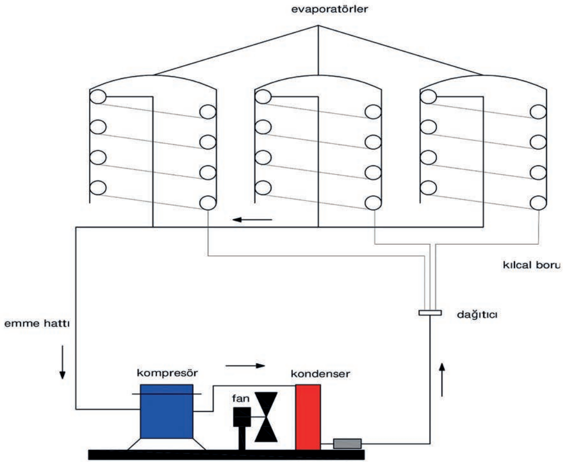
Görsel 3.7: Şerbetlik soğutma devre şeması
