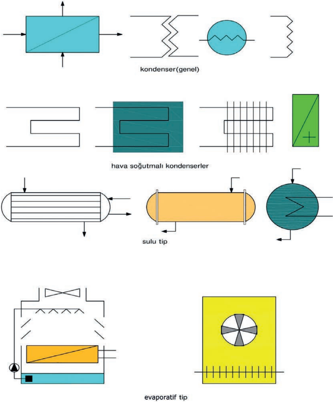
Görsel 3.2: Kondenser sembolleri
