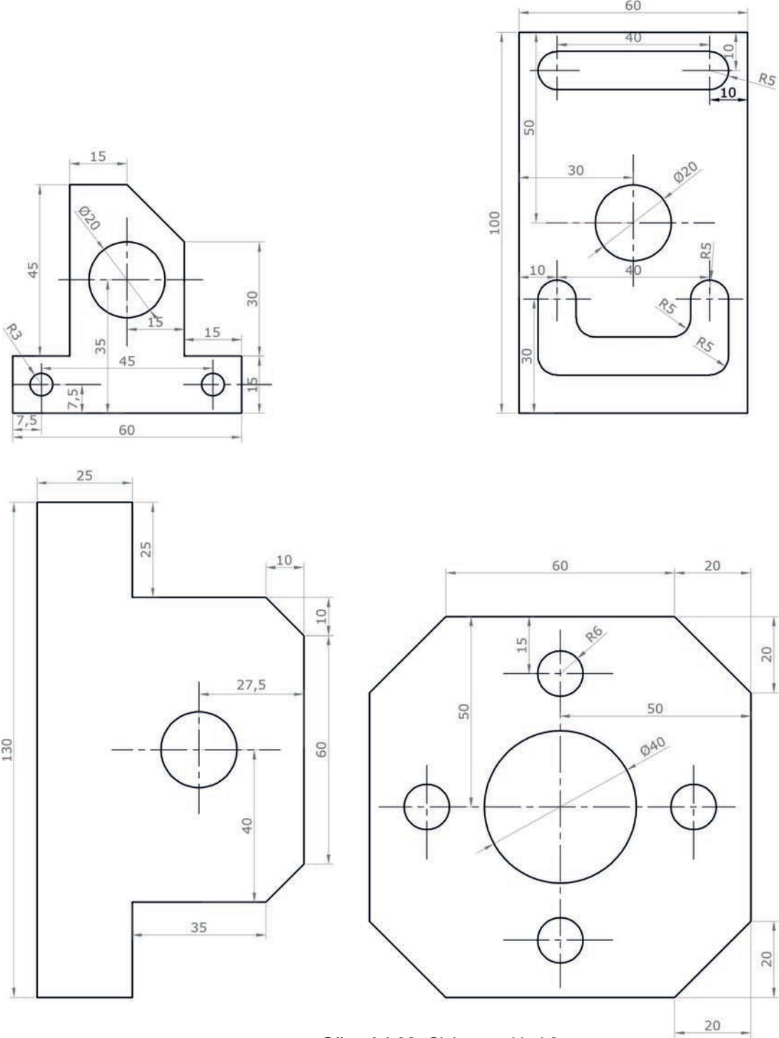
Görsel 1.92: Çizim örnekleri 2
