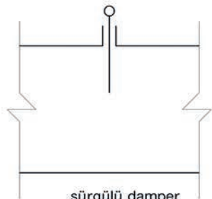
sürgülü damper
