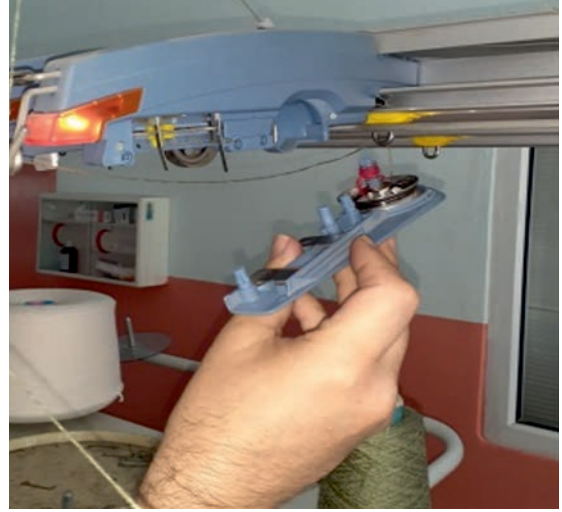
Görsel 5.8: Çardaktaki toz ve ipliklerin temizlenmesi
