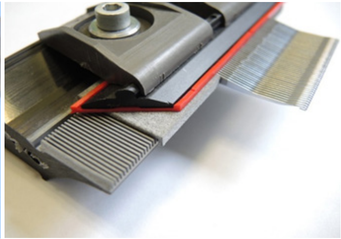
Görsel 1.21: Çözümlü örme makinelerinde kullanılan blok iğne rayları
