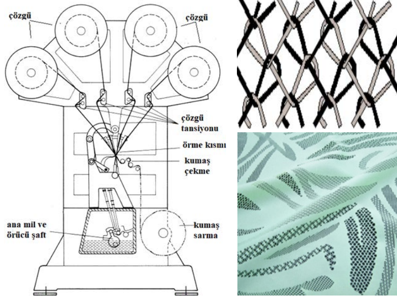
Görsel 1.55: Raşel çözümlü örme makinelerinde örme kısmı ve ilmek yapısı
