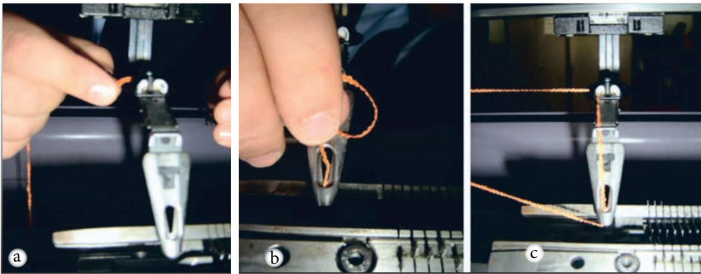
Görsel 2.17 (a, b, c): Düz örmeye ipliğin mekiklerden geçirilişi
