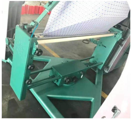
Görsel 1.51: Yuvarlak örme makinelerinde kumaş çekme ve sarma sistemi
