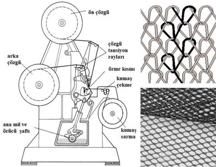
Görsel 1.54: Trikot çözgü örmek makinelerinde örmek kısmı ve ilmek yapısı
