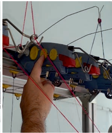
Görsel 5.7: Çardak düğüm algılayıcı ayarı
