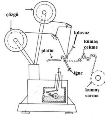
Görsel 1.56: Çözümlü örme makinelerinde kumaş çekme ve sarma sistemi
