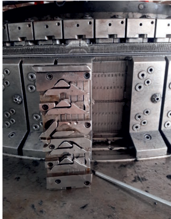
Görsel 3.4: Dört yollu çelik kanalı ve dört ayaklı iğnelerin olduğu sökümüş silindir plakası sistemi
