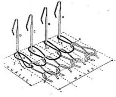
Görsel 1.36: İlmek oluşumu
