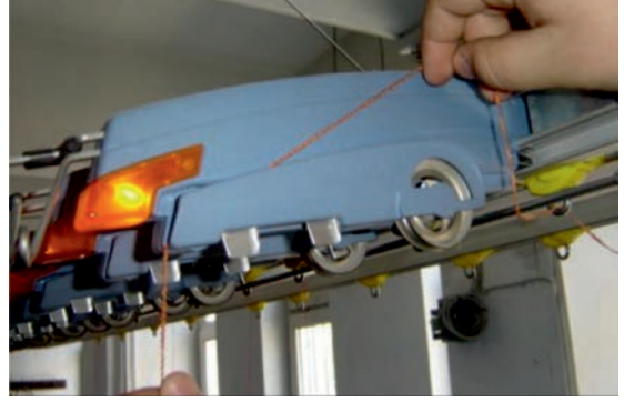
Görssel 2.8: Üst çardaktan ipliğin geçirilişi
