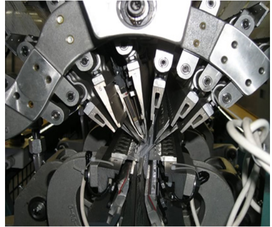
Görsel 1.42: İğne rayları
