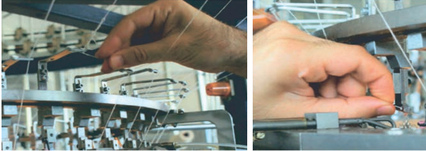
Görsel 2.16: Yuvarlak örmeye ipliğin mekiklerden geçirilişi
