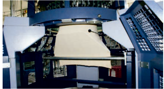
Görssel 2.10: Yuvarlak örme makinesinde kumaş çekme sistemi
