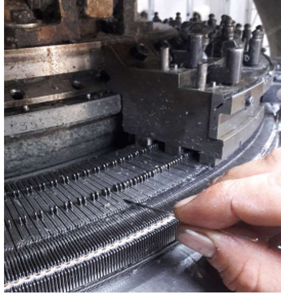
Görsel 3.3: İki ayaklı kapak plaka iğnelerinin 1x1 olarak elle dizimi
