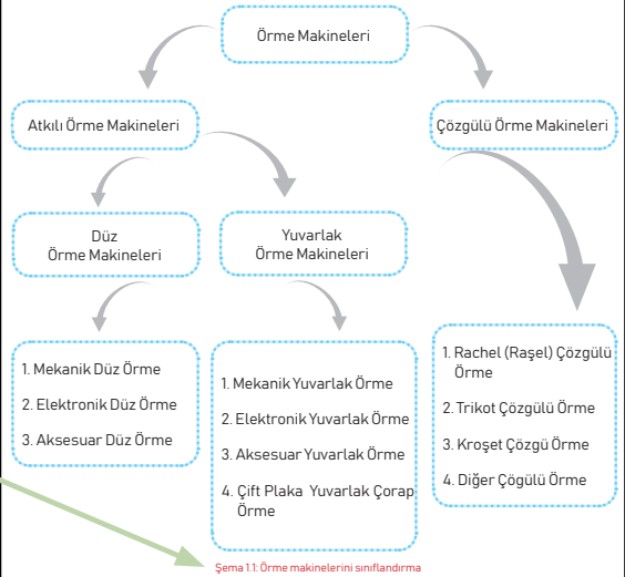
Şema 1.1. Örme makinelerini sınıflandırma
