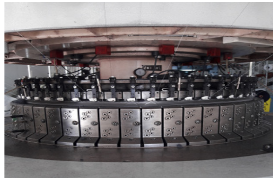
Görsel 3.1: Mekanik çift plakalı yuvarlak örme makinesi örücü elemanları
