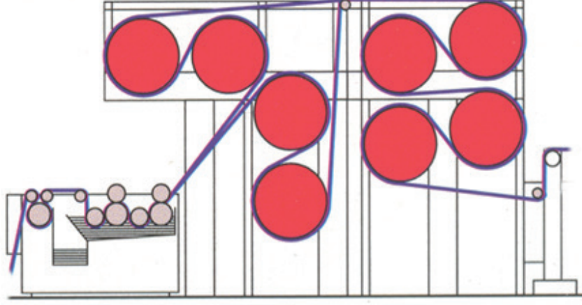
Görsel 2.10: Silindirli kurutma
