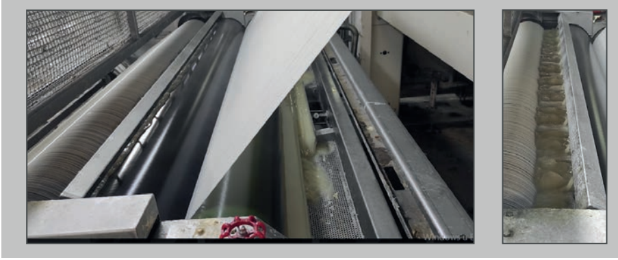
Görsel 2.9: Haşıl teknesi ve sıkma silindirleri
