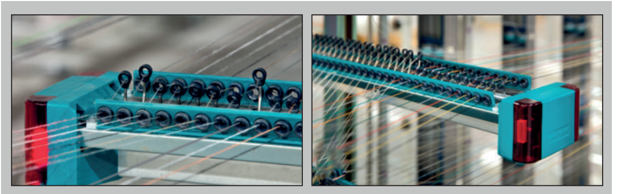
Görsel 1.9: İplik yoklayıcılar
