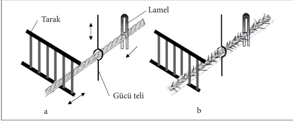
Görsel 2.1: Dokuma işleminde çözgü ipliklerinin konumu
