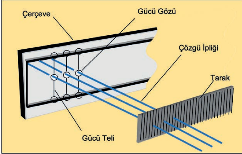
Görsel 3.1: Tahar işlemi
