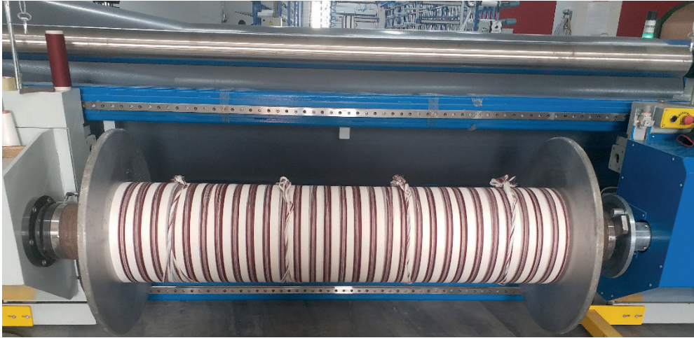
Görsel 1.58: Hazırlanmış çözügü leventi
