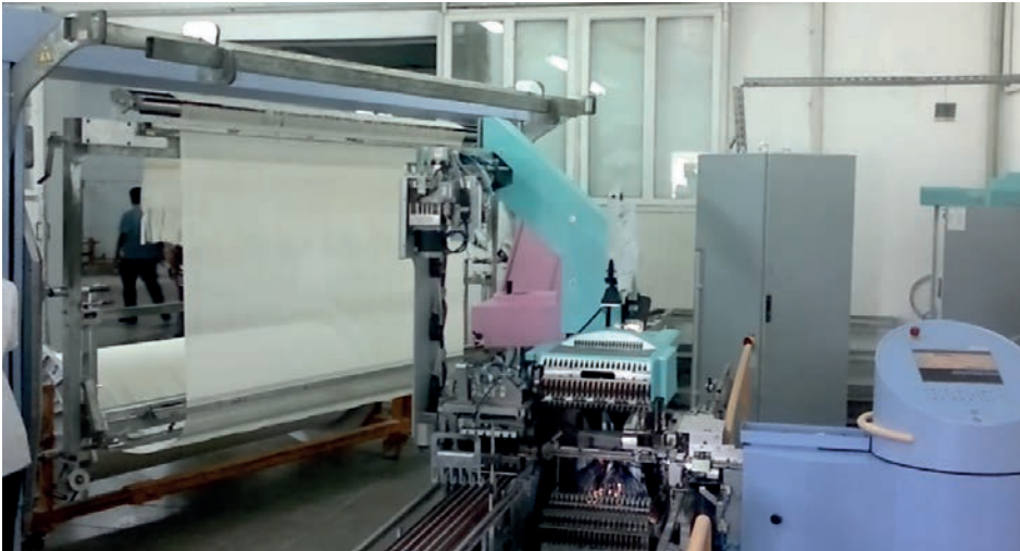
Görsel 3.16: İplik bölümü
