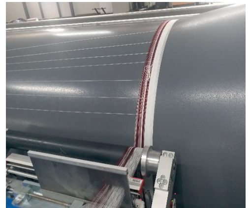
Görsel 1.45: Çapraz ipliklerinin tambura bağlanması
