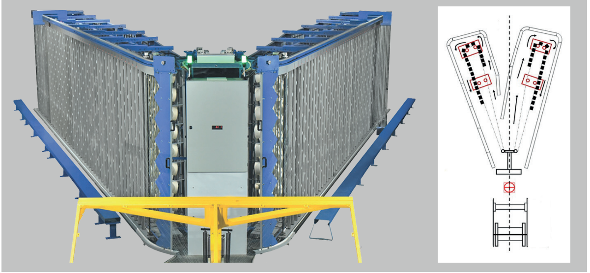
Görsel 1.74: V çağlık ve şematik gösterim
