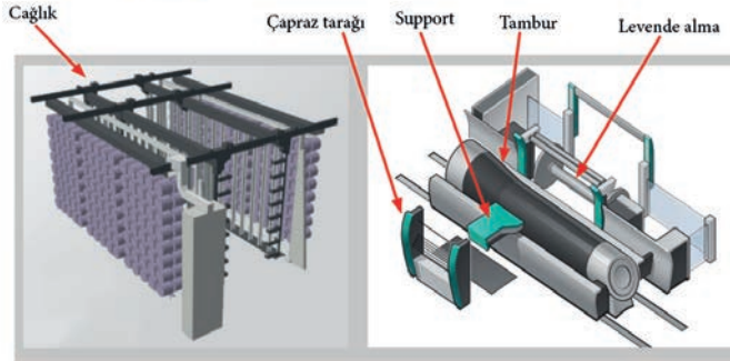
Görsel 1.3: Konik çözgü makinesi ana elemanları
