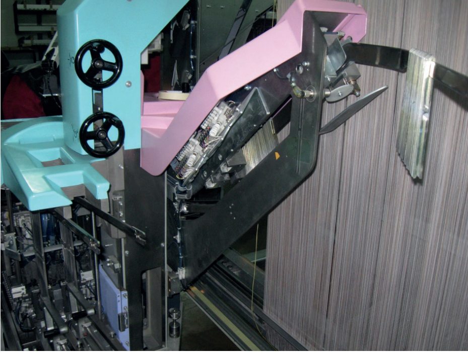
Görsel 3.15: Lamel bölümü
