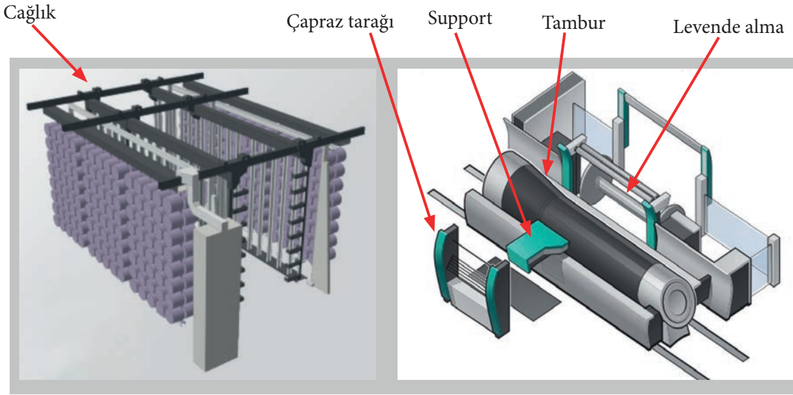
Görsel 1.3: Konik çözü makinesi ana elemanları
