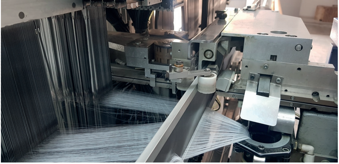
Görsel 3.21: Tahar işleminin yandan görünüşü
