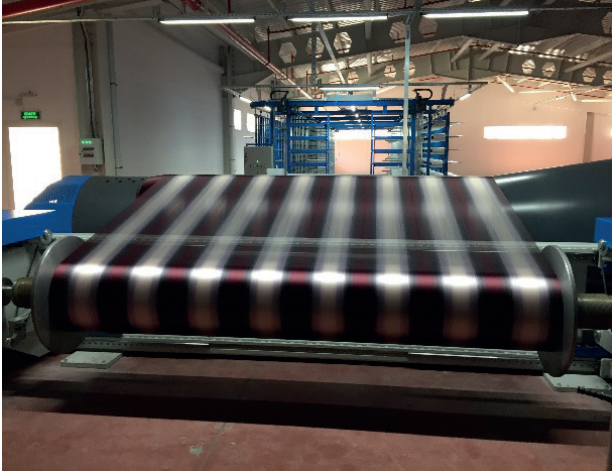
Görsel 1.23: Levende alma kısmı
