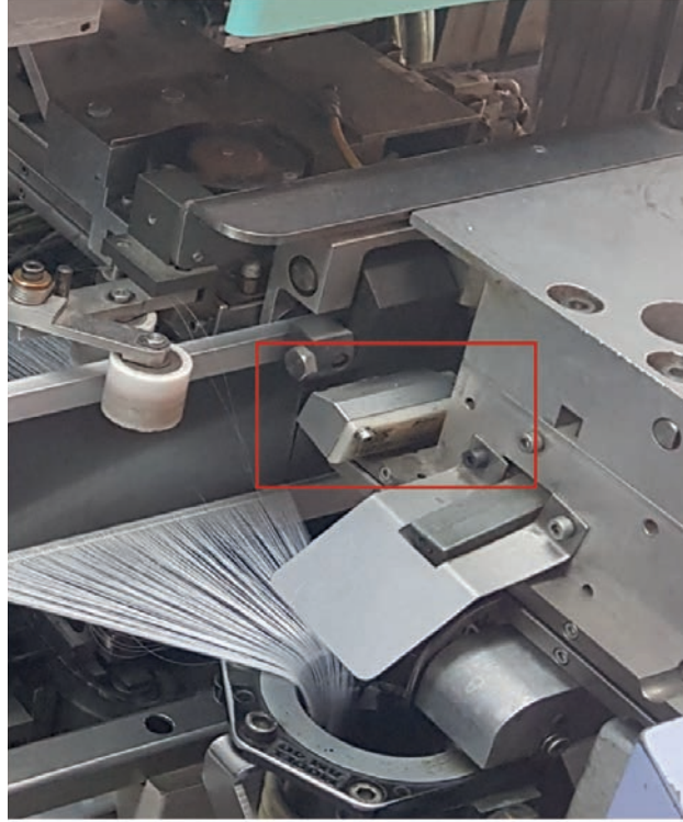
Görsel 3.28: Tarak bıçağı ve tarak görücü
