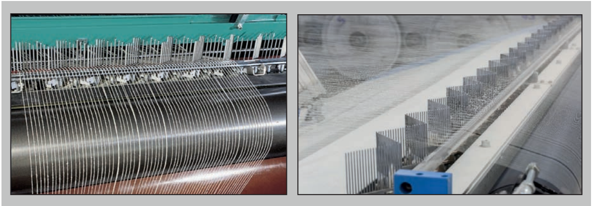
Görsel 1.75: Toplama tarağı
