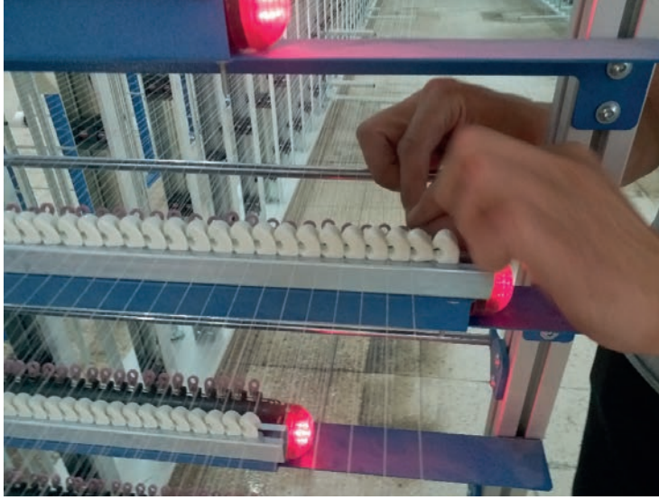
Görsel 1.83: İpliklerin yoklayıcılardan alınması
