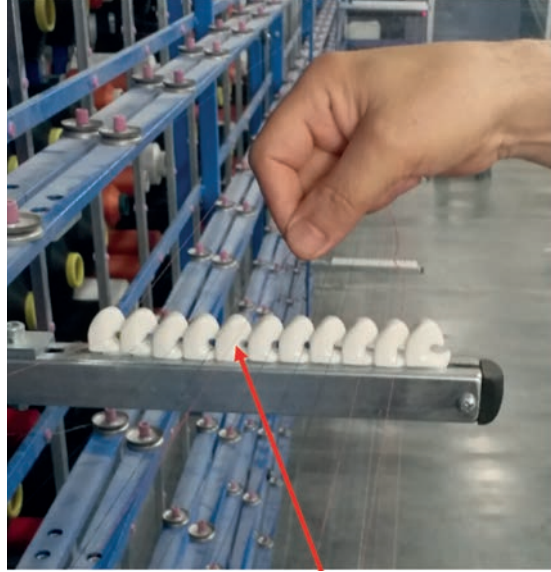
Görsel 1.31: İpliklerin tutuculardan geçirilmesi
