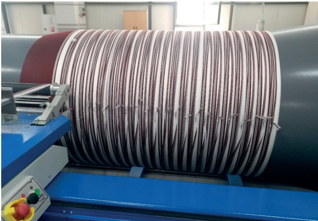
Görsel 1.47: Kalbaların tambura sarılması
