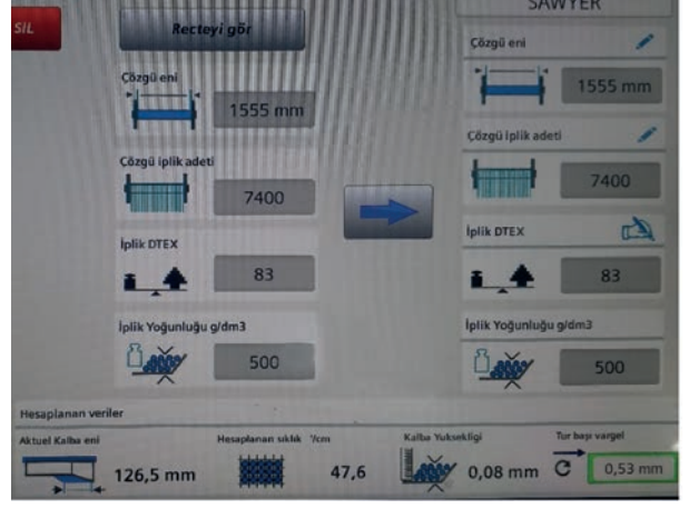
Görsel 1.70: İş talimatındaki verilerin girildiği bölüm
