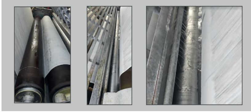
Görsel 2.49: Haşıl teknesinin yıkanması
