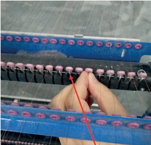
Görsel 1.32: İpliklerin yoklayıcılardan geçirilmesi
