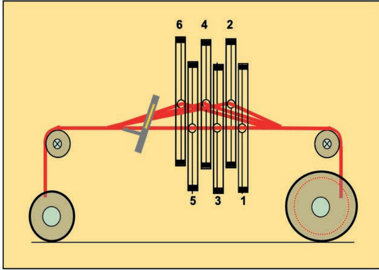
Görsel 3.4: Dokuma taraklarının numaralandırılması
