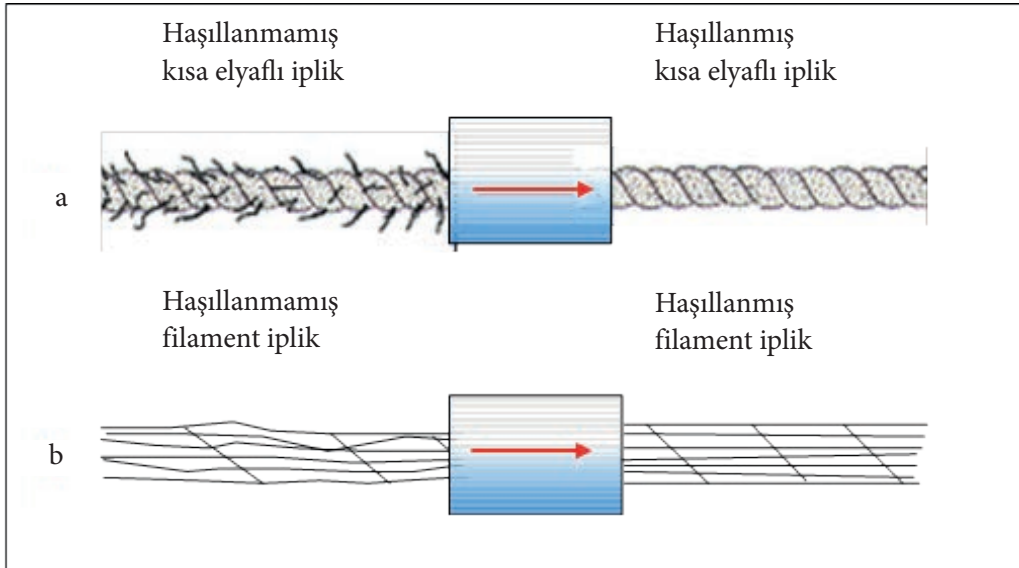
Görsel 2.2: Haşılı ve haşılsız iplik çizim gösterimi
