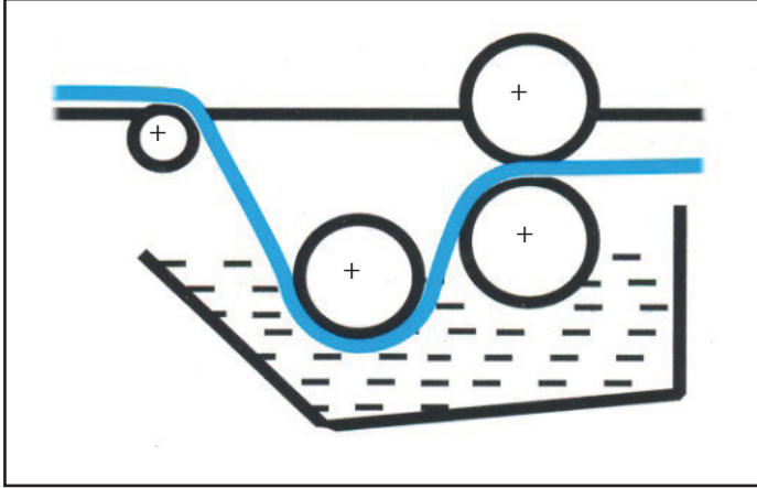
Görsel 2.7: Daldırma tekniğiyle haşılama
