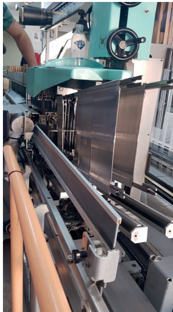
Görsel 3.29: Tarak kızağı yolu
