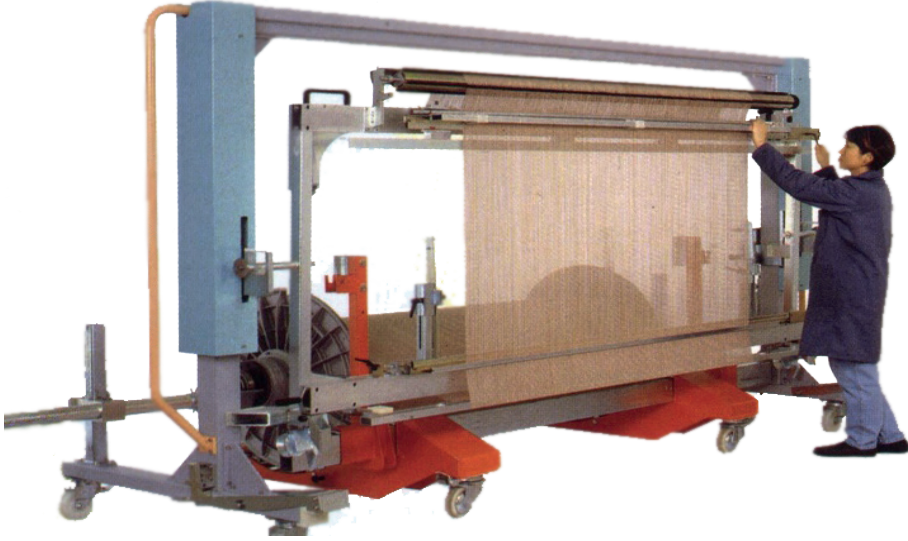
Görsel 3.11: Tahar sehpası ve tahar makinesine çözgü hazırlama
