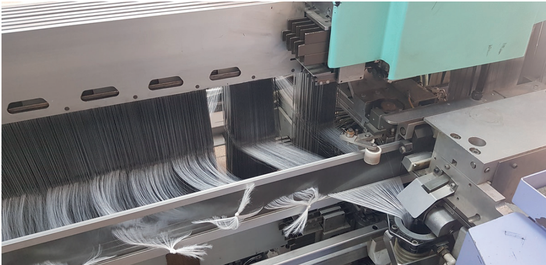
Görsel 3.20: Tahar işlemi
