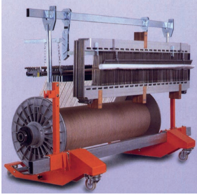
Görsel 3.23: Tahar nakil arabası
