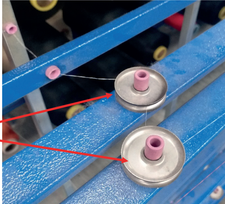
Görsel 1.63: Frenleme aparatları
