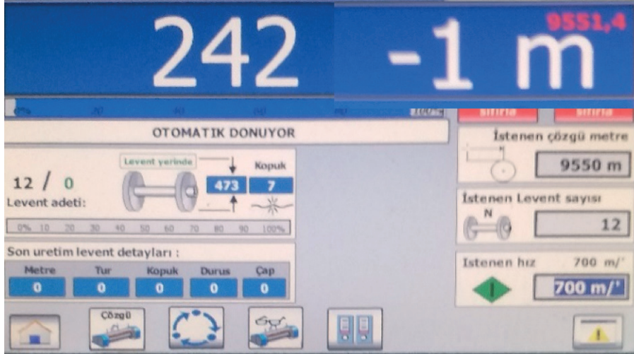
Görsel 1.96: Kumanda paneli
