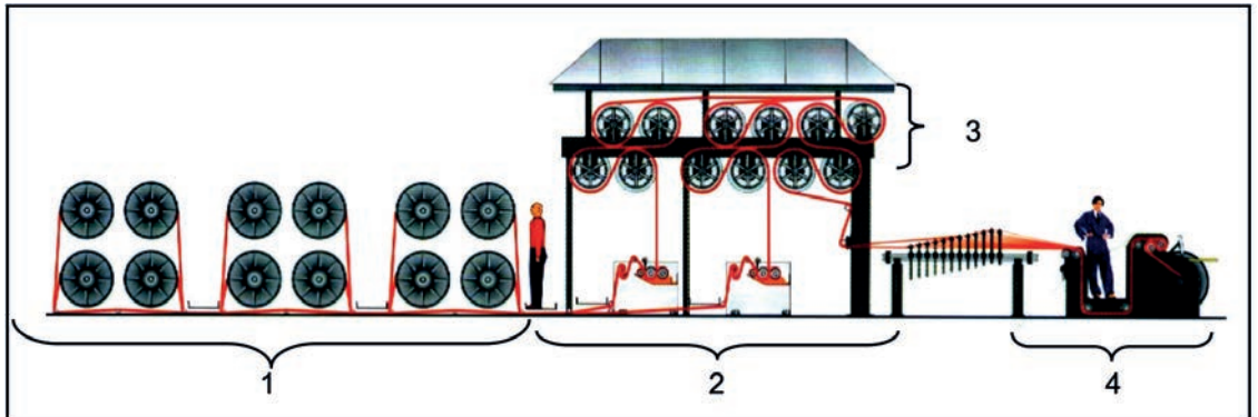
Görsel 2.4: Haşıl makinesinin genel görünüşü
