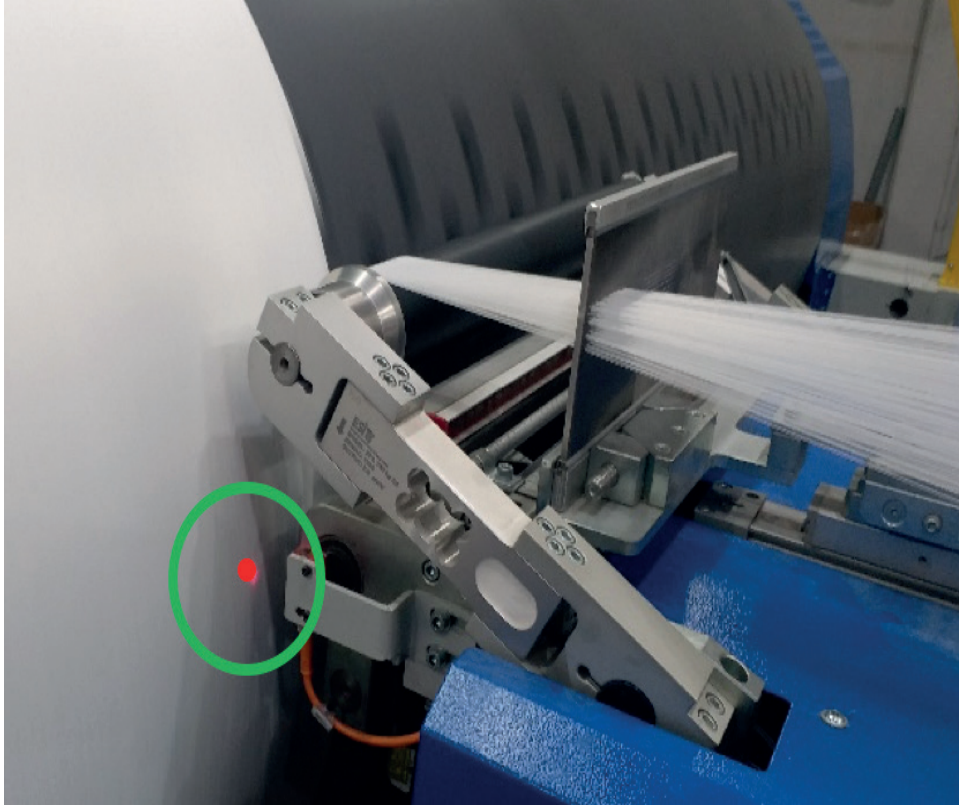
Görsel 1.68: Lazer ölçüm sensörü
