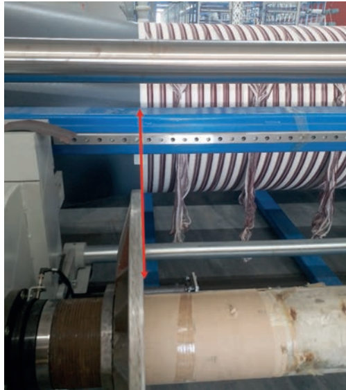
Görsel 1.53: Levendin başlangıç hizalaması
