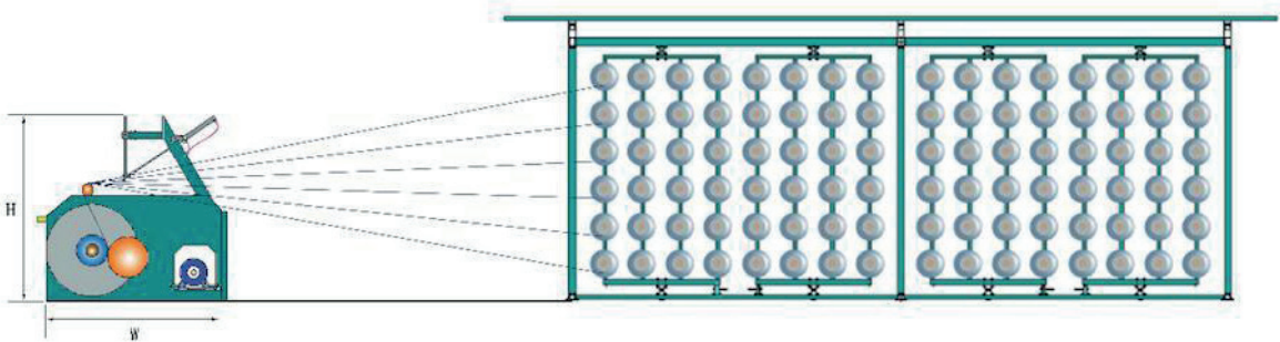
Görsel 1.73: Seri çözgü makinesinin şematik gösterimi
