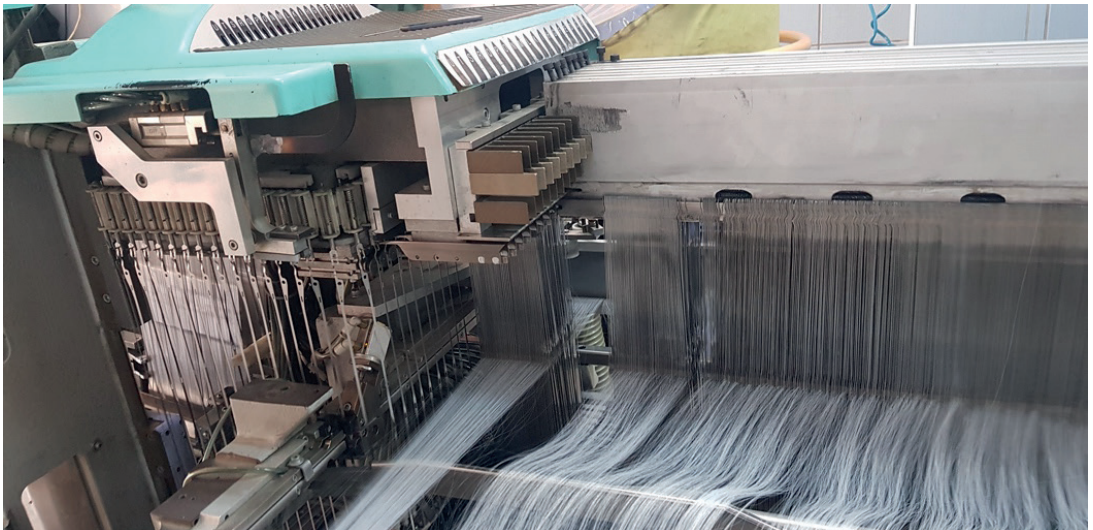
Görsel 3.14: Gücü sevk bölümü
