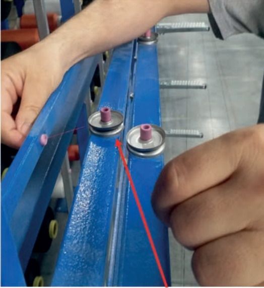
Görsel 1.30: İpliklerin frenlerden geçirilmesi
