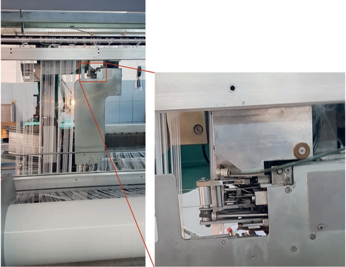
Görsel 3.25: İplik ayırıcı bölümün arkadan görünüşü
