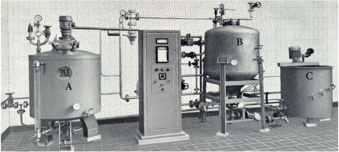
Görsel 2.21: Haşıl pişirme aparatı
