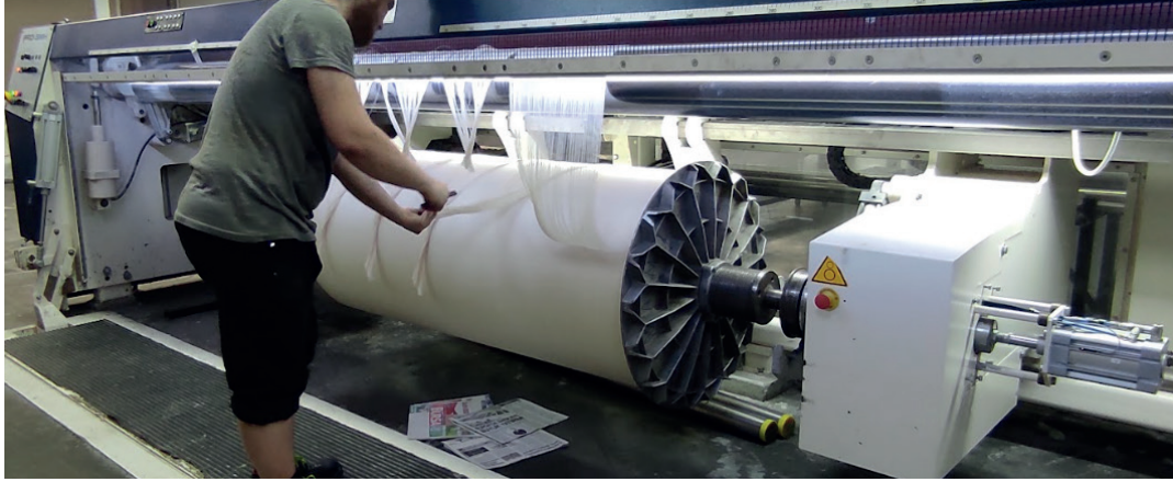
Görsel 2.42: Çözülerin kesilmesi
