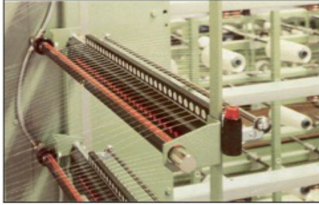
Görsel 1.10: İplik yoklayıcı grubu ve bu gruba ait uyarı lambası
