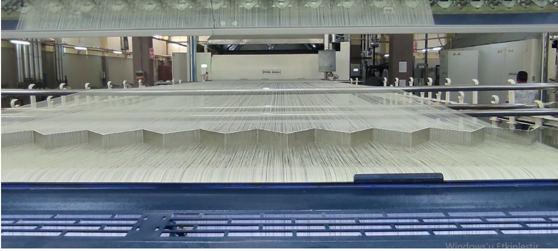
Görsel 2.16: Haşıl tarağı
