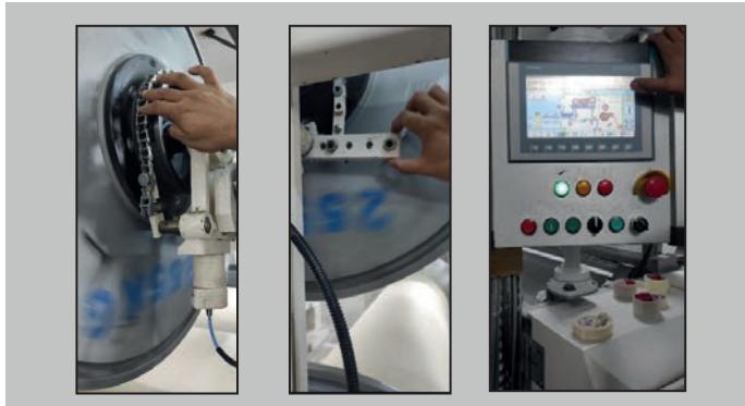
Görsel 2.48: Kısmi levent besleme sisteminde fren ayarlarının yapılması
