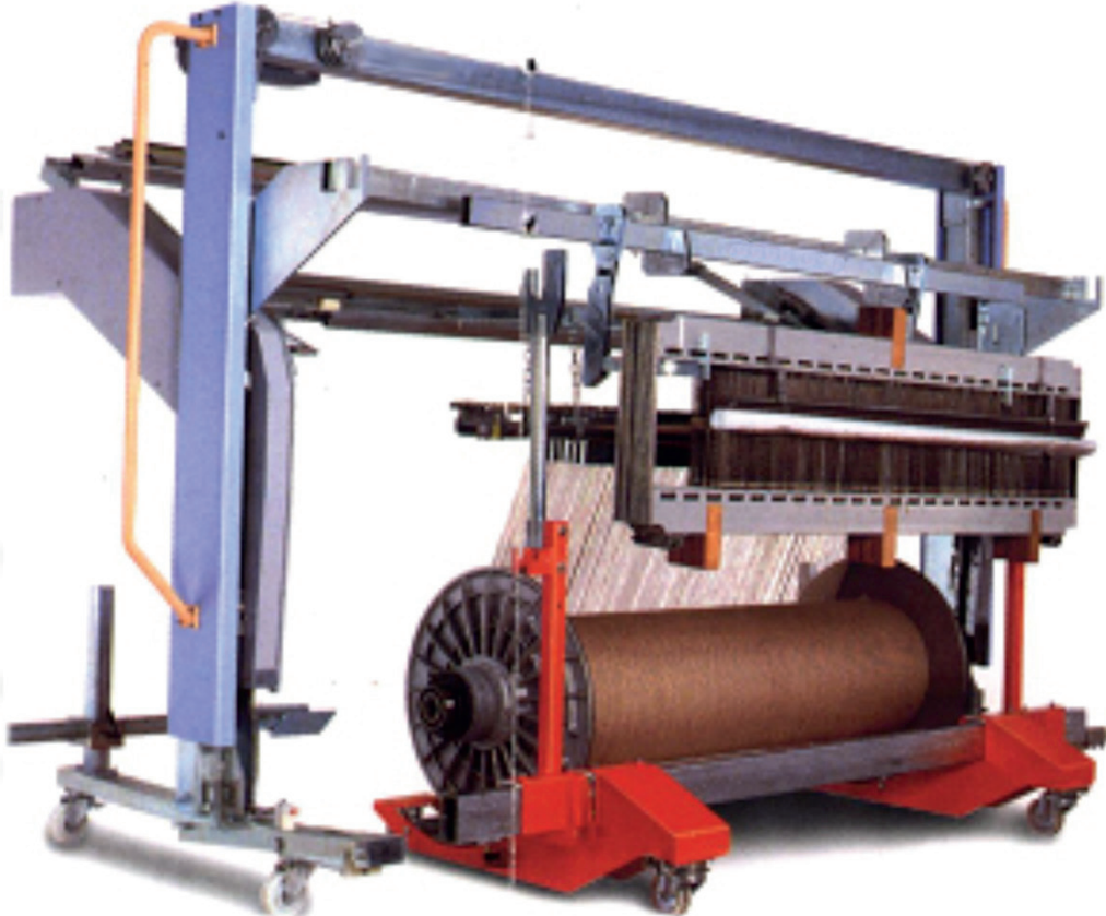
Görsel 3.22: Çözümlerin tahar nakil arabasına alınması
