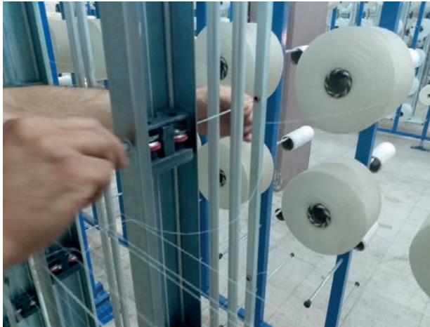
Görsel 1.81: İpliklerin fren tertibatından alınması
