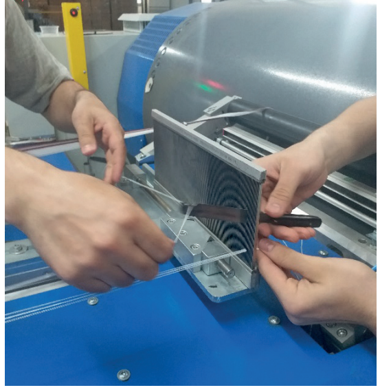
Görsel 1.39: Çözgülerin toplama tarağından geçirilmesi
