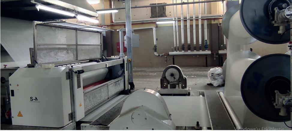
Görsel 2.22: Haşıl makinesi ön kısmı
