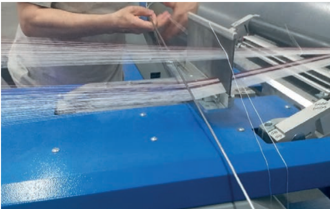
Görsel 1.44: Çapraz işleminin yapılması
