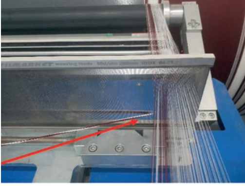
Görsel 1.48: Fazla çözgülerin iptal edilmesi
