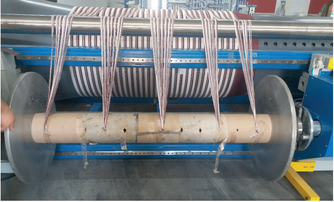
Görsel 1.54: Çözgü uçlarının dokuma levendine bağlanması
