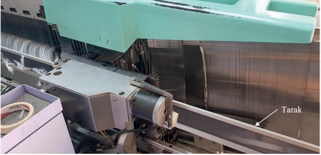
Görsel 3.17: Tarak bölümü
