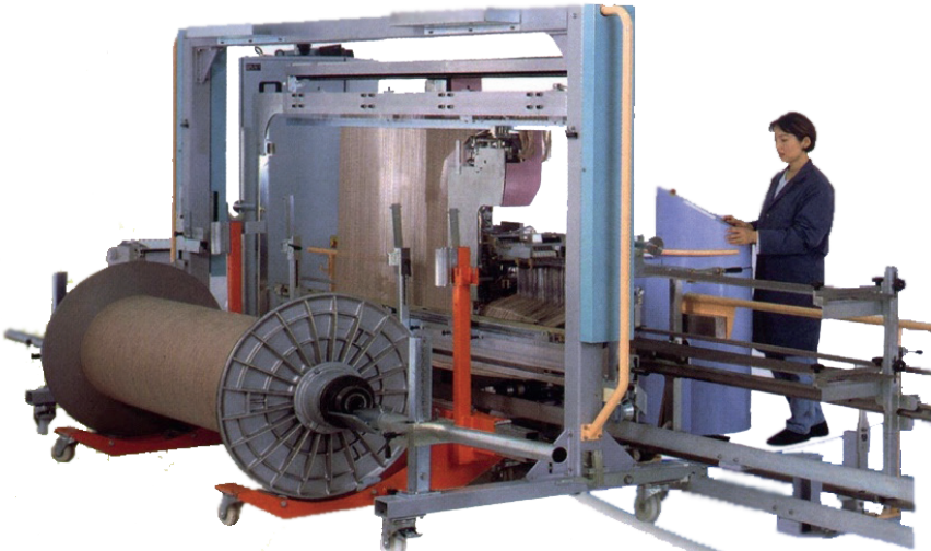
Görsel 3.12: Tahar makinesine çözgü yerleştirme
