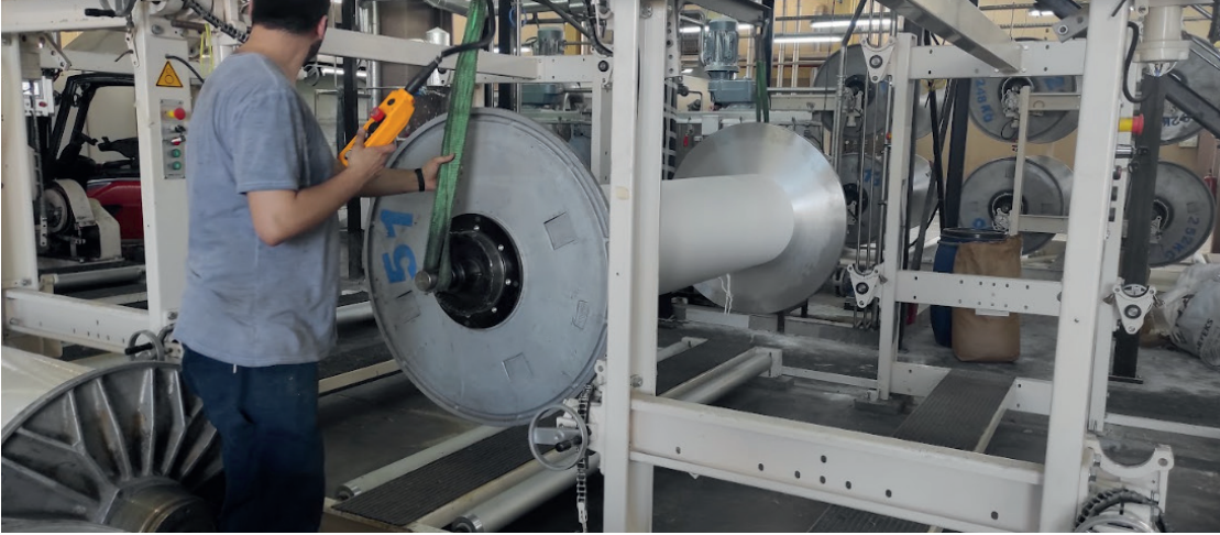
Görsel 2.30: Kısmi levent besleme sisteminde leventin haşıl sehpasına taşınması
