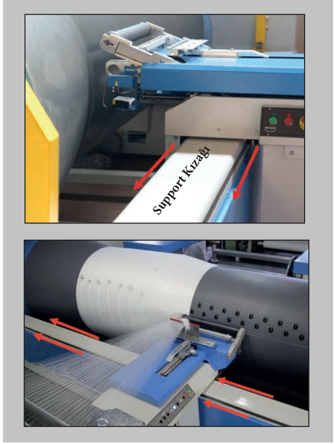
Görsel 1.21: Support kızağı
