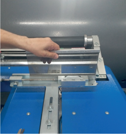
Görsel 1.38: Toplama tarağının takılması
