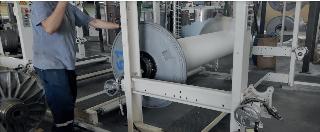
Görsel 2.31: Kısmi levent besleme sisteminde leventin haşıl sehpasına takılması
