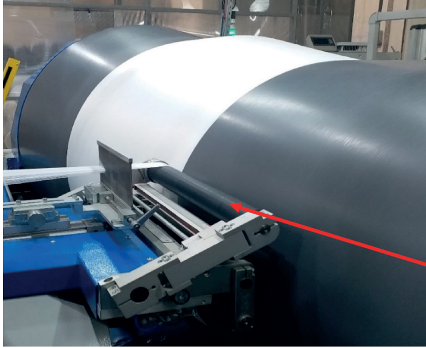
Görsel 1.19: Kılavuz silindir
