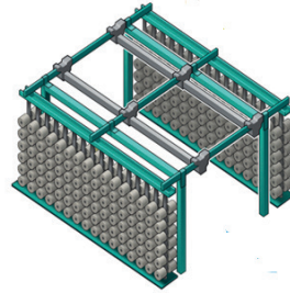
Görsel 1.5: Paralel çağlık
