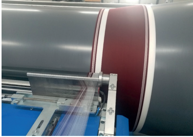
Görsel 1.46: Kalbaların tambura sarılması
