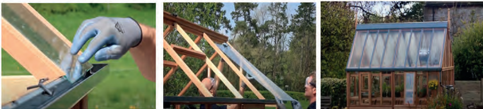
Görsel 4.12: Seranın camla kaplanması
