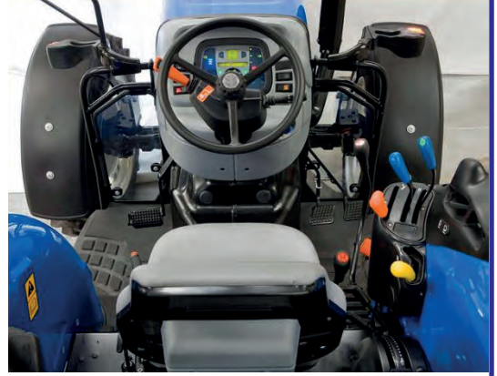
Görsel 9.38: Traktörün sevk ve idaresinde kullanılan kol ve cihazlar
