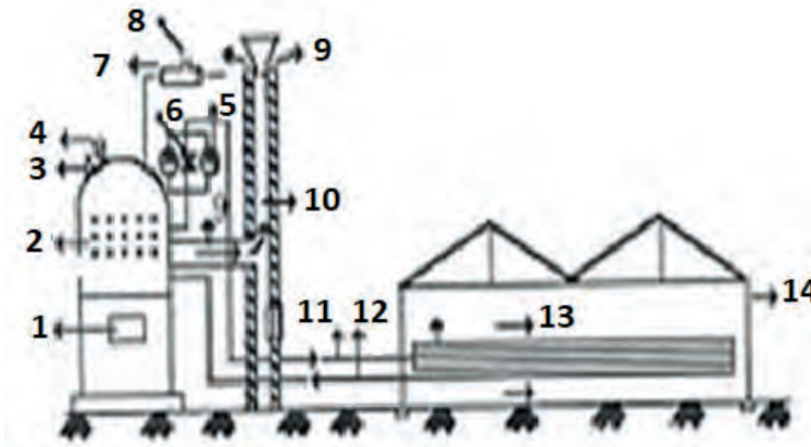
Görsel 4.22: Sera kalorifer sistemi
