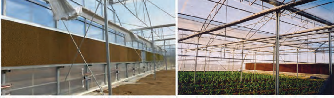
Görsel 4.28: Soğutma yastıklarıyla soğutma
