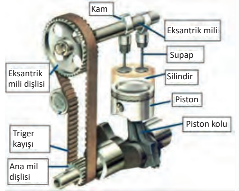
Görsel 9.12: Eksantrik mili
