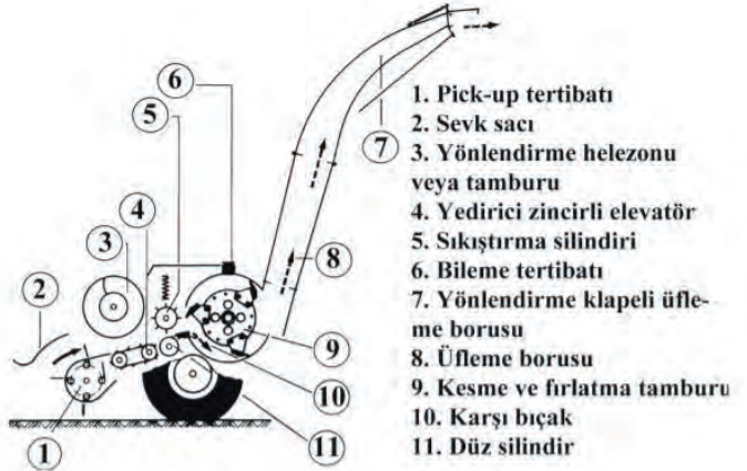
Şekil 6.47: Tamburlu bıçaklı silaj makinelerinin parçaları
