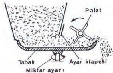
Şekil 6.12: Sandıklı gübre dağıtma makinelerinin parçaları
