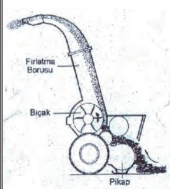
Şekil 6.42: Tamburlu bıçaklı silaj makinesi
