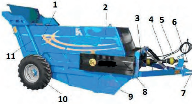
Şekil 6.1: Taş toplama makinesinin parçaları
