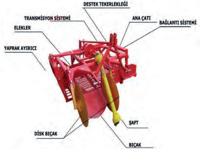
Görsel 6.123: Patates hasat makinesinin parçaları
