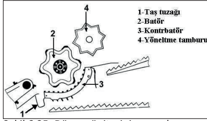
Şekil 6.35: Dövme ünitesinin parçaları
