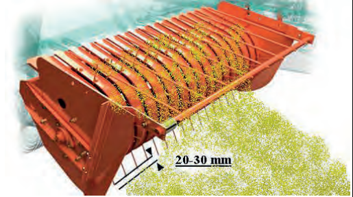
Görsel 6.110: Pikap yüksekliği
