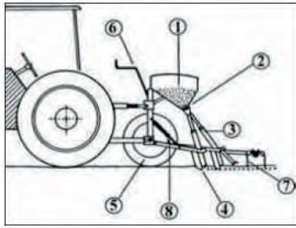
Görsel 6.51: Mekanik hububat dane ekim makinesinin parçaları
