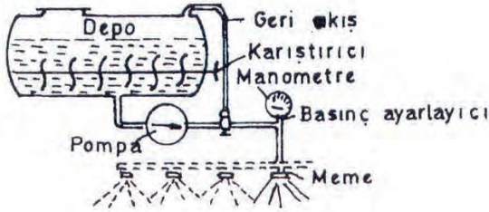
Şekil 6.24: Pülverizatörün çalışması
