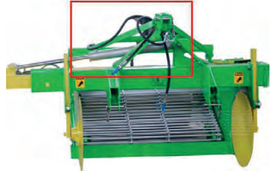
Görsel 6.118: Çalışma derinlik ayarı
