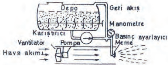
Şekil 6.25: Atomizörün çalışması
