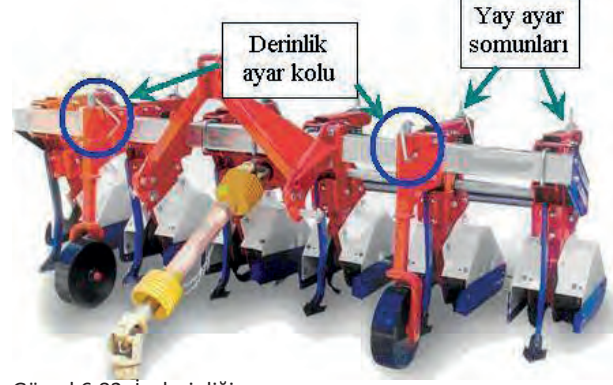
Görsel 6.82: İş derinliği ayarı
