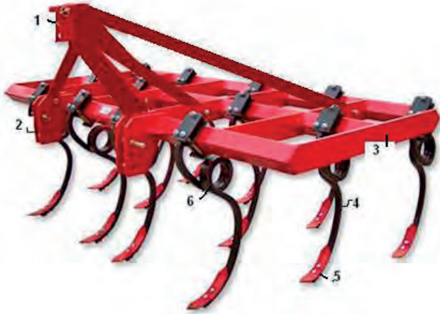
Görsel 6.33: Kültivatörün parçaları
