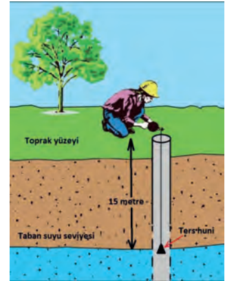
Şekil 3.2: Mekanik ses yöntemi ile ölçüm yapma
