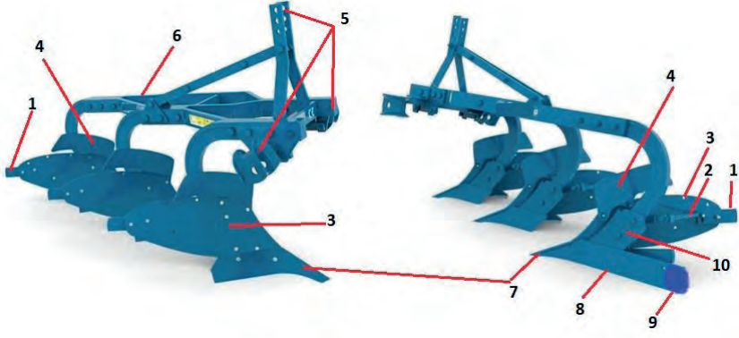
Görsel 6.28: Kulaklı pulluğun parçaları
