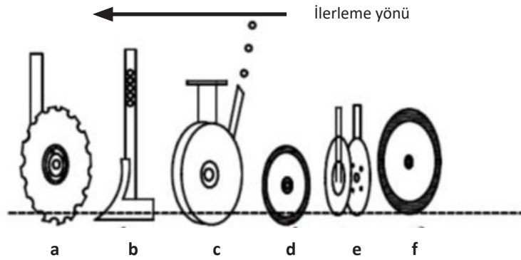
Görsel 2.29: Anıza ekim makinesinin makine üzerindeki dizilişi
