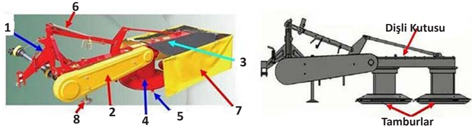
Görsel 3.7: Tamburlu çayır biçme makinesinin parçaları
