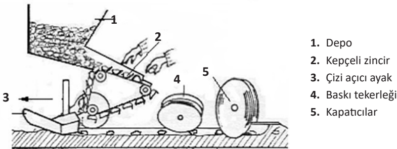
Görsel 2.37: Kepçeli zincirli patates dikim makinesi
