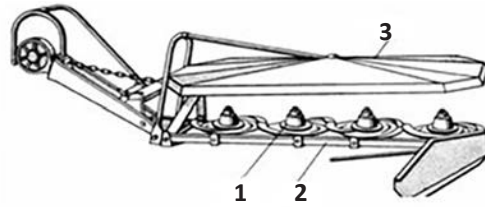
Görsel 3.8: Diskli çayır biçme makinesinin parçaları
