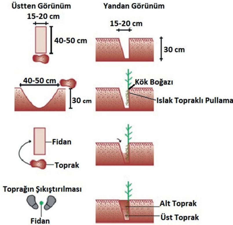
Görsel 1.27: Çukurda kenar dikimi
