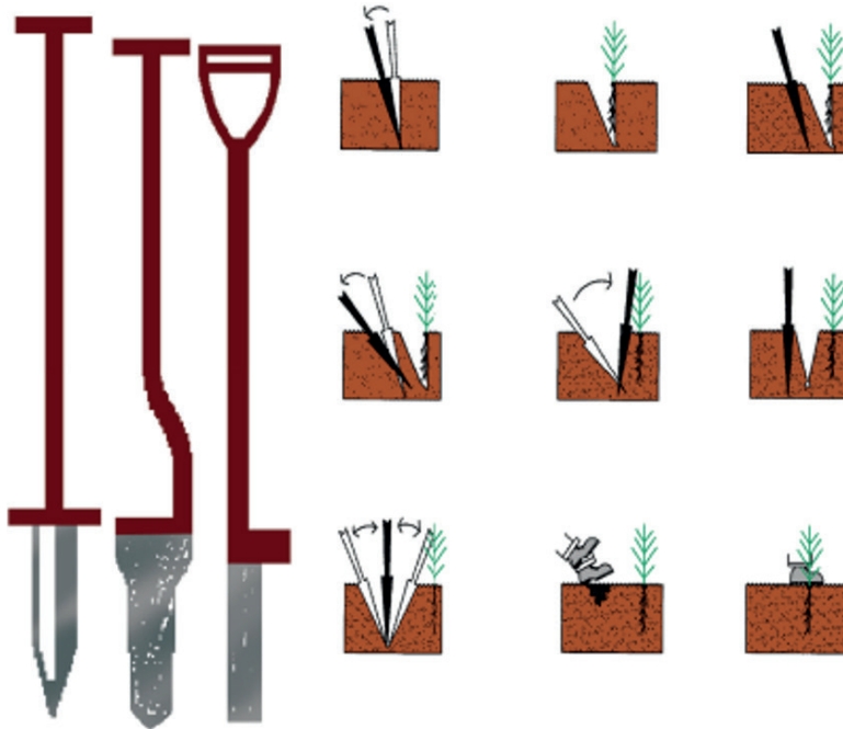
Görsel 1.26: Görsel plantuvar modelleri ve plantuvar dikimi şekilleri
