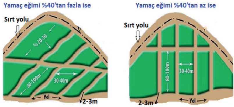
Görsel 3.9: Genç meşcere bakım patikaları
