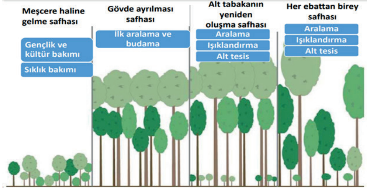
Görsel 3.3: Ormanda gelişme çağlarına uygulanacak bakım tedbirleri
