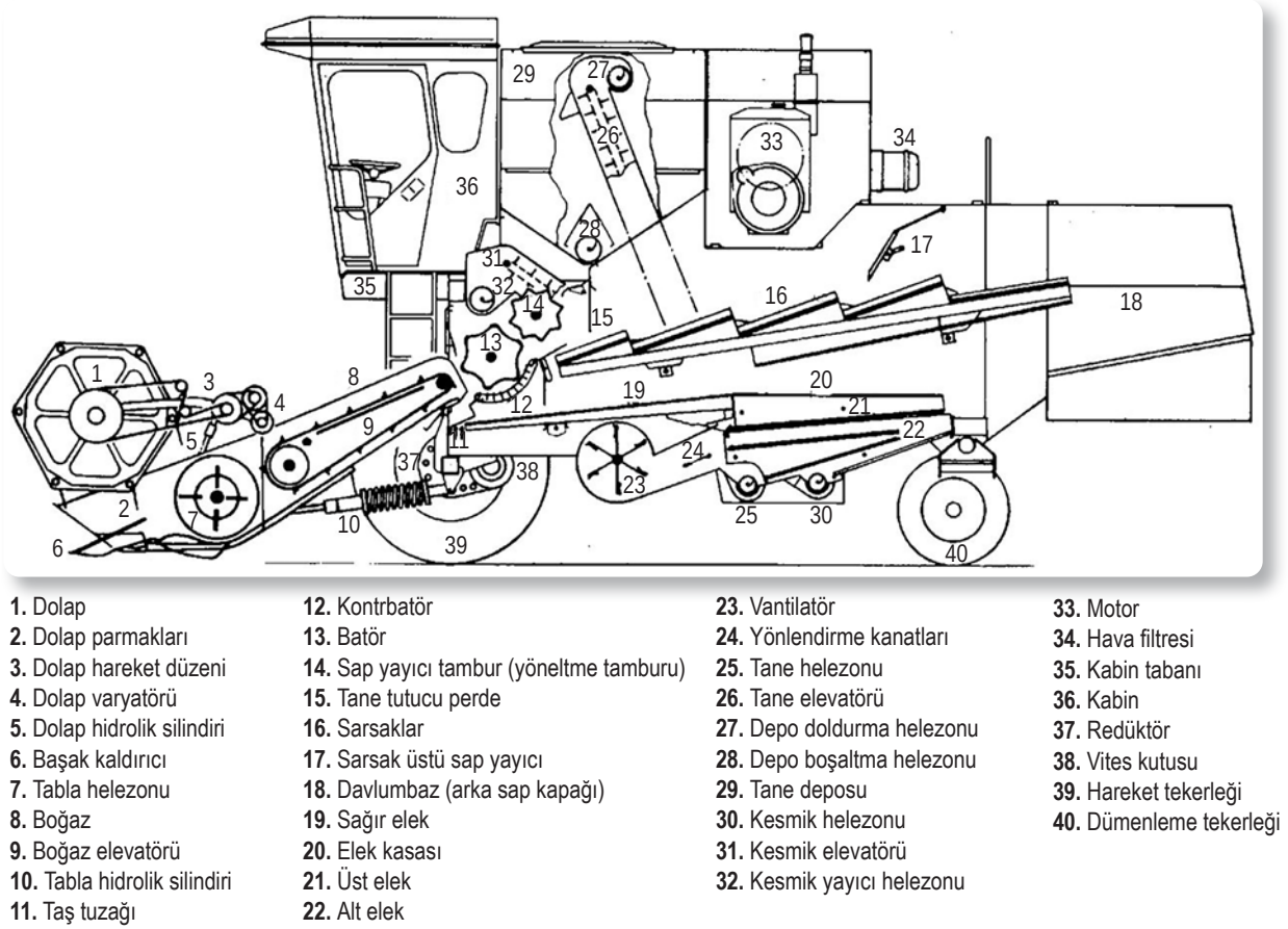
Görsel 1.1: Bıçerdöverin parçaları
