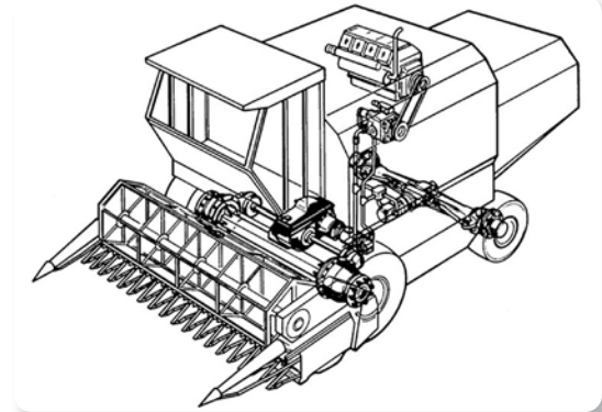
Görsel 1.2: Biçerdöverde hidrostatik güç iletimi
