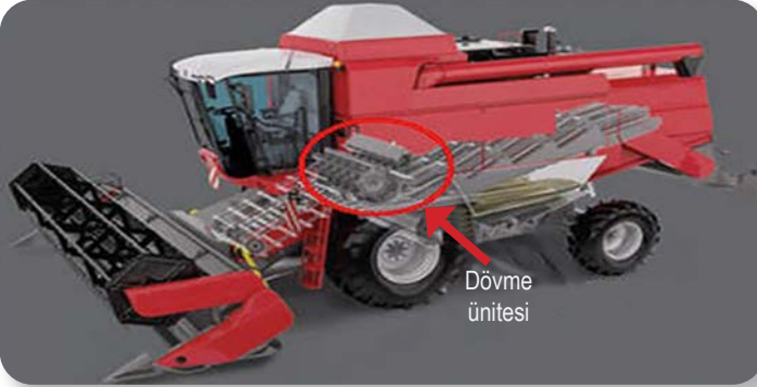
Görsel 1.16: Teğetsel akışlı biçerdöver
