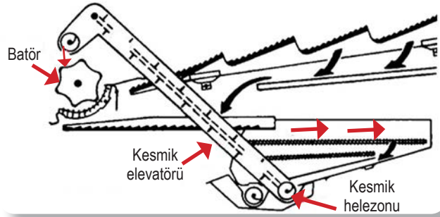
Görsel 1.41: Keskik elevatörünün çalışması
