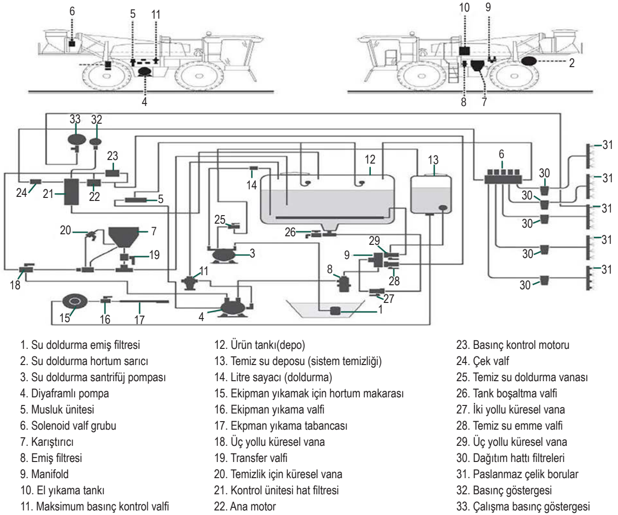
Görsel 3.5: Kendi yürür bitki koruma makinesinin ilaçlama ünitesi parçaları
