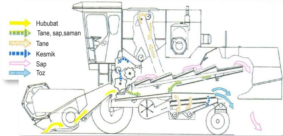
Görsel 1.5: Bıçerdöverin çalışma prensibi
