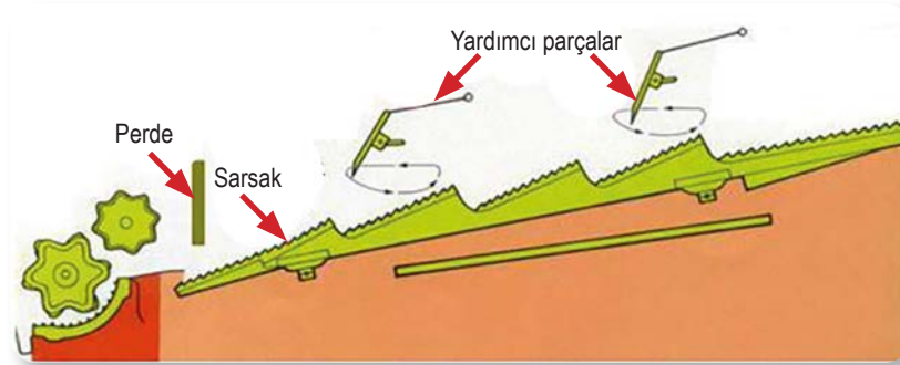
Görsel 1.25: Biçerdöverin ayırma ünitesinin parçaları
