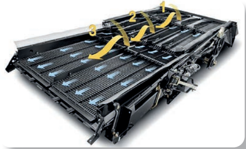
Görsel 1.33: Üst elek ve uzantısı
