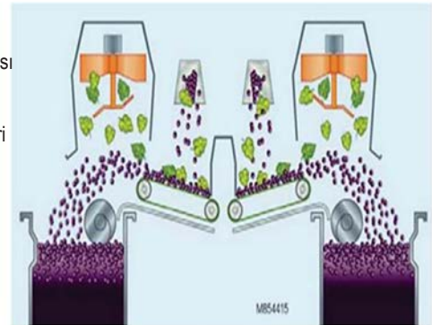
Görsel 2.19: Ürün iletim, depolama ve boşaltma üniteleri
