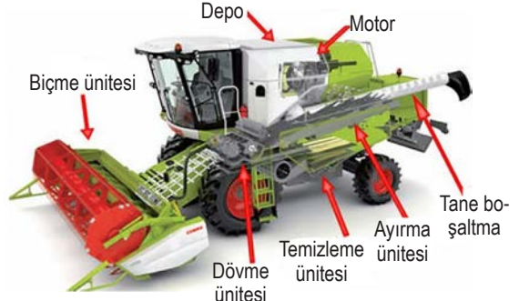
Görsel 1.4: Bıçerdöverin ana üniteleri/düzenleri
