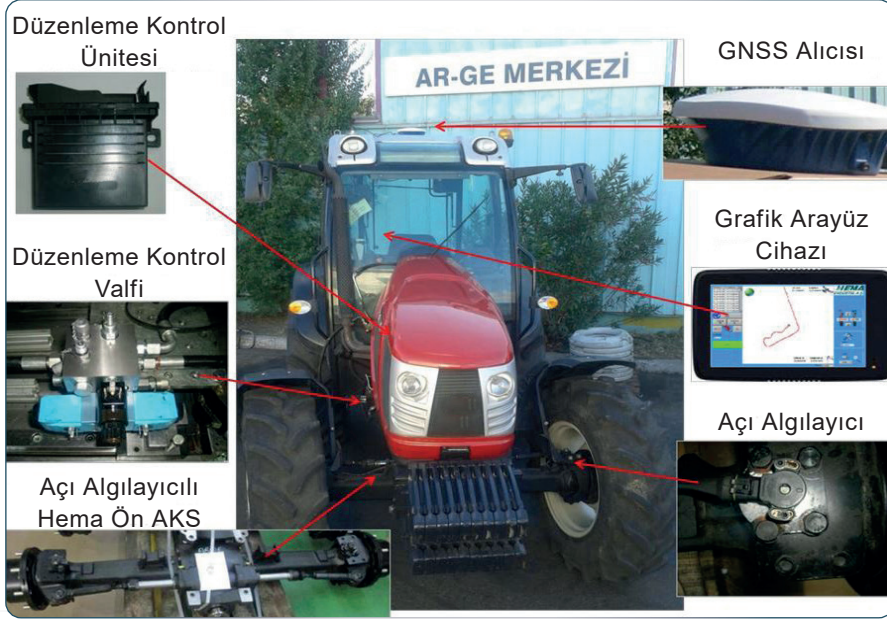
Görsel 3.17: Otomatik dümenleme sisteminin oluşturulan elemanların traktör üzerindeki yerleşimi
