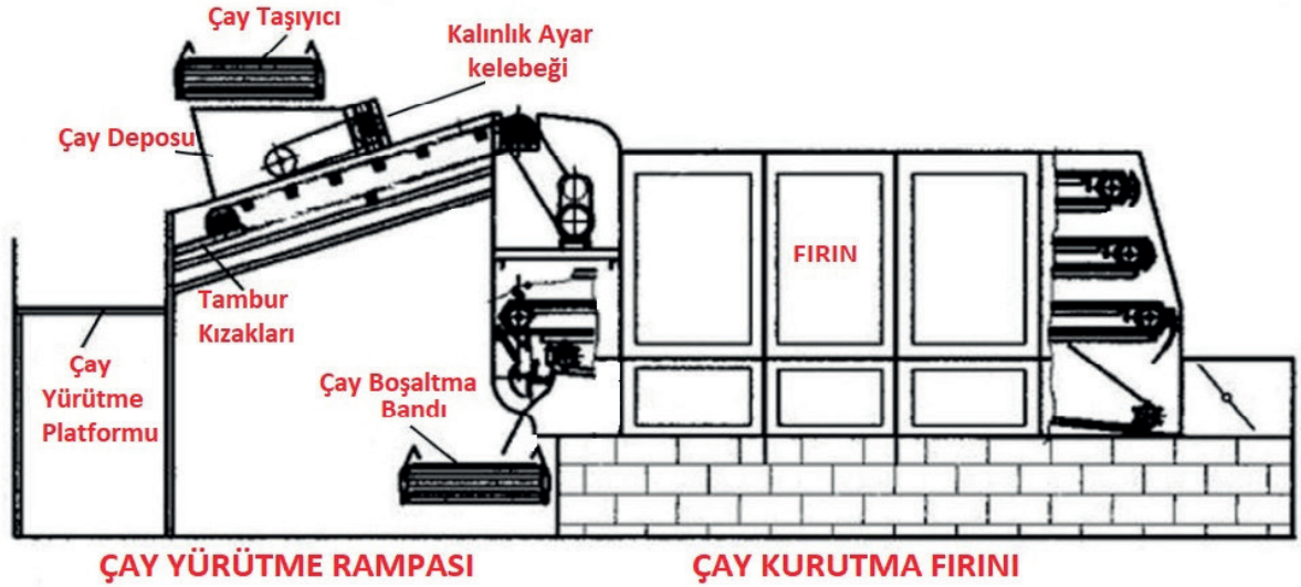
Görsel 4.14: Çay kurutma sisteminin yerleşim şekli
