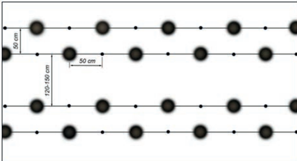
Görsel 2.5: Fidan çukurunun yerlerini belirleme şeması
