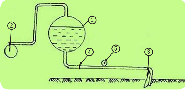
Görsel 3.11: Alçak basınçlı sıvı gübrelerin toprağa verilmesinde kullanılan makinelerin parçaları
