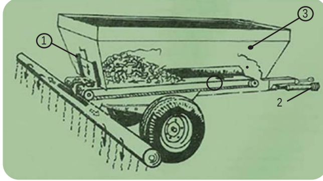
Görsel 3.6: Geniş dağıtma düzenli gübre dağıtma makinesinin parçaları
