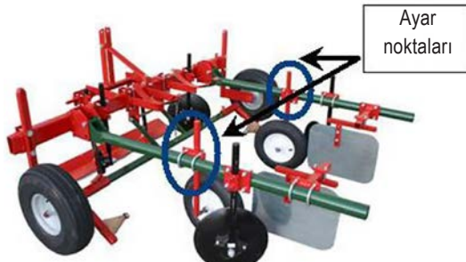
Görsel 1.13: Malç bastırma tekerlerinin ayarı
