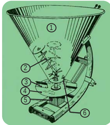
Görsel 3.3: Santrifüjlü gübre atma makinesinin parçaları
