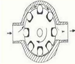
Görsel 2.18: Rulolu pompa
