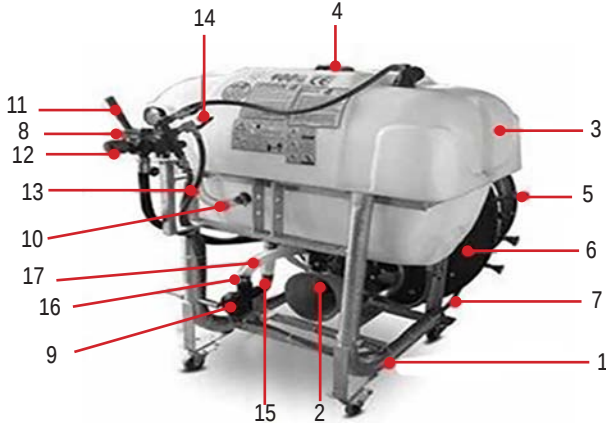
Görsel 2.40: Askılı tip atomizörün parçaları
