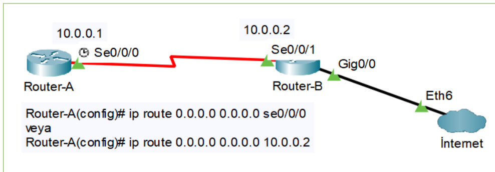
Görsel 2.18: Varsayılan rota ile yönlendirme
