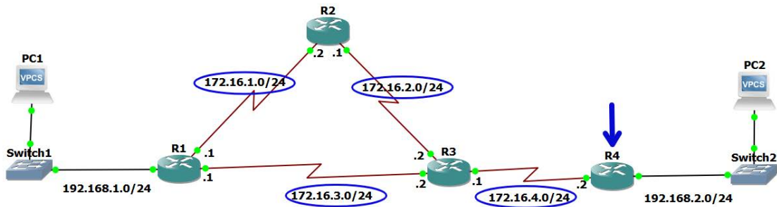
Görsel 2.29: Özet statik rotanın uygulanacağı cihazın belirlenmesi
