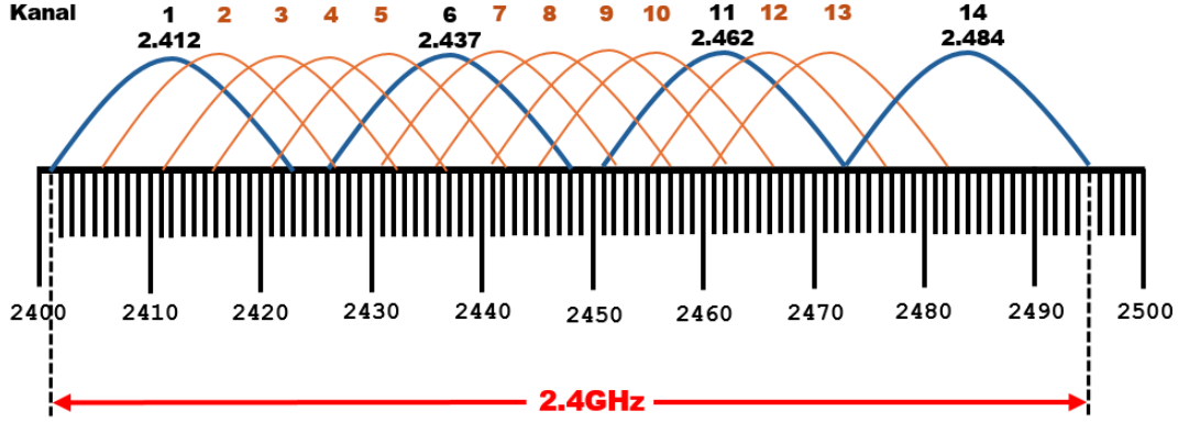
Görsel 3.39: 2.4 GHz kanal yapısı
