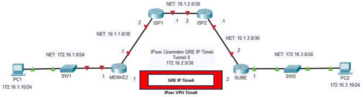
Görsel 4.50: IPsec üzerinden GRE protokolüyle IP tüneli ağ topolojisi
