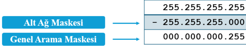
Görsel 2.79: Genel arama maskesini hesaplama
