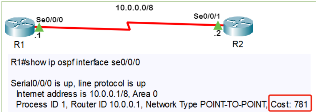
Görsel 2.73: Arayüz maliyetinin görüntülenmesi
