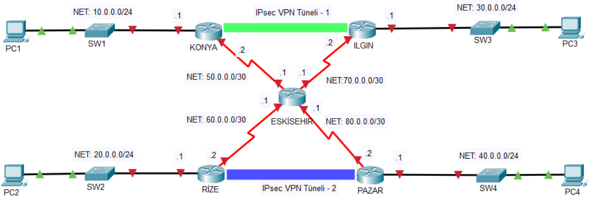
Görsel 4.43: IPsec protokolüyle iki VPN tüneli oluşturma ağ topolojisi
