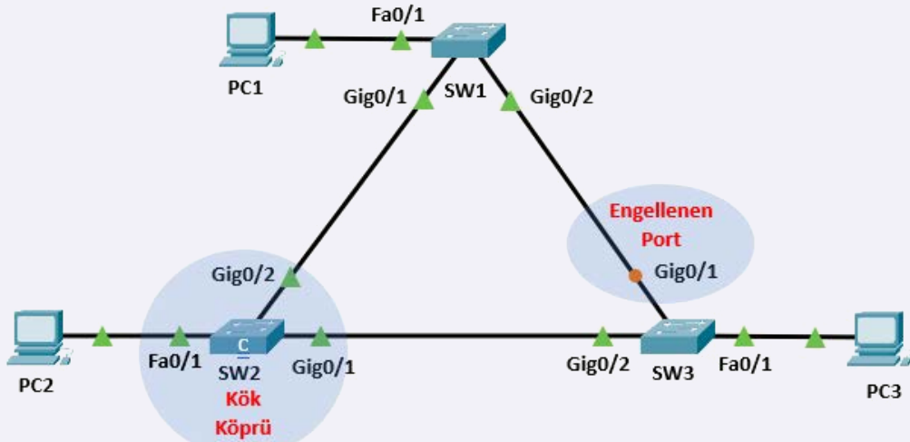
Görsel 1.62: SW2'nin kök köprü olmasının sağlanması
