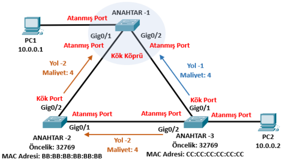
Görsel 1.55: STP atanmış port belirleme
