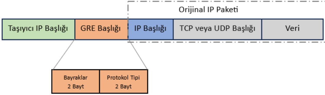
Görsel 4.4: GRE protokolü paket yapısı
