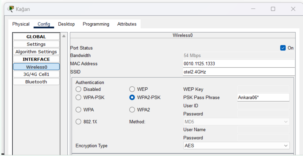
Görsel 3.64: Kablosuz istemcinin ağa dâhil olması
