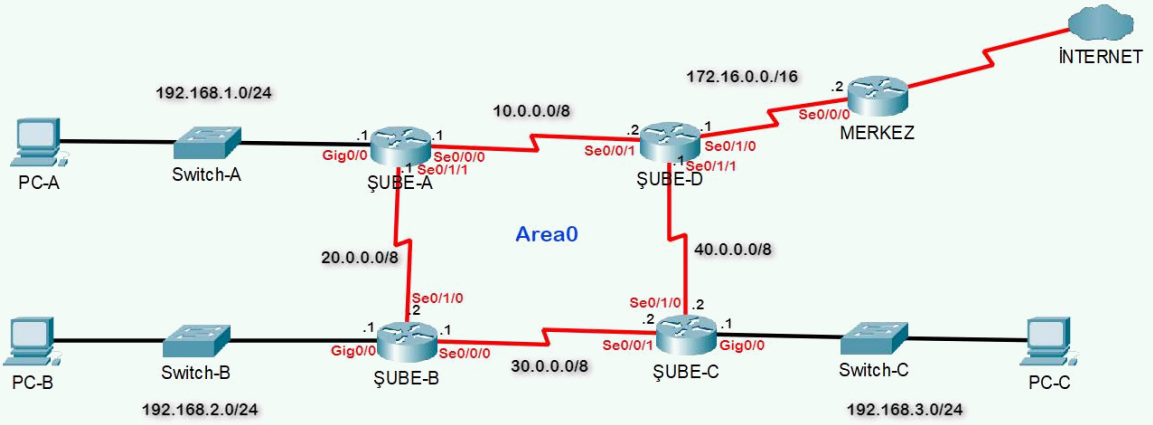
Görsel 2.88: 9. uygulamanın ağ topolojisi
