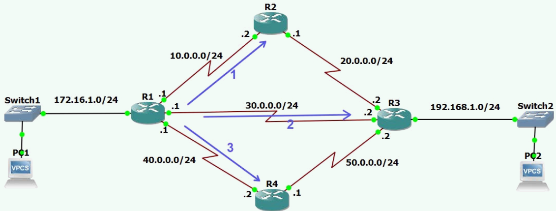
Görsel 2.35: 5. uygulamanın ağ topolojisi
