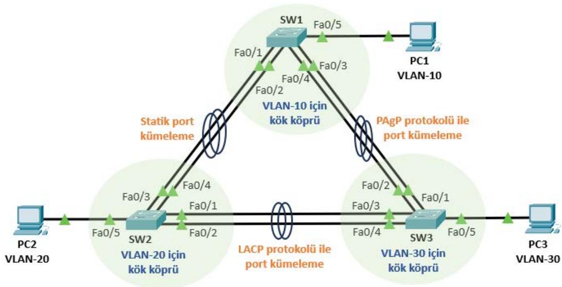
Görsel 1.72: Üç anahtar arası döngüsüz port kümeleme uygulama topolojisi
