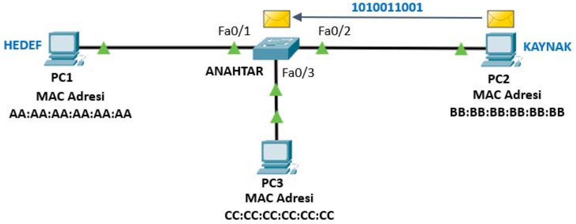
Görsel 1.7: PC2'den fiziksel katmana gönderilen çerçevenin anahtara ulaşması
