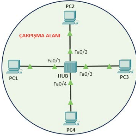
Görsel 1.12: Hub cihazı çarpışma alanı
