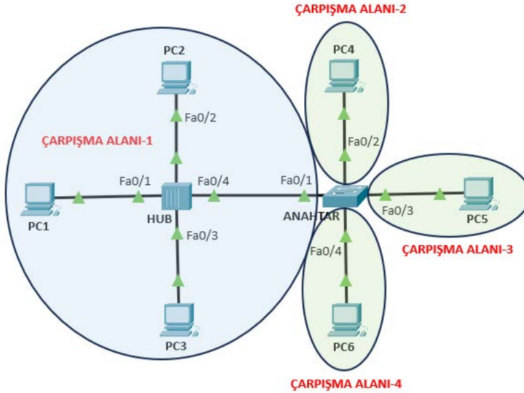
Görsel 1.14: Hub ve anahtar birlikte kullanıldığında oluşan çarpışma alanları
