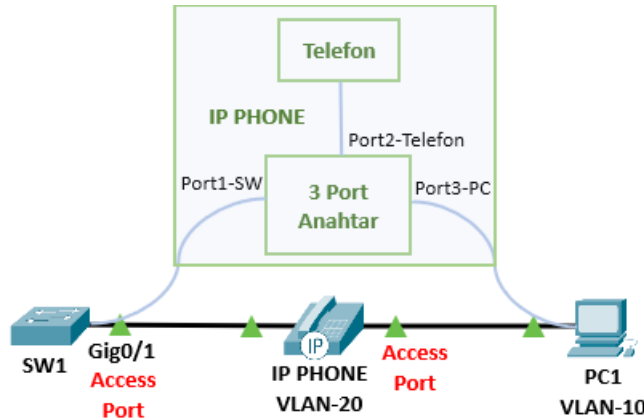
Görsel 1.26: IP telefon bağlantı şeması
