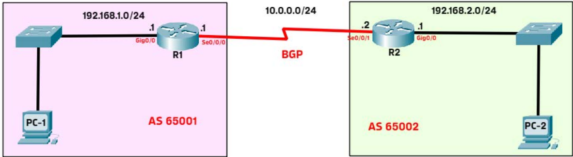
Görsel 2.101: BGP ile yönlendirme
