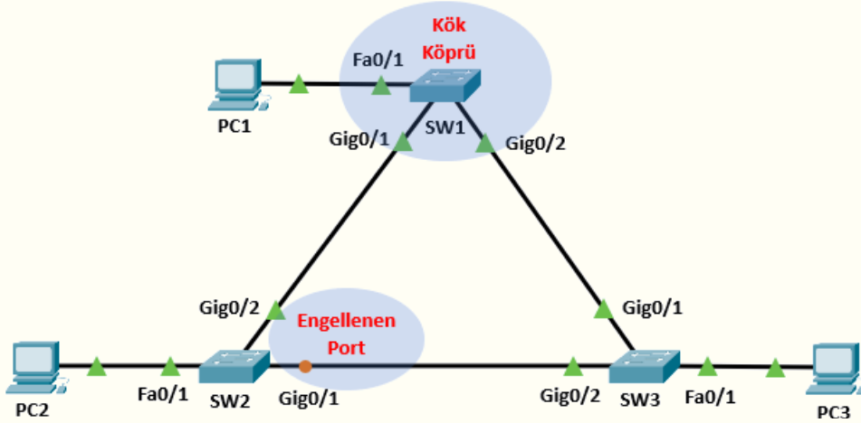
Görsel 1.58: STP protokolü uygulama topolojisi
