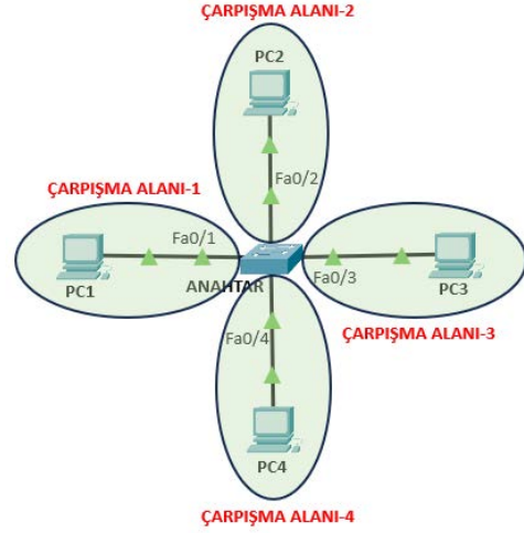
Görsel 1.13: Anahtar portları çarpışma alanı
