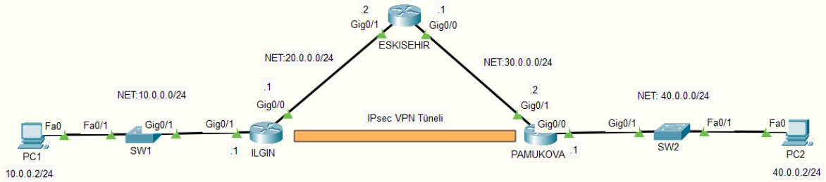
Görsel 4.38: IPsec VPN tüneli ağ topolojisi
