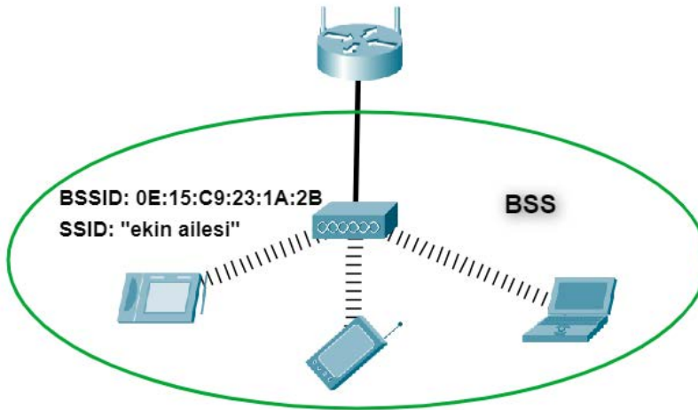
Görsel 3.24: BSS
