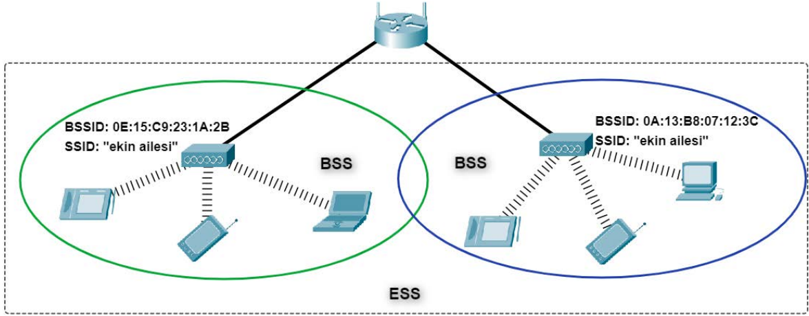
Görsel 3.25: ESS
