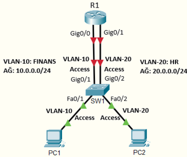
Görsel 1.42: Geleneksel IVR uygulama topolojisi
