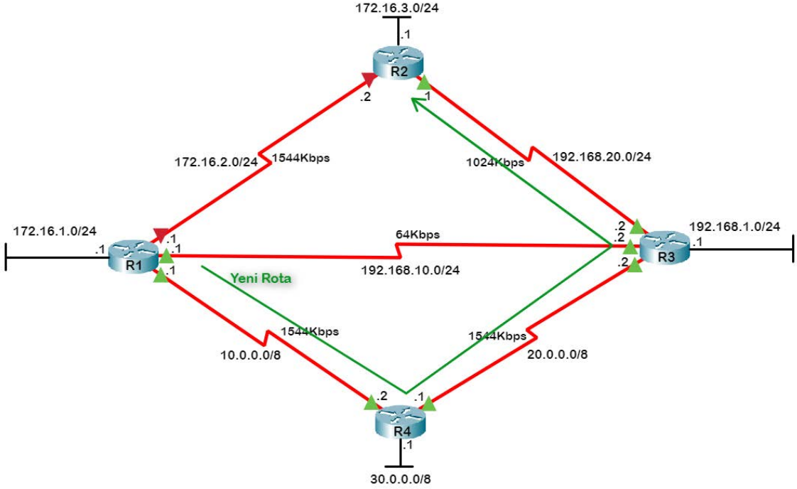
Görsel 2.76: Yeni rota bilgisi
