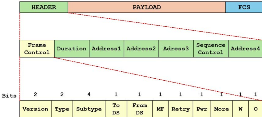
Görsel 3.27: 802.11 çerçeve yapısı
