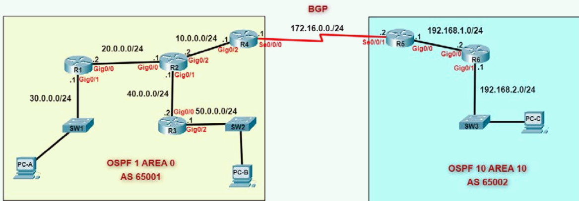
Görsel 2.108: 11. uygulamanın ağ topolojisi
