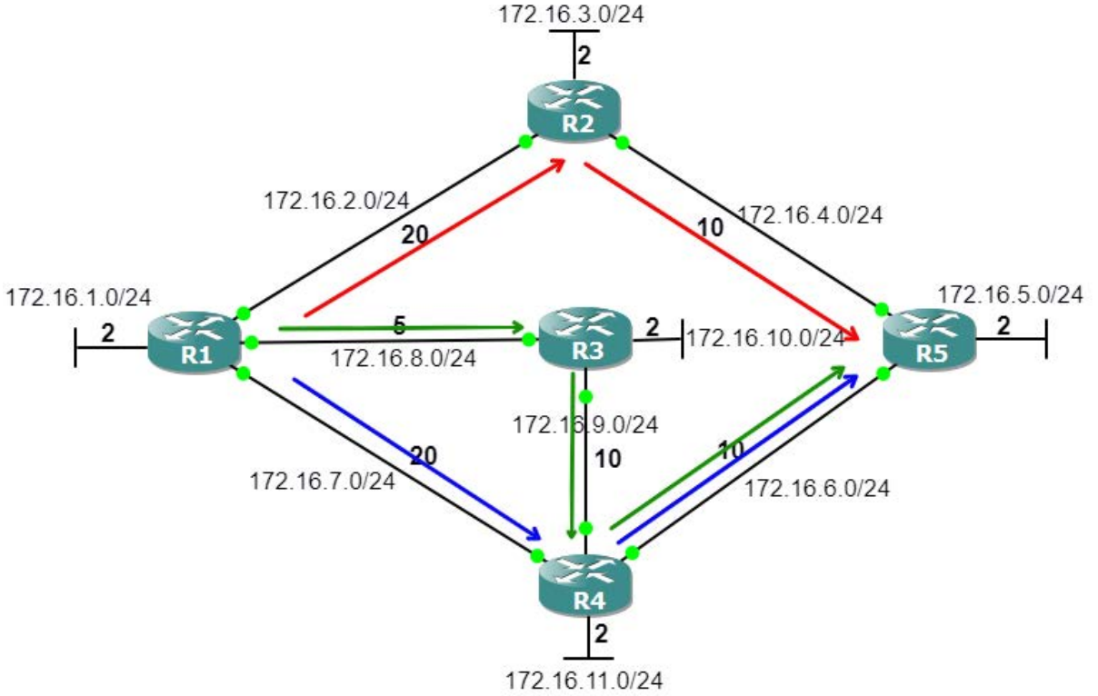
Görsel 2.67: En iyi yolun seçilmesi
