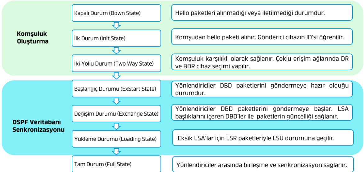
Görsel 2.68: OSPF işleyiş durumları
