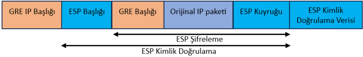
Görsel 4.21: Taşıma modu IPsec VPN üzerinden GRE IP tüneli paket yapısı
