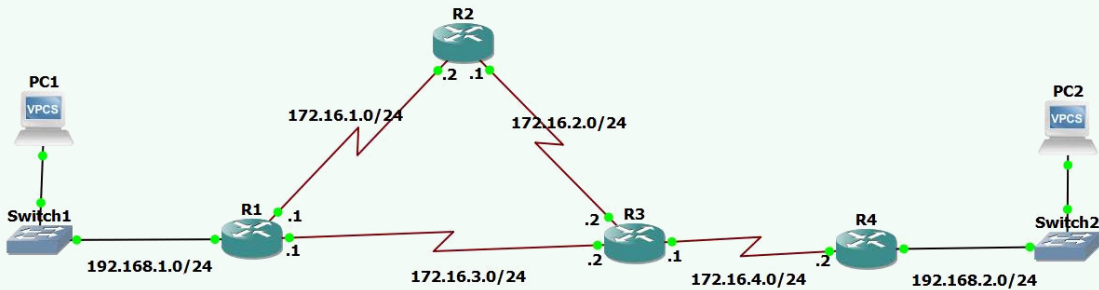
Görsel 2.26: 4. uygulamanın ağ topolojisi
