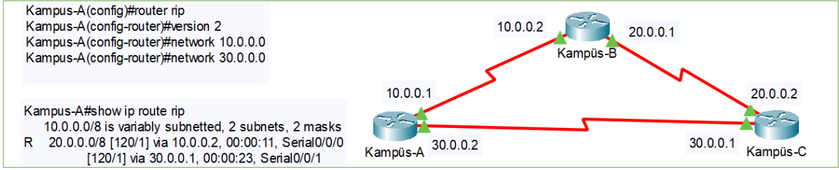
Görsel 2.47: RIPv2 ile yönlendirme
