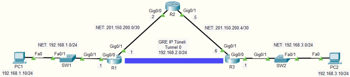
Görsel 4.33: GRE protokolü IP tüneli ağ topolojisi
