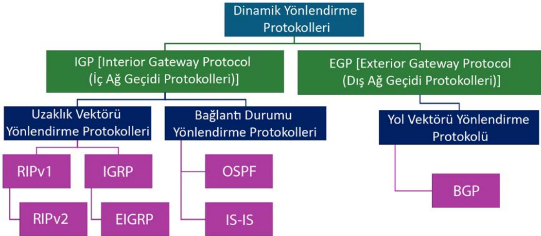
Görsel 2.42: Dinamik yönlendirme protokolleri
