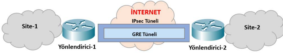
Görsel 4.20: IPsec VPN üzerinden GRE IP tüneli yapısı
