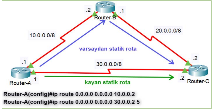
Görsel 2.34: Kayan statik rota
