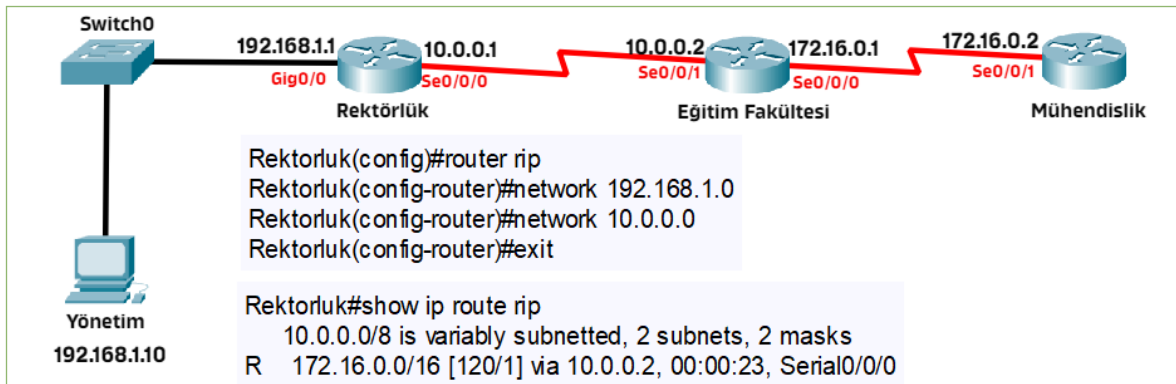
Görsel 2.46: RIP ile yönlendirme
