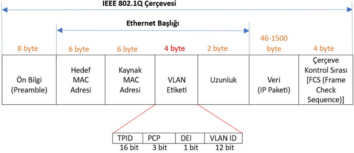
Görsel 1.17: VLAN etiketinin Ethernet çerçevesine eklenmesi
