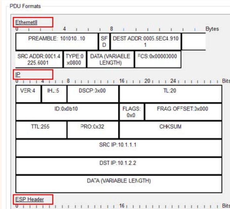
Görsel 4.46: MERKEZ yönlendiricisinde ethernet çerçevesine ESP ve yeni IP başlığı eklenmesi
