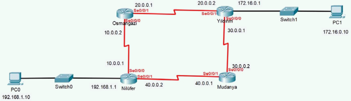
Görsel 2.58: 7. uygulamanın ağ topolojisi
