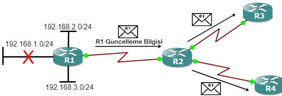
Görsel 2.44: Güncelleme bilgisi paylaşımı
