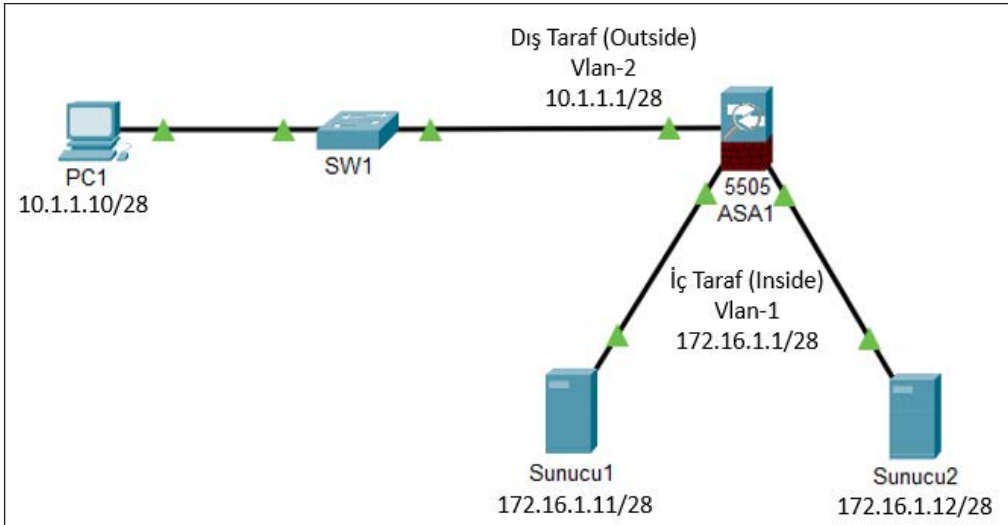
Görsel 4.32: İstemcisiz SSL web VPN ağ topolojisi
