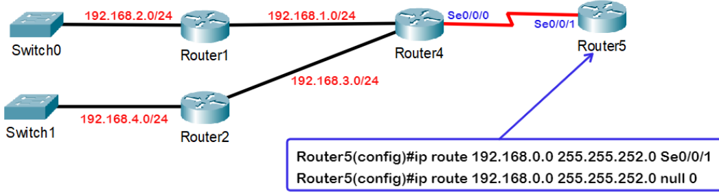
Görsel 2.24: Özet statik rota
