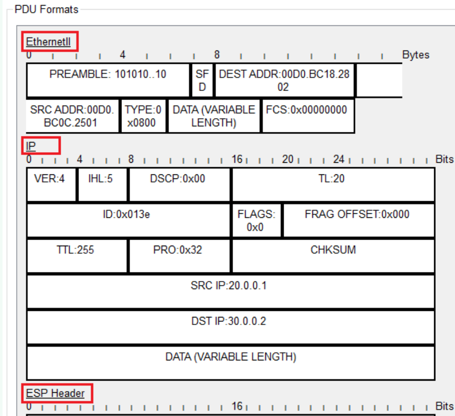
Görsel 4.40: ILGIN yönlendiricisinde ethernet çerçevesine ESP ve yeni IP başlığı eklenmesi
