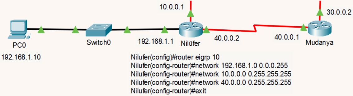
Görsel 2.60: EIGRP ile yönlendirme
