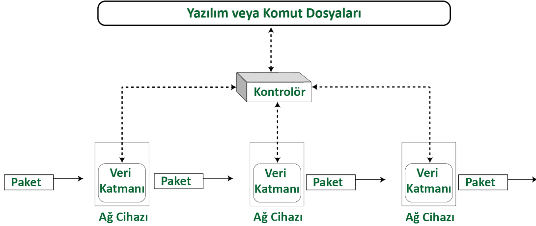
Şema 5.1: Denetleyici tabanlı ağ modeli
