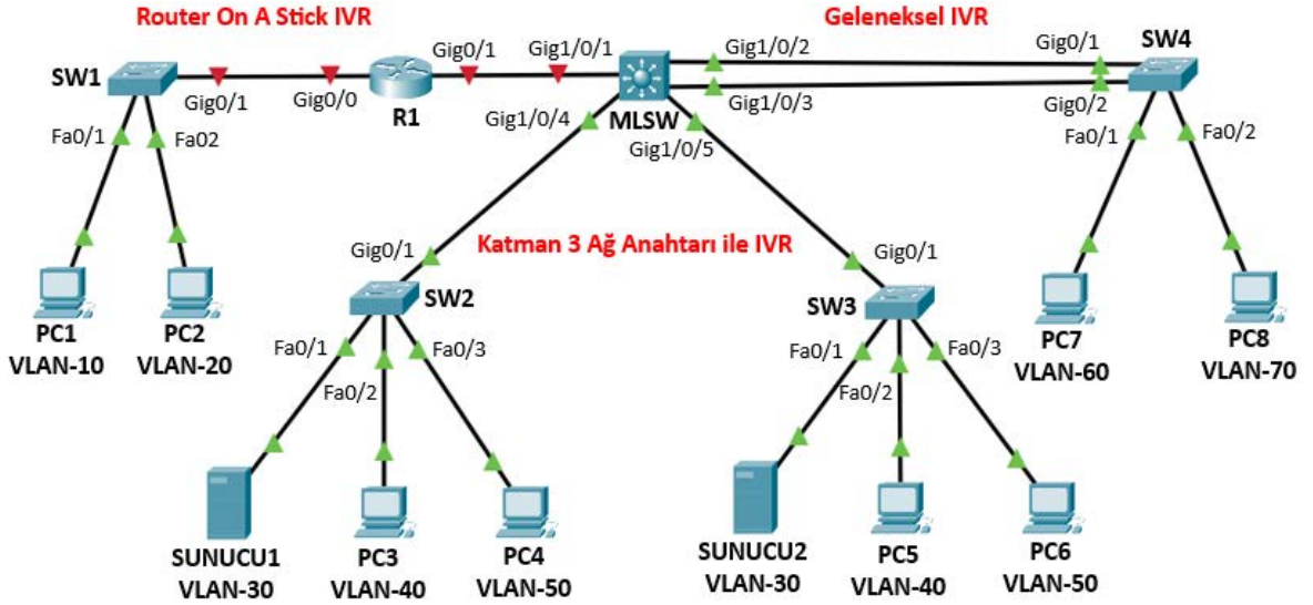
Görsel 1.48: VLAN'lar arası yönlendirme uygulama topolojisi
