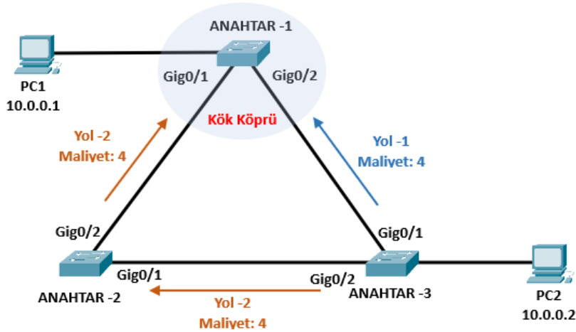
Görsel 1.53: STP kök yol hesaplaması
