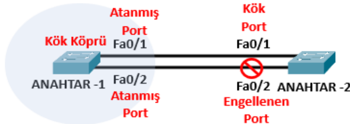
Görsel 1.57: İki anahtar arasında STP süreci
