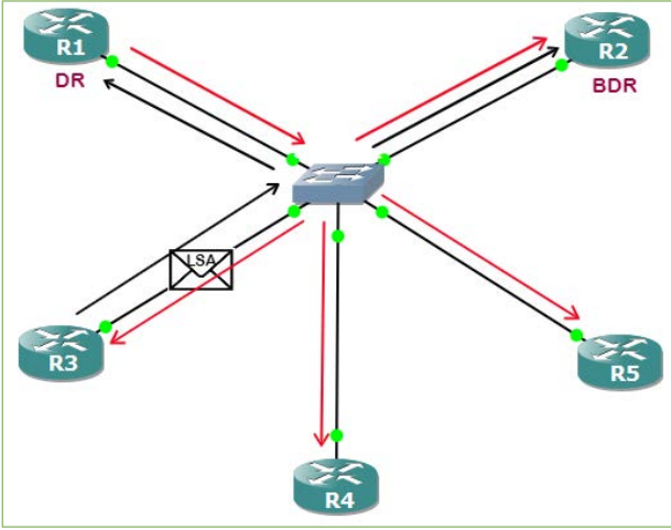
Görsel 2.70: DR ve BDR cihaz seçimi
