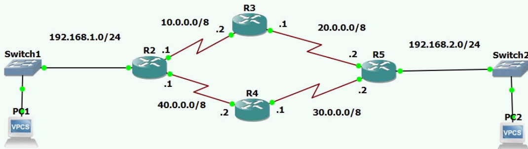
Görsel 2.12: 2. uygulamanın ağ topolojisi
