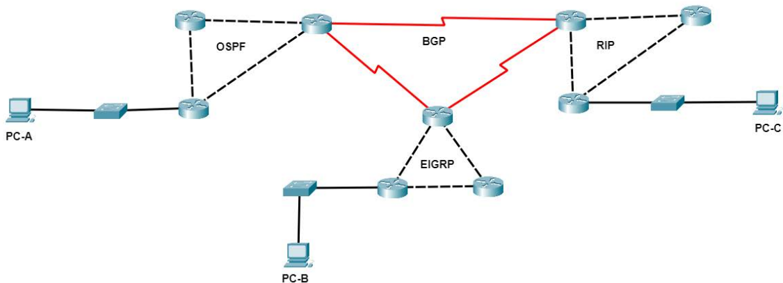
Görsel 2.116: Sıra sizde etkinliğinin ağ topolojisi
