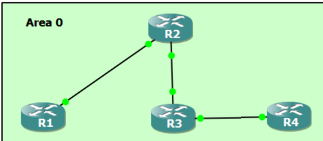
Görsel 2.71: Tek alanlı OSPF
