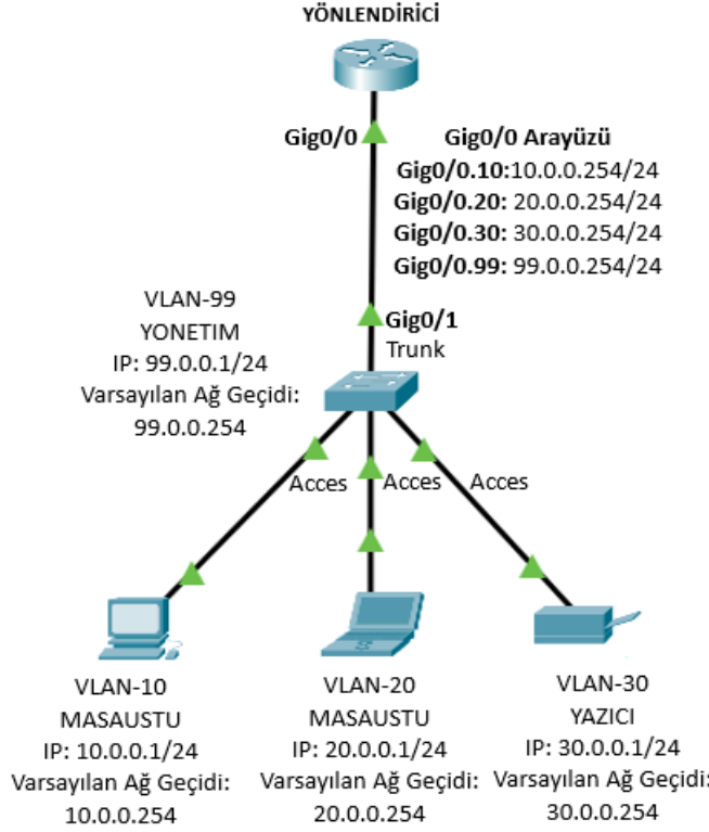
Görsel 1.40: Router On A Stick IVR yöntemi
