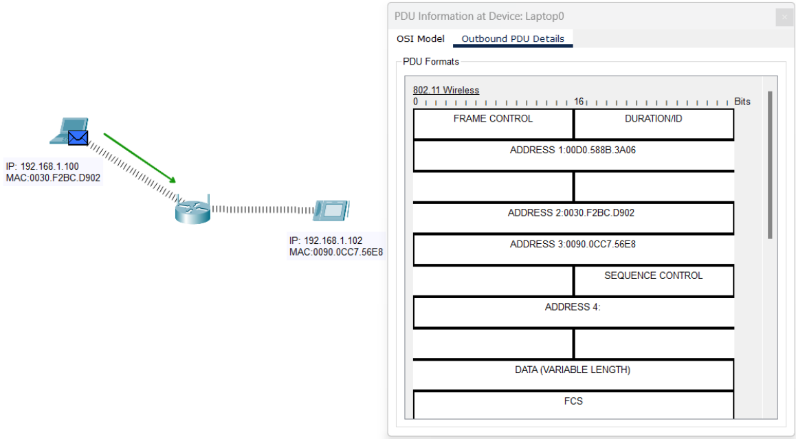
Görsel 3.28: 802.11 çerçeve yapısı
