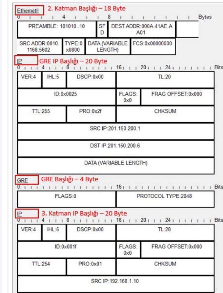
Görsel 4.34: R1 yönlendiricisinde ethernet çerçevesine GRE ve GRE IP başlığı eklenmesi
