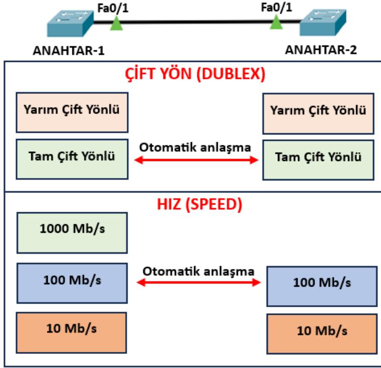
Görsel 1.11: Çift yön modunun ve port hızlarının eşleştirilmesi
