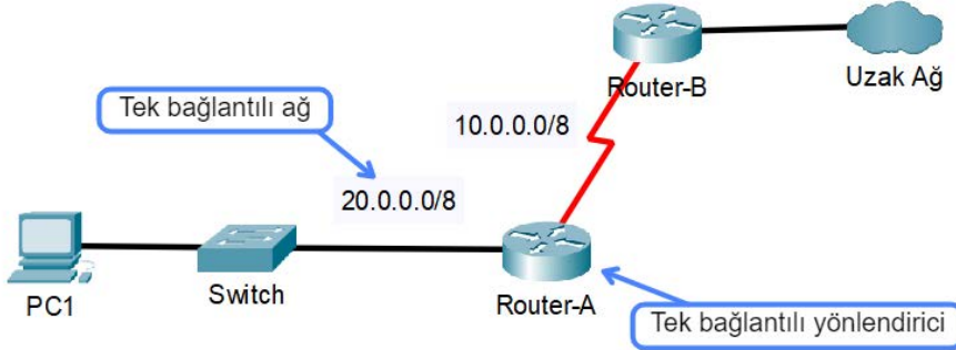
Görsel 2.4: Standart statik rota
