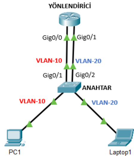
Görsel 1.39: Geleneksel IVR yöntemi
