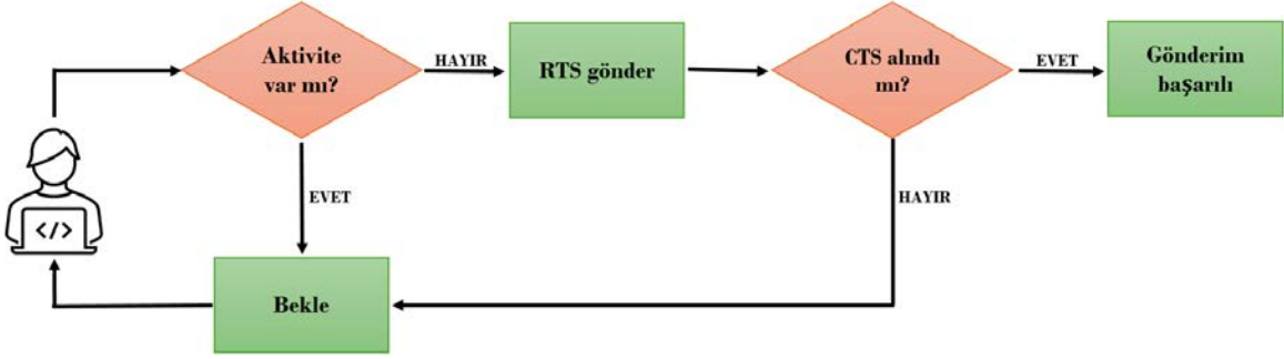
Görsel 3.29: CSMA/CA
