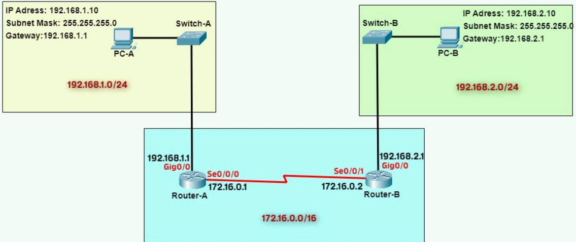
Görsel 2.5: 1. uygulamanın ağ topolojisi
