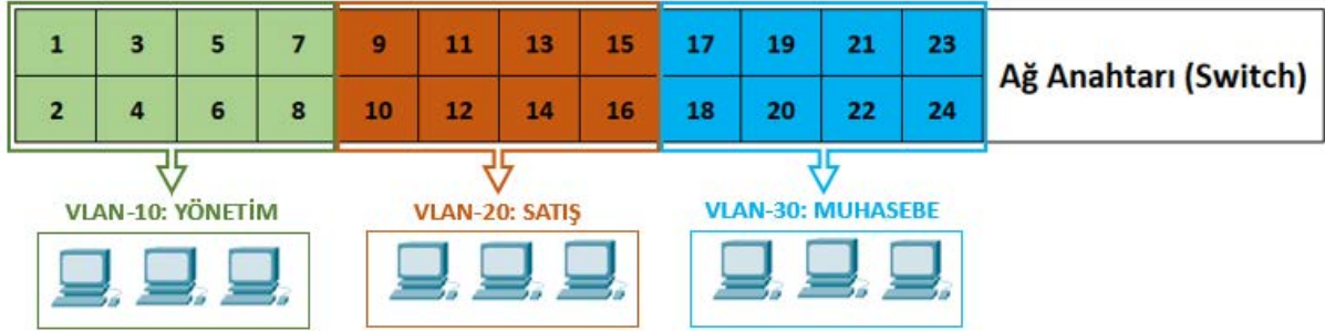
Görsel 1.15: Anahtar üzerinde oluşturulan VLAN grupları
