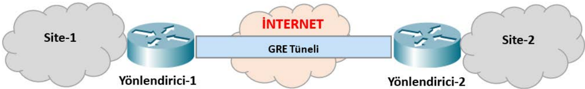
Görsel 4.3: GRE tünel yapısı
