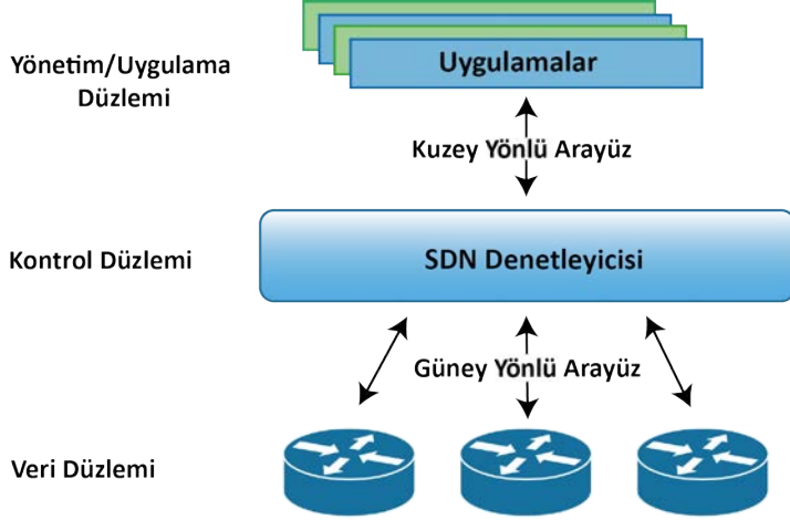
Görsel 5.5: SDN mimarisindeki üç düzlem
