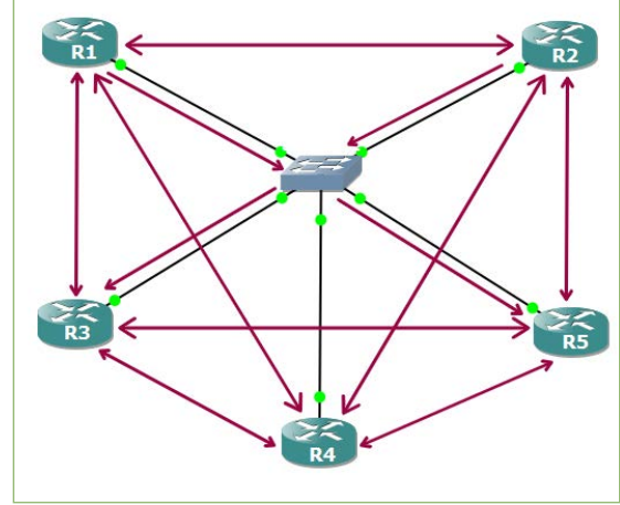
Görsel 2.69: Cihazlar arasında komşuluk bağlantısı
