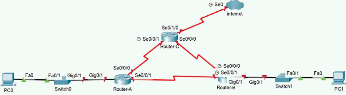
Görsel 2.19: 3. uygulamanın ağ topolojisi
