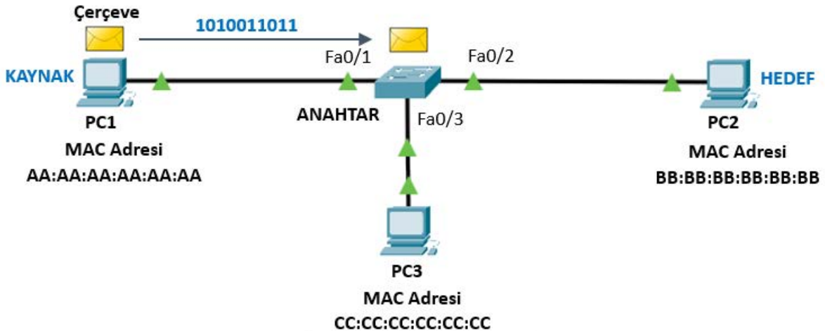
Görsel 1.5: PC1'den fiziksel katmana gönderilen çerçevenin anahtara ulaşması
