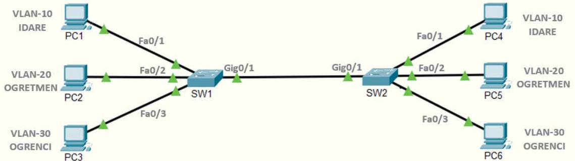
Görsel 1.34: VLAN'lar arası haberleşme ağ topolojisi
