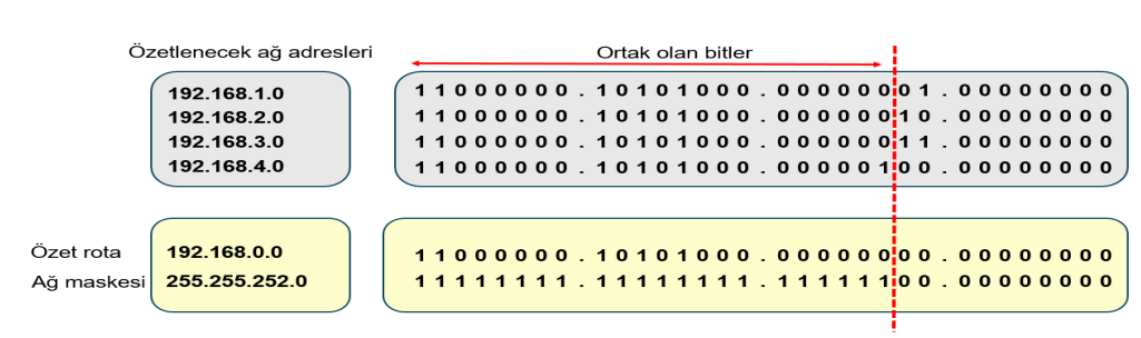
Görsel 2.25: Özet rota hesaplama
