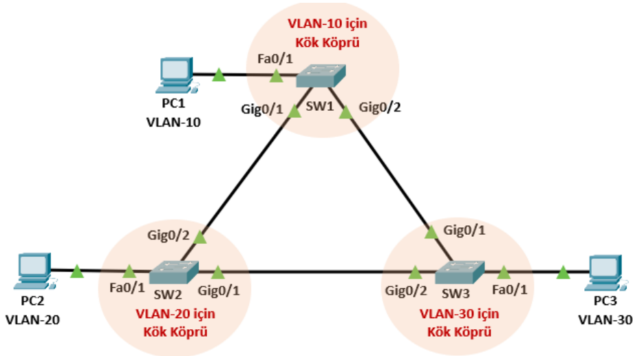
Görsel 1.64: Her VLAN için ayrı kök köprü belirleme ağ topolojisi
