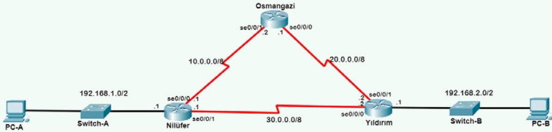
Görsel 2.80: 8. uygulamanın ağ topolojisi
