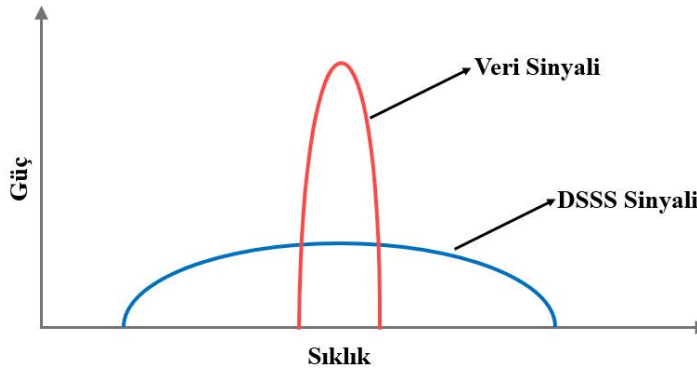
Görsel 3.36: DSSS
