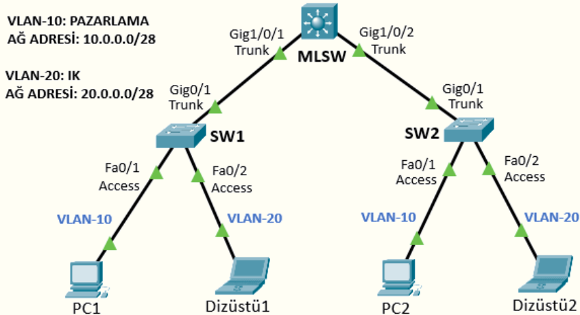
Görsel 1.47: Çok katmanlı ağ anahtarıyla IVR uygulama topolojisi
