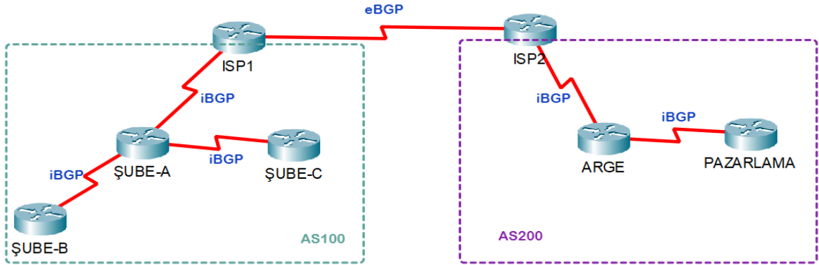
Görsel 2.97: BGP’de komşuluk türleri
