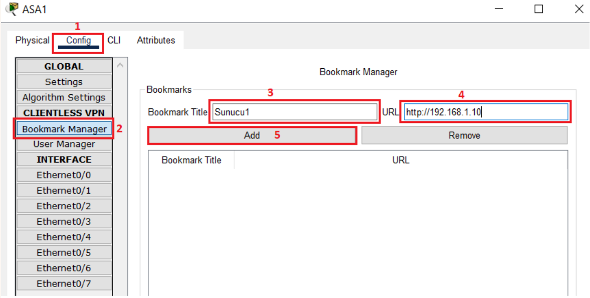
Görsel 4.27: Güvenlik duvarında CLIENTLESS VPN servisine Sunucu1'in web sayfasının adresinin eklenmesi
