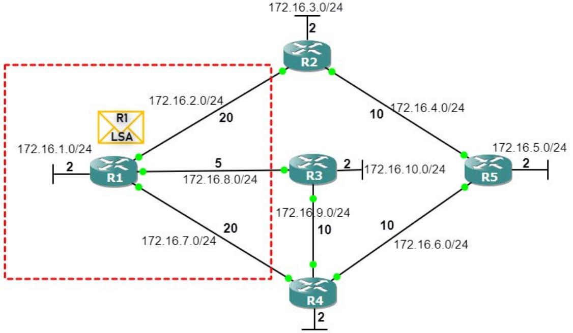
Görsel 2.66: LSA paketinin gönderimi
