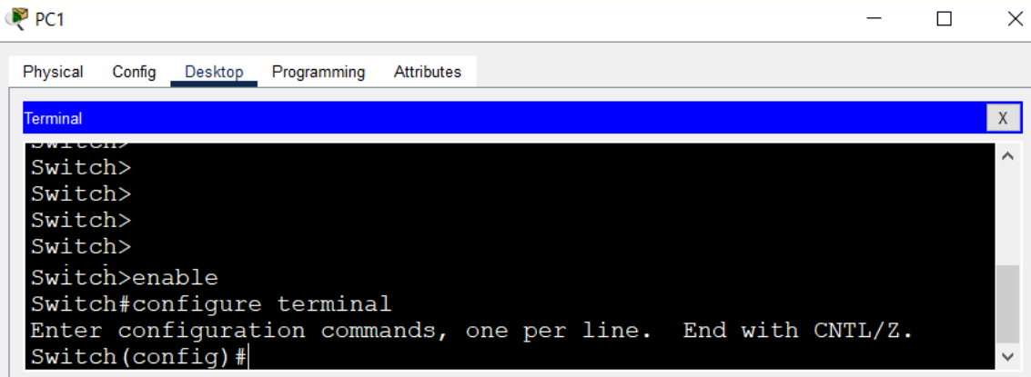
Görsel 1.31: Yetkili moda ve konfigürasyon moduna geçiş yapma
