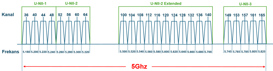
Görsel 3.40: 5 GHz kanal yapısı
