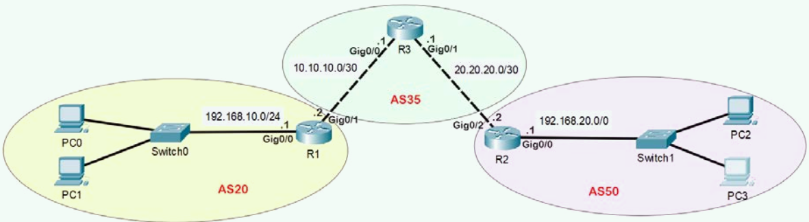
Görsel 2.102: 10. uygulamanın ağ topolojisi
