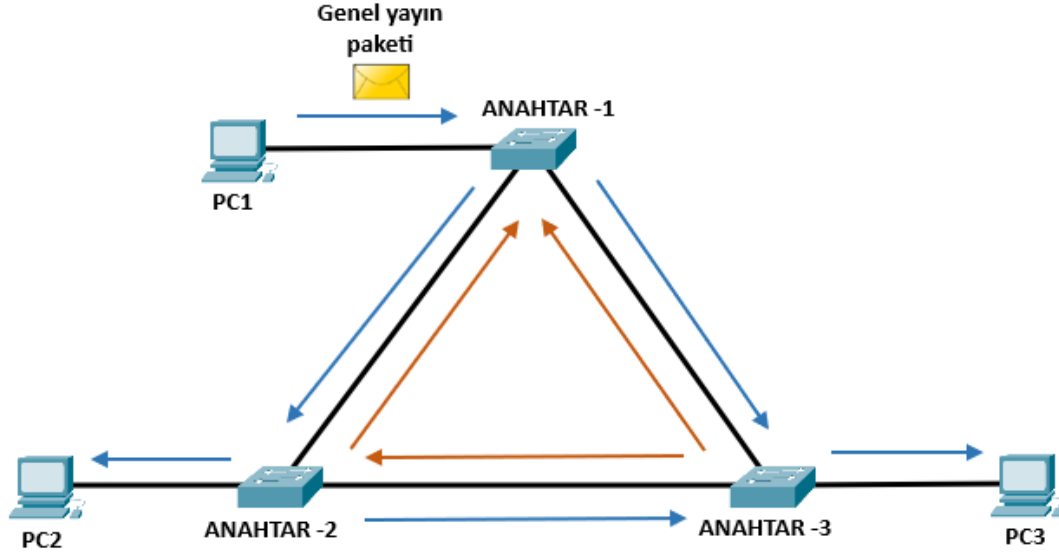
Görsel 1.50: Genel yayın fırtınası
