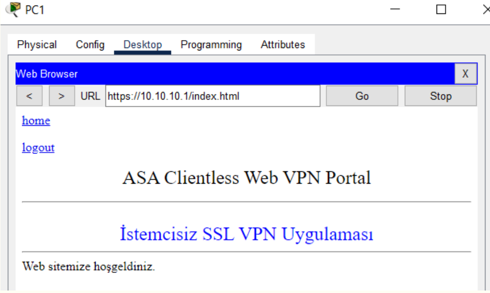
Görsel 4.31: PC1'den VPN ile sunucu üzerindeki web sayfasına erişim
