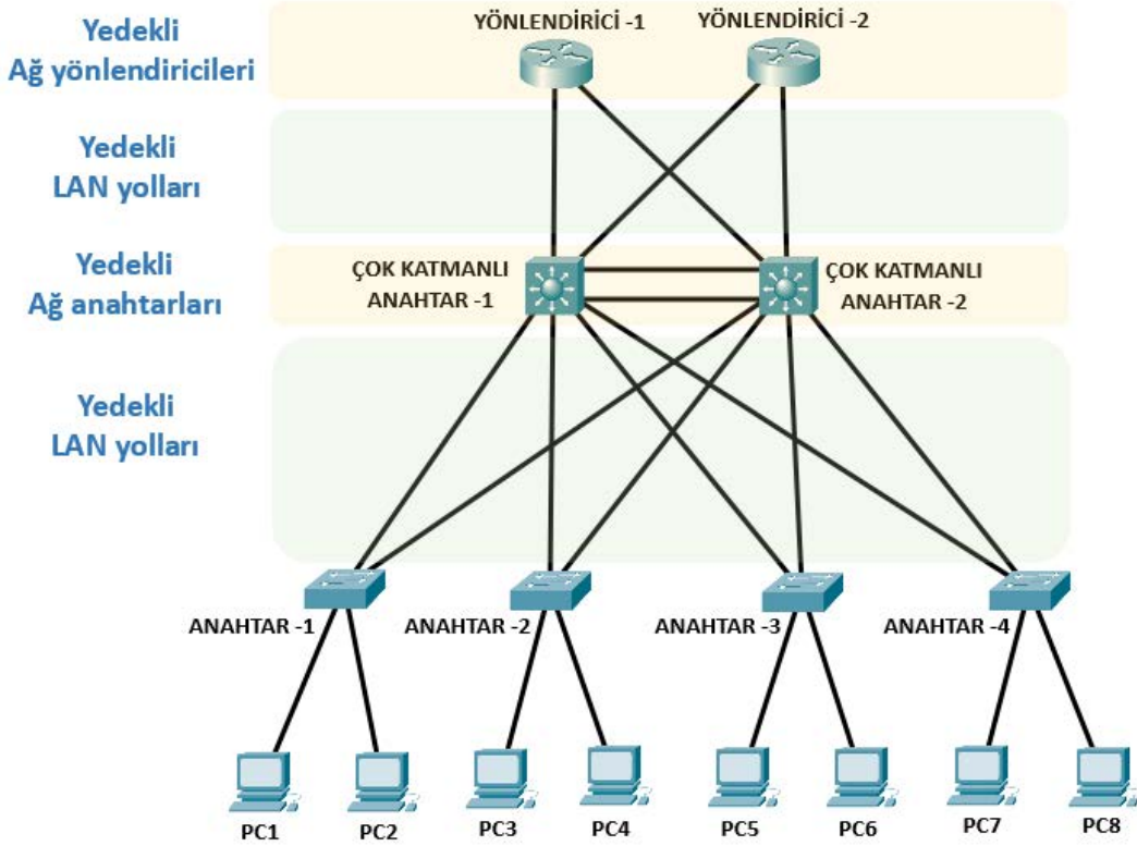
Görsel 1.49: Yedekli yerel alan ağı topolojisi
