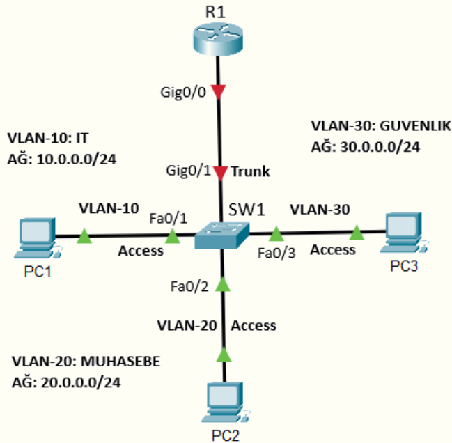
Görsel 1.44: Router On A Stick IVR uygulama topolojisi
