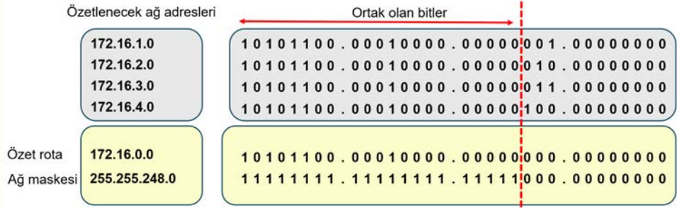
Görsel 2.30: Özet rotanın hesaplanması
