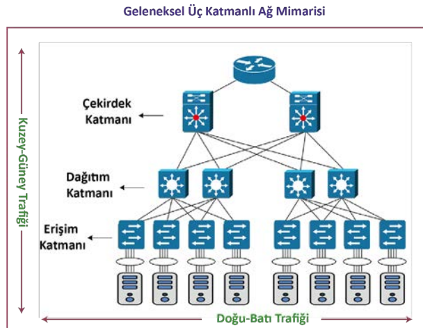
Görsel 5.16: Üç katmanlı ağ mimarisi
