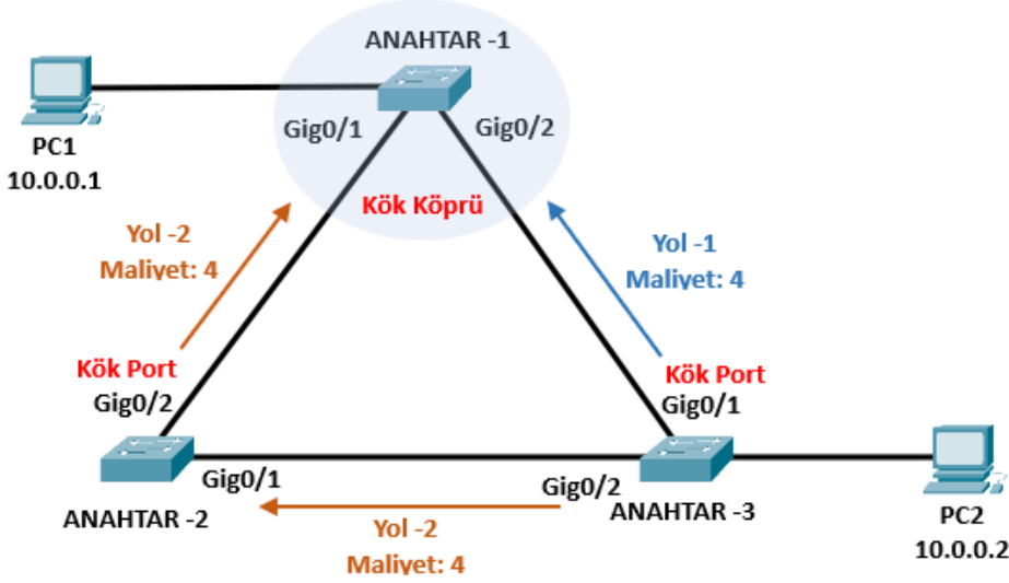
Görsel 1.54: STP kök port belirleme
