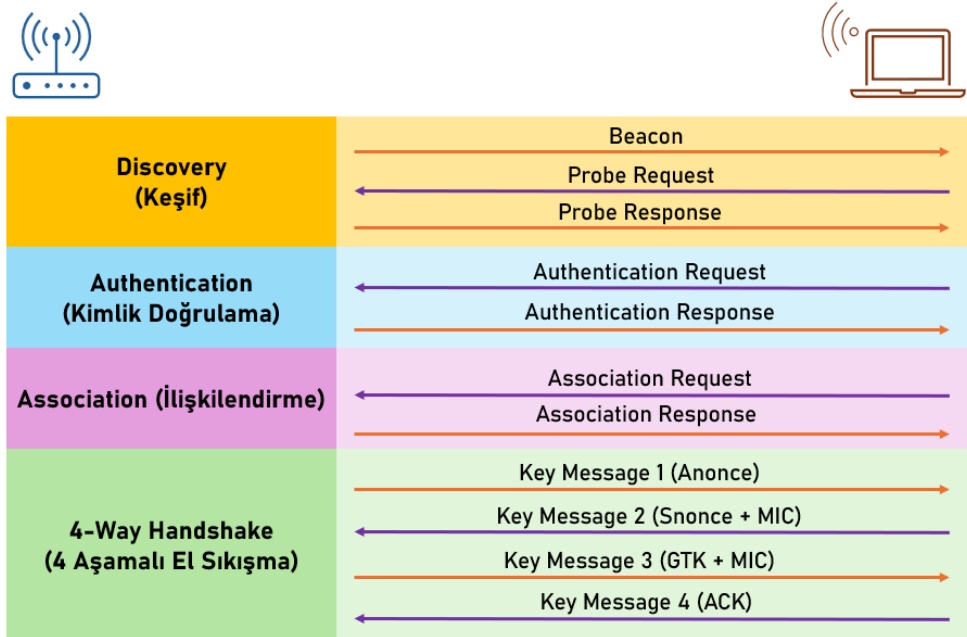
Görsel 3.30: Kablosuz bağlantı süreci
