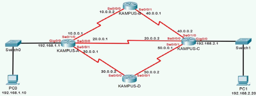
Görsel 2.48: 6. uygulamanın ağ topolojisi
