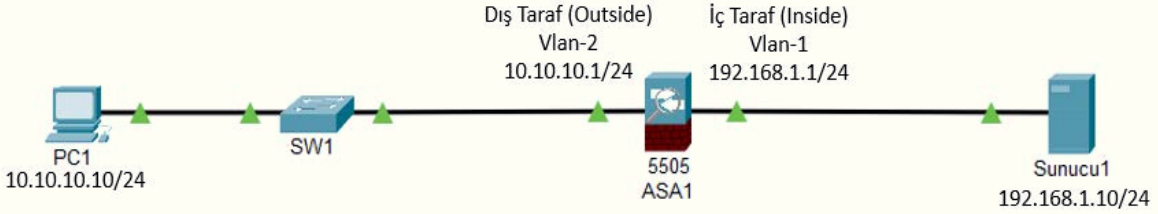
Görsel 4.24: İstemcisiz SSL web VPN ağ topolojisi
