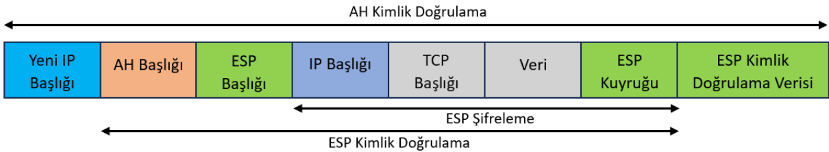
Görsel 4.18: IPsec ESP+AH tünel modu
