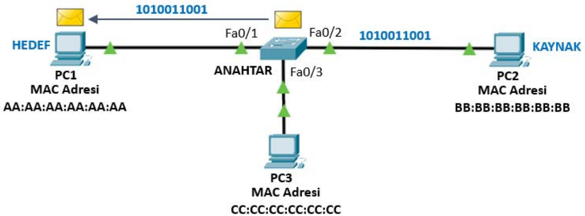
Görsel 1.8: Anahtarın çerçeveyi hedefe tekil yayın olarak iletmesi
