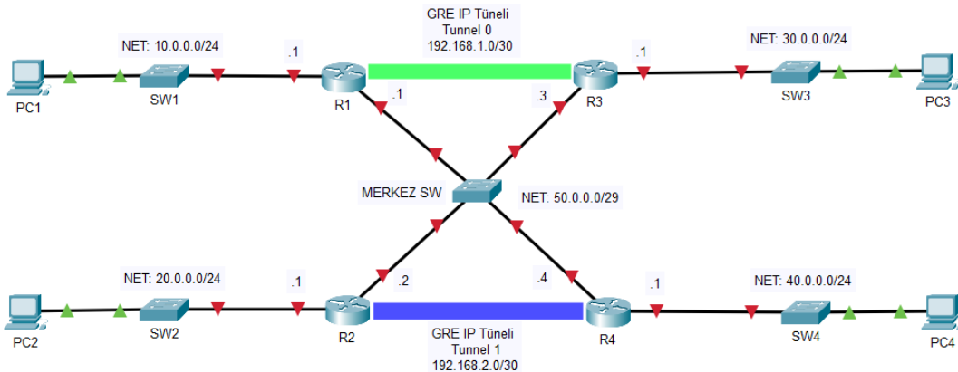
Görsel 4.37: GRE protokolüyle oluşturulmuş iki IP tüneli ağ topolojisi
