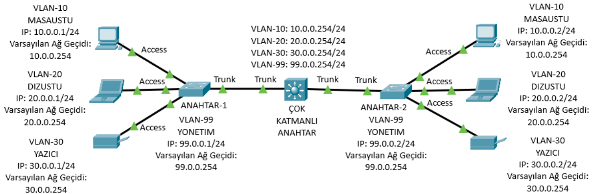
Görsel 1.41: Çok katmanlı ağ anahtarıyla IVR yöntemi
