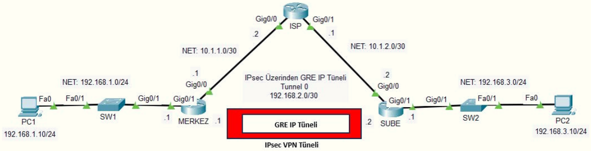
Görsel 4.44: IPsec üzerinden GRE protokolüyle IP tüneli ağ topolojisi
