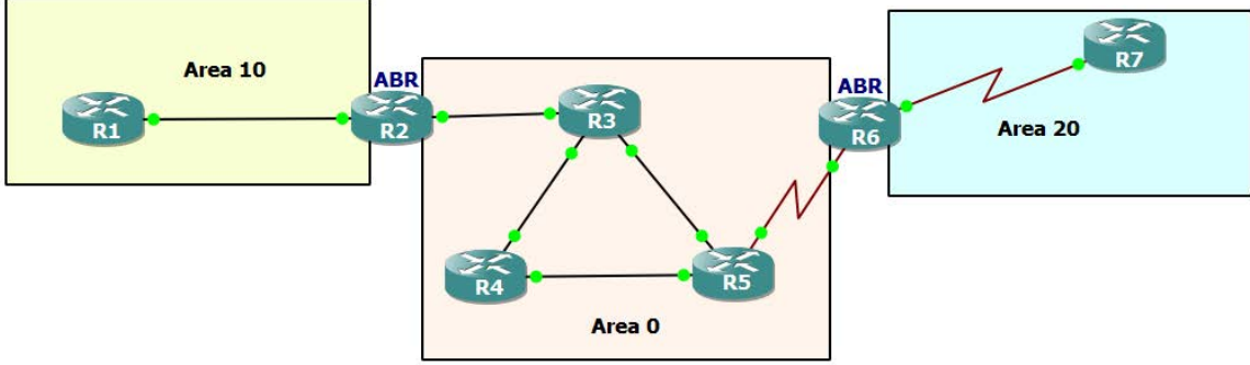
Görsel 2.72: Çok alanlı OSPF
