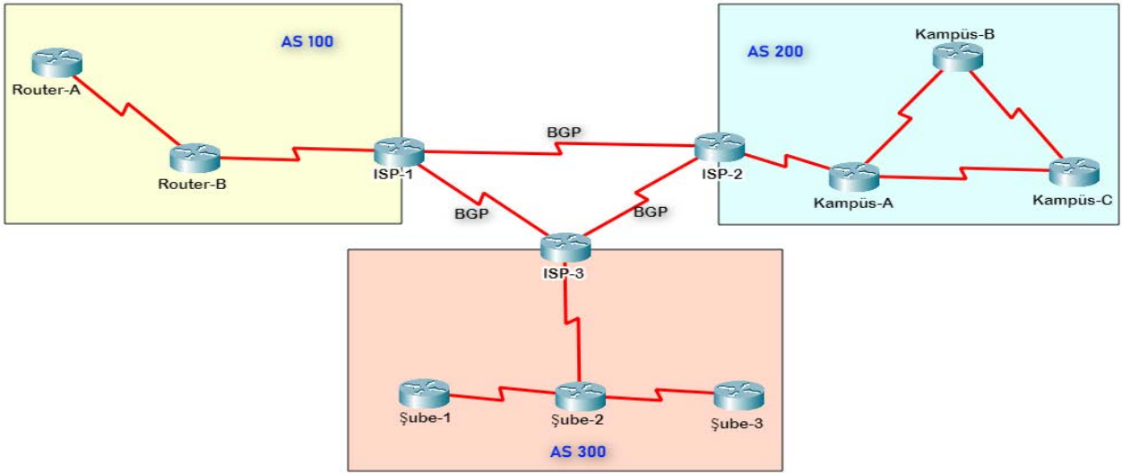
Görsel 2.96: BGP protokolü
