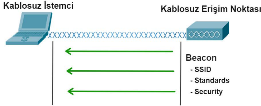
Görsel 3.31: Beacon mesajı
