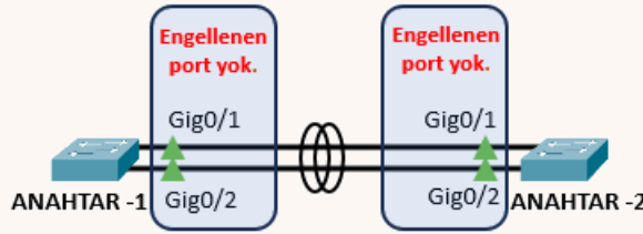
Görsel 1.67: Port kümeleme
