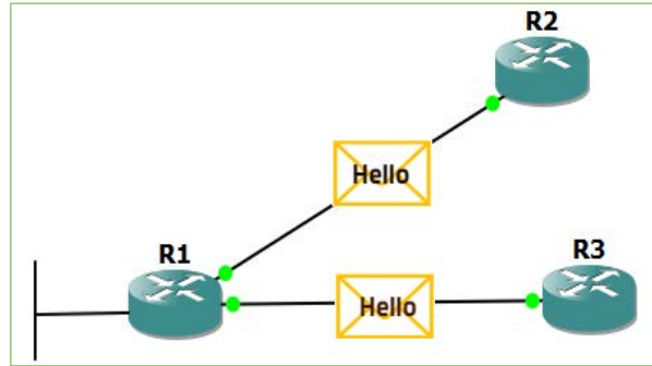
Görsel 2.65: Hello paketi gönderimi
