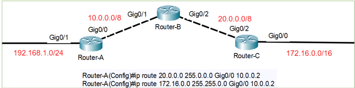
Görsel 2.11: Tamamen tanımlı statik rota
