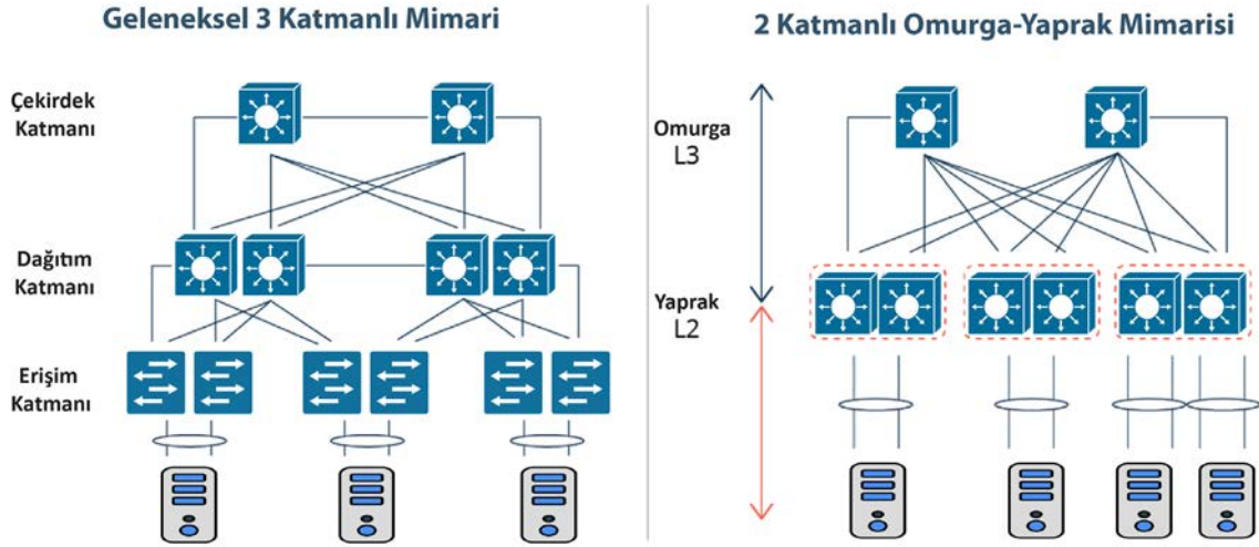
Görsel 5.18: Geleneksel üç katmanlı mimari ve Omurga-Yaprak mimarisi
