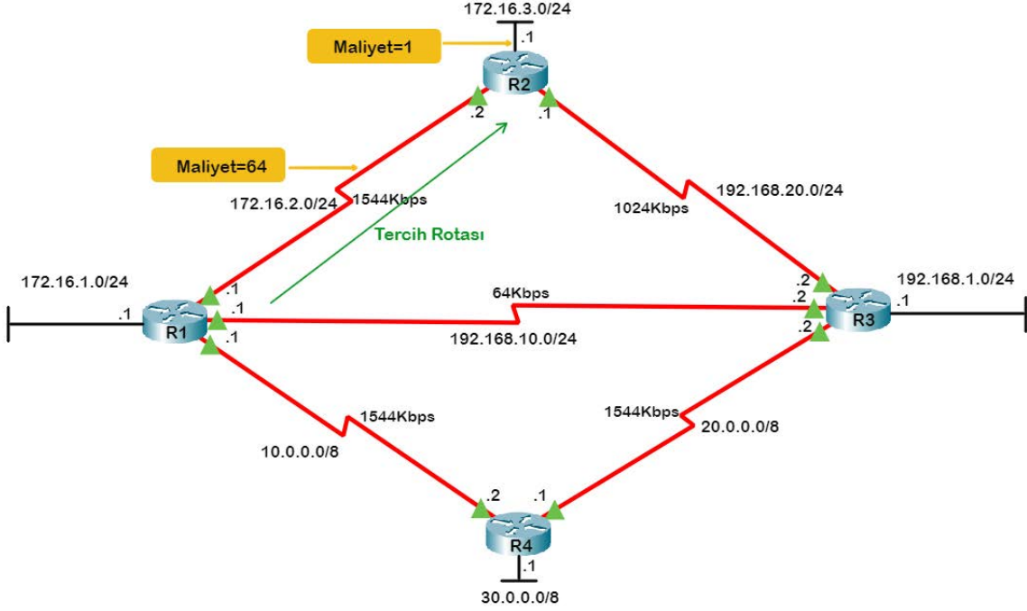
Görsel 2.74: En düşük maliyetli rotanın belirlenmesi
