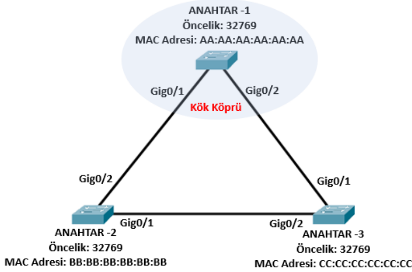
Görsel 1.52: Kök köprü seçimi
