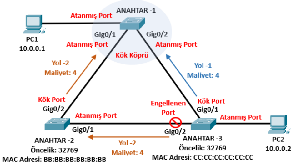
Görsel 1.56: STP engellenen portu belirleme
