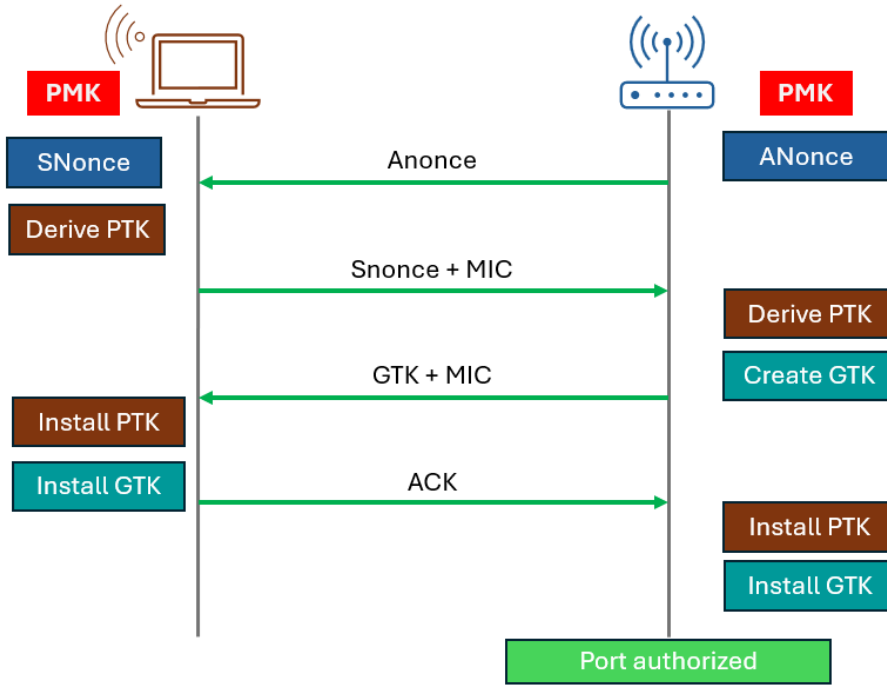
Görsel 3.34: 4-Way Handshake aşamaları
