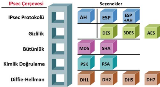
Görsel 4.6: IPsec çerçevesi
