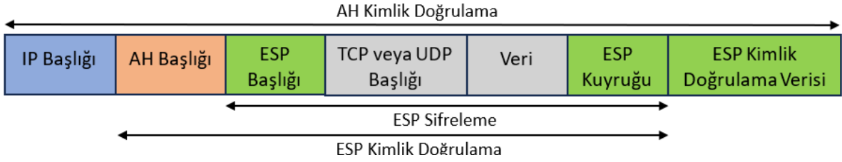
Görsel 4.16: IPsec ESP+AH taşıma modu
