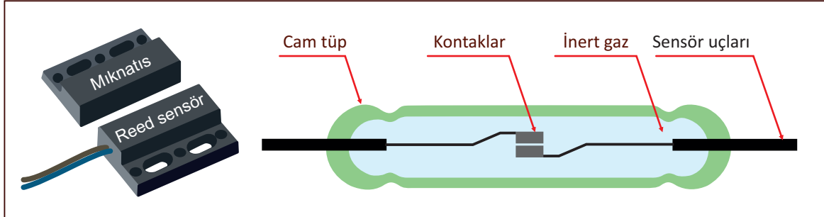
Görsel 1.11: Reed rölenin yapısı ve bileşenleri
