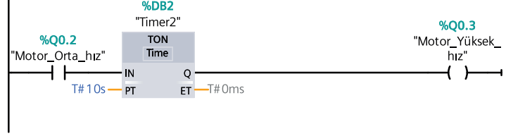
Görsel 5.10: PLC dijital çıkış kontrol program bloğu
