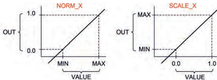
Görsel 3.40: NORM_X ve SCALE_X grafikleri
