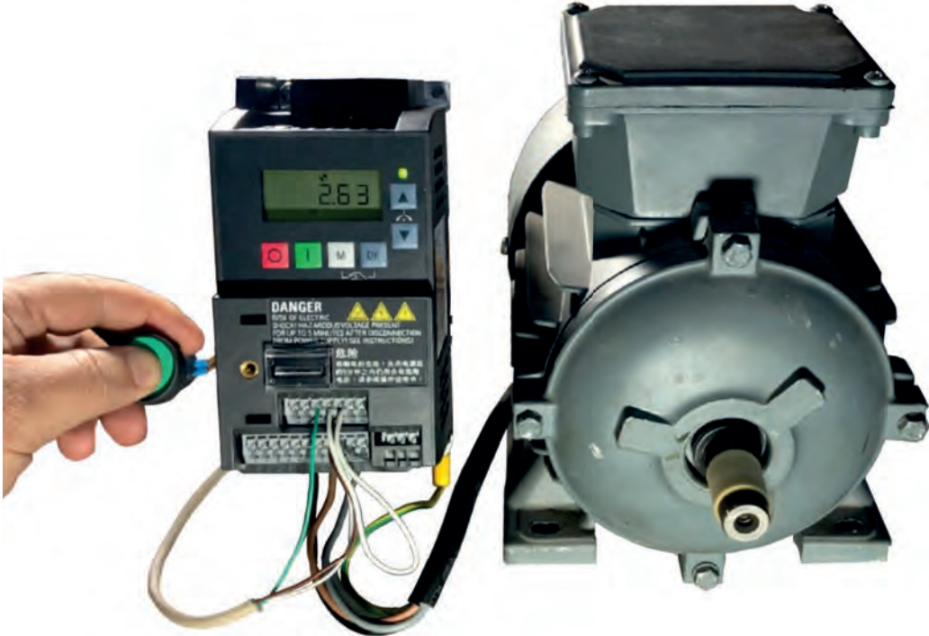
Görsel 5.5: Üç fazlı asenkron motorun periyodik çalışma sürücü ve PLC bağlantıları
