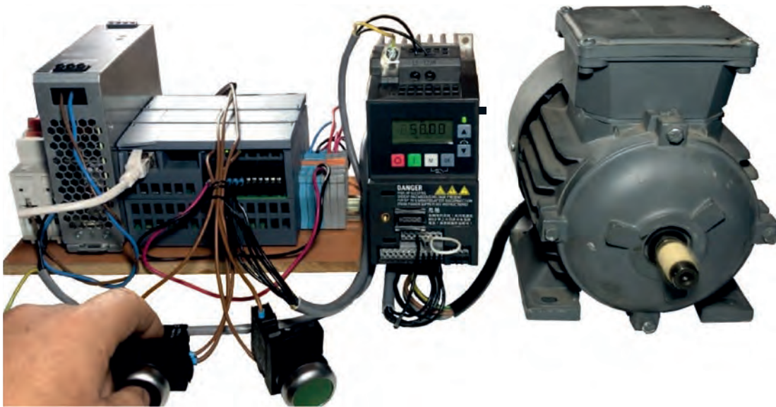
Görsel 5.9: Üç fazlı asenkron motor sürücü ve PLC dijital çıkış bağlantıları
