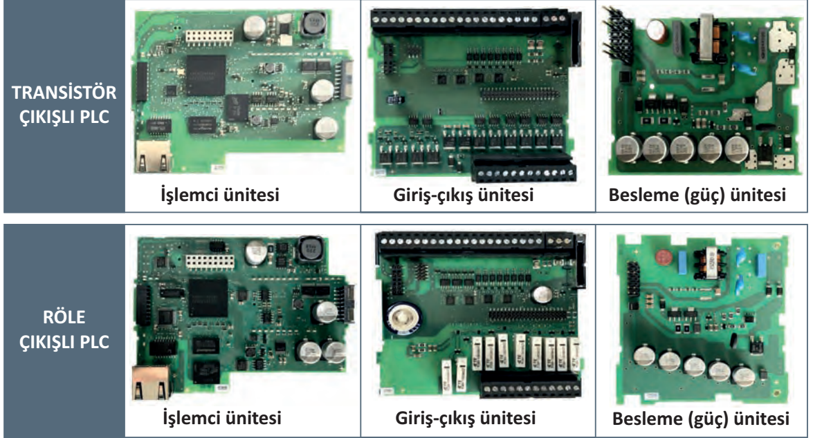
Görsel 2.2: PLC yapısını oluşturan üniteler
