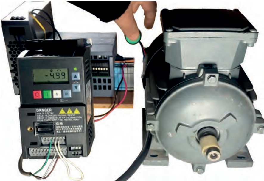
Görsel 5.7: Üç fazlı asenkron motor devir yönü değiştirme sürücü ve PLC bağlantıları
