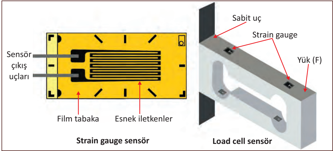
Görsel 1.33: Strain Gauge ve Load Cell basınç sensörleri
