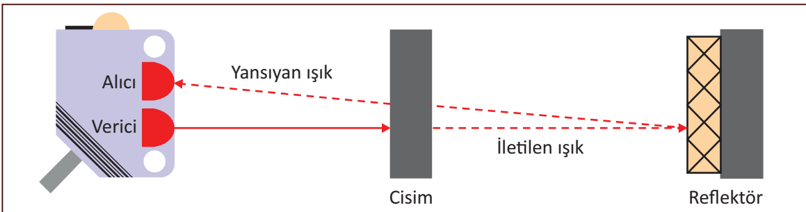
Görsel 1.16: Reflektörden yansımali optik sensörler
