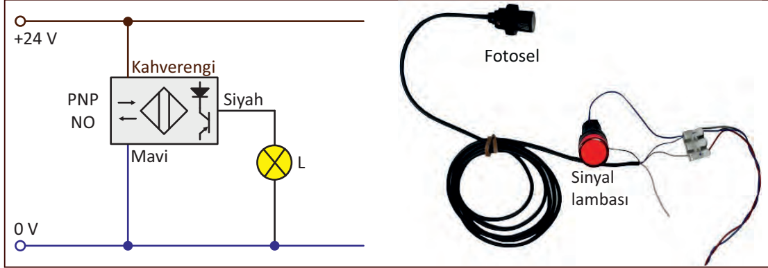
Görsel 1.19: Fotosel sensör devre bağlantısı
