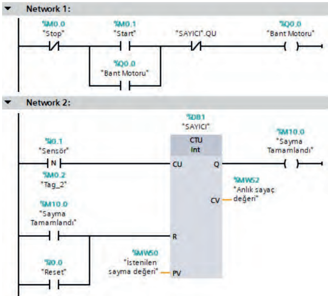
Görsel 4.38: PLC programı
