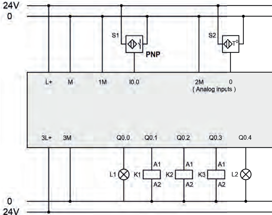
Görsel 3.41: PLC bağlantı şeması
