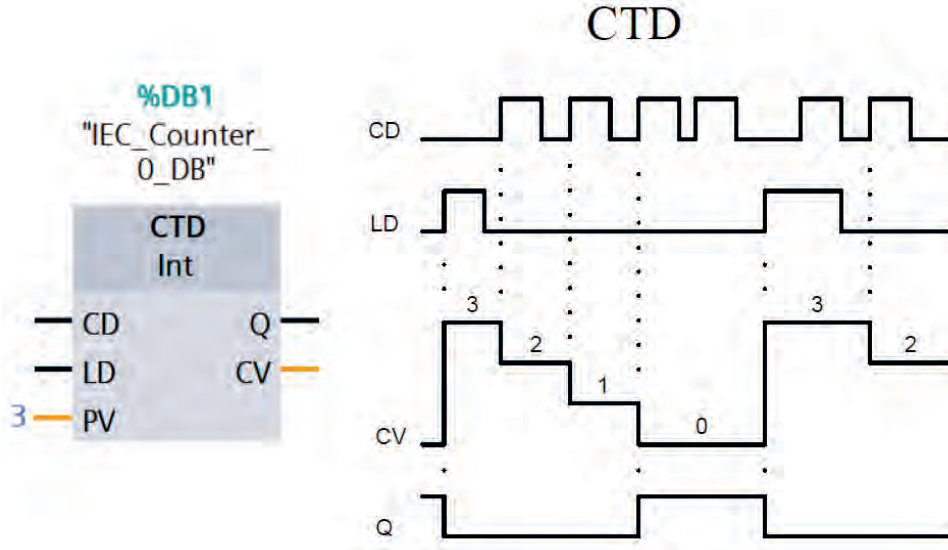
Görsel 3.24: Aşağı sayıcı sembolü ve çalışma grafiği
