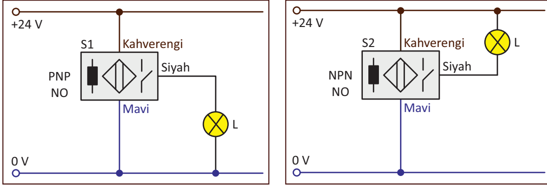
Görsel 1.9: PNP ve NPN endüktif yaklaşım sensörü devre bağlantıları
