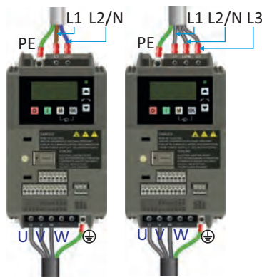
Görsel 5.1: Bir ve üç fazlı sürücülerin motor bağlantıları
