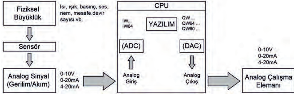
Görsel 3.37: Analog sinyallerin PLC'de işlenmesi
