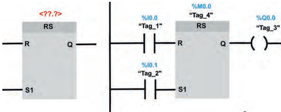
Görsel 3.16: SET (S1) öncelikli flip flop sembolü ve örnek bağlantısı
