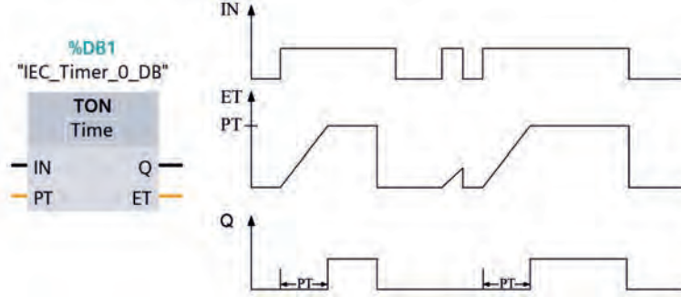
Görsel 3.19: TON tipi zamanlayıcı sembolü ve zaman grafiği
