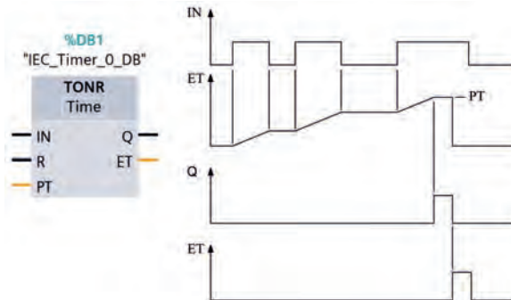
Görsel 3.21: TONR tipi zamanlayıcı sembolü ve zaman grafiği
