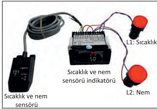
Görsel 1.30: Sıcaklık ve nem sensörü indikatör bağlantısı
