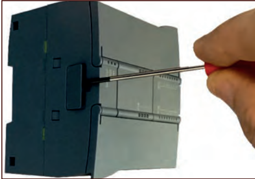
Görsel 2.15: Haberleşme modülü montajı
