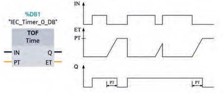
Görsel 3.20: TOF tipi zamanlayıcı sembolü ve zaman grafiği
