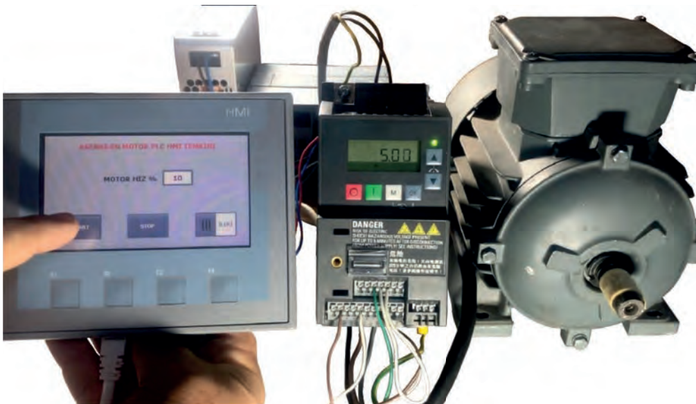
Görsel 5.11: Asenkron motor sürücü PLC ve HMI bağlantıları
