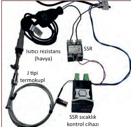
Görsel 1.32: SSR sıcaklık kontrol cihazı ve elemanlarının bağlantısı
