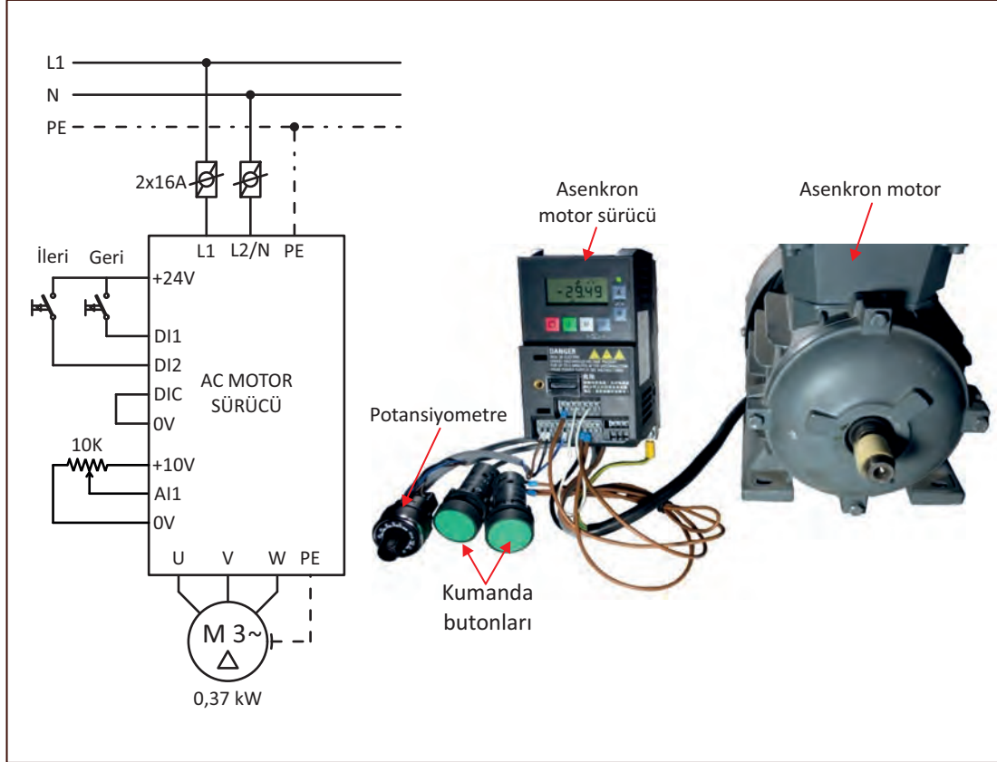
Görsel 5.3: Üç fazlı asenkron motor sürücü, buton ve potansiyometre bağlantıları
