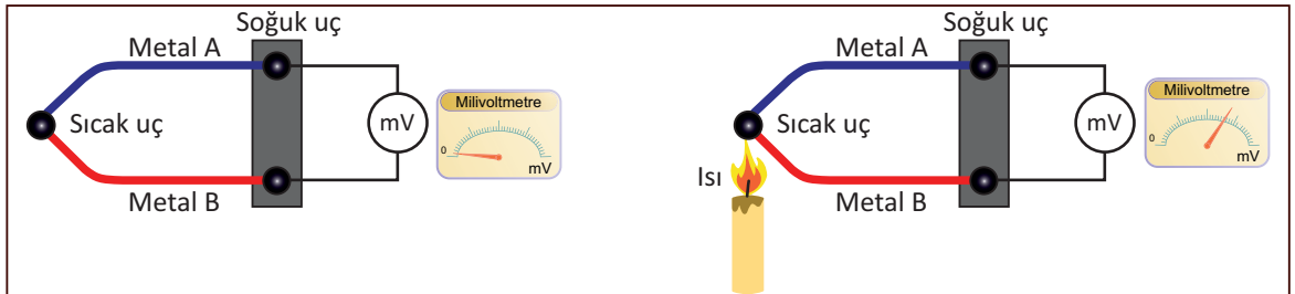
Görsel 1.27: Termokuplun yapısı ve ısıtılması
