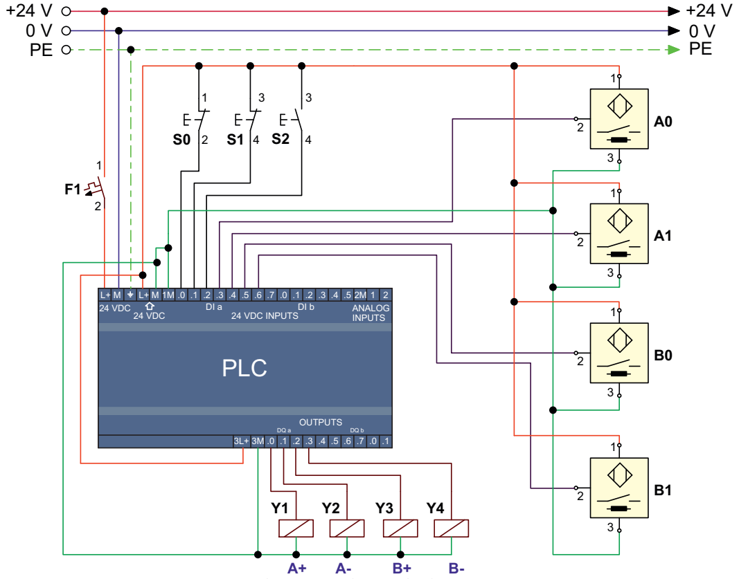
Görsel 3.43: PLC kumanda devre şeması
