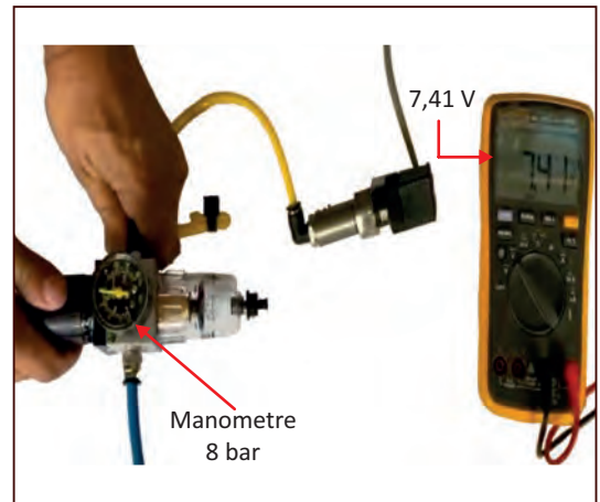
Görsel 1.42: Sıcaklık ve basınç sinyal dönüştürücü elemanlarının bağlantısı
