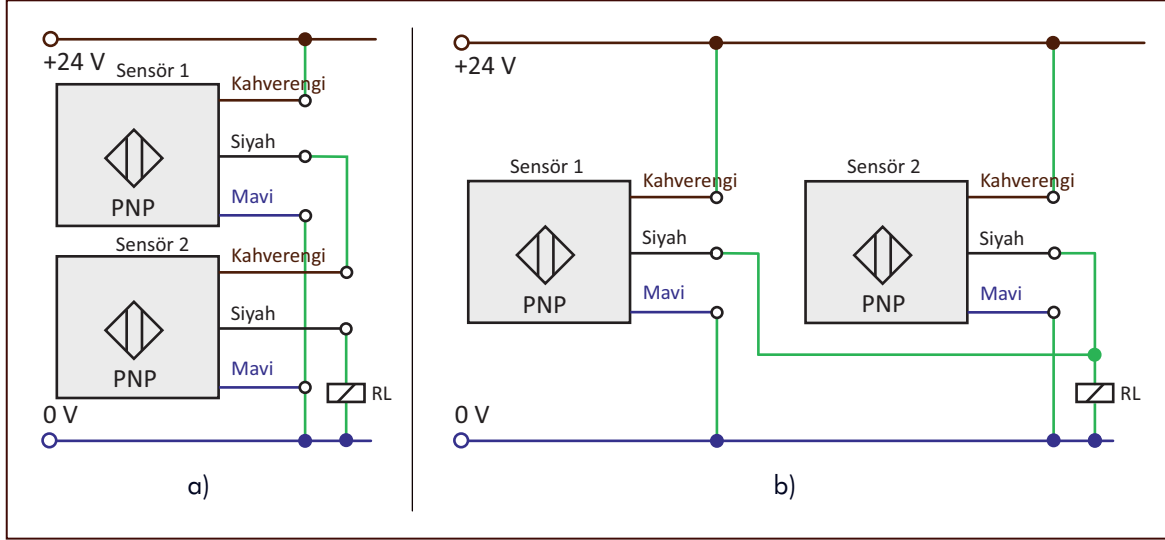
Görsel 1.4a-b: Sensörlerin seri ve paralel bağlantısı
