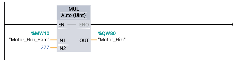
Görsel 5.12: PLC analog modül kontrol program bloğu
