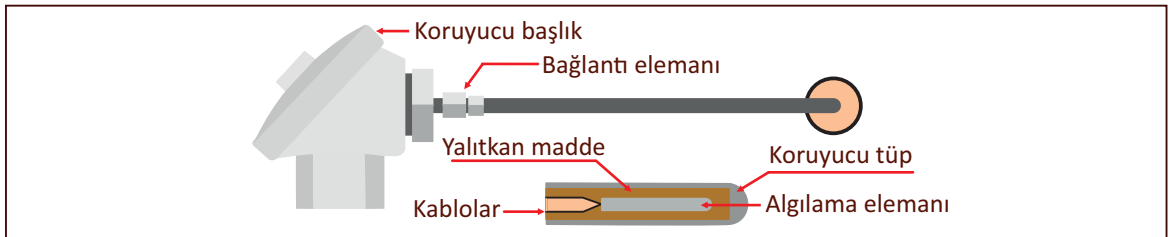
Görsel 1.28: Direnç sıcaklık dedektörünün yapısı
