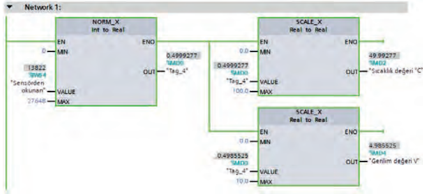
Görsel 3.38: Analog sinyallerin işlenmesi
