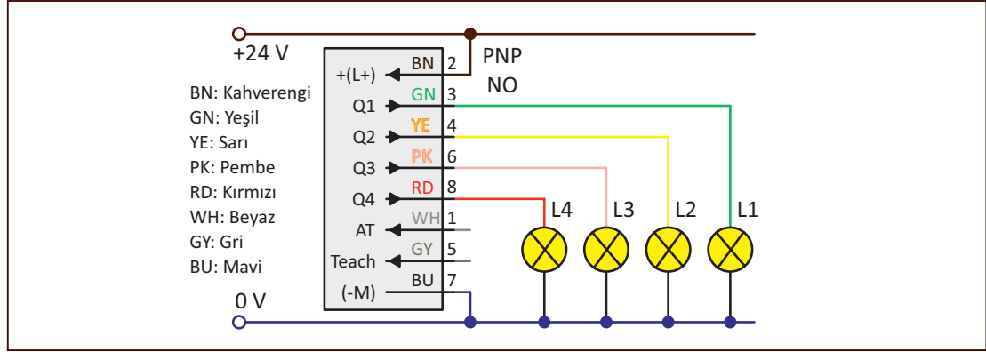
a) Renk sensörü bağlantı şeması
