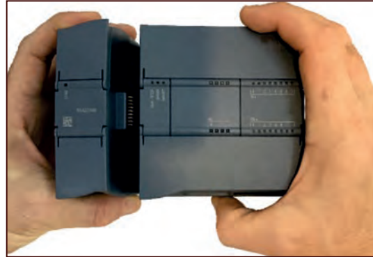
Görsel 2.15: Haberleşme modülü montajı
