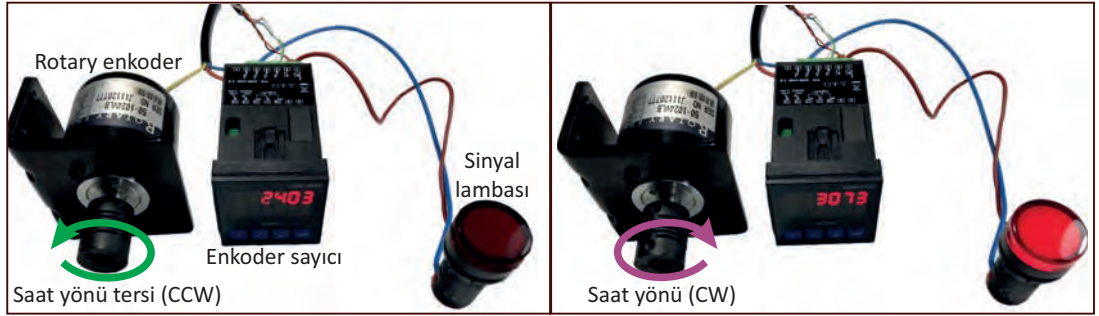
Görsel 1.25: Enkoder sayıcı şema ve bağlantıları
