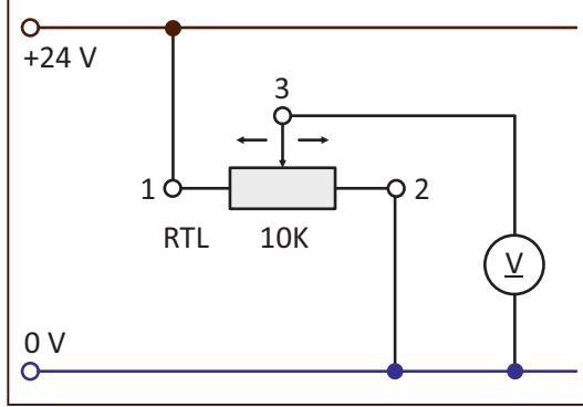
Görsel 1.40: Lineer potansiyometrik cetvel ve devre bağlantısı
