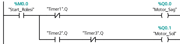
Görsel 5.8: Üç fazlı asenkron motor devir yönü değiştirme PLC program bloğu
