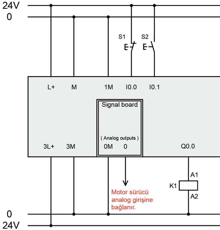
Görsel 3.42: PLC bağlantı şeması
