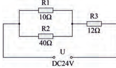
Görsel 3.32: Karışık bağlı direnç devresi
