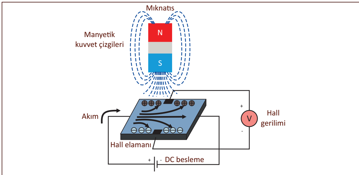
Görsel 1.12: Hall sensörü ve sensörün devreye bağlanması
