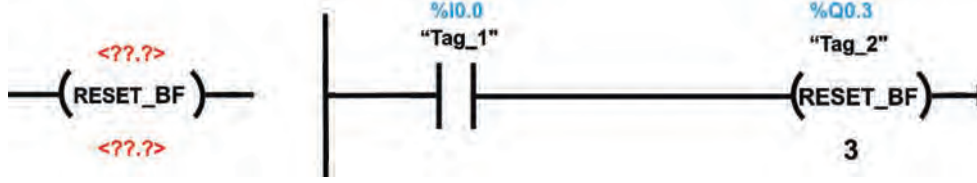
Görsel 3.14: RESET_BF sembolü ve örnek bağlantısı
