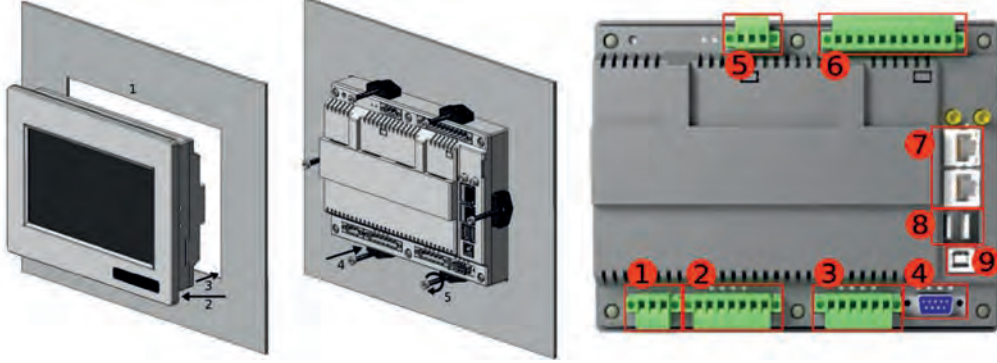
Görsel 4.4: Operatör panelinin montajı ve panelin bağlantısı
