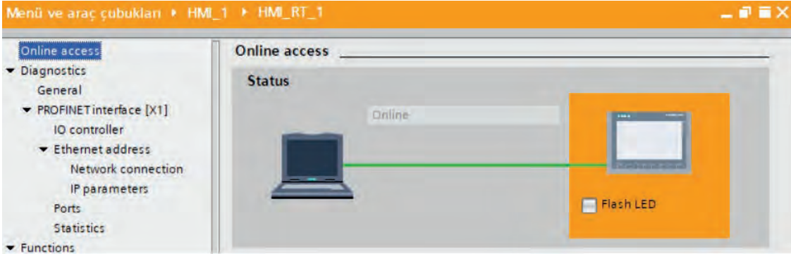
Görsel 4.15: Bilgisayar ile panel arasında çevrim içi bağlantı kurulması
