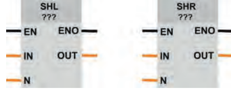
Görsel 3.34: SHL (sola kaydırma) ve SHR (sağa kaydırma) komutları sembolleri
