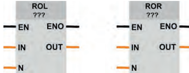
Görsel 3.35: ROL (sola döndürme) ve ROR (sağa döndürme) komutları sembolleri
