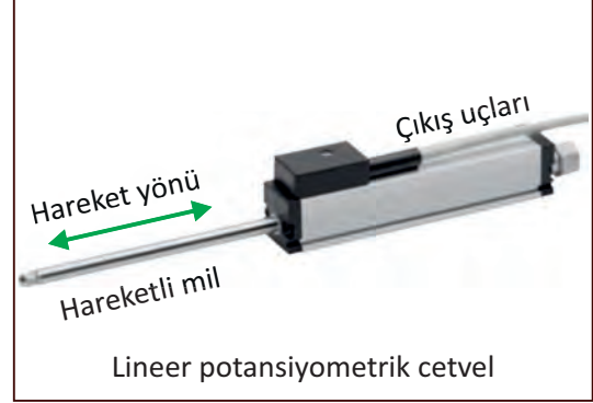
Görsel 1.40: Lineer potansiyometrik cetvel ve devre bağlantısı
