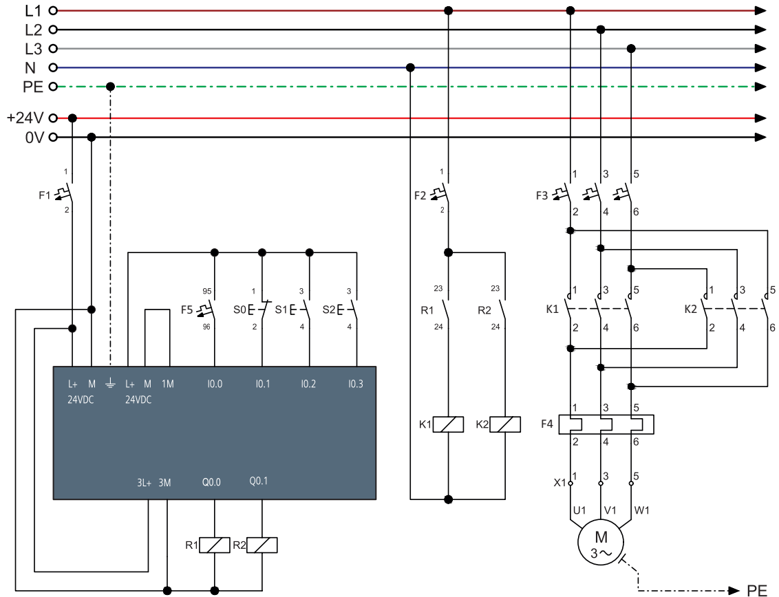
Görsel 2.8: Dâhilî rölesiz PLC alıcı bağlantısı (PNP bağlantı)
