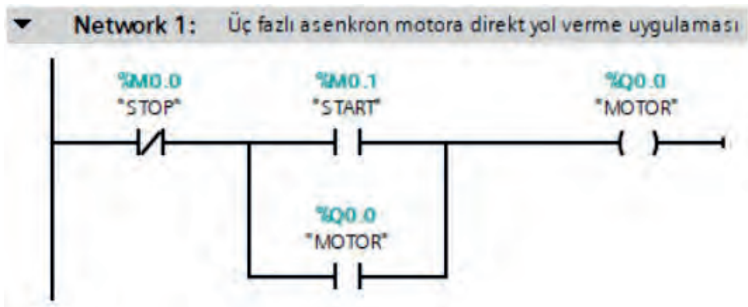
Görsel 4.24: Üç fazlı asenkron motora direkt yol verme ladder diyagramı
