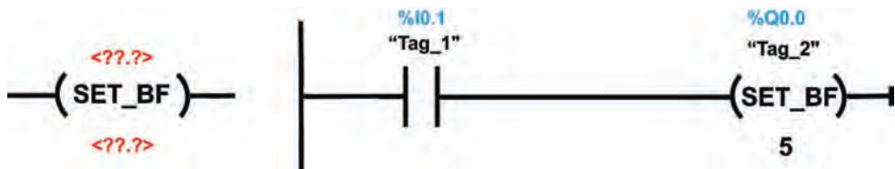
Görsel 3.13: SET_BF sembolü ve örnek bağlantısı
