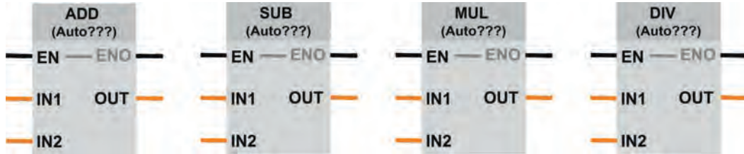
Görsel 3.30: Toplama, çıkarma, çarpma ve bölme işlemleri sembolleri
