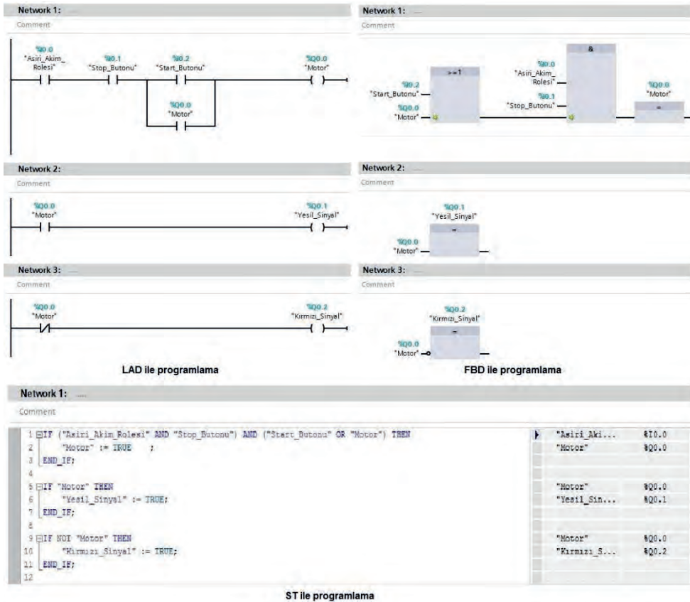
Görsel 3.2: Devrenin LD, FBD ve ST diyagramları
