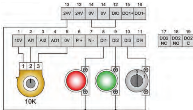
Görsel 5.2: Sürücü terminallerine kontrol elemanlarının bağlantısı
