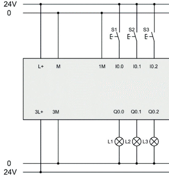
Görsel 3.10: PLC bağlantı şeması
