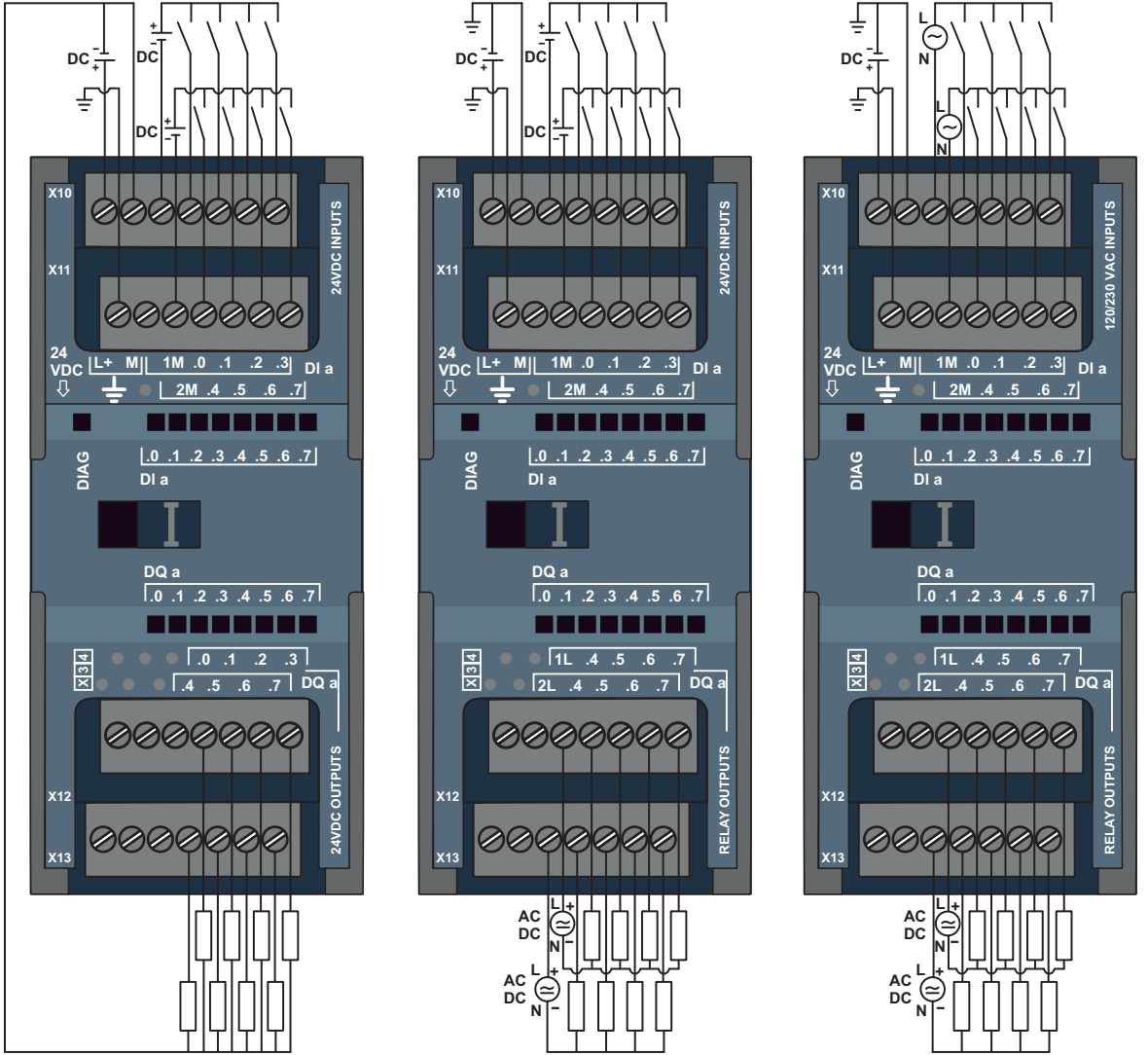
Görsel 2.12: PLC dijital giriş-çıkış modülleri ve bağlantıları
