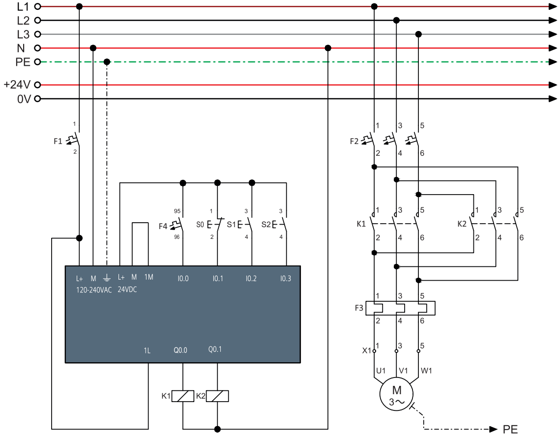
Görsel 2.9: Dâhilî röleli PLC alıcı bağlantısı
