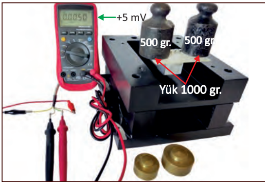
Görsel 1.35: Yük hücresi devre bağlantısı ve avometreyle çıkış gerilimi ölçümü
