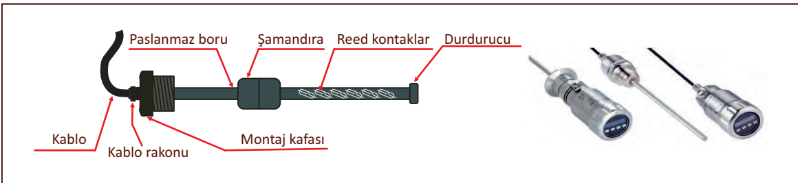
Görsel 1.39: Seviye sensörü yapısı
