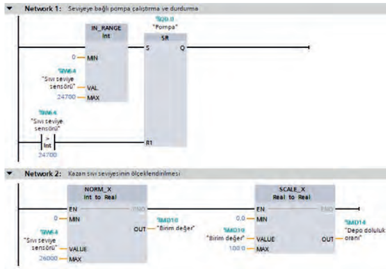
Görsel 4.42: PLC programı
