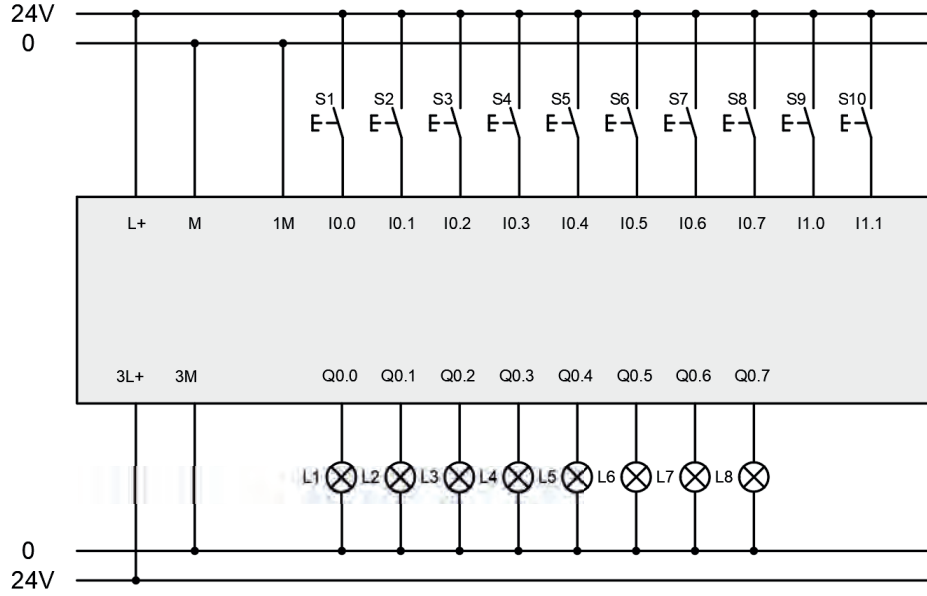
Görsel 3.9: PLC bağlantı şeması
