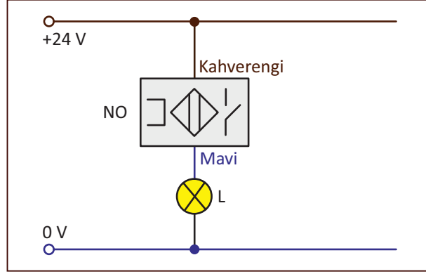
Görsel 1.13: Manyetik yaklaşım sensörü devre bağlantıları
