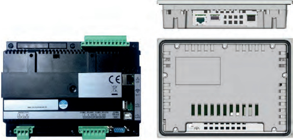
Görsel 4.3: Farklı operatör panellerine ait haberleşme portları ve bağlantı klemensleri
