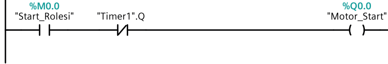
Görsel 5.6: Üç fazlı asenkron motorun periyodik çalışma PLC program bloğu
