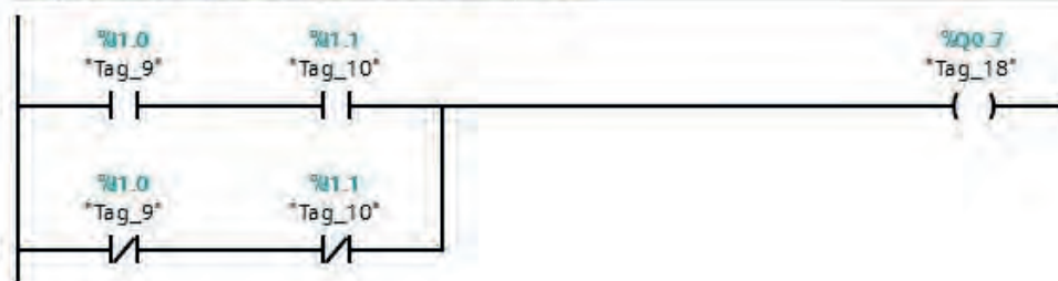
Network 8: ÖZEL VEYA DEĞİL KAPISI (XNOR GATE)
