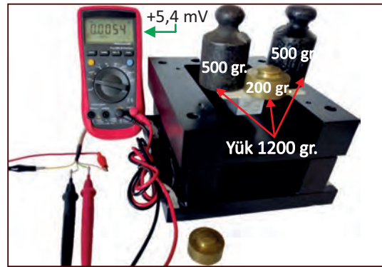
Görsel 1.35: Yük hücresi devre bağlantısı ve avometreyle çıkış gerilimi ölçümü
