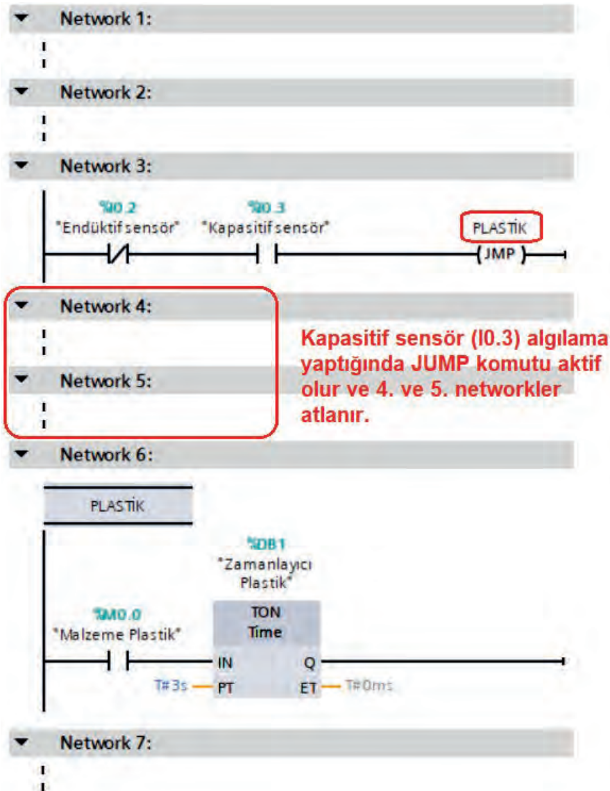
Görsel 3.36: Jump ve label komutlarının kullanımı
