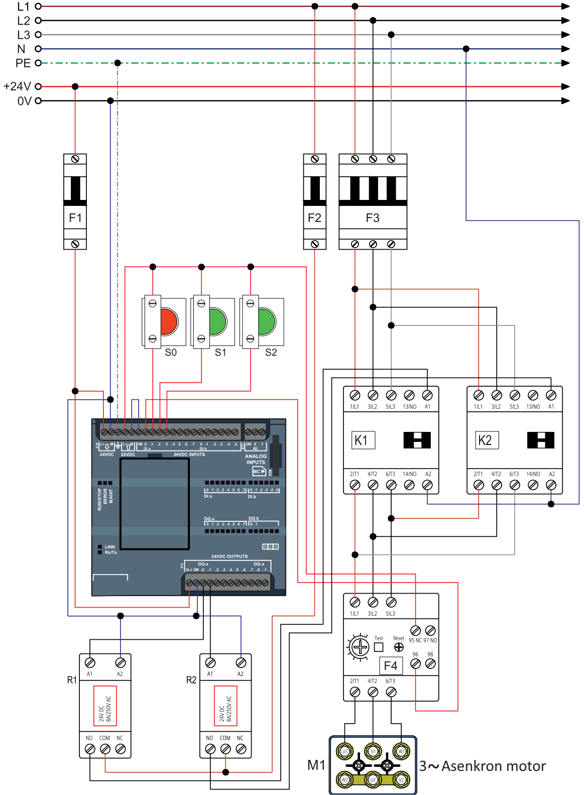
Görsel 2.10: Çıkışı rölesiz PLC ile devir yönü değiştirme devresi açık bağlantı şeması
