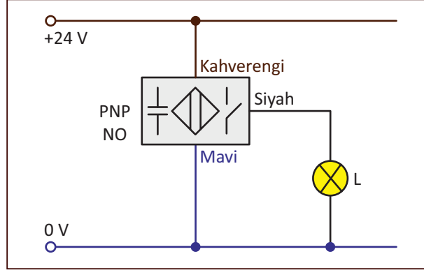
Görsel 1.10: Kapasitif yaklaşım sensörü devre bağlantıları
