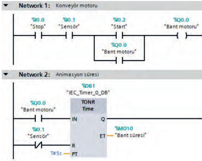
Görsel 4.50: PLC programı
