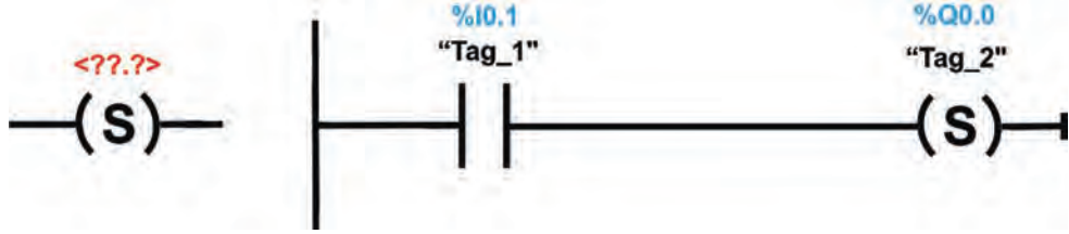
Görsel 3.11: SET çıkış rölesi sembolü ve örnek bağlantısı
