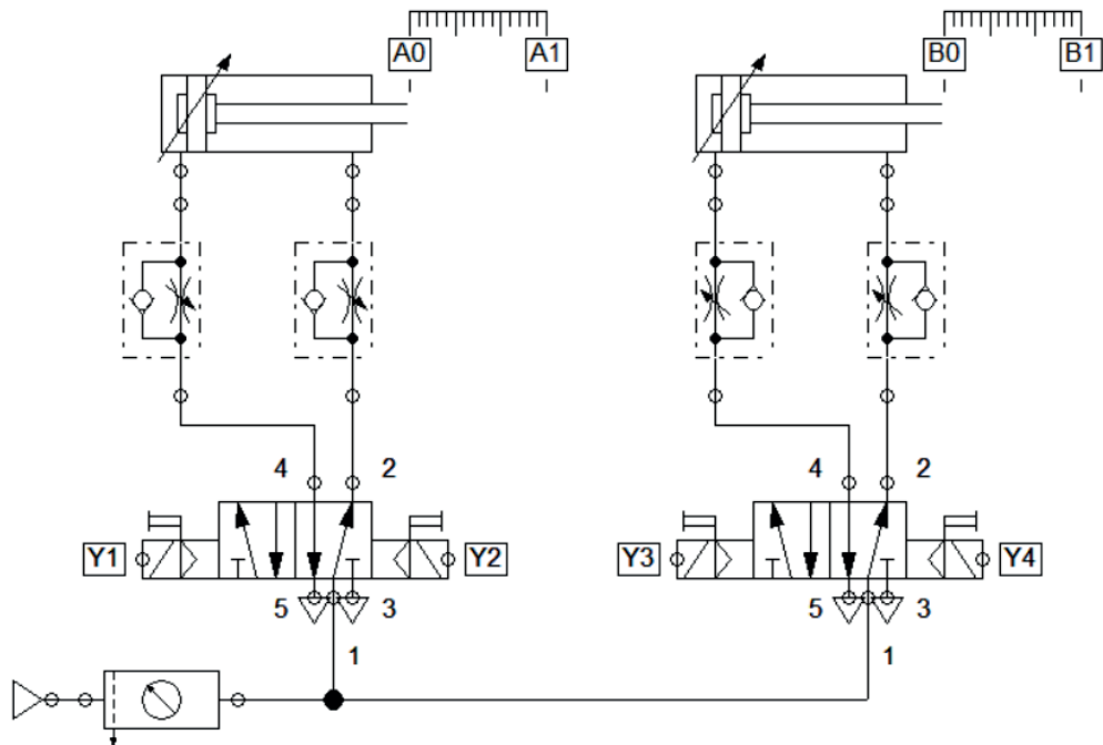
Görsel 3.44: Elektropnömatrik devre şeması
