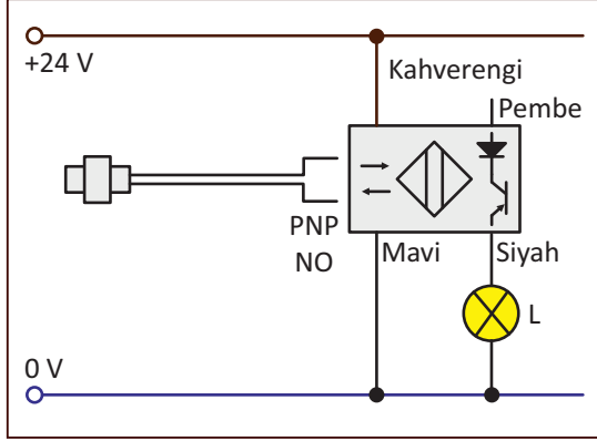
a) Fiber optik sensör devre şeması
