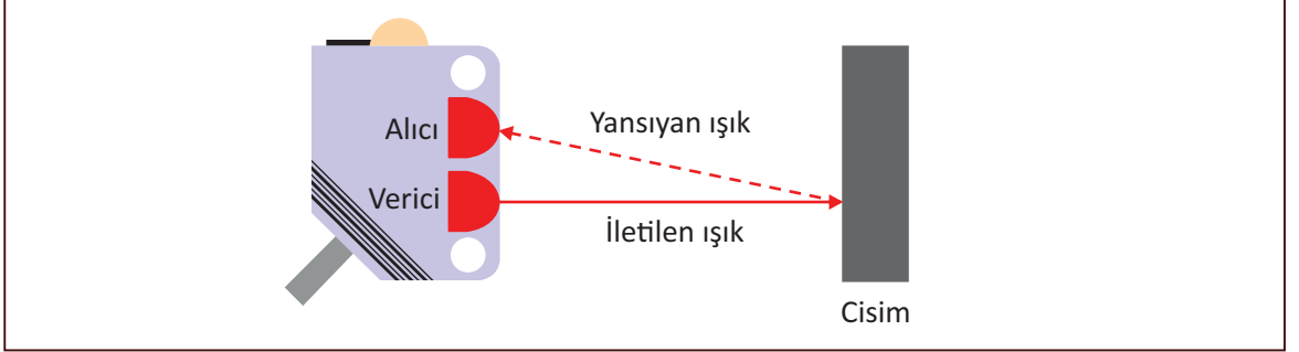
Görsel 1.17: Cisimden yansımali optik sensörler
