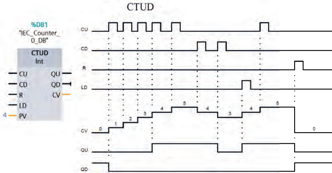
Görsel 3.25: Yukarı-aşağı sayıcı sembolü ve çalışma grafiği
