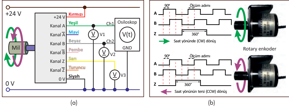
Görsel 1.24: Rotary enkoder devre bağlantısı ve çıkış sinyalleri
