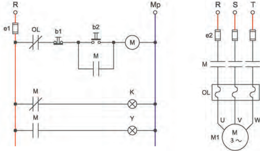
Görsel 3.1: Üç fazlı asenkron motorun sürekli çalışması (ANSI)
