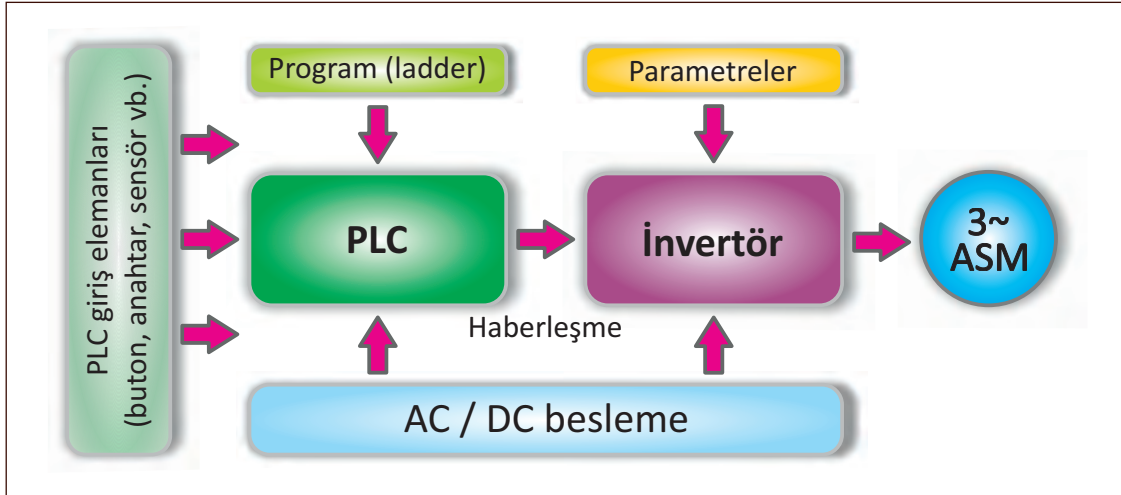
Görsel 5.4: PLC ve invertör bağlantısı prensip şeması
