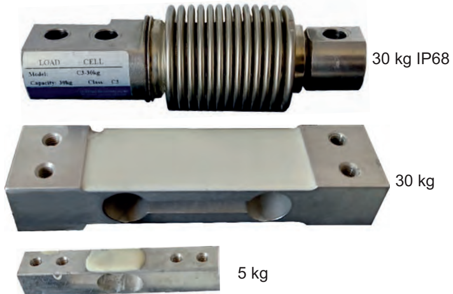
Görsel 1.34: Load cell çeşitleri
