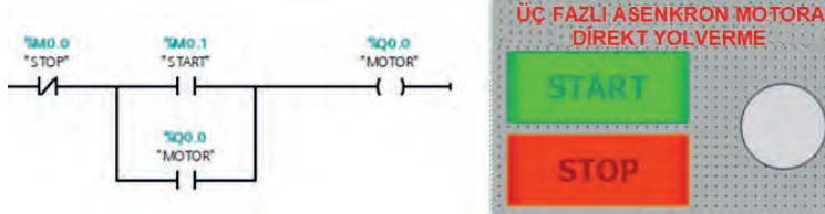
Görsel 4.28: PLC programı ve panel görünümü
