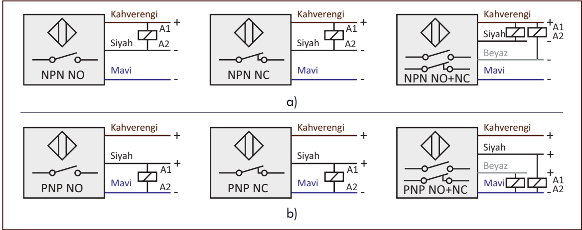
Görsel 1.3a-b: NPN-PNP sensörler ve bu sensörlerin kontak durumları
