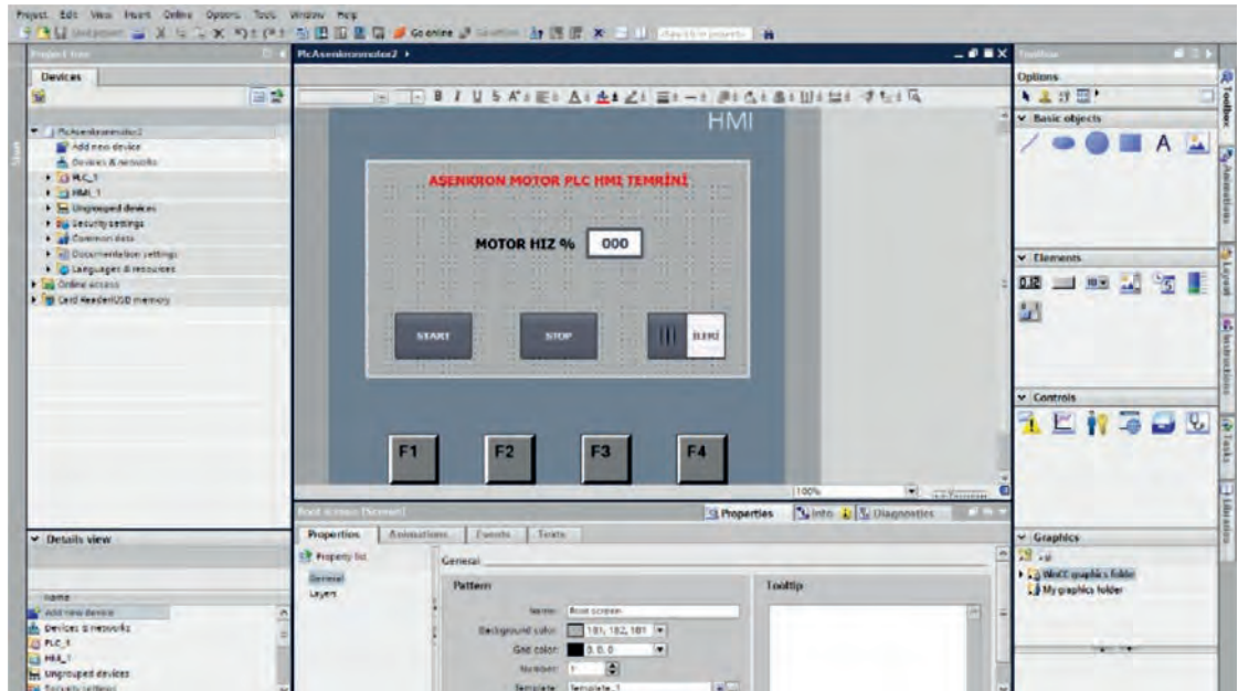
Görsel 5.13: Operatör paneli tasarım görüntüsü
