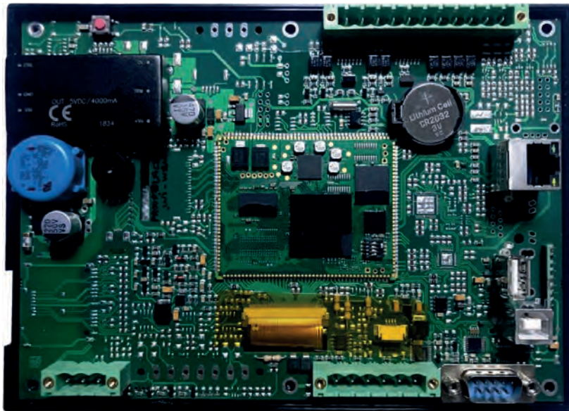
Görsel 4.2: Operatör panelinin iç yapısı
