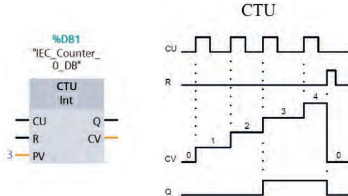
Görsel 3.23: Yukarı sayıcı sembolü ve çalışma grafiği
