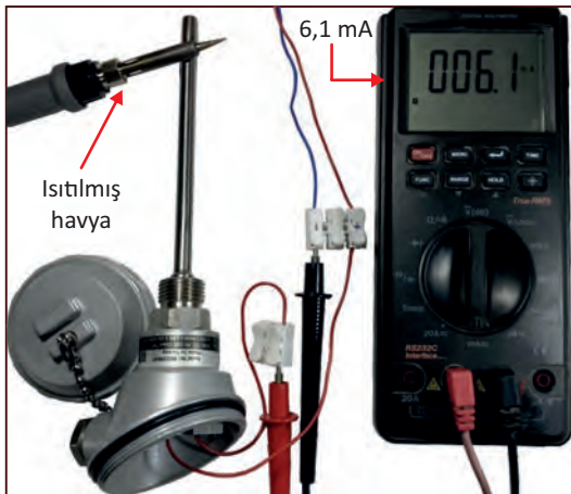
Görsel 1.42: Sıcaklık ve basınç sinyal dönüştürücü elemanlarının bağlantısı
