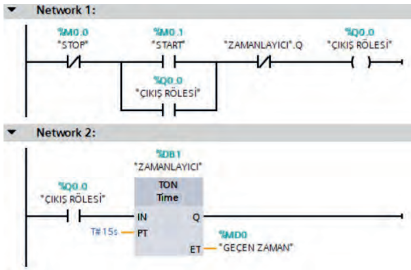
Görsel 4.33: PLC programı
