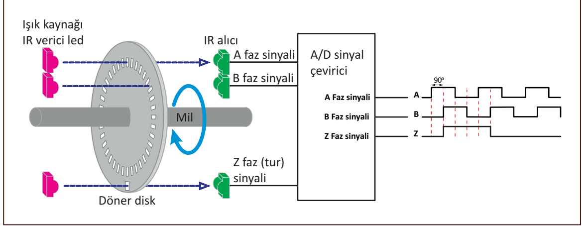
Görsel 1.22: Enkoder bağlantısı
