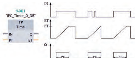
Görsel 3.18: TP tipi zamanlayıcı sembolü ve zaman grafiği
