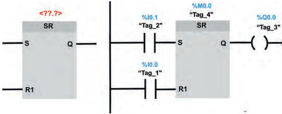
Görsel 3.15: RESET (R1) öncelikli flip flop sembolü ve örnek bağlantısı
