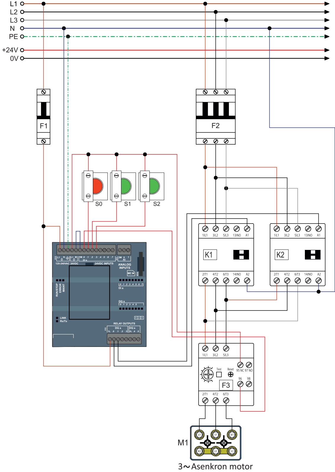
Görsel 2.11: Çıkışı dâhilî röleli PLC ile devir yönü değiştirme devresi açık bağlantı şeması
