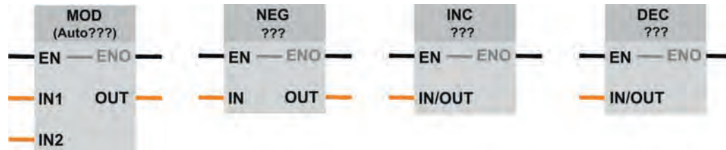
Görsel 3.31: Mod, negatifini alma, arttırma, azaltma işlemleri sembolleri
