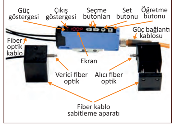
b) Fiber optik sensör elemanları
