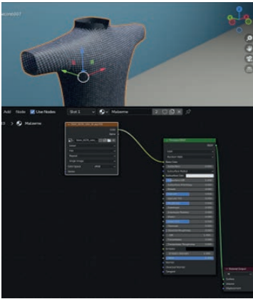
Görsel 4.83: Shader Editör bölümünde özellik haritalarının bağlanması
