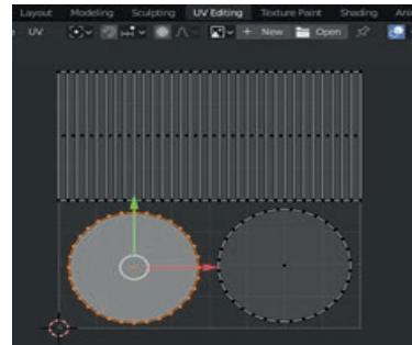
Görsel 4.59: Unwrap yapılarak UV Editing görünümünde şeklin UVMaap açılmış hâli
