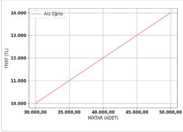
Grafik 2.3: Arz eğrisi
