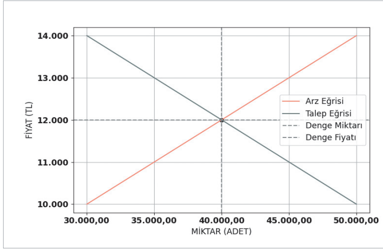
Grafik 2.5: Piyasa dengesi
