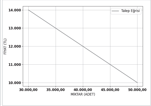
Grafik 2.4: Talep eğrisi
