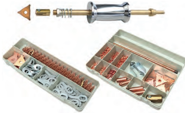
Görsel 3.77: Spot hızlı çekirme cihazı aksesuar seti
