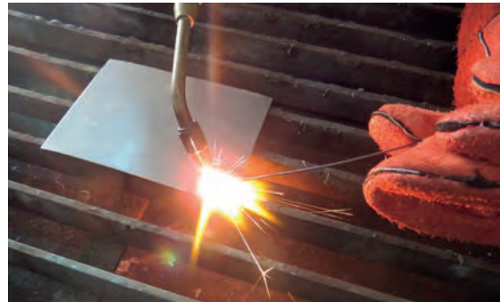
Görsel 1.16: Oksi-gaz kaynağında sağa kaynak uygulaması
