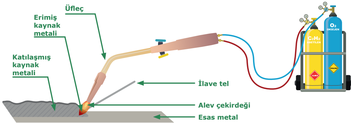
Şekil 1.1: Oksî-gaz kaynağı
