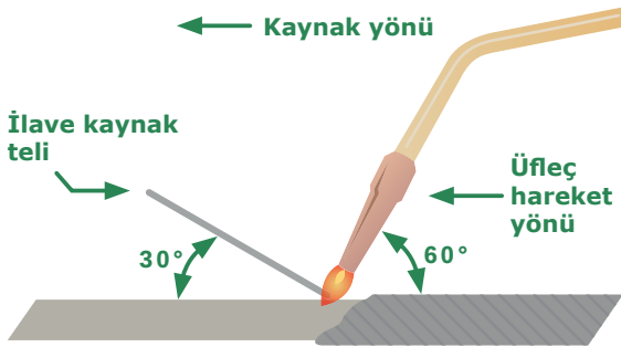
Şekil 1.5: Oksi-gaz kaynağında sola kaynak
