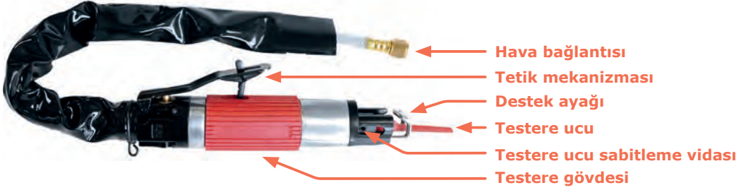
Görsel 2.13: Pnömatik karoseri testeresi ve yapısı
