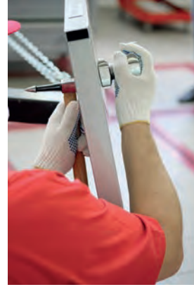
Görsel 5.64: Çekiç dayama yöntemi
