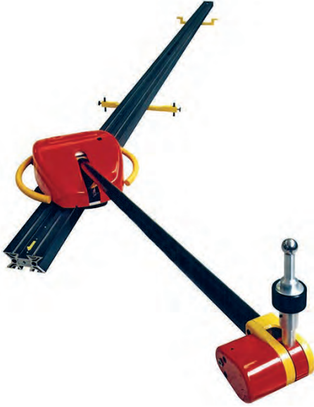
Görsel 4.6: Ölçüm başlığı ve ölçü köprüsü
