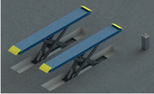
Görsel 3.109: Zemine gömülü tek makaslı lift
