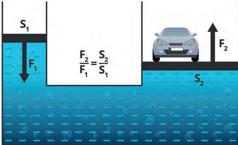
Görsel 4.31: Pascal prensibi
