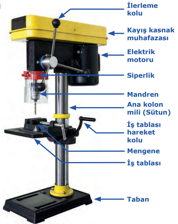
Görsel 3.16: Matkap tezgâhının yapısı
