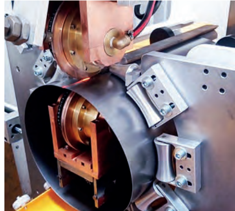
Görsel 1.83: Dikiş kaynağının yapısı
