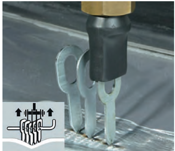
Görsel 3.79: Pul kaynatarak çekirme
