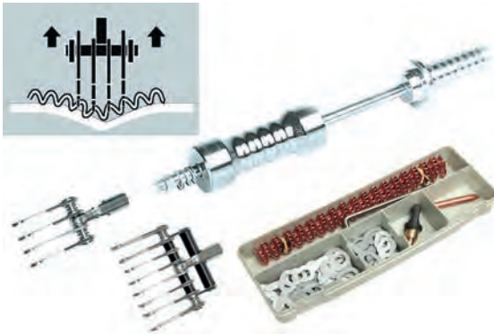
Görsel 3.78: Çok noktadan telli çekirme
