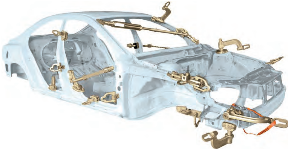
Görsel 5.19: Çeşitli şekillerde bağlanan kurt ağızları
