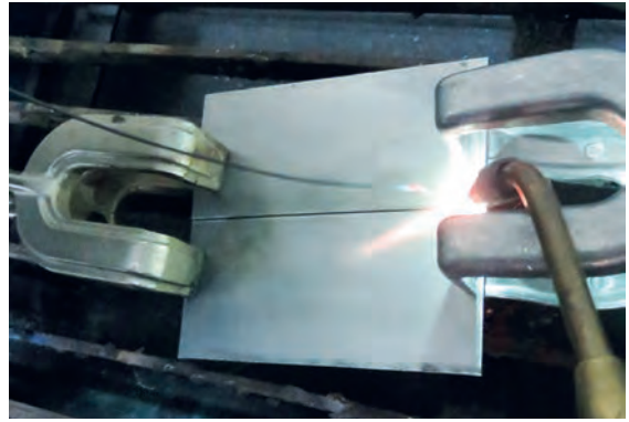
Görsel 1.17: Oksi-gaz kaynağında sol kaynak uygulaması
