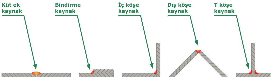
Şekil 1.6: Kaynak birleştirme pozisyonları
