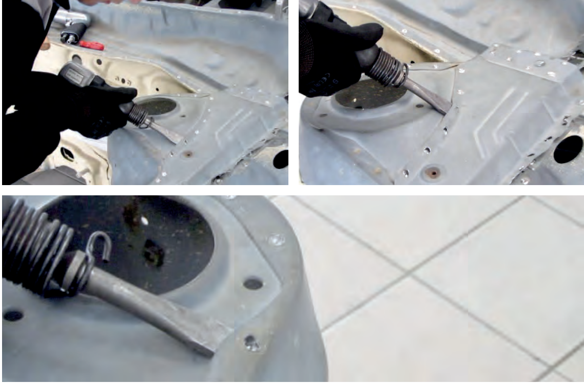
Görsel 2.46: Pnömatik keski ile parça ayırma işlemleri
