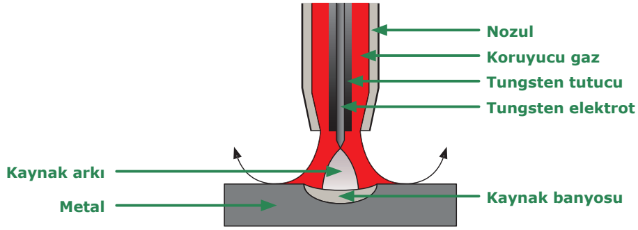
Şekil 1.11: TIG kaynağı çalışma prensibi
