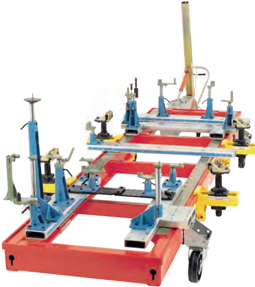
Görsel 4.19: Kalıplı sistem düzeltme tezgâhı
