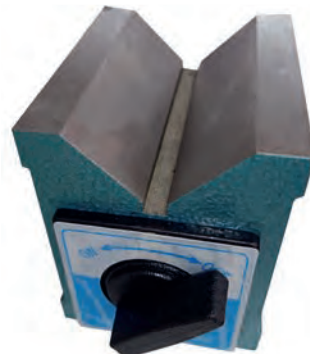
Görsel 5.45: Manyetik V yatağı
