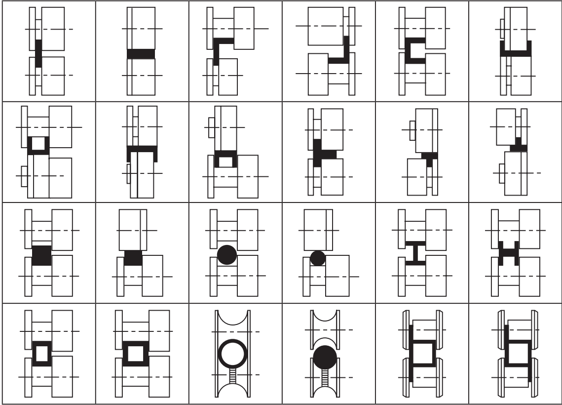
Şekil 5.3: Farklı profil yapısına sahip malzemelerin bükülmesi için kullanılan makara çeşitleri
