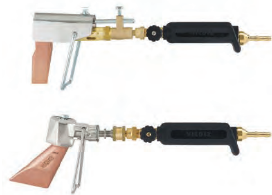
Görsel 1.111: Havyalı propan hamlaçları
