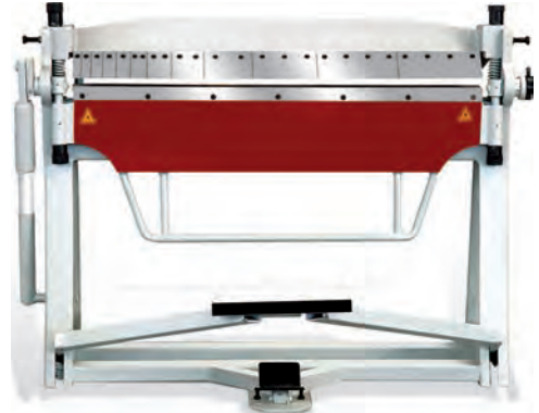
Görsel 5.33: Parçalı bıçaklı sac kıvrma makinesi
