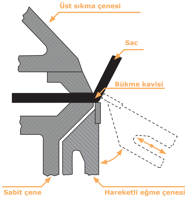
Şekil 5.4: Sac kıvrma makinesi çeneleri
