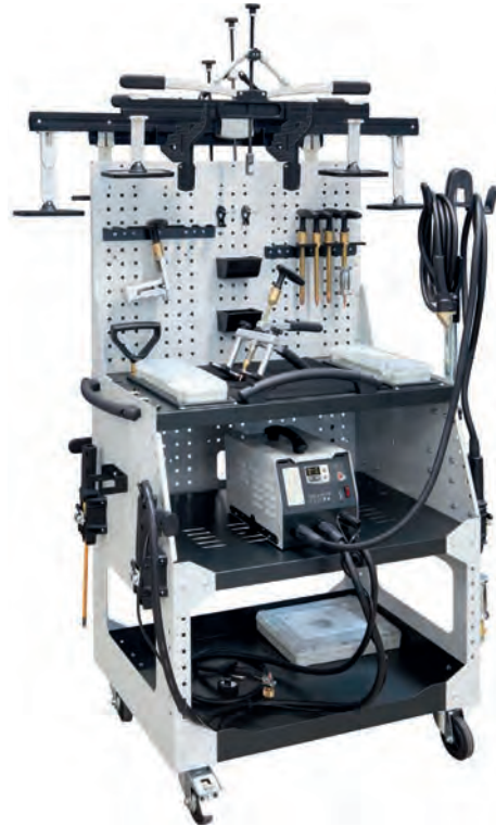
Görsel 3.83: Spot hızlı çekirme seti
