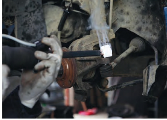
Görsel 3.58: Rot başı somununun ısıtılması
