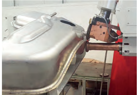
Görsel 1.54: Yakıt deposunun dikiş kaynağı yapılması
