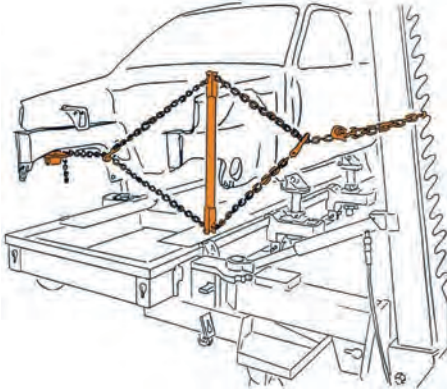
Görsel 4.28: İtme pistonu kullanılarak yapılan düzeltme işlemleri
