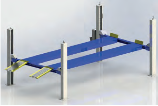
Görsel 3.98: Dört sütunlu liftin yapısı
