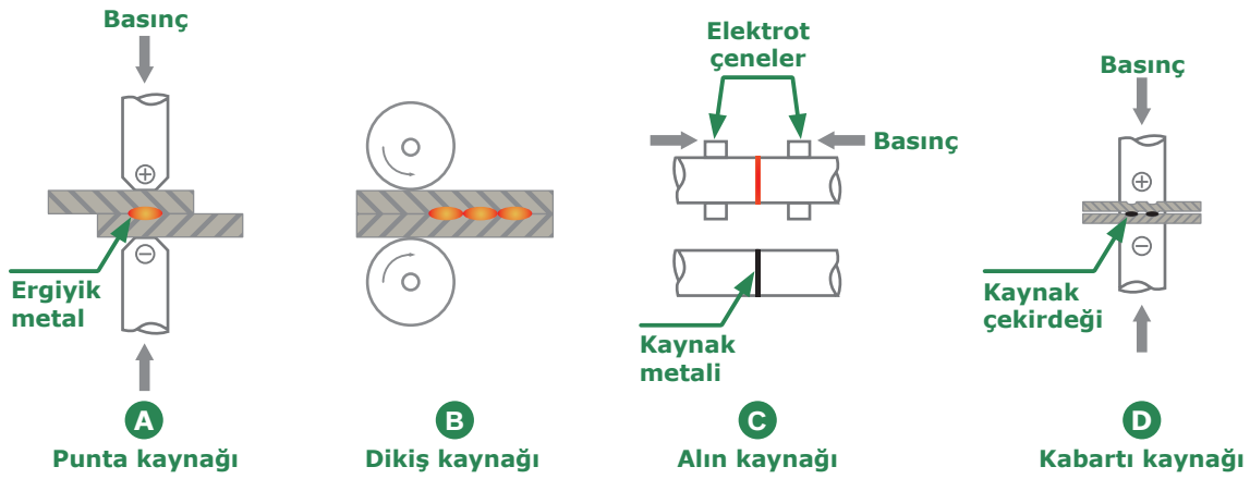
Şekil 1.9: Direnç kaynağı çeşitlerinin çalışma prensipleri
