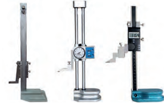
Görsel 5.48: Mihengir çeşitleri
