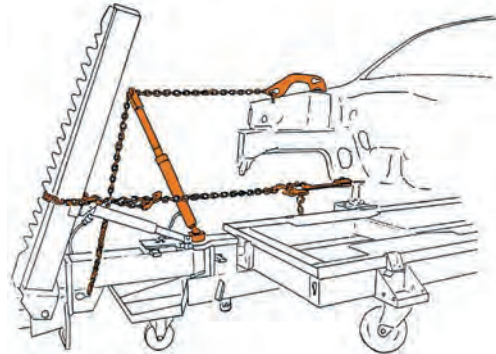
Görsel 4.28: İtme pistonu kullanılarak yapılan düzeltme işlemleri
