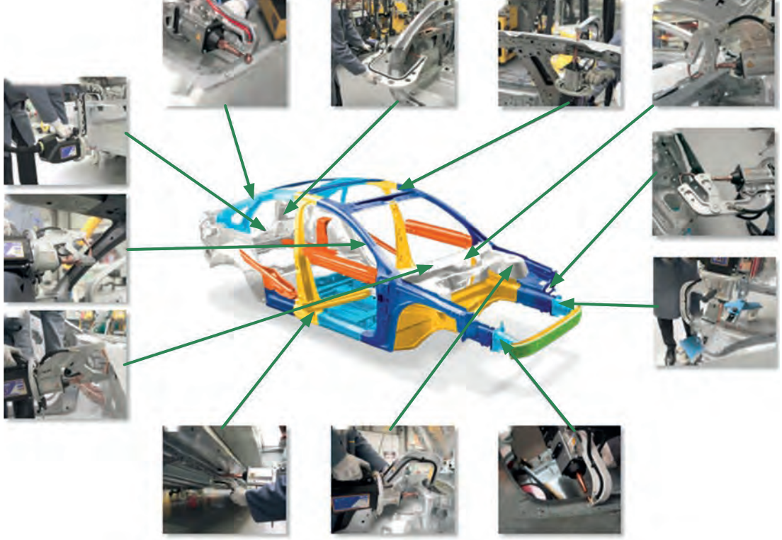
Görsel 1.60: Araç gövdesi üzerinde punta kaynağı ile montaj işlemleri
