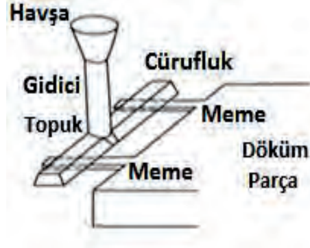
Resim 2.39: Yolluk sistemi
