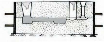
Resim 2.49: Kalıplamada besleyicilerin konumu
