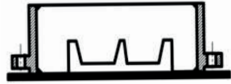
Resim 2.50: Model ve derecenin kalıplama altlığına yerleştirilmesi
