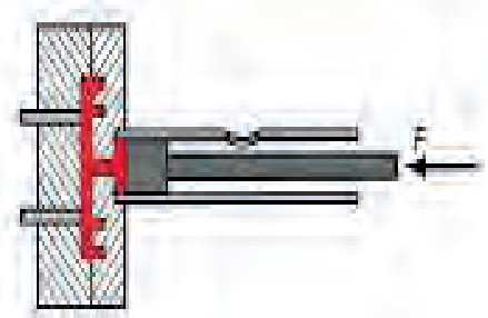
Resim 2.35: Basınçlı döküm sistemi
