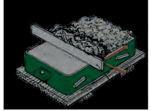
Resim 2.1: Fazla kumun mastarı ile sıyırılması
