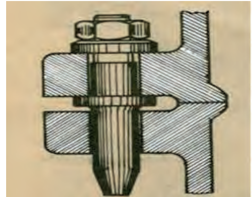
Resim 2.4: Pim, pim delikleri, el sapları
