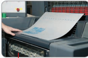
Görsel 2.1: Ofset baskı kalıbı
