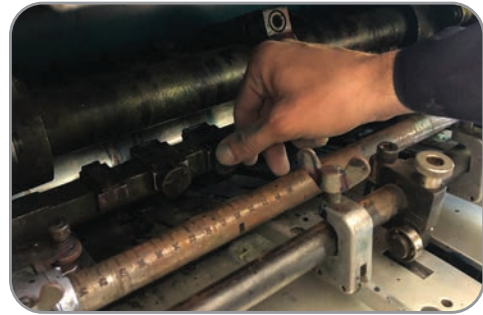
Görsel 6.11: Ön siperin ayarlanması
