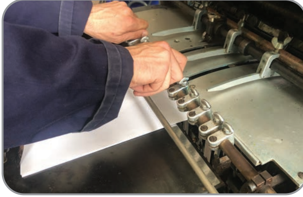
Görsel 5.27: Emicilerin ayarı
