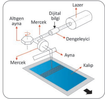
Şekil 2.5: Düz yataklı CTP makinesinin iç kesiti
