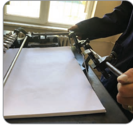
Görsel 6.24: Arka destek demirinin ayarlanması
