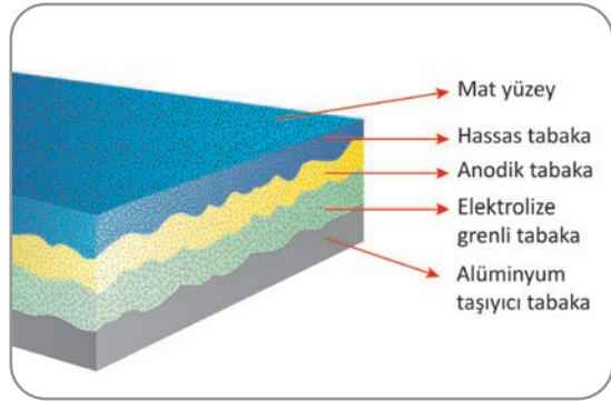
Şekil 2.1: Alüminyum kalıbın katmanları
