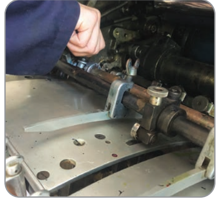
Görsel 6.21: Pozanın ayarlanması
