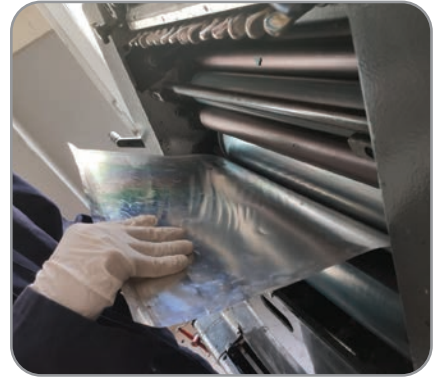
Görsel 5.62: Kalıbın sökülmesi
