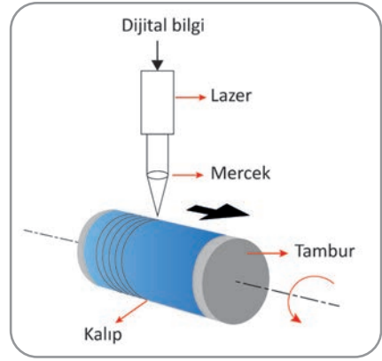
Şekil 2.4: Dış tamburlu CTP makinesinin iç kesiti
