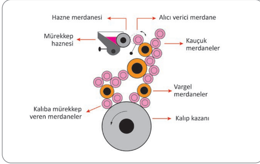
Şekil 3.5: Ofset baskı makinesinin mürekkep ünitesi
