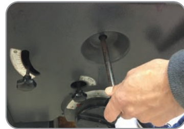
Görsel 4.12: Yan destek demirinin ayarlanması
