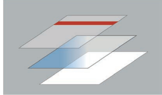
Görsel 3.4: Katmanlar
