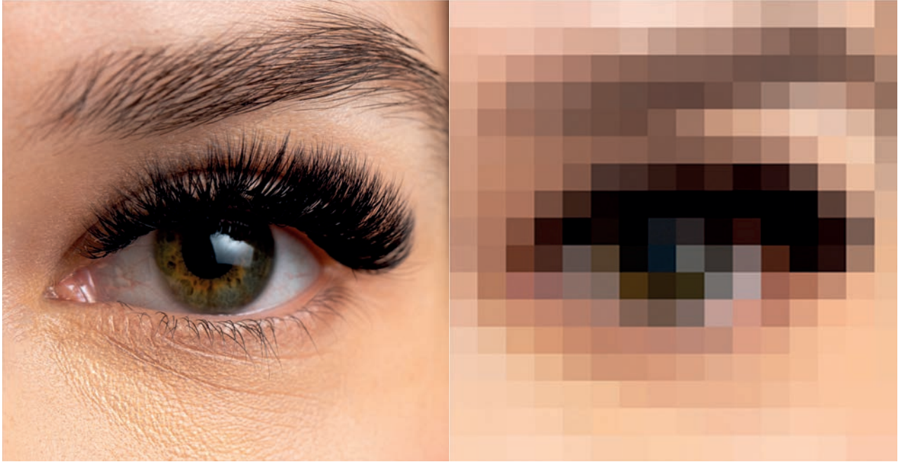
Görsel 1.9: Pikseller
