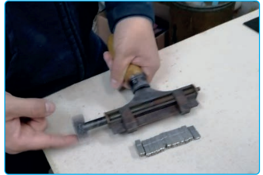
Görsel 4.7: Hurufatların kumpasa dizilmesi
