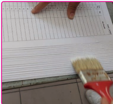
Görsel 6.24: Sırtı elle açarak tutkalın sürülmesi
