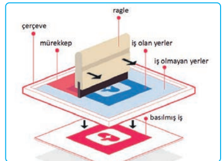
Görsel 4.32: Serigrafi baskı
