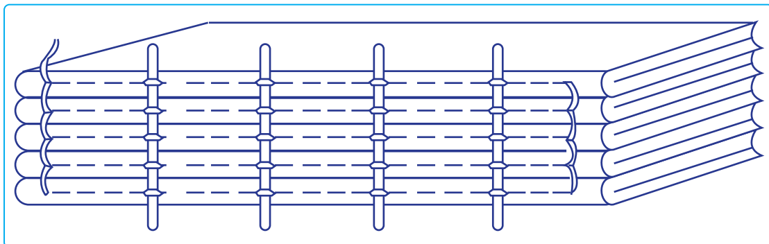
Görsel 1.18: Sicimle esnek dikiş
