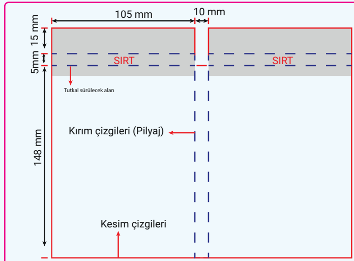
Görsel 5.13: Bloknott kapağı
