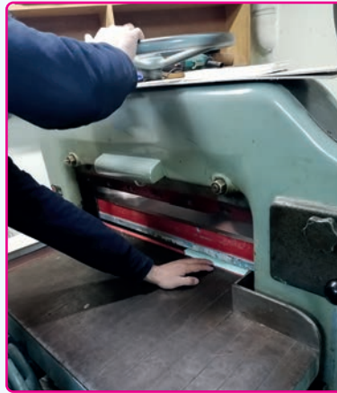
Görsel 2.15: İç bloğun baş kısmının sipere yaslanması
