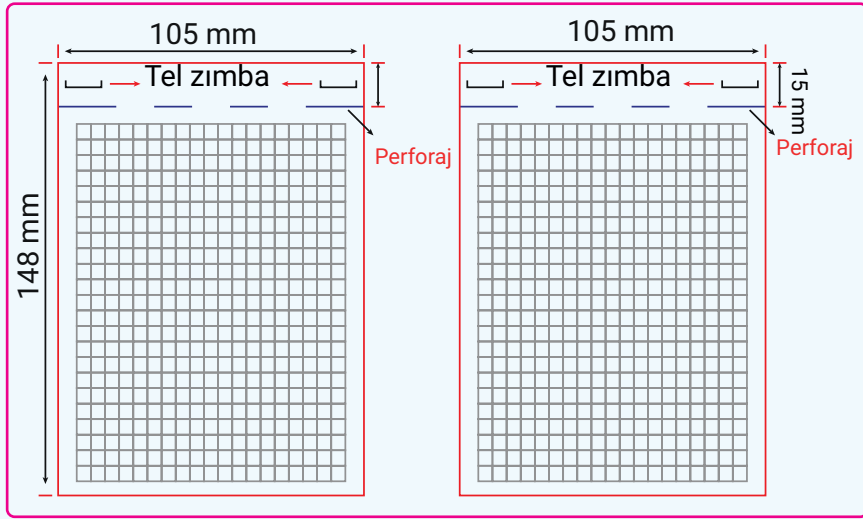
Görsel 5.14: Bloknot iç sayfaların ölçüsü
