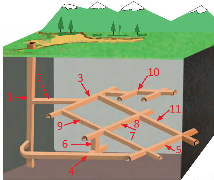
Şekil 1.2: Yer altı maden ocağının genel görünüşü
