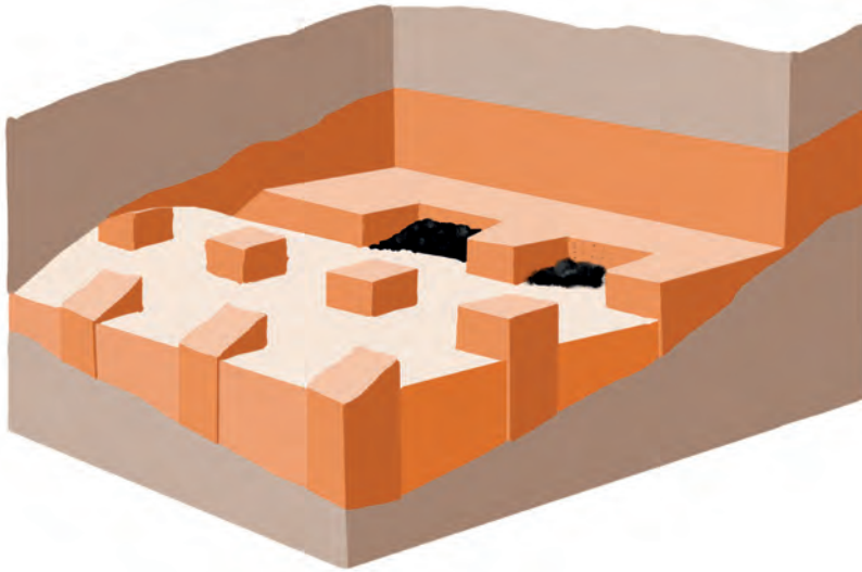
Şekil 4.1: Oda topuk yöntemi
