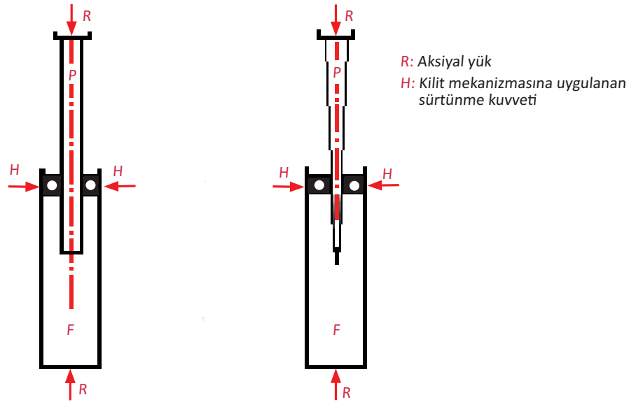
Şekil 7.5: Teleskopik direk
