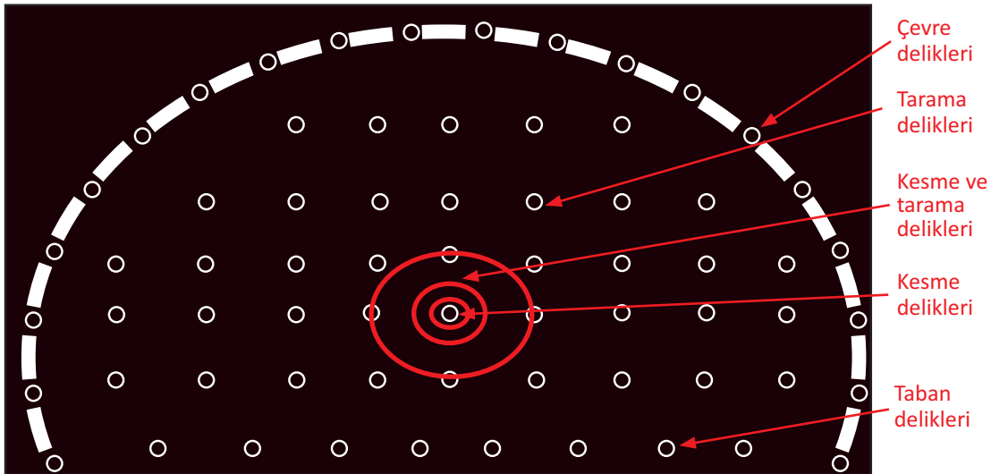
Şekil 1.8: Yer altı maden patlatma aynası delik tipleri
