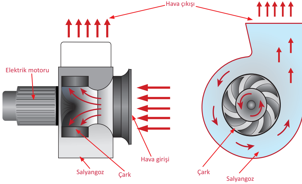
Şekil 3.2: Radyal ventilatörünün kesiti ve yandan görünüşü
