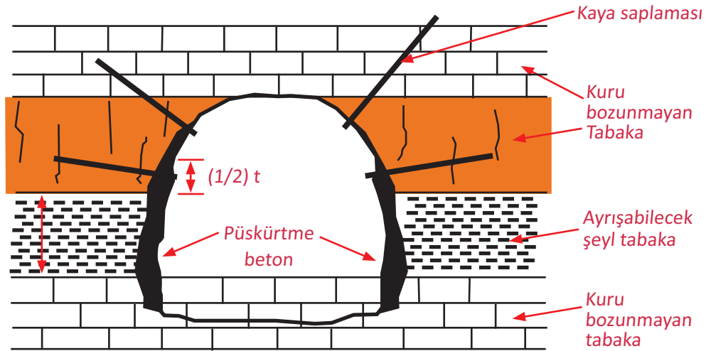
Şekil 7.4: Kaya saplama
