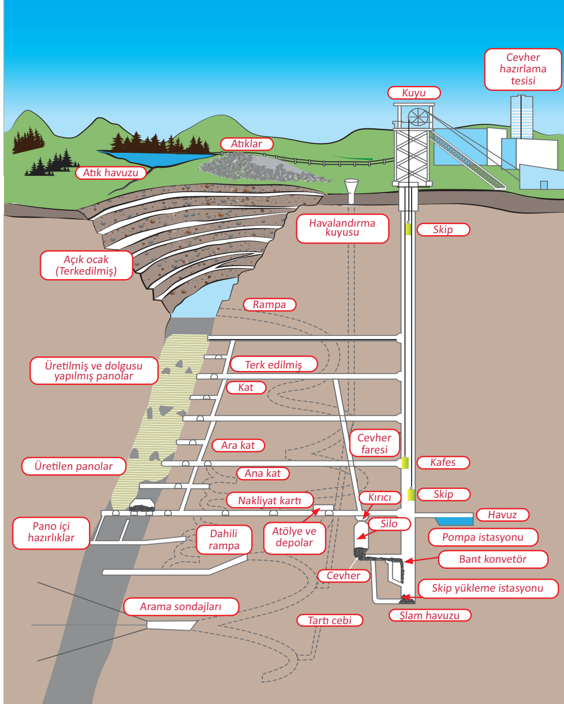
Şekil 4.9: Yer altı madenciliğinden bir kesit
