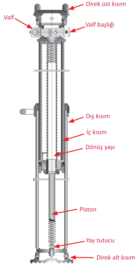
Şekil 7.6: Hidrolik direk
