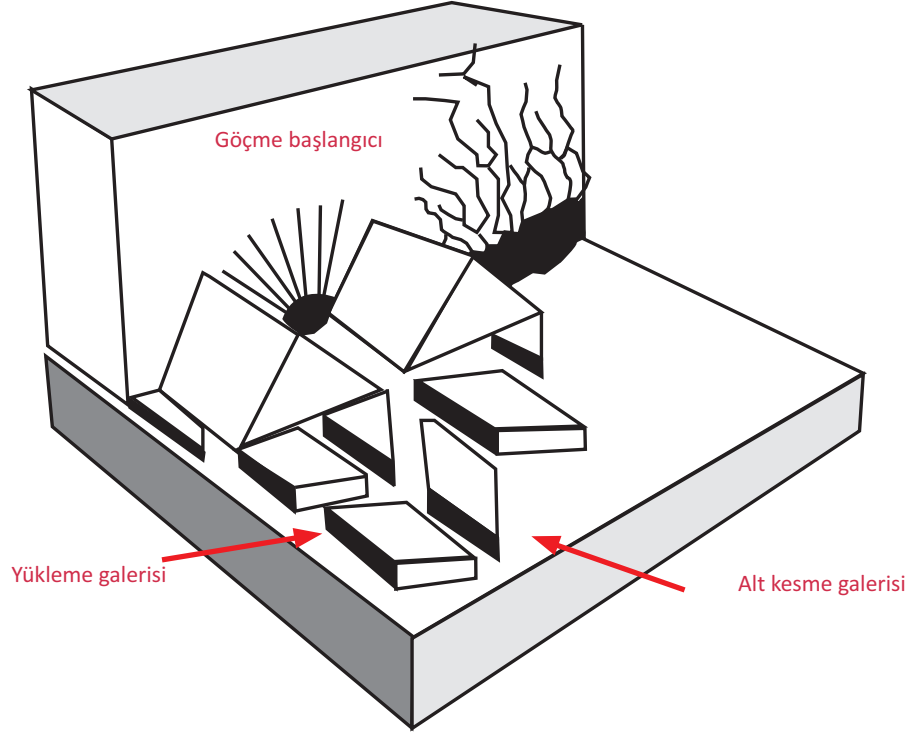
Şekil 4.8: Blok göçertme
