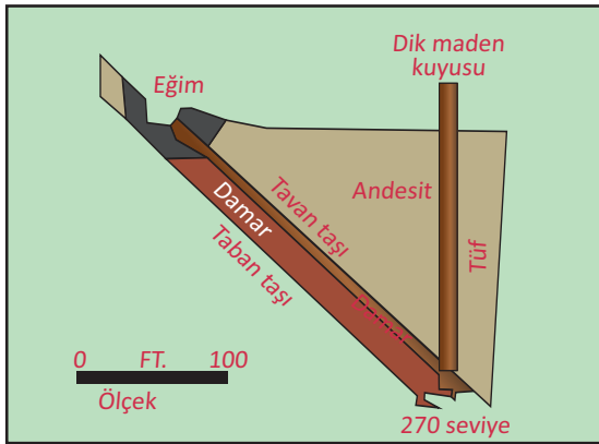
Şekil 6.2: Yatak kuyu
