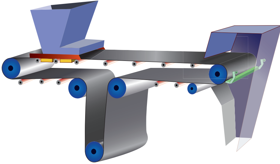
Şekil 5.5: Bantlı konveyör
