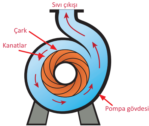
Şekil 5.3: Santrifüj pompa
