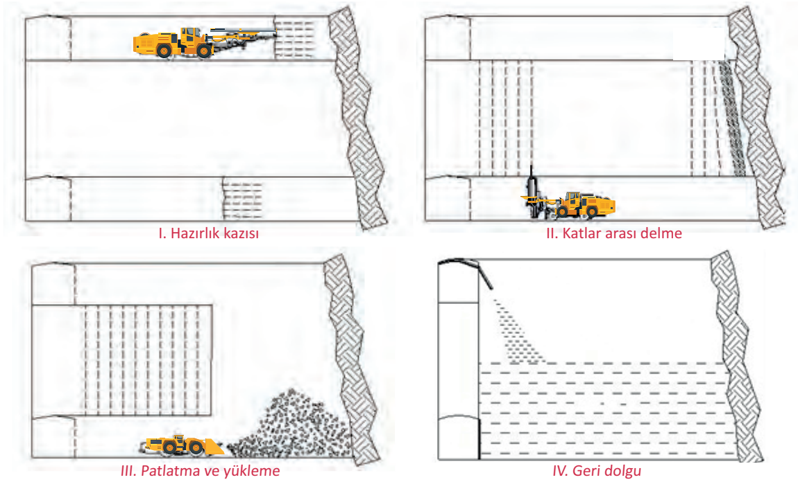
Şekil 4.6: Ara katlı kazı ilerleme aşaması
