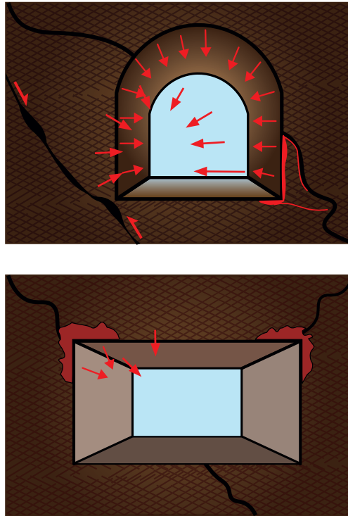
Şekil 7.1: Galerinin üzerine gelen baskı
