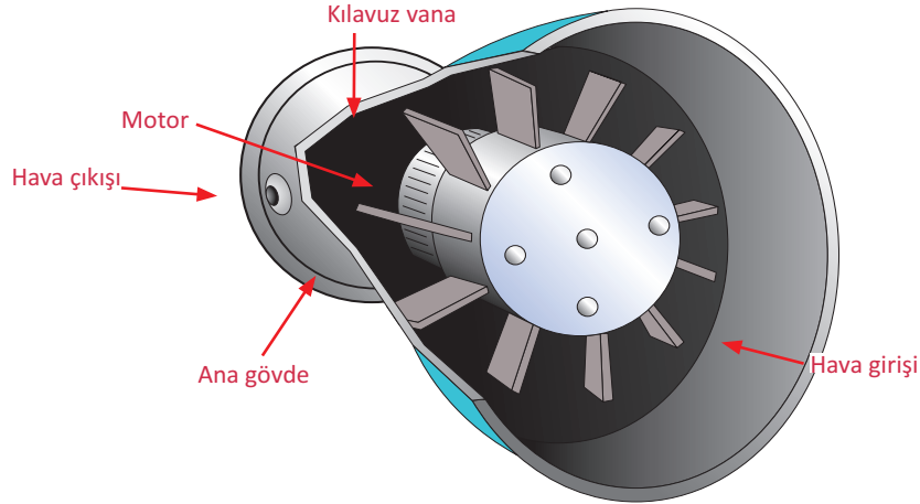
Şekil 3.3: Aksiyel ventilatörünün kesiti ve yandan görünüşü
