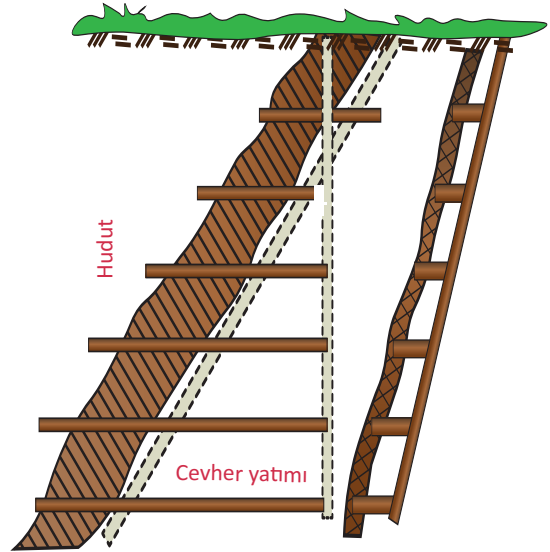
Şekil 1.6: Meyilli kuyu
