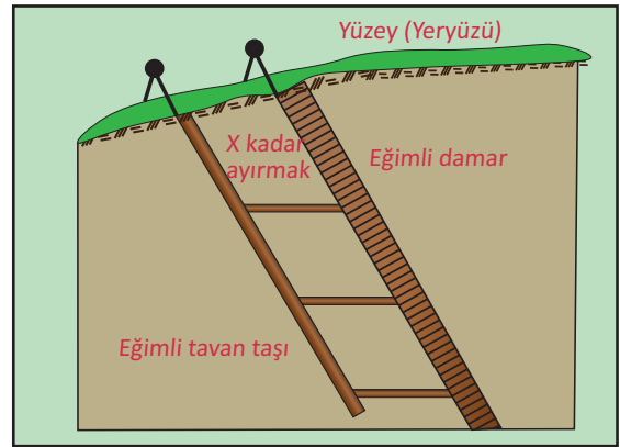
Şekil 6.3: Meyilli kuyu
