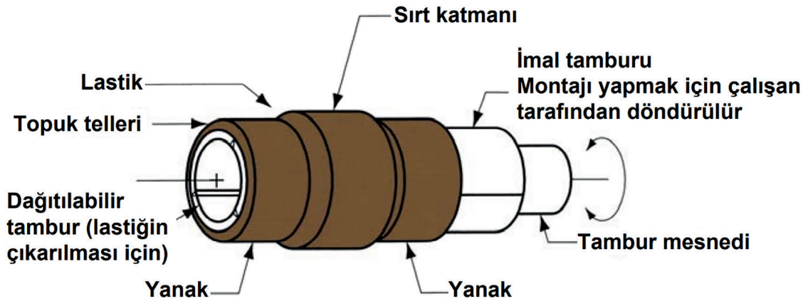
Şekil 3.1: Tambur çizimi
