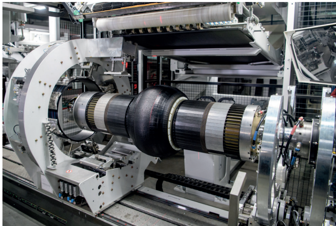
Görsel 3.1: Tamburlama makinesi
