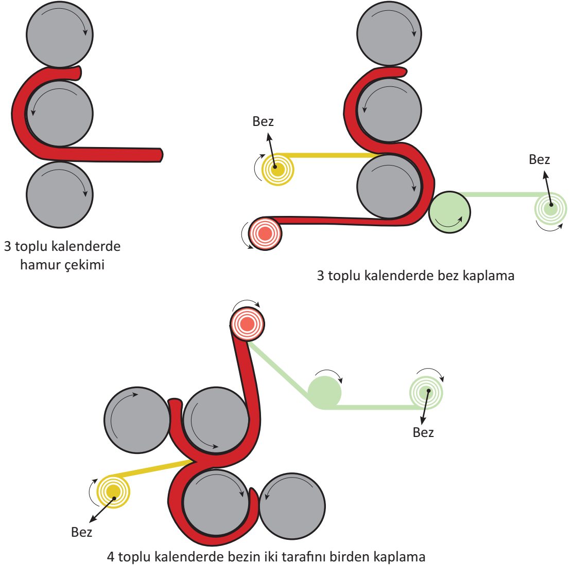
Şekil 2.7: Kalenderleme uygulamaları
