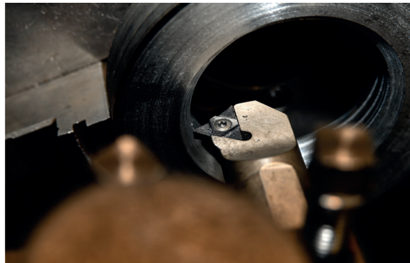
Görsel 5.2: Tıraşlama makinesi uçları
