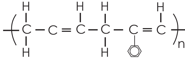
Şekil 1.8: Stiren bütadien
