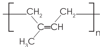
Şekil 1.3: cis -1,4- poliizopren
