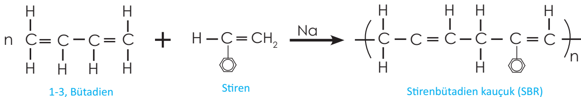
Şekil 1.9: Stiren bütadien kauçuğunun eldesi tepkimesi
