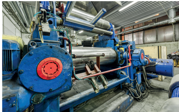
Görsel 1.16: Açık mikser
