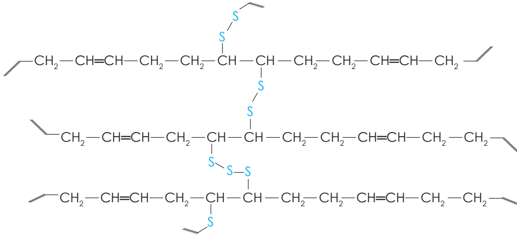
Şekil 1.4: Çapraz bağlı polimer zinciri
