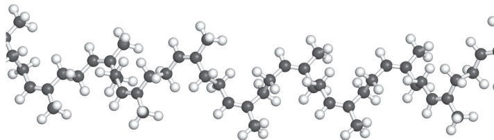
Şekil 1.6: Poliizopren
