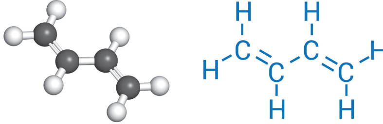
Şekil 1.5: 1-3 Bütadien yapısı
