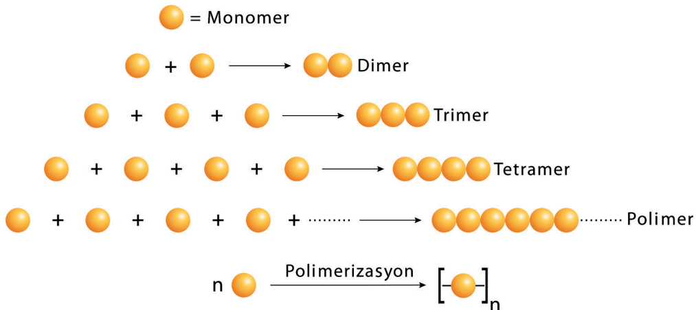
Şekil 1.1: Polimer oluşumu
