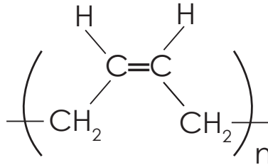
Şekil 1.10: Polibütadien
