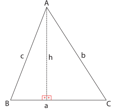
Şekil 2.7: Üçgenin alanı
