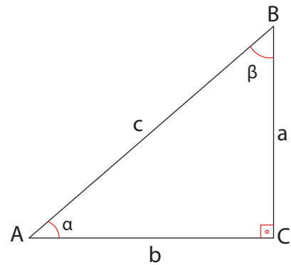
Şekil 1.7: Dik üçgen
