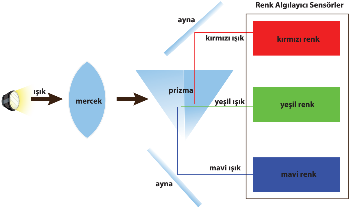
Şekil 1.2: Kamerada RGB renk sinyali
