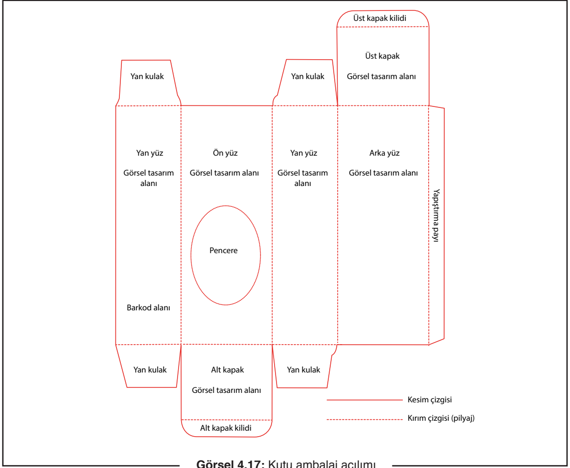
Görsel 4.17: Kutu ambalaj açılımı
