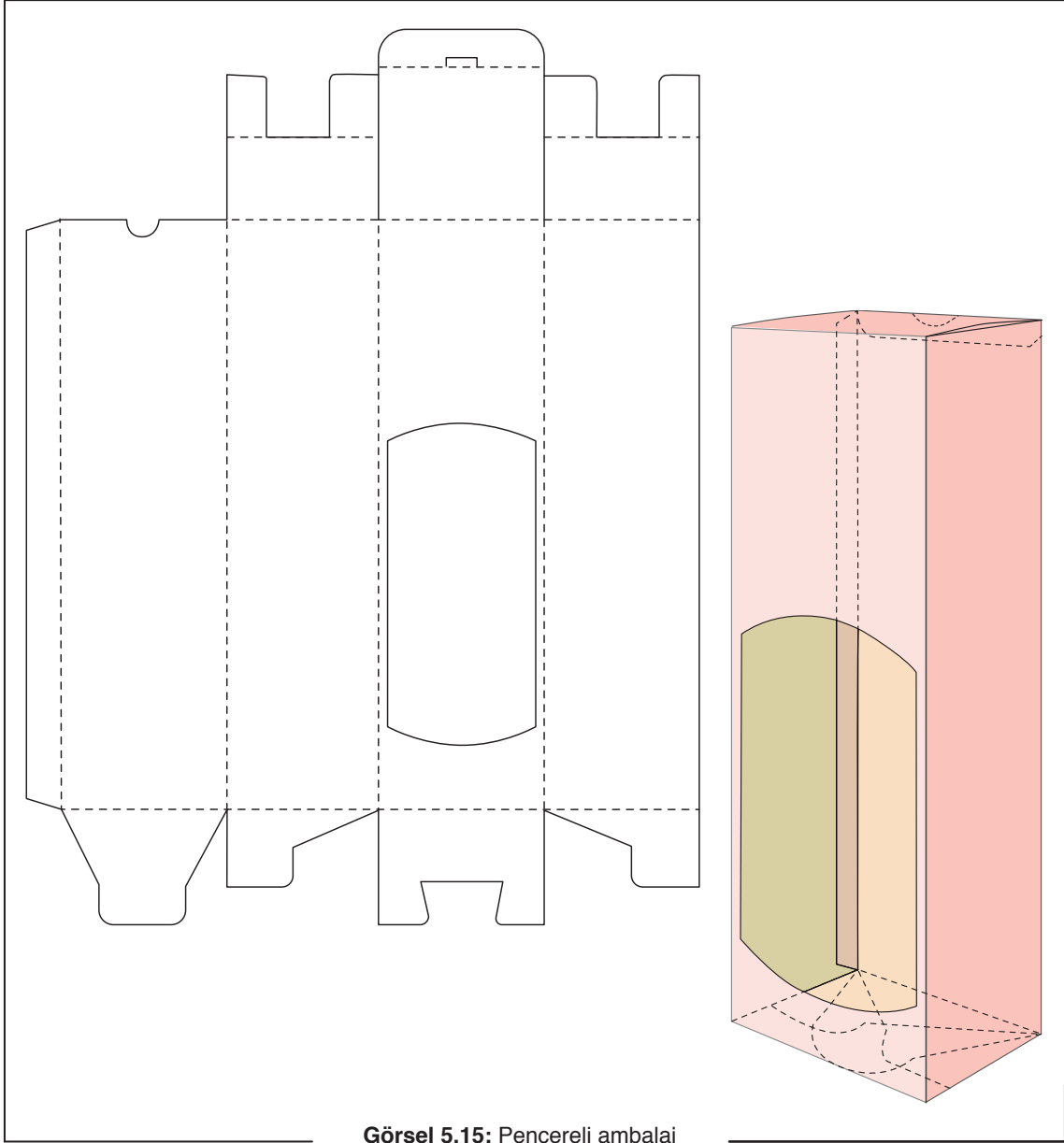
Görsel 5.15: Pencere ambalaj
