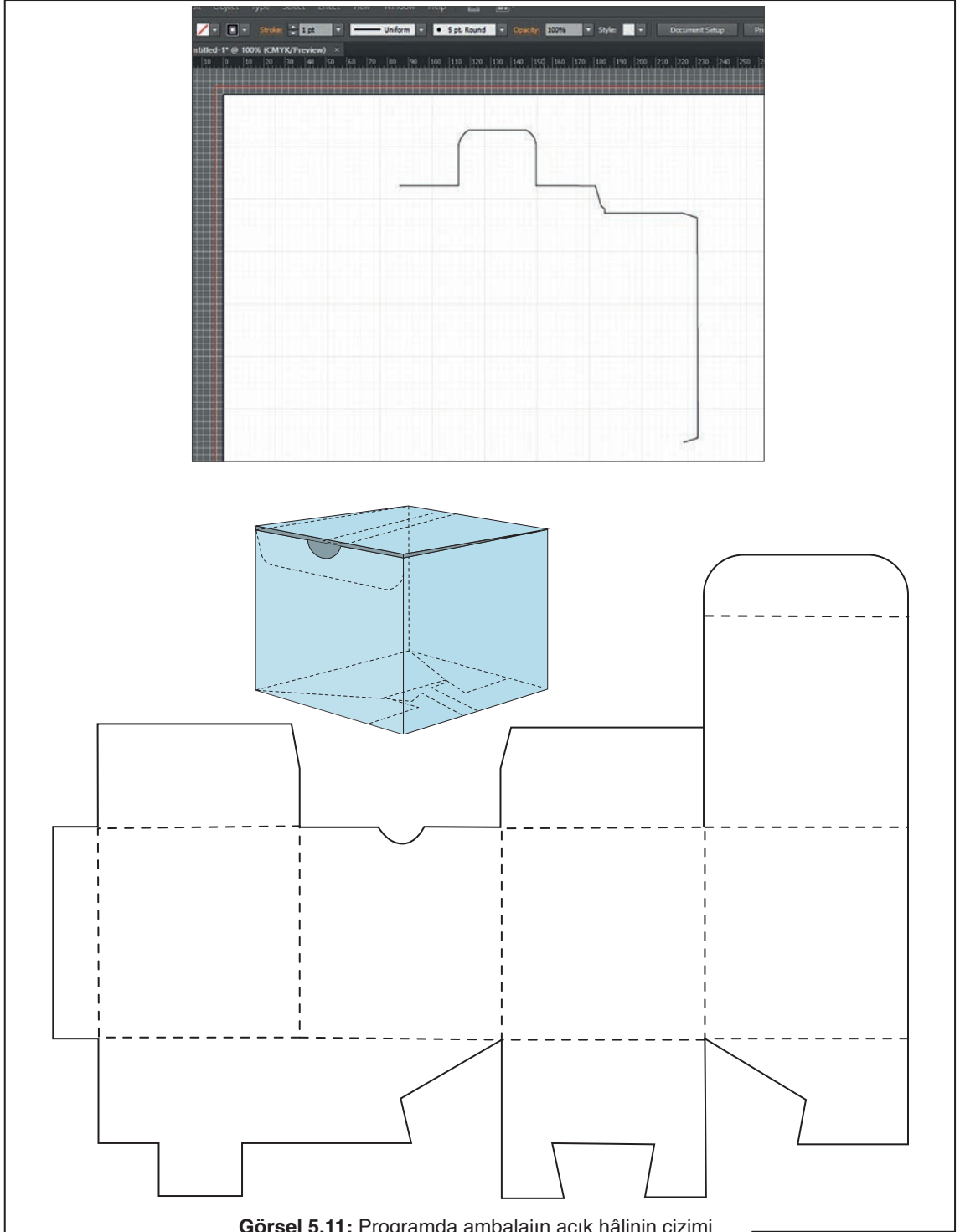
Görsel 5.11: Programda ambalajın açık hâlinin çizimi
