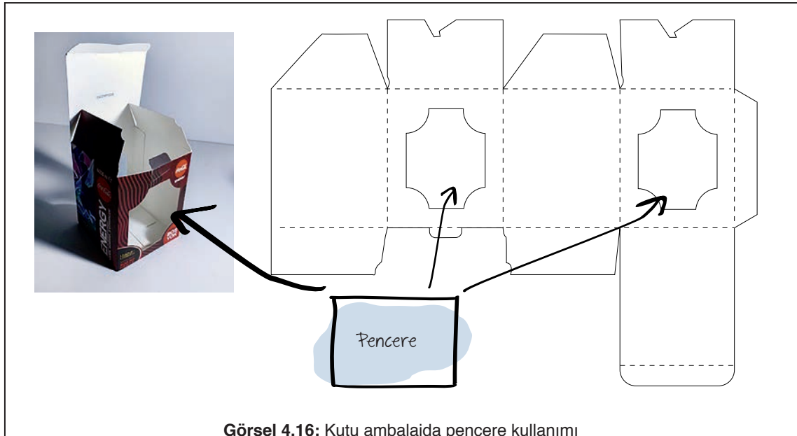
Görsel 4.16: Kutu ambalajda pencere kullanımı
