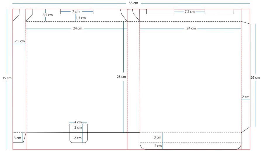
Görsel 4.22: Kutu ambalaj açılımının çizimi
