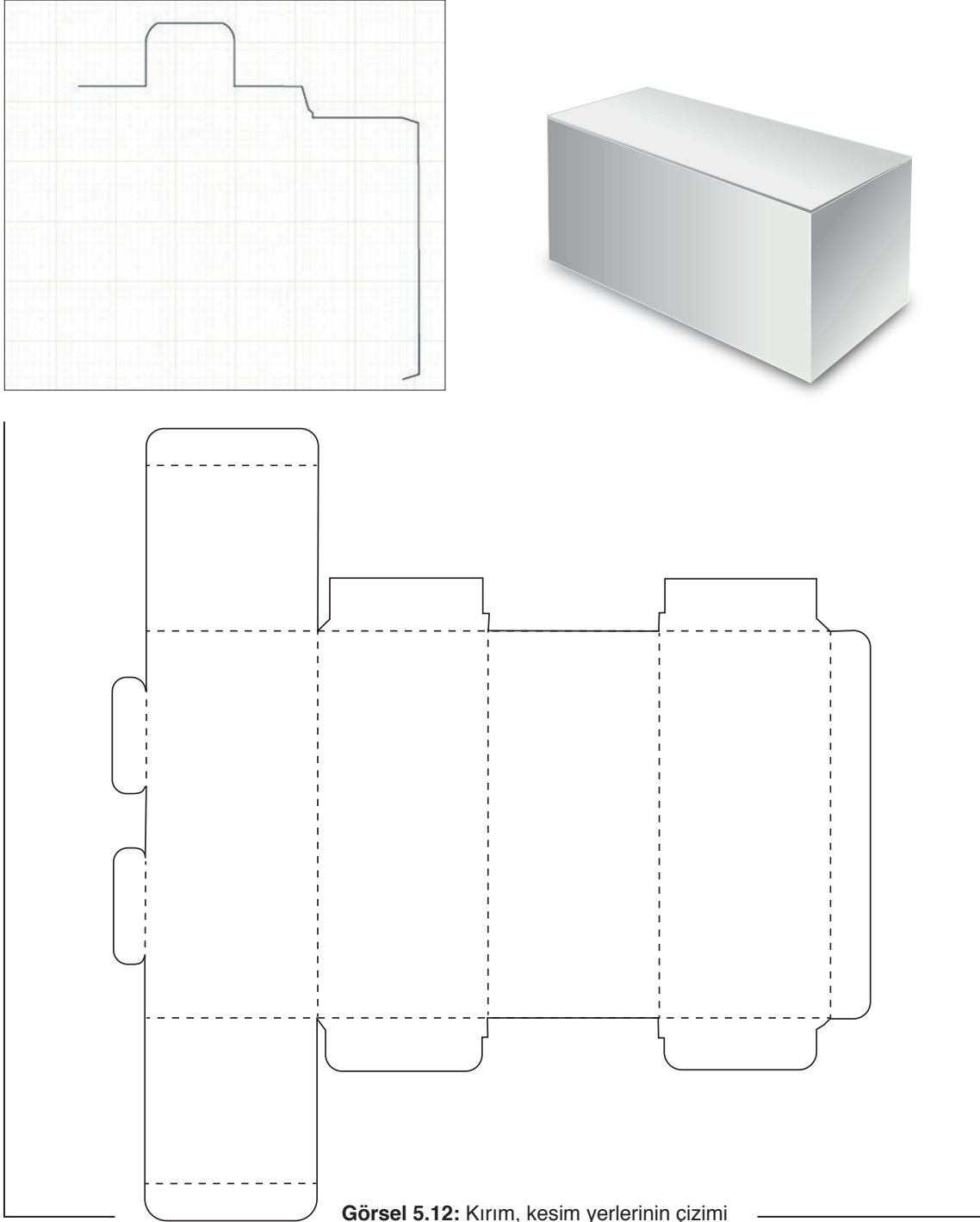
Görsel 5.12: Kırım, kesim yerlerinin çizimi
