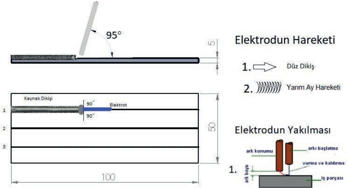
Şekil 2.3: Sağ kaynak
