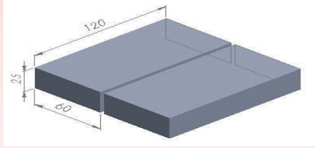
Şekil 1.4: Gemi borda sacı
