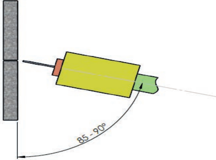
Şekil 3.8: Yan küt ek kaynağı torç açısı
