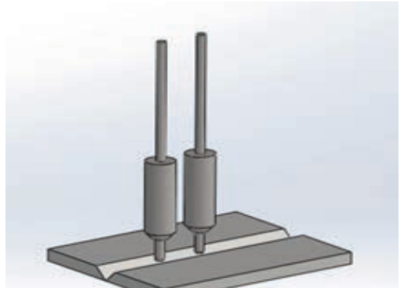
b) Tandem (tandem) tozaltı ark kaynak yöntemi
