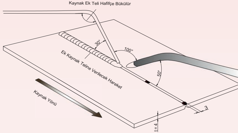
Şekil 4.9: Sac levha
