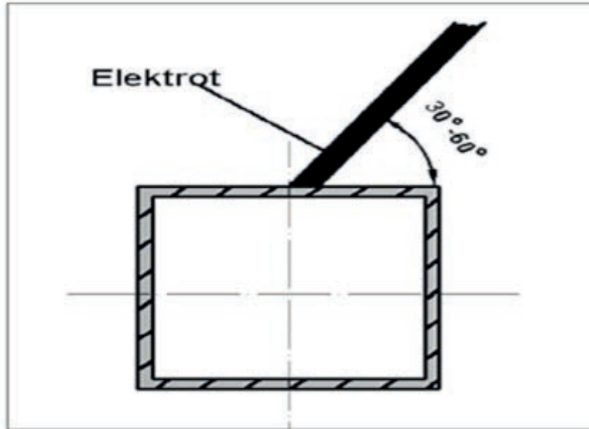
Şekil 2.17: Profil kaynağında elektrot açısı
