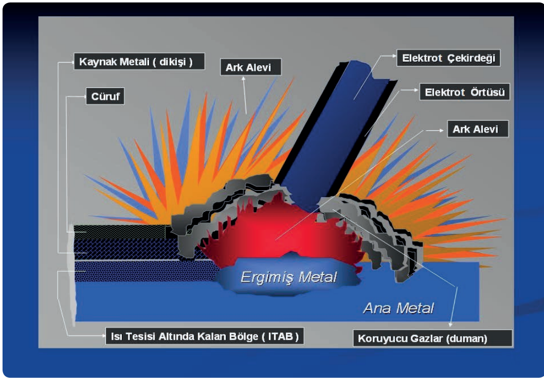
Şekil 2.1: Ergiyen ana metal ve elektrot
