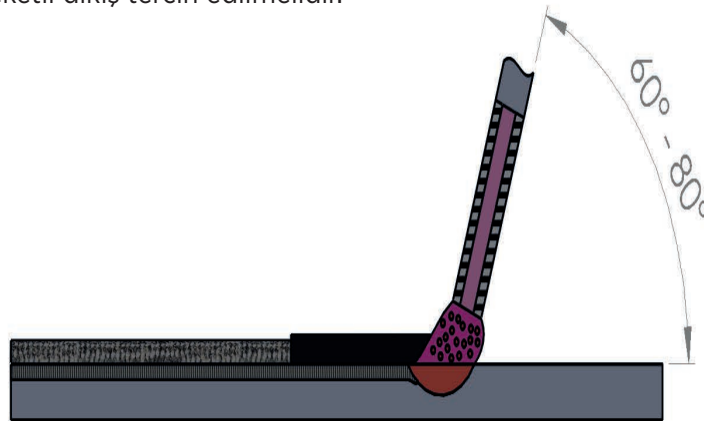
Şekil 2.2: Yatay kaynak elektrot açısı
