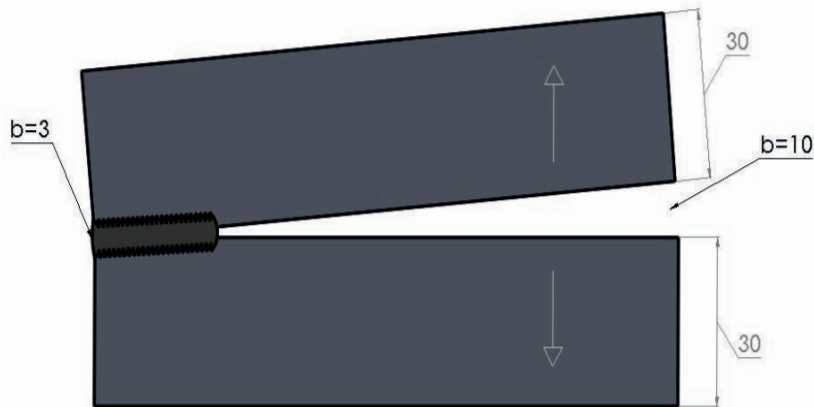
Şekil 2.4: Puntalama yapılmamış iş parçası
