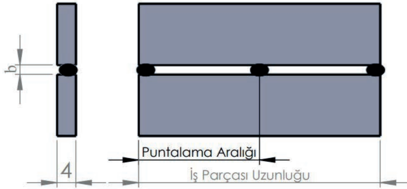
Şekil 2.5: Puntalama işlemi
