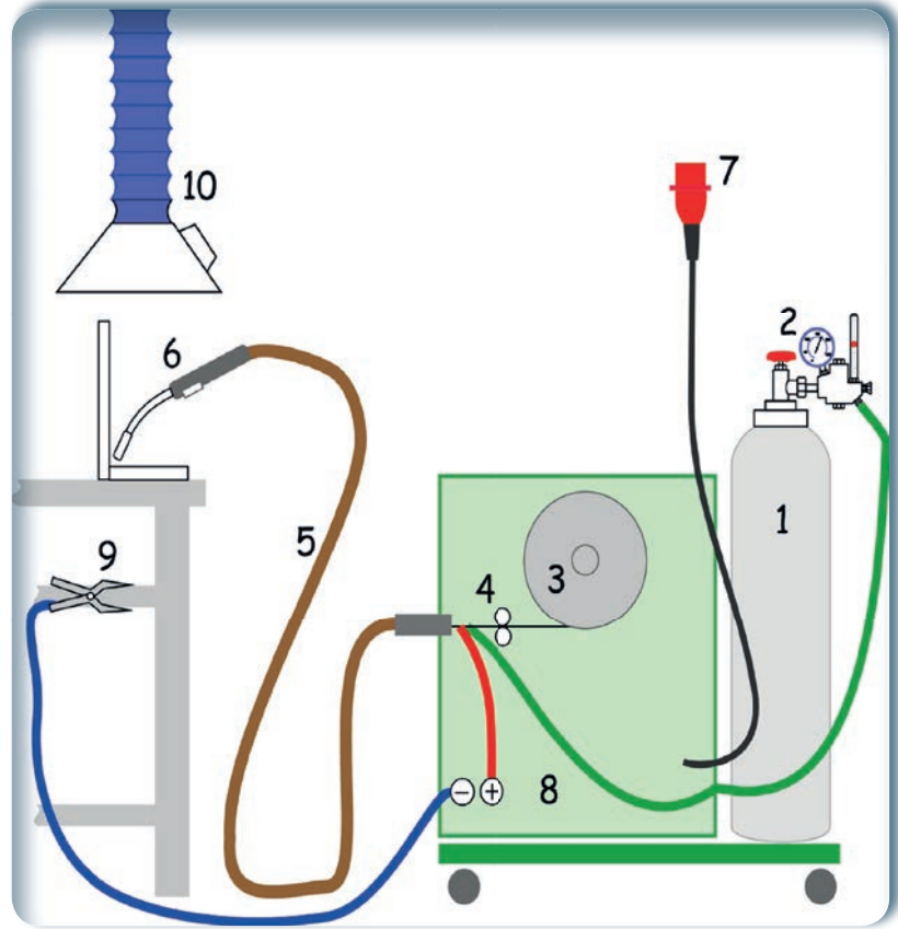
Şekil 1.1: MIG-MAG kaynak ünitesi
