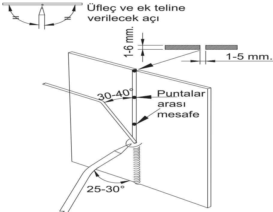
Şekil 4.5: Dik kaynak pozisyonu ve kaynak açıları
