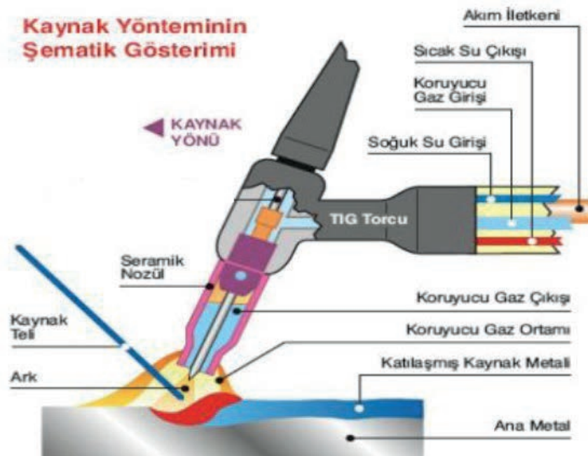
Şekil 6.1: TIG kaynağının prensip şeması
