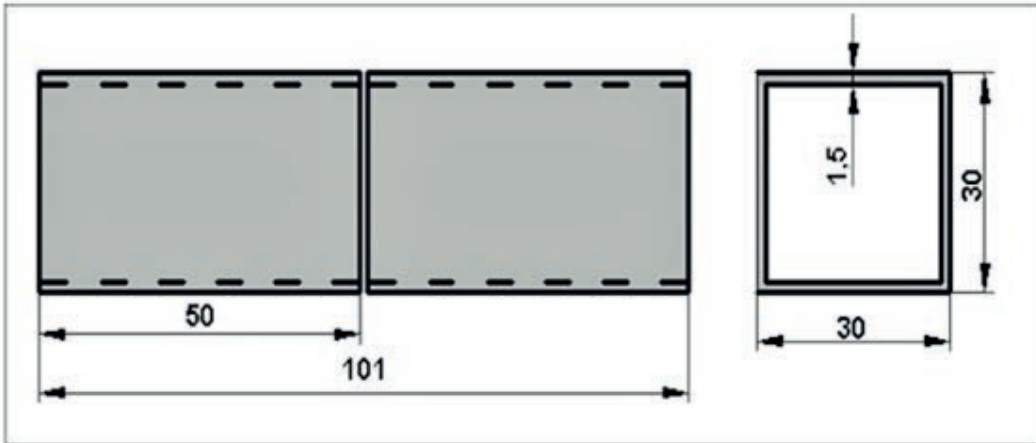
Şekil 2.15: Profil kaynağında mesafe
