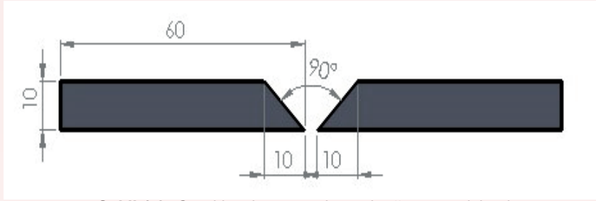
Şekil 1.3: Gemi borda sacına kaynak ağzı açma işlemi
