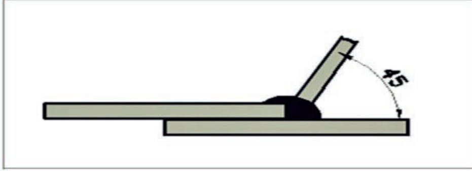
Şekil 2.14: Bindirme kaynağında elektrot açısı
