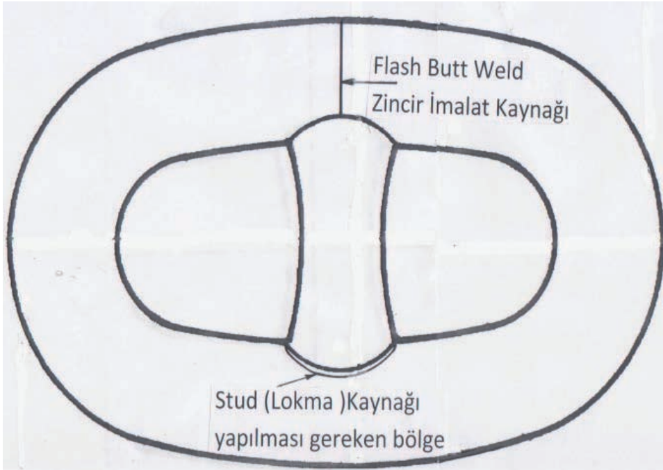
Şekil 2.20: Gemi zincir lokması
