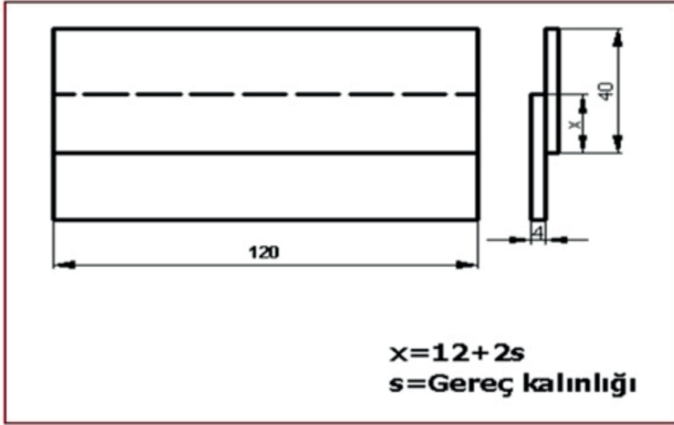
Şekil 2.12: Bindirme kaynağında ölçü
