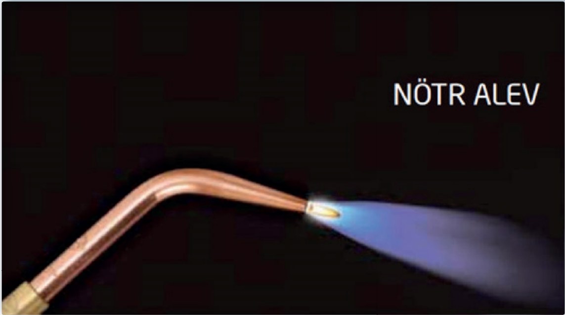
Görsel 4.8: Normal alev
