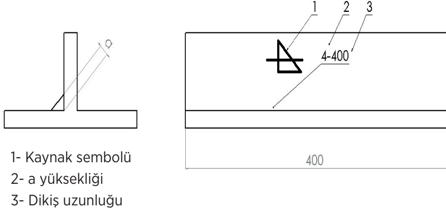
Şekil 3.14: Kaynak sembolleri 2
