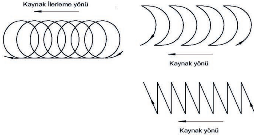
Şekil 3.11: Boru küt ek kaynağı torç hareketi
