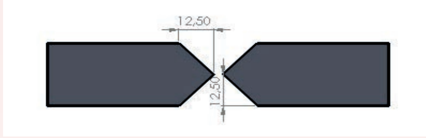
Şekil 1.5: Gemi borda sacına X kaynak ağzı açma
