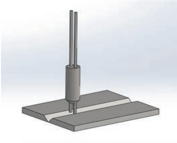
a) Paralel iki elektrotlu tozaltı ark kaynak yöntemi
