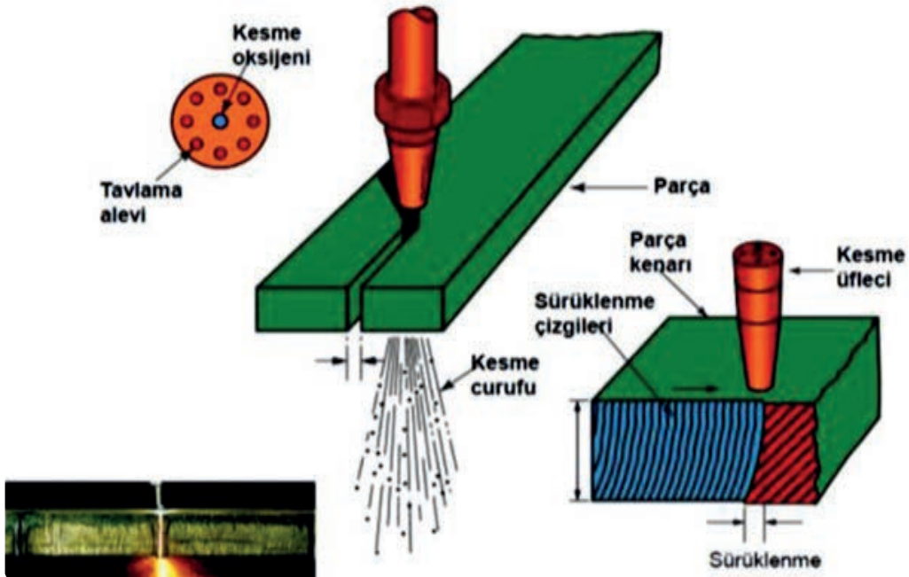
Şekil 7.1: Oksi-gaz ile kesme 1
