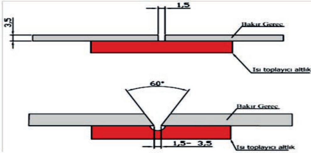
Şekil 2.18: Bakır kaynağında aç, mesafe ve altlık
