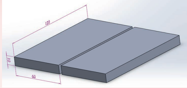
Şekil 1.2: Gemi borda sacı
