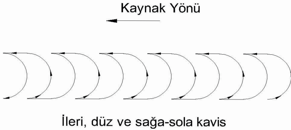
Şekil 3.13: Dış köşe kaynağı torç hareketi
