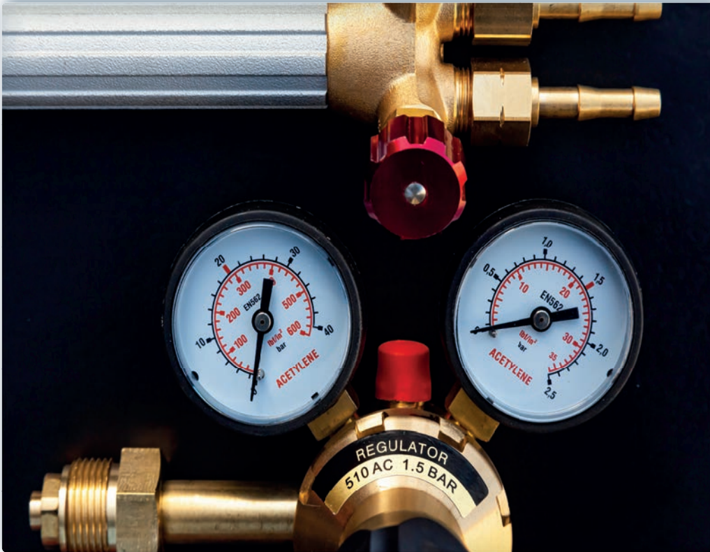
Görsel 4.5: Regülatör ve manometreler
