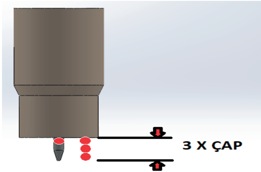
Şekil 6.3: Tungsten elektrodun nozulden çıkış miktarı
