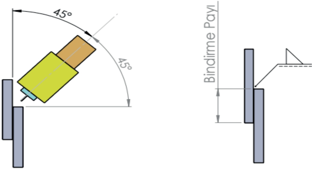
Şekil 3.10: Bindirme kaynağında torç açısı
