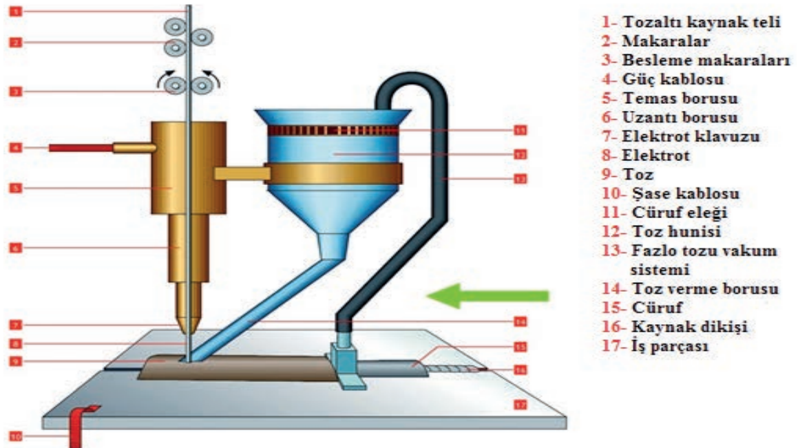
Şekil 5.2: Tozaltı kaynak şeması
