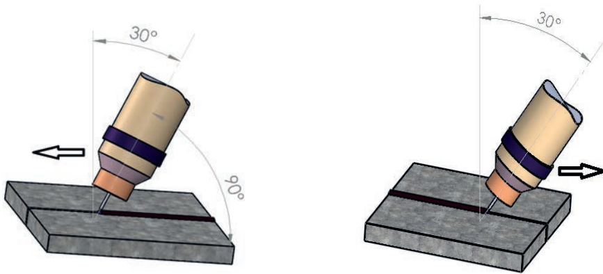
Şekil 3.2: Küt kaynağı torç açısı
