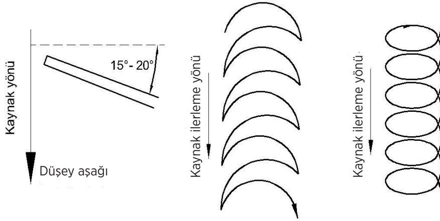
Şekil 3.5: Yukarıdan aşağıya kaynakta torç hareketi ve açısı
