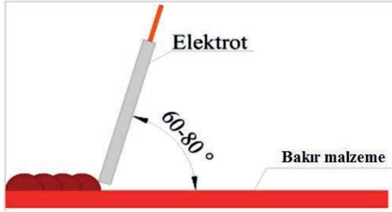
Şekil 2.19: Pirinç kaynağında elektrot açısı
