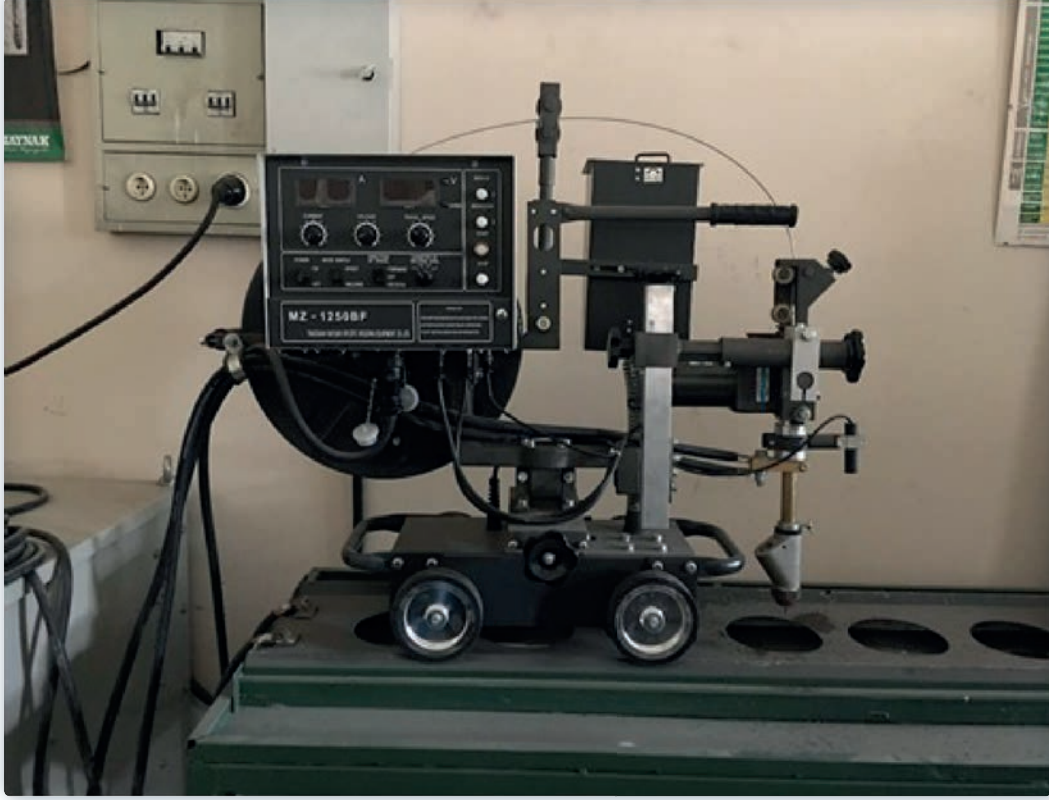
Görsel 5.1: Tozaltı kaynak makinesi
