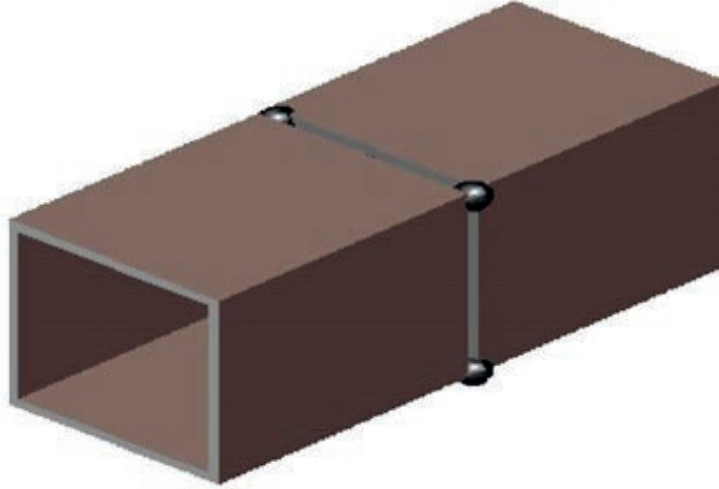
Şekil 2.16: Profil kaynağında puntalama
