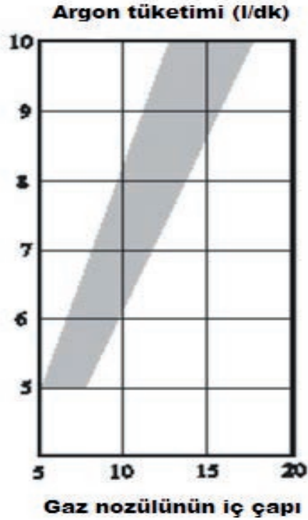
Şekil 6.4: Koruma gazının miktarı
