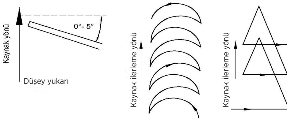
Şekil 3.6: Aşağıdan yukarıya kaynak torç hareketi ve açısı
