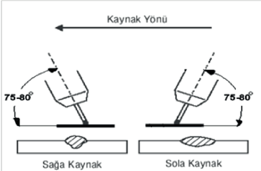
Şekil 3.7: Duvar kaynağında torç açısı
