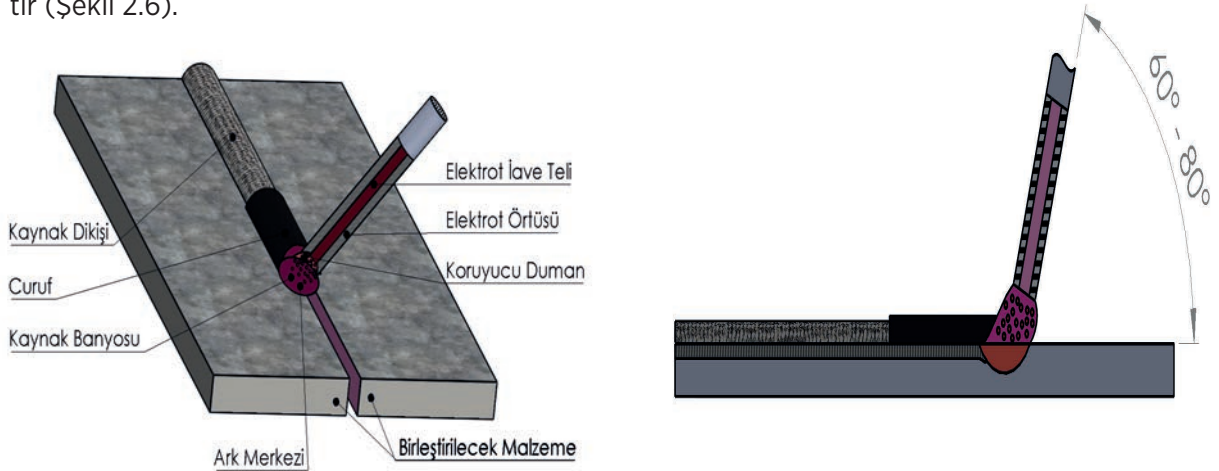
Şekil 2.6: Küt ek kaynağında elektrot açısı
