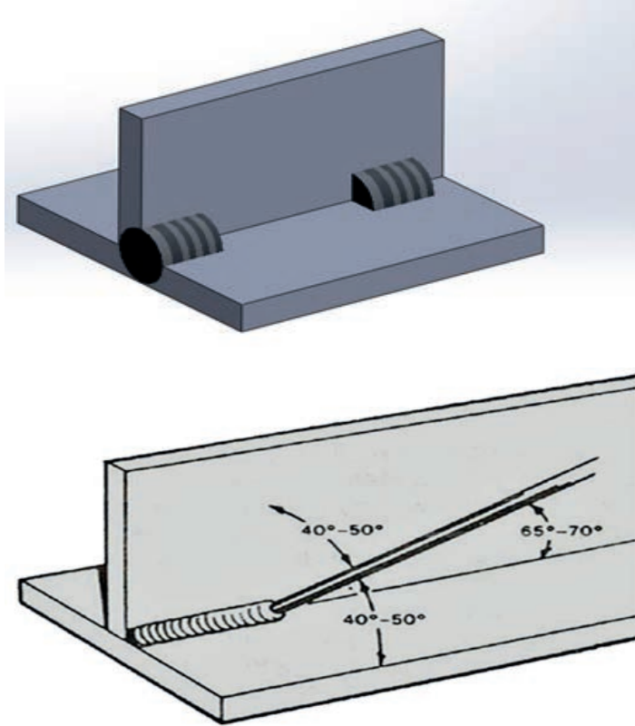
Şekil 2.10: T kaynağı
