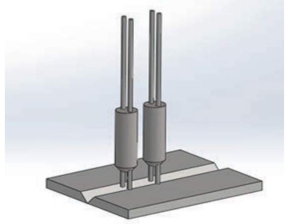
b) Tandem iki elektrotlu tozaltı ark kaynak yöntemi
