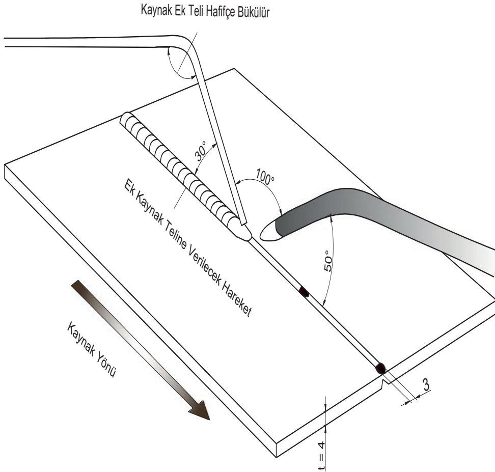
Şekil 4.4: Yatayda küt ek kaynağı ve kaynak açıları
