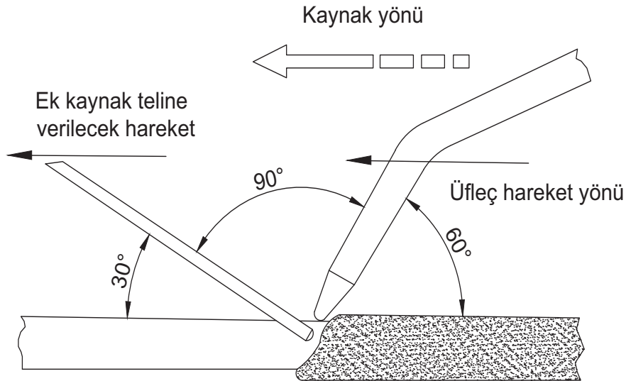
Şekil 4.3: Sol kaynak
