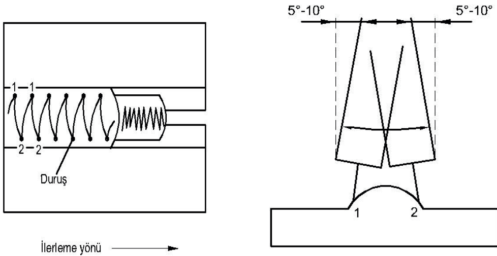
Şekil 3.4: Çok pasolu küt kaynağı torç hareketi ve açısı
