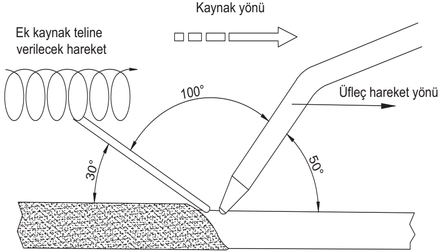
Şekil 4.2: Sağ kaynak
