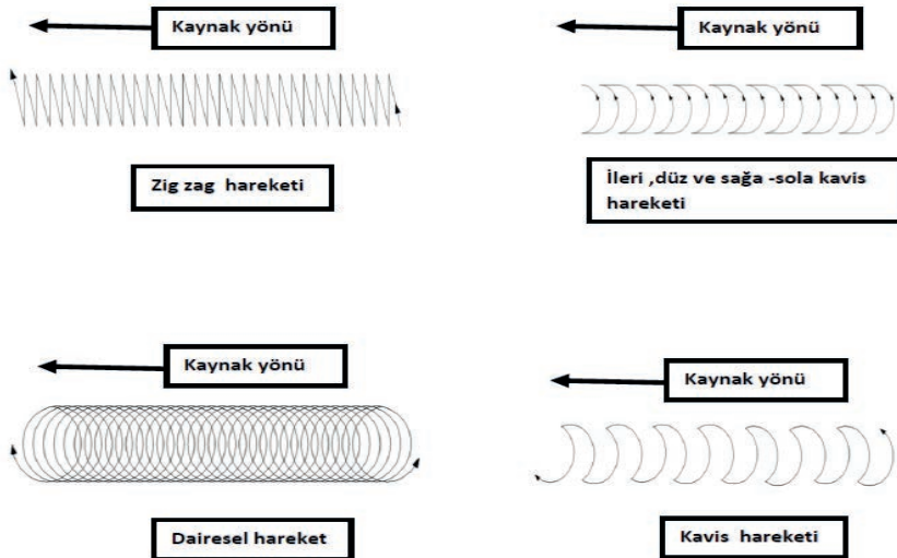
Şekil 4.1: Üfleç hareketleri
