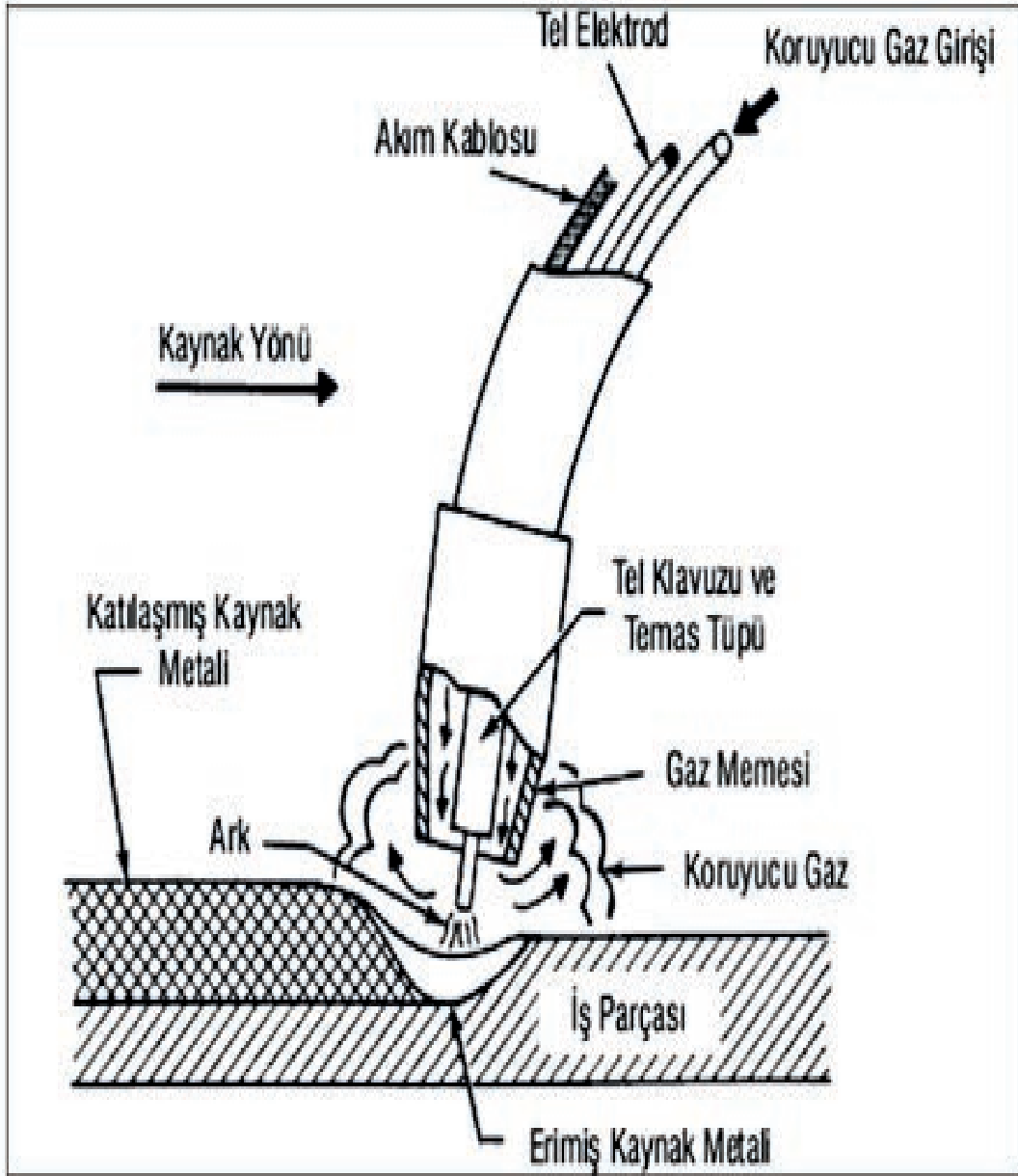
Şekil 3.1: Gazaltı kaynak uygulaması çalışma prensibi
