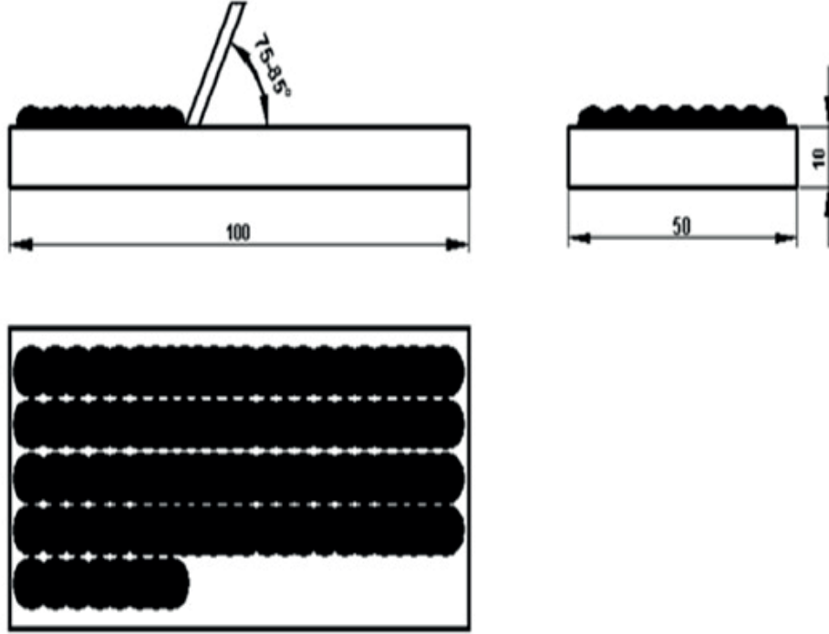
Şekil 2.11: Dolgu kaynağı
