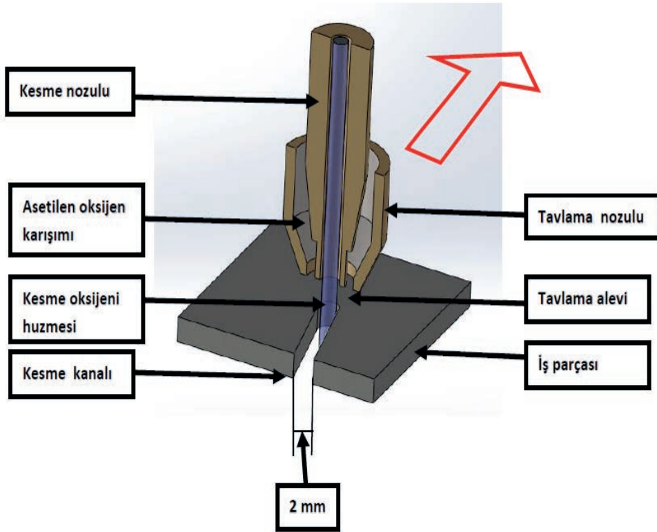
Şekil 7.2: Oksi-gaz ile kesme 2
