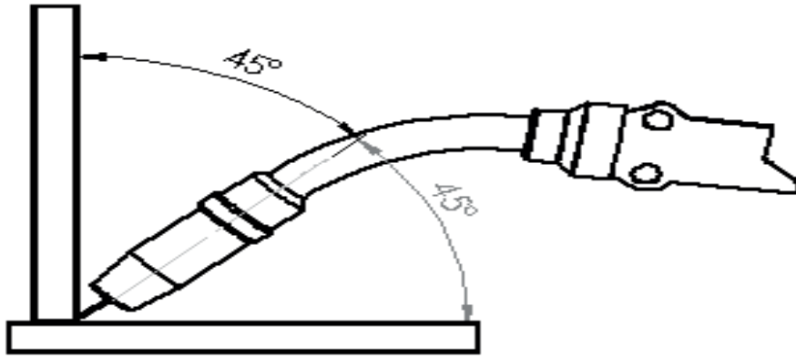
Şekil 3.12: İç köşe kaynağı torç açısı
