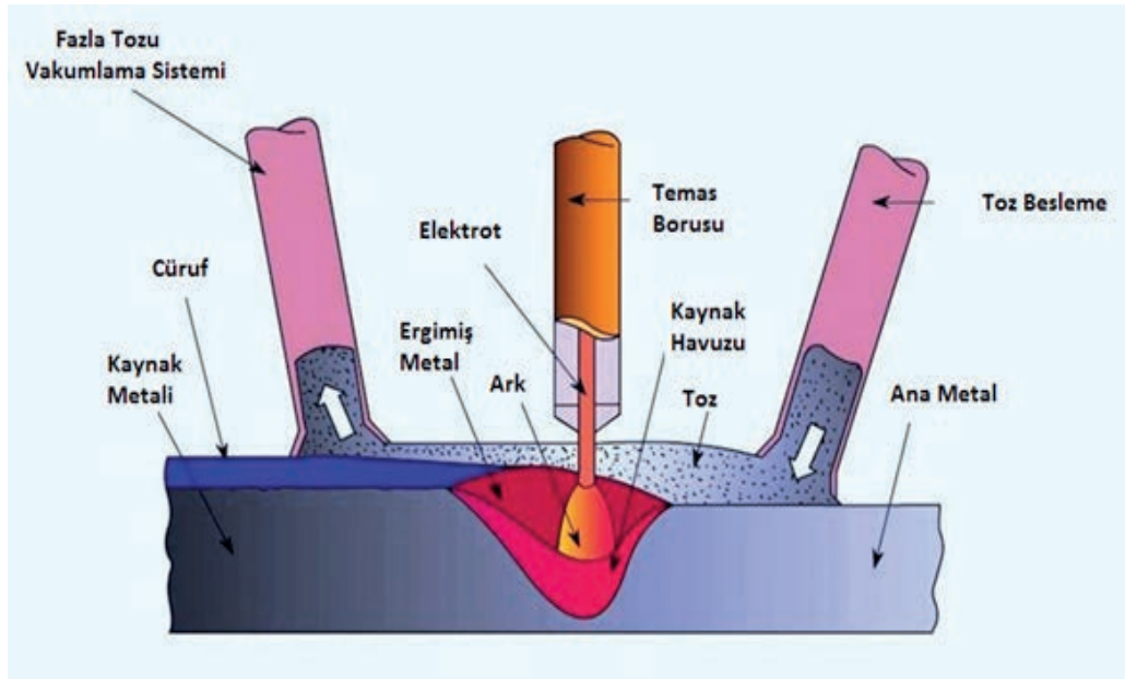
Şekil 5.1: Tozaltı kaynak bölgesi şeması
