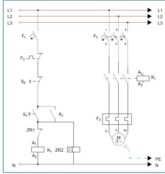
GörSEL 4.9: Zaman ayarlı çalışma kumanda ve güç devresi
