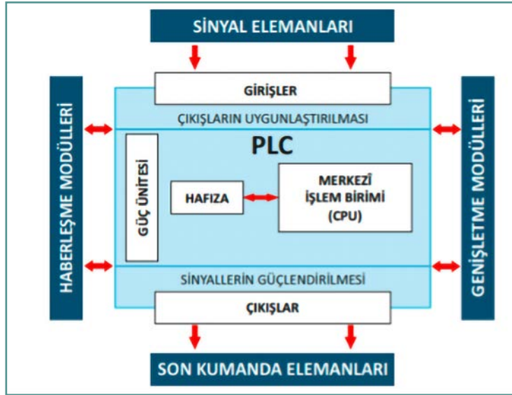
Görsel 4.13: PLC'nin yapısı
