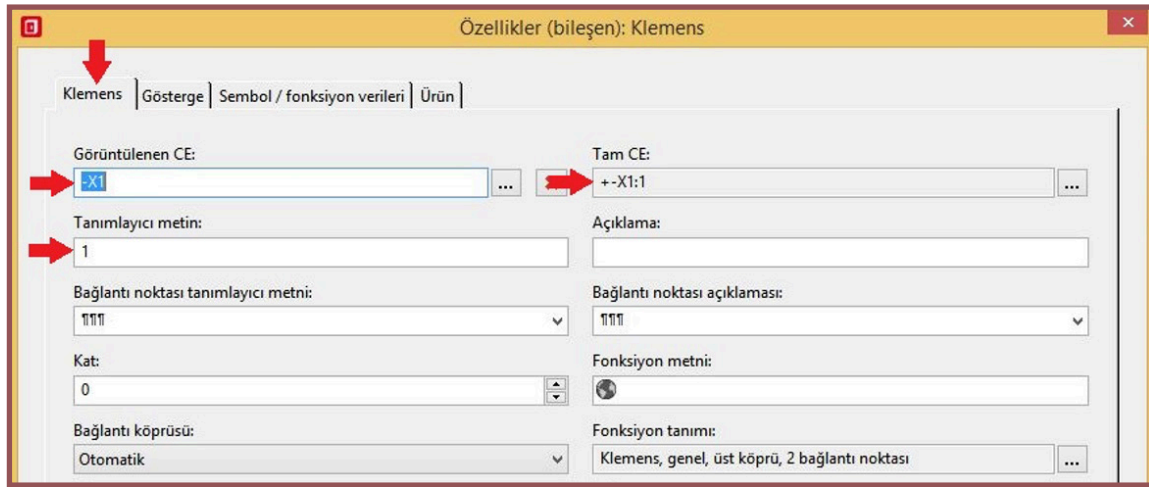
Görsel 3.38: Klemens özellikleri penceresi
