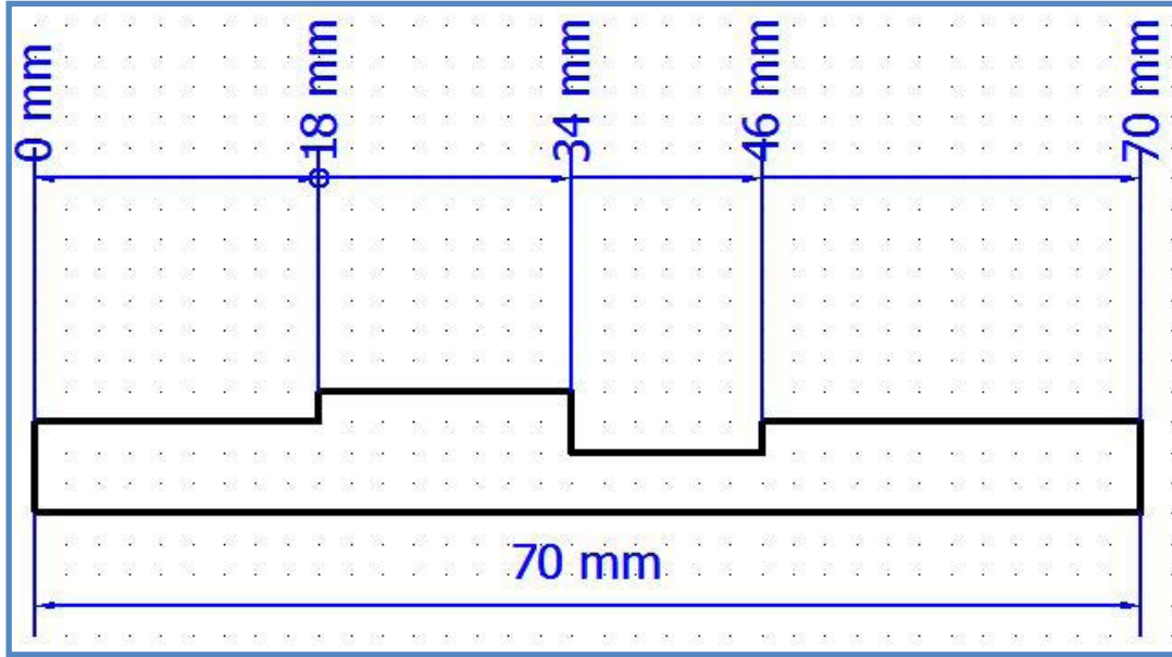
Görsel 2.54: Artan ölçülendirmenin gösterimi
