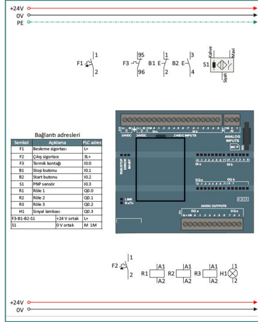
Görsel 4.16: Transistör Çıkışlı PLC kumanda ve güç devresi çizimi
