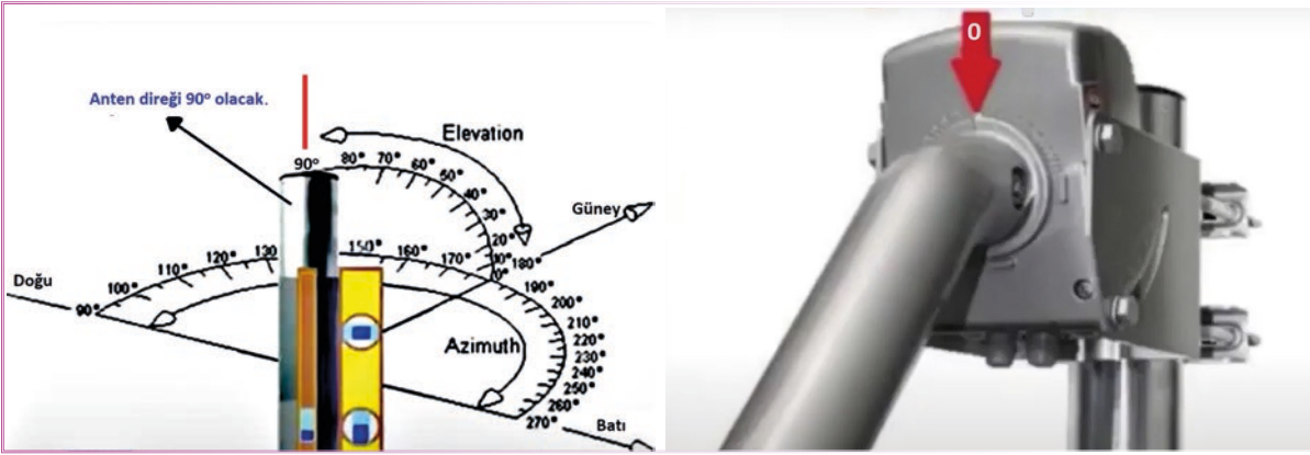
Görsel 2.46: Açı değerleri ve diseqc motor
