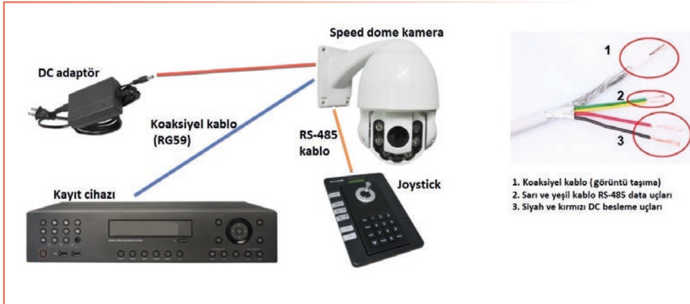
Görsel 3.57: Speed dome kameranın kurulumu
