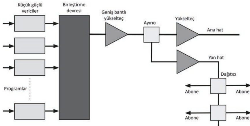
Görsel 1.2: Kablo TV sisteminin blok diyagramı
