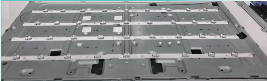
Görsel 1.86: Arka panelin sökülmüş görünümü
