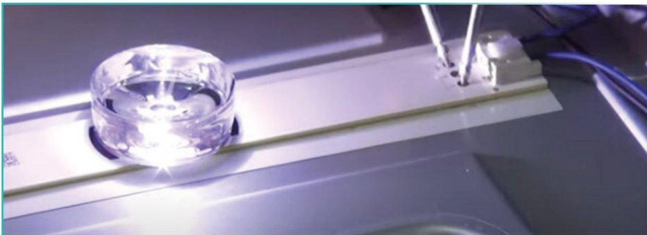
Görsel 1.87: Test cihazıyla LED'lerin kontrol edilmesi ve arızalı LED barların değiştirilmesi
