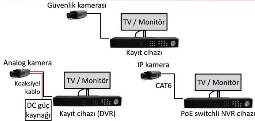
Görsel 3.48: Tek kameralı sistemler
