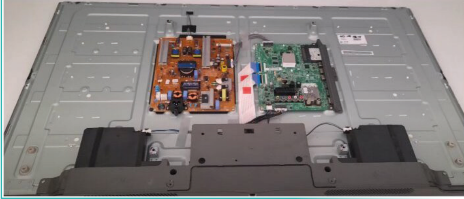
Görsel 1.77: LED TV arka aydınlatma LED'lerinin değiştirilmesi için arka kapak vidalarının sökülmesi
