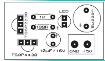
Görsel 1.96: Kızılötesi kumanda test devresinin yerleşim planı
