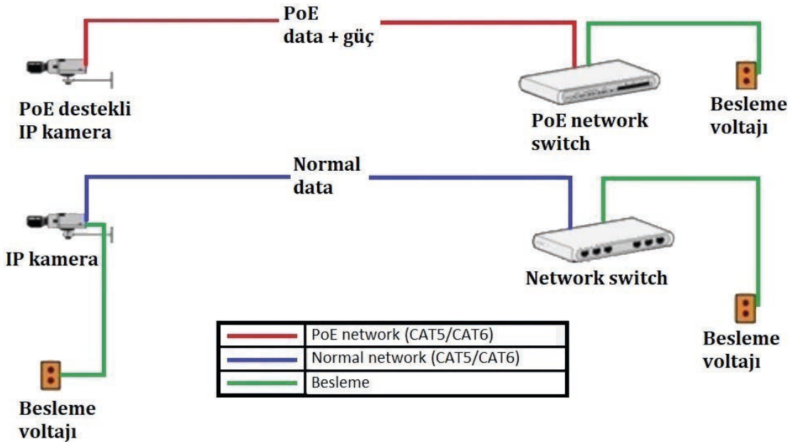
Görsel 3.33: PoE ile normal sistem kurulumu
