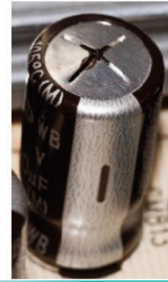
Görsel 1.46: Arızalı kondansatör
