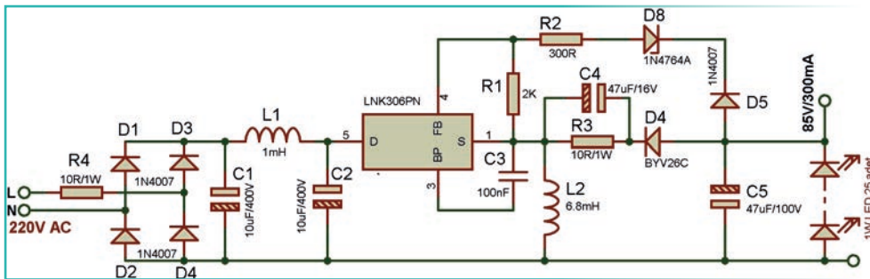
Görsel 1.55: LNK306 entegresi alternatif devre uygulaması
