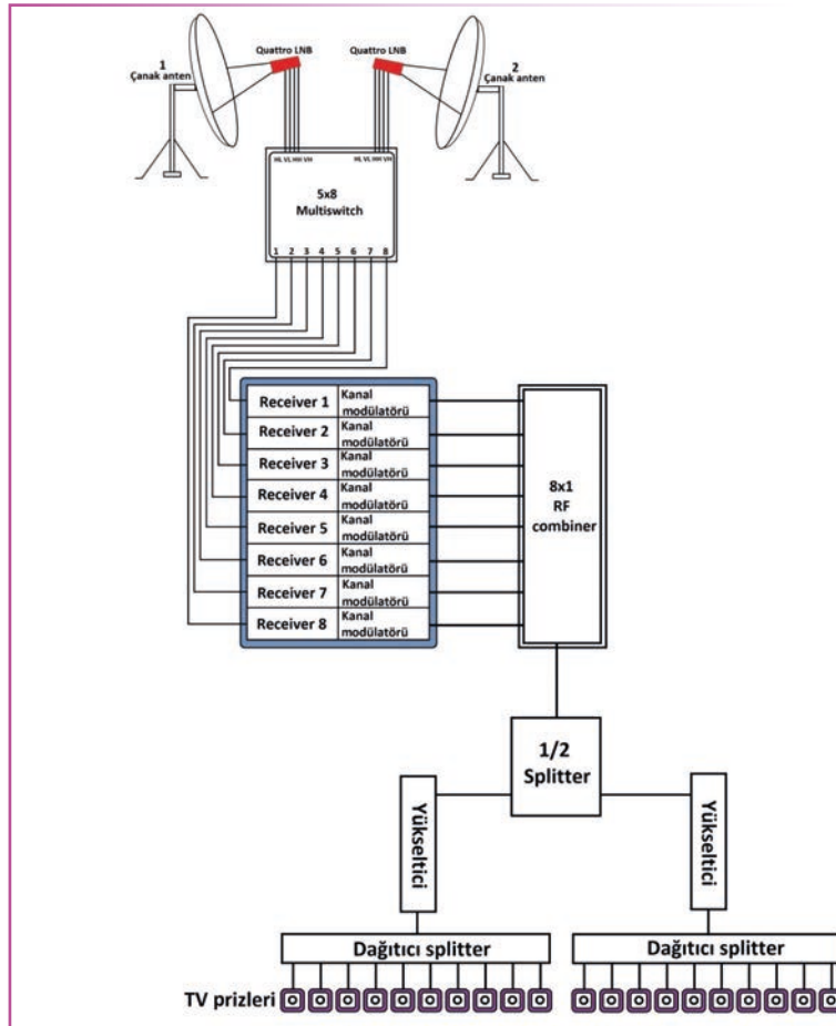
Görsel 2.67: Sekiz kanal yayınına dağıtan head-end uydu anteni sisteminin şeması
