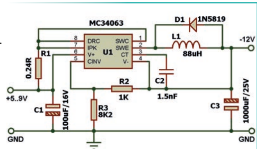
Görsel 1.100: MC34063 entegresiyle yapılmış alternatif uygulama
