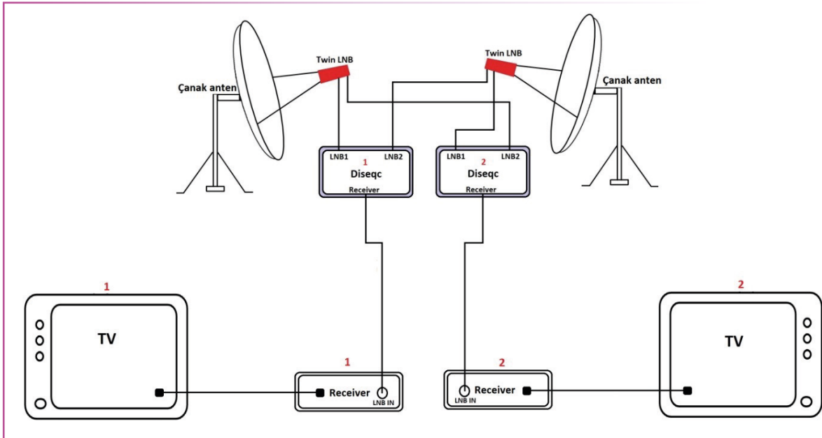
Görşel 2.44: İki çanak antenle iki ayrı aboneye yayın gönderilmesi
