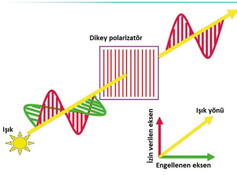
Görsel 1.14: Işığın polarizatörden geçerek tek yönlü olması
