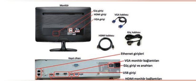
Görsel 3.12: Kayıt cihazı ve monitör bağlantı elemanları
