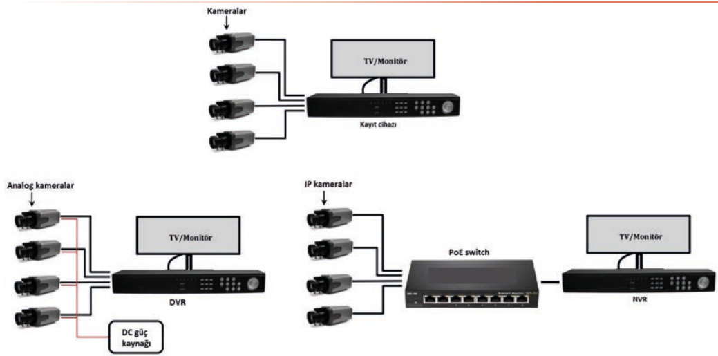
Görsel 3.54: Çok kameralı sistemler
