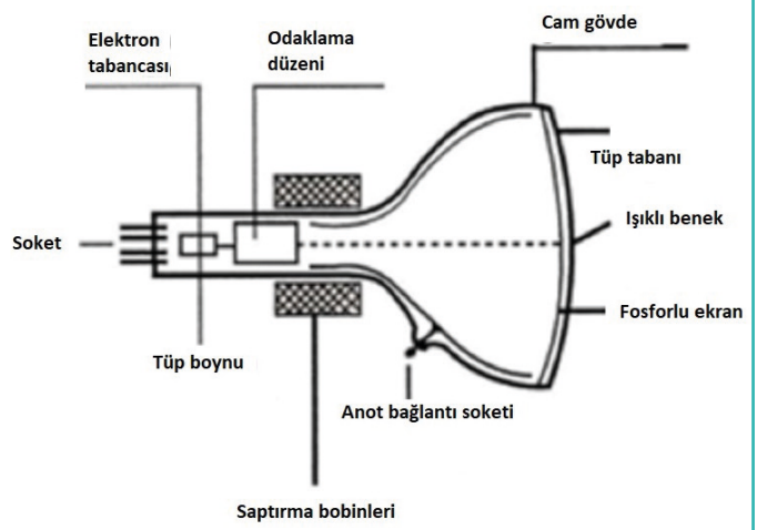
Görsel 1.39: CRT resim tüpü
