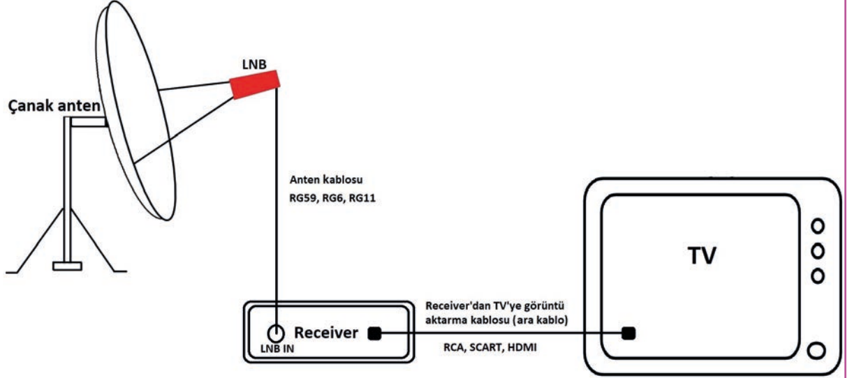
Görsel 2.40: Tek uydu antenli, bir aboneli uydu anteni tesisatının blok şeması
