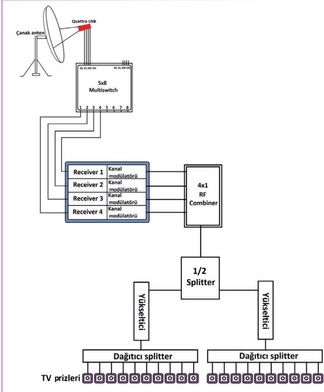
Görsel 2.68: Dört kanal yayını yapan head-end sisteminin şeması
