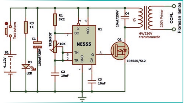
Görsel 1.34: NE555 ile CCFL floresan lamba test devresinin şeması
