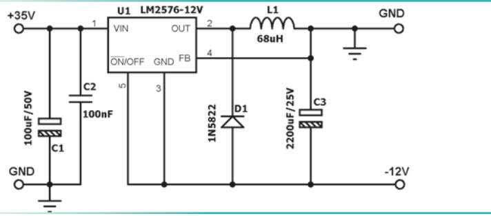
Görsel 1.60: LM2576 entegresiyle alternatif devre uygulaması
