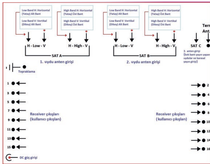
Görsel 2.56: Multiswitch bağlantı noktalarının açıklaması
