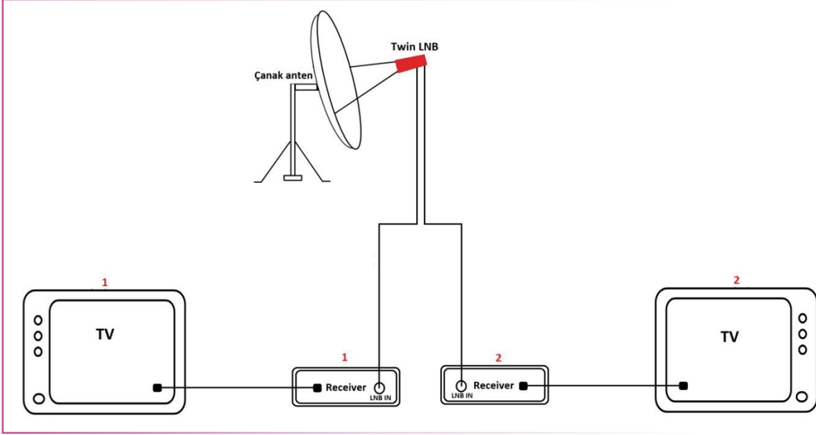
Görşel 2.43: Bir çanak antenle iki aboneye yayın gönderilmesi
