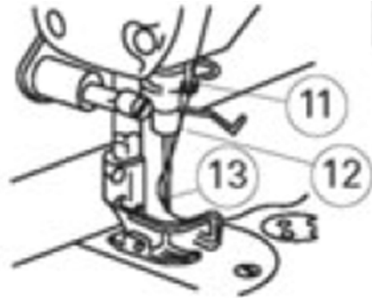
Görsel 3.12: İğne kısmından iplik geçirme
