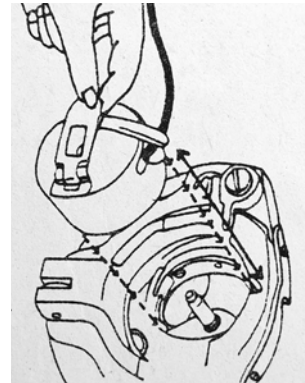
Görsel 3.18: Mekiki mekik yuvasına geçirme
