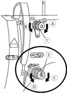
Görsel 3.16: Üst iplik geçirme kısım-2
