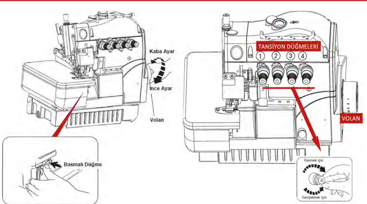
Görsel 4.10: Overlok dikiş sıklık ayar düğmesi
