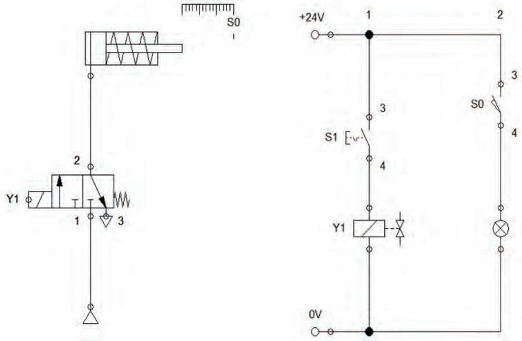
Şekil 3.29: Sınır anahtarı kullanılmış elektropnömatik devre şeması
