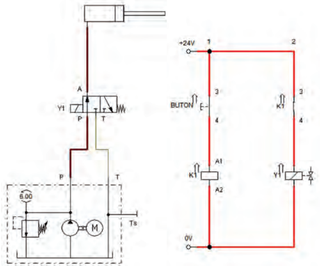
Şekil 1.60: Tek etkili hidrolik silindirin elektrohidrolik devresinin 1. konumu
