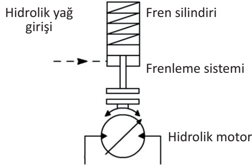
Şekil 2.6: Kreyn vinci frenleme sistemi
