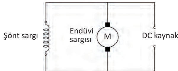
Şekil 6.4: Şönt motor
