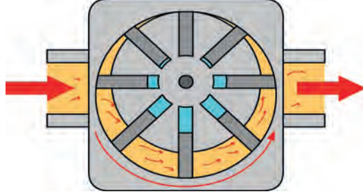
Şekil 1.15: Paletli pompa
