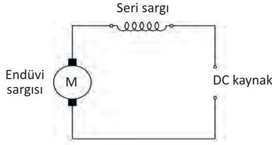
Şekil 6.3: Seri motor
