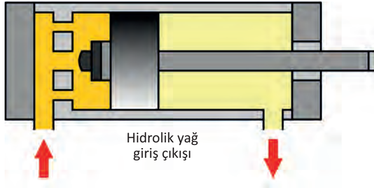
Şekil 1.34: Yastıklı hidrolik silindir
