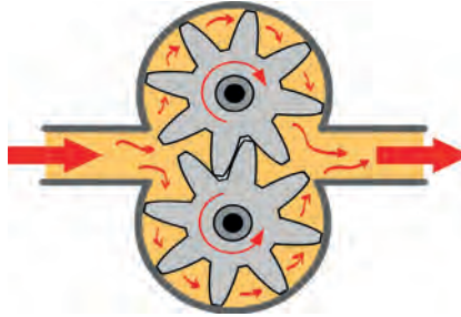
Şekil 1.10: Dış dişli pompa
