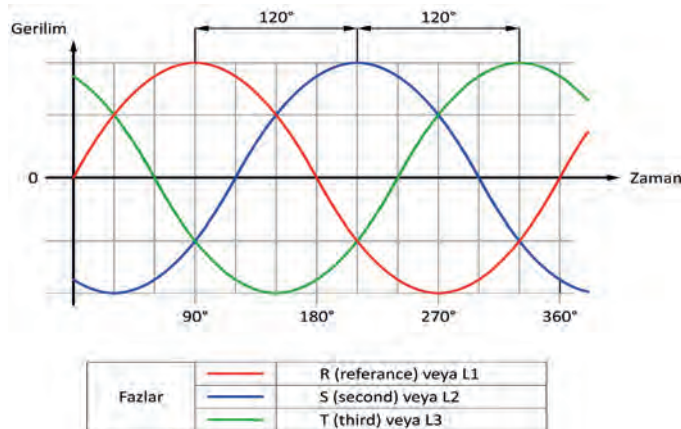
Şekil 5.4: Üç fazlı sistem
