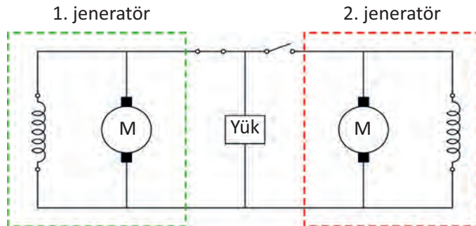
Şekil 6.13: Şönt jeneratörlerin paralel bağlanması
