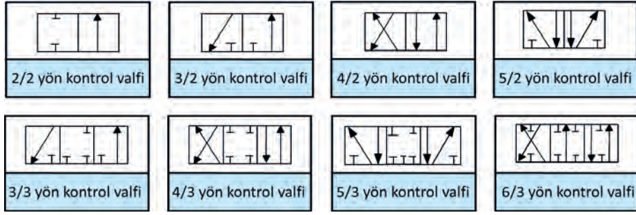
Şekil 3.16: Pnömatik devrelerde yaygın olarak kullanılan yön kontrol valflerinin sembolleri
