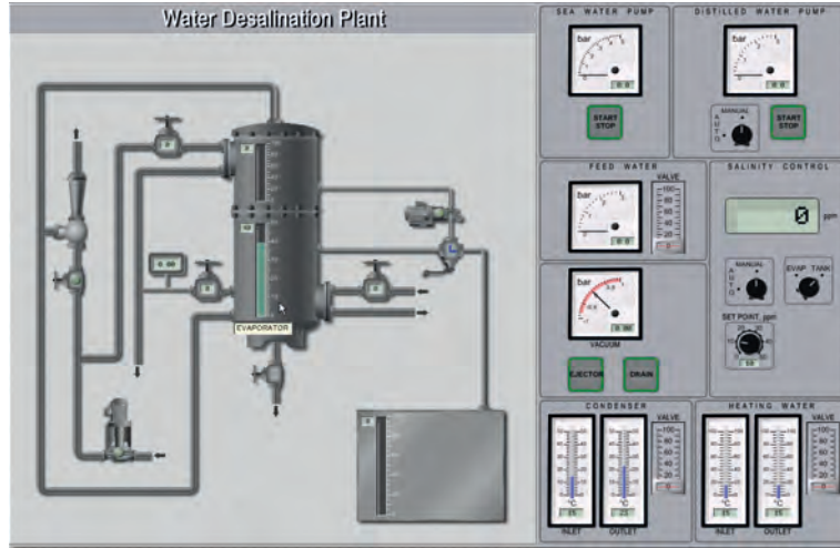
Şekil 8.8: Tatlı su üretme otomasyon kontrol ekranı
