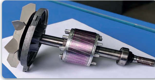
Görsel 5.3: Sincap kafesli rotor
