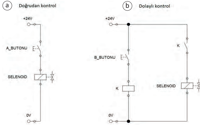
Şekil 3.26: Doğrudan kontrol (a) ve dolaylı kontrol (b) elektrik devre şemaları
