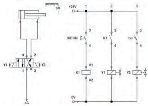
Şekil 3.31: Çift etkili pnömatik silindirin elektropnömatik kontrolü
