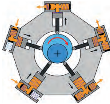
Şekil 1.14: Radyal pistonlu pompa
