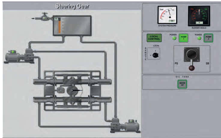
Şekil 8.14: Dümen monitör otomasyon kontrol ekranı
