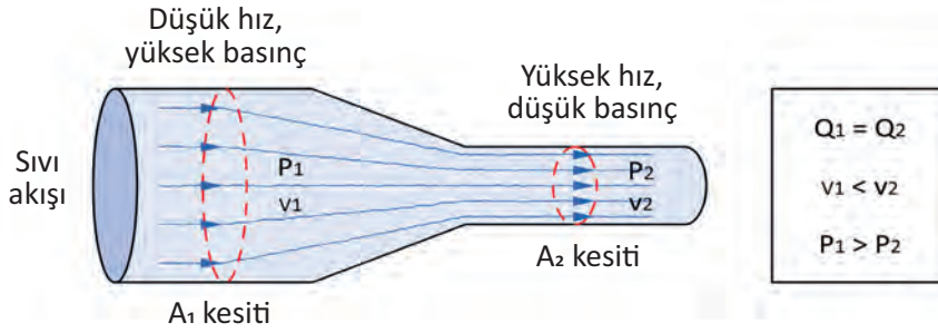
Şekil 1.7: Bernoulli prensibi
