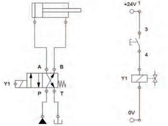
Şekil 1.61: Çift etkili hidrolik silindirin elektrohidrolik doğrudan kontrol devresi
