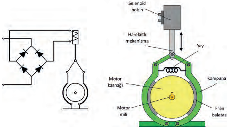
Şekil 5.18: Balatalı fren
