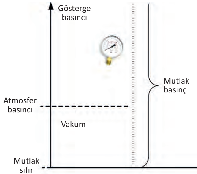
Şekil 3.1: Basıncı çeşitleri arasındaki ilişki
