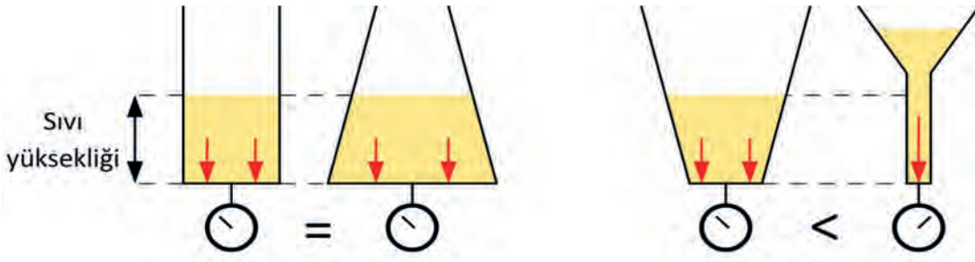
Şekil 1.2: Hidrostatik basınç
