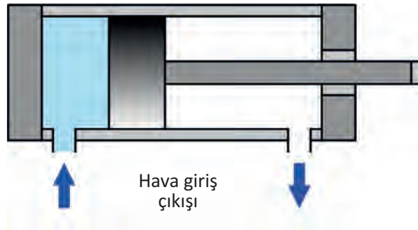
Şekil 3.6: Çift etkili pnömatik silindir
