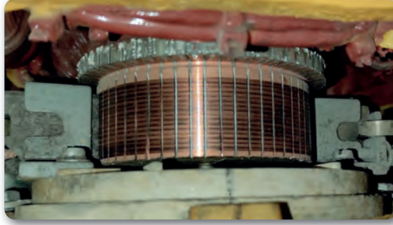
Görsel 6.5: Kollektör
