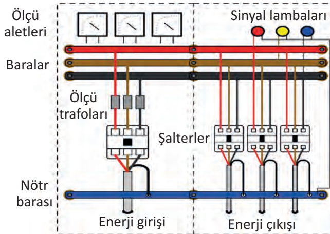
Şekil 7.12: Örnek dağıtım panosu bağlantıları
