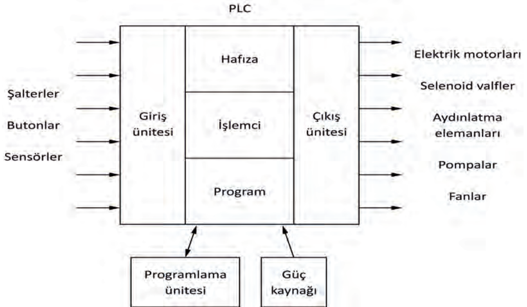
Şekil 8.2: PLC'nin yapısı
