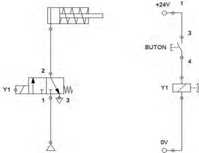
Şekil 3.25: Elektropnömatik devre şeması
