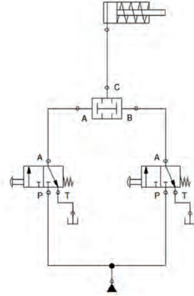
Şekil 1.51: VE valfiyle tek etkili hidrolik silindirin kontrolü
