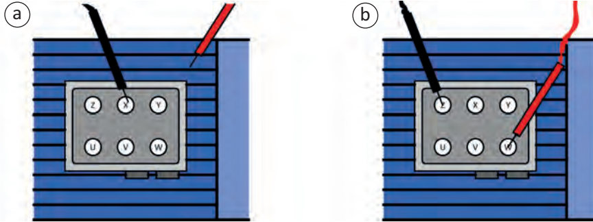
Şekil 5.15: Sargılarda gövdeye kaçak kontrolü (a) ile sargılarda kopukluk ve kısa devre kontrolü (b)
