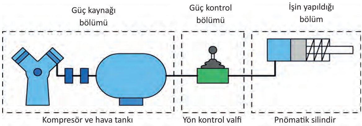
Şekil 3.11: Pnömatik sistemin bölümleri
