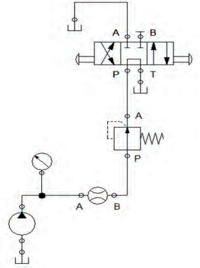
Şekil 2.7: Hidrolik pompa test düzeneği
