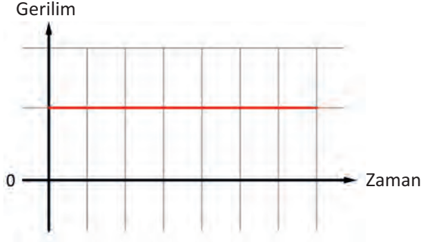
Şekil 6.1: Doğru akım
