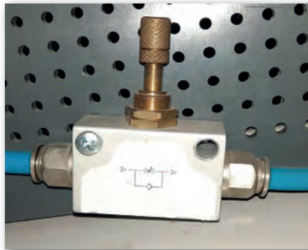
Görsel 3.10: Akış kontrol valfi
