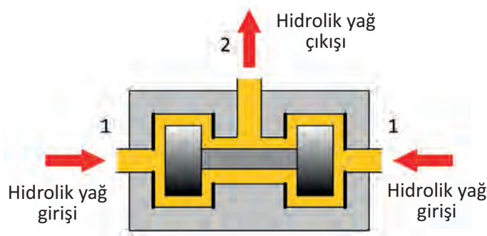
Şekil 1.22: VE valfi
