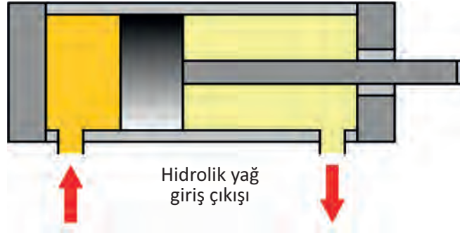
Şekil 1.30: Çift etkili hidrolik silindir
