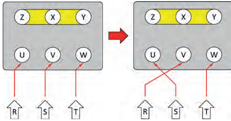
ŞEKİL 5.14: Üç fazlı asenkron motorun dönüş yönünün değiştirilmesi
