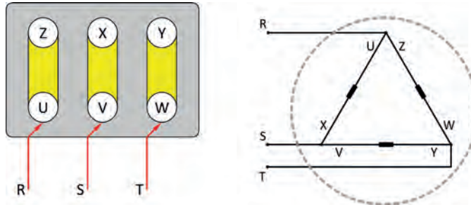
Şekil 5.7: Üçgen bağlantı
