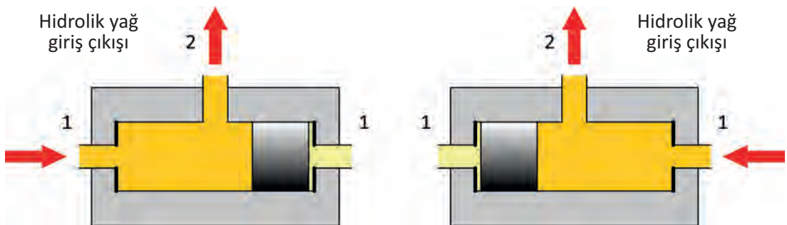
Şekil 1.21: VEYA valfi
