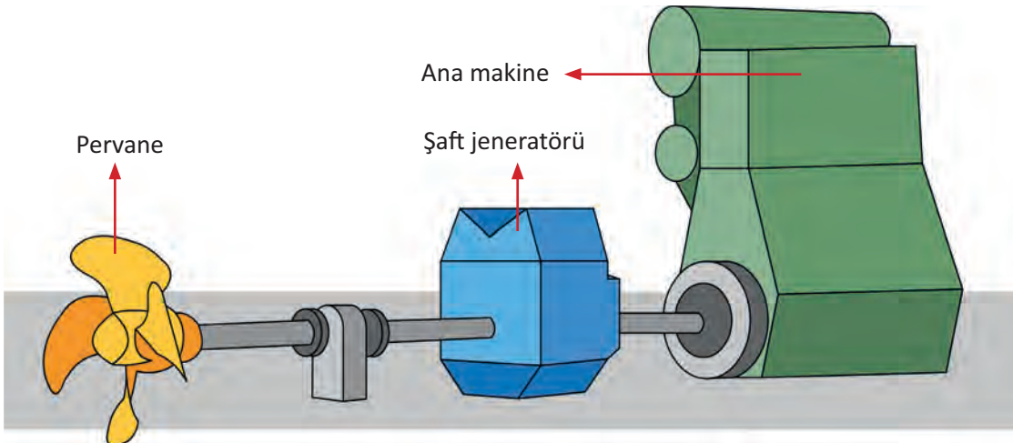
Şekil 7.3: Şaft jeneratörü
