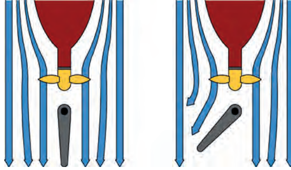
Şekil 2.9: Dümen yelpazesinin döndürülmesiyle geminin yön değişmesi
