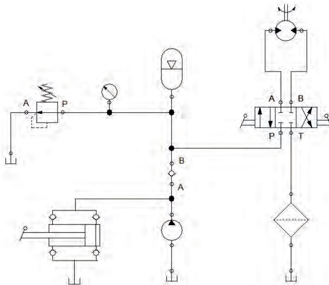
Şekil 2.4: Tek kollu matafora hidrolik devresi
