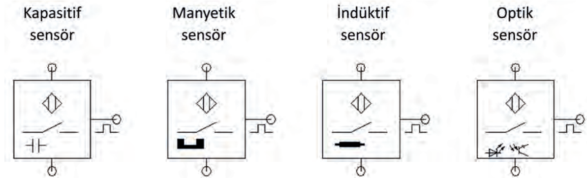
Şekil 1.53: Temassız sensör çeşitleri ve sembolleri
