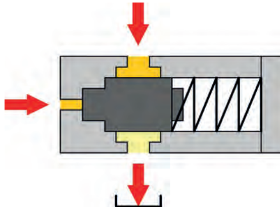
Şekil 1.26: Boşaltma valfi
