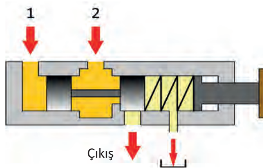
Şekil 1.23: Basınç sıralama valfi
