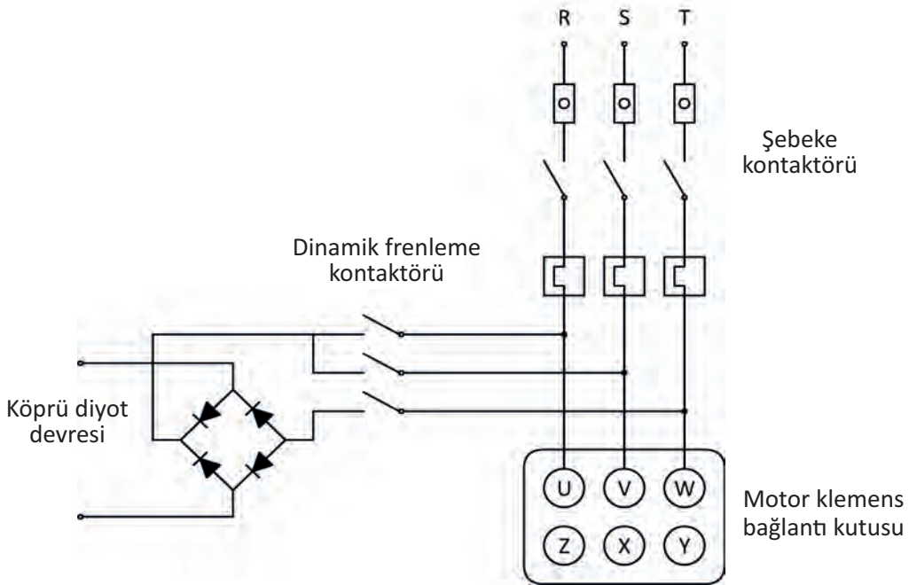
Şekil 5.17: Dinamik fren
