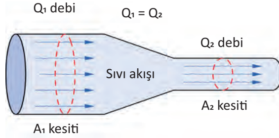
Şekil 1.6: Süreklilik prensibi
