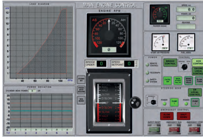
Şekil 8.11: Gemi ana makine otomasyon kontrol ekranı
