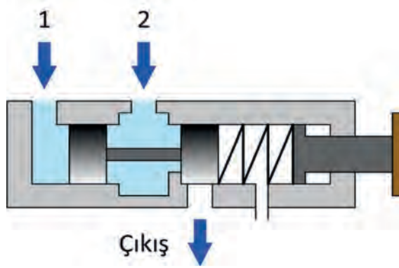
Şekil 3.3: Basınç sıralama valfi
