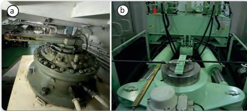
Görsel 2.14: Döner kanatlı tip (a) ve silindirli tip (b) dümen donanımları
