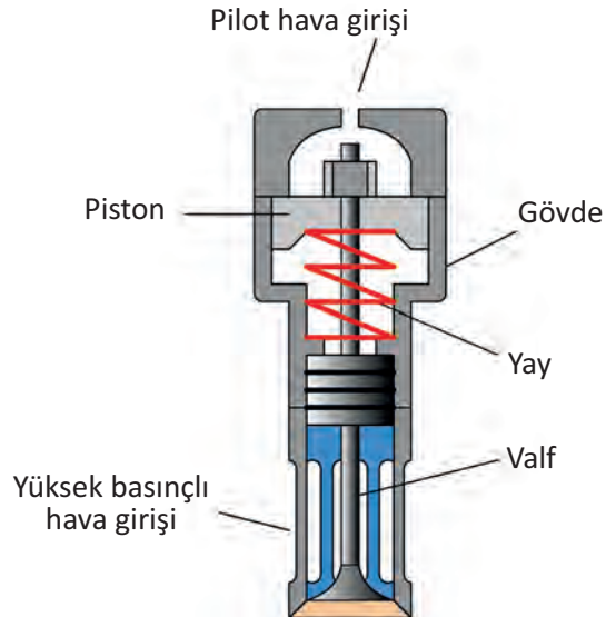
Şekil 4.4: Starting valf kesiti
