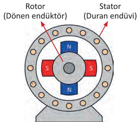
Şekil 7.5: Duran endüvili AC jeneratör
