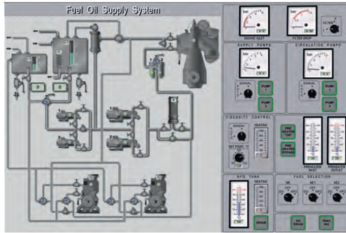
Şekil 8.13: Yakıt besleme otomasyon kontrol ekranı
