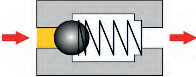
Şekil 1.28: Çek valf
