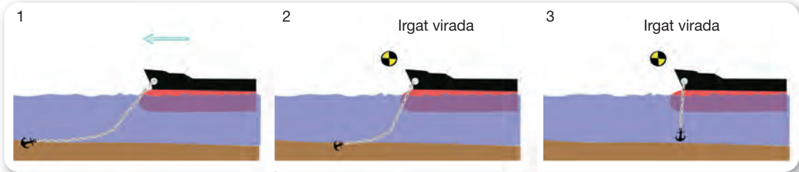
Şekil 8.12: Demir alma operasyonu
