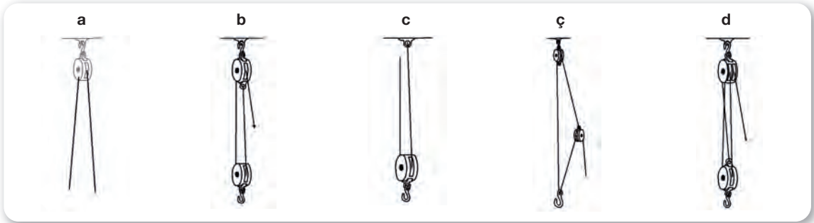
Şekil 4.6: Palangalar 1
