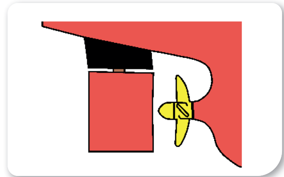
Şekil 6.4: Okyanus tipi Schilling dümen
