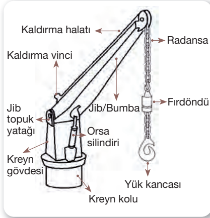
Şekil 4.14: Kreyinin kısımları
