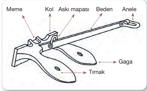
Şekil 4.2: Demirin kısımları
