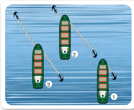
Şekil 8.9: İleriye boyuna demirleme
