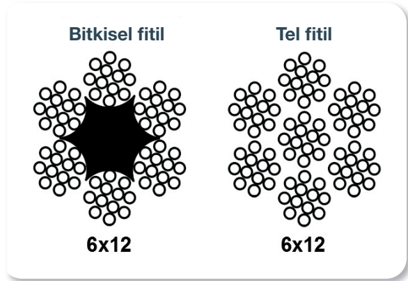
Şekil 2.1: Tel halat kesiti
