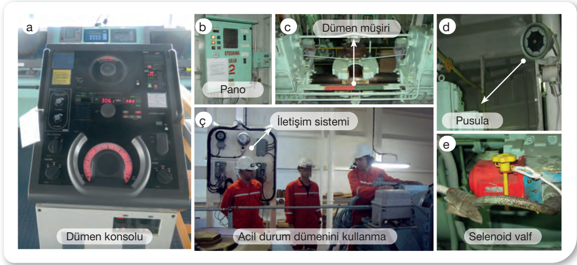
Görsel 9.4: Acil durum dümen donanımını kullanma
