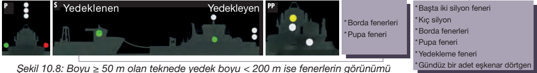
Şekil 10.8: Boyu >= 50 m olan teknede yedek boyu < 200 m ise fenerlerin görünümü
