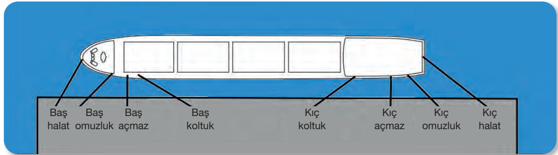
Şekil 2.2: Bağlama halatları
