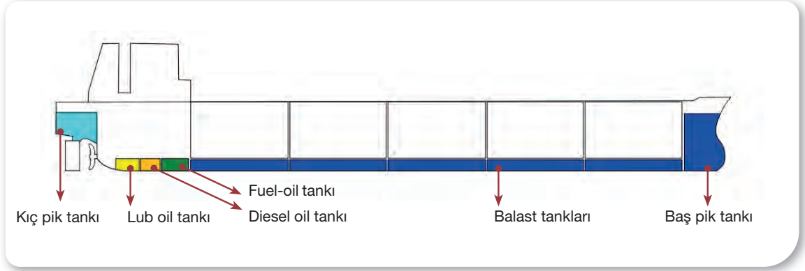
Şekil 5.4: Geminin bünyesel tankları
