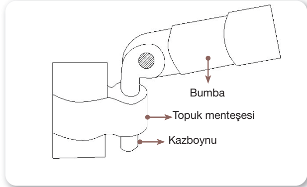
Şekil 4.12: Kazboynu
