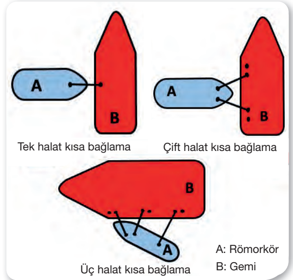
Şekil 6.7: Römorkör kısa bağlama yöntemi
