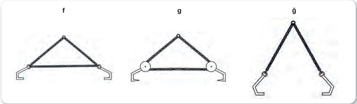
Şekil 4.10: Sapanlar 3
