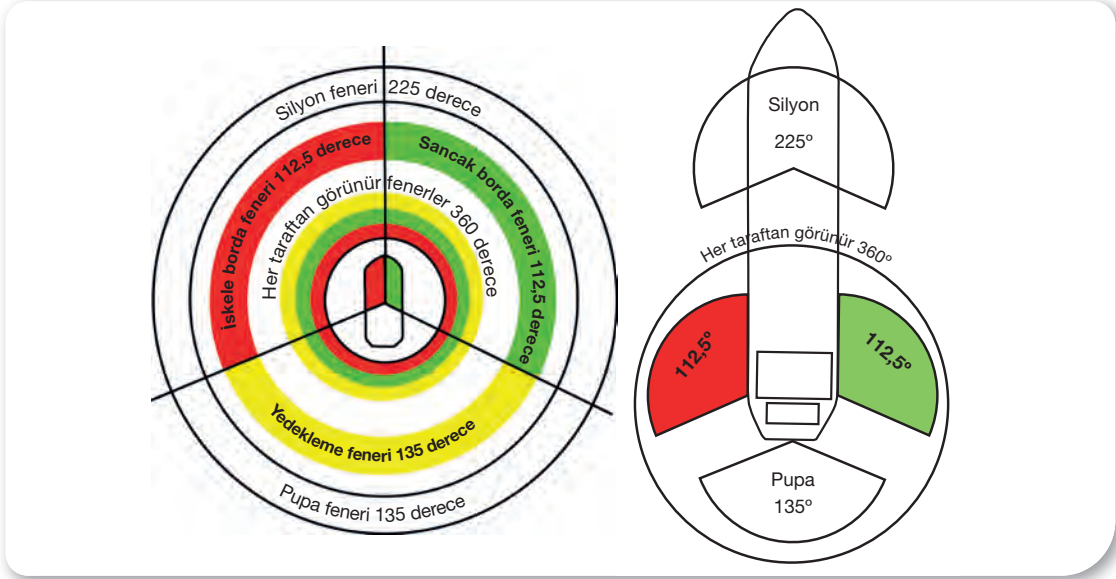
Şekil 10.1: Fenerlerin görülme sektörleri
