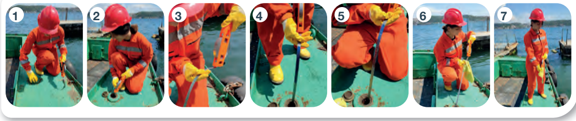
Görsel 5.8: İskandil alma aşamaları
