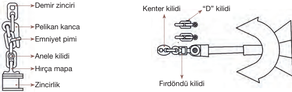
Şekil 4.3: Zincir bağlantıları
