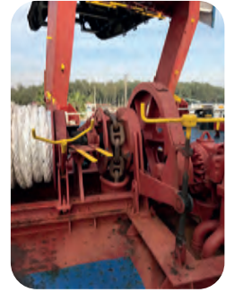
Görsel 4.1: İrgat
