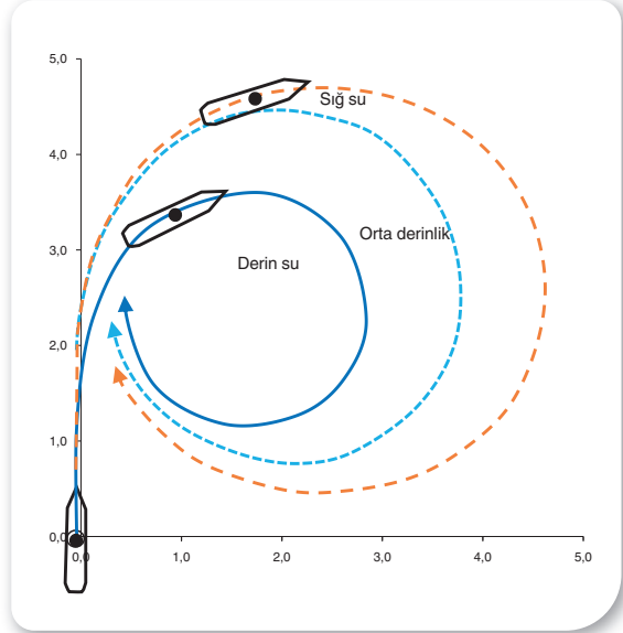
Şekil 7.4: Derin ve sığ suda dönme çemberi
