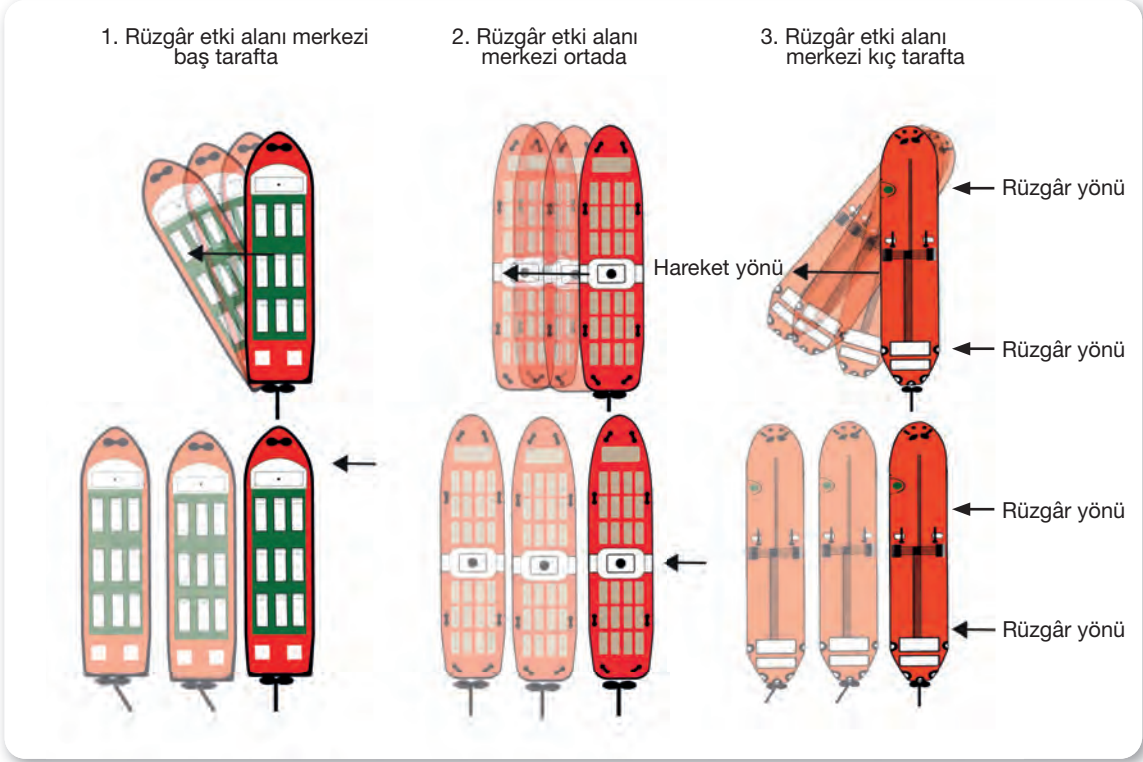
Şekil 9.5: Rüzgâr etki merkezleri
