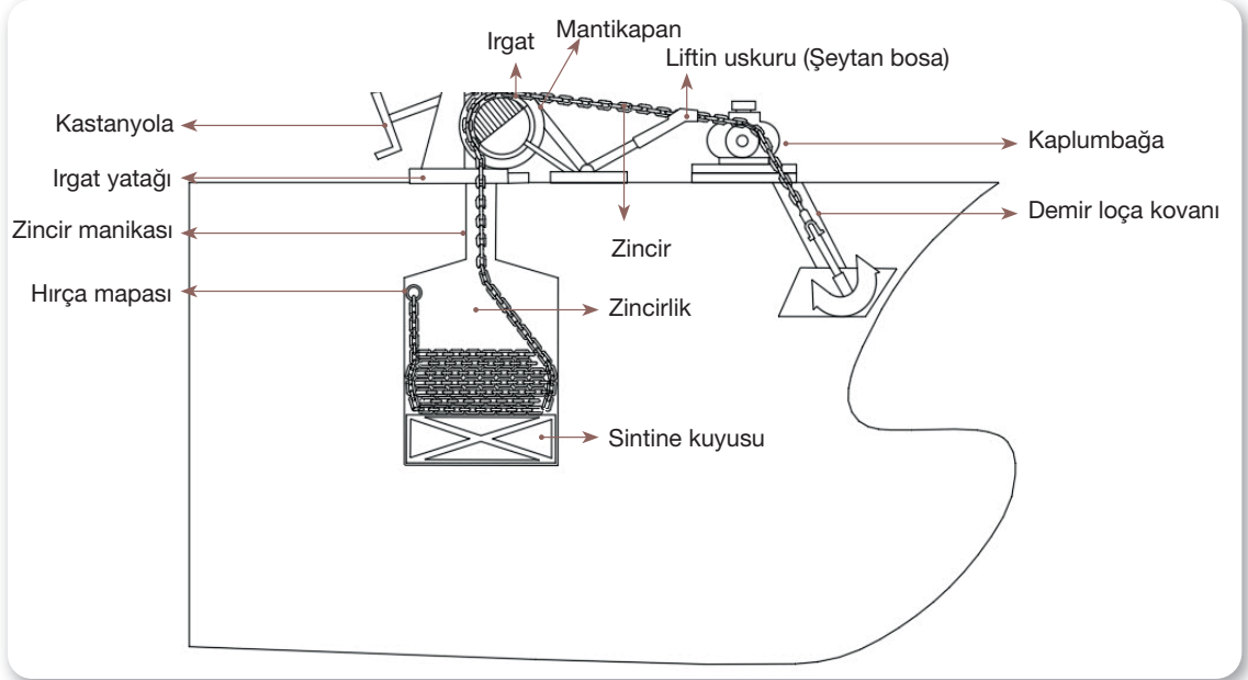
Şekil 4.1: Demirleme donanımları
