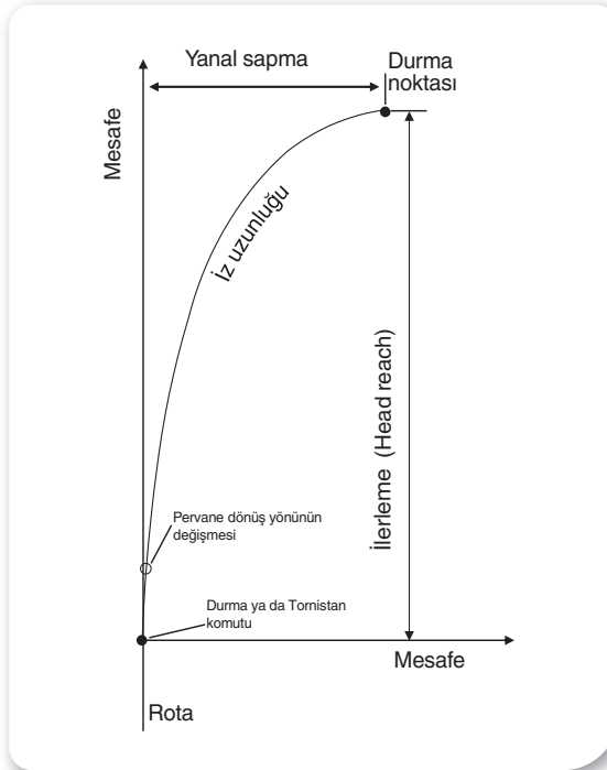
Şekil 7.3: Durma mesafesi
