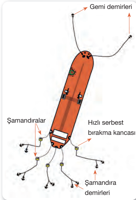
Şekil 8.15: Çok şamandıralı bağlama sistemi
