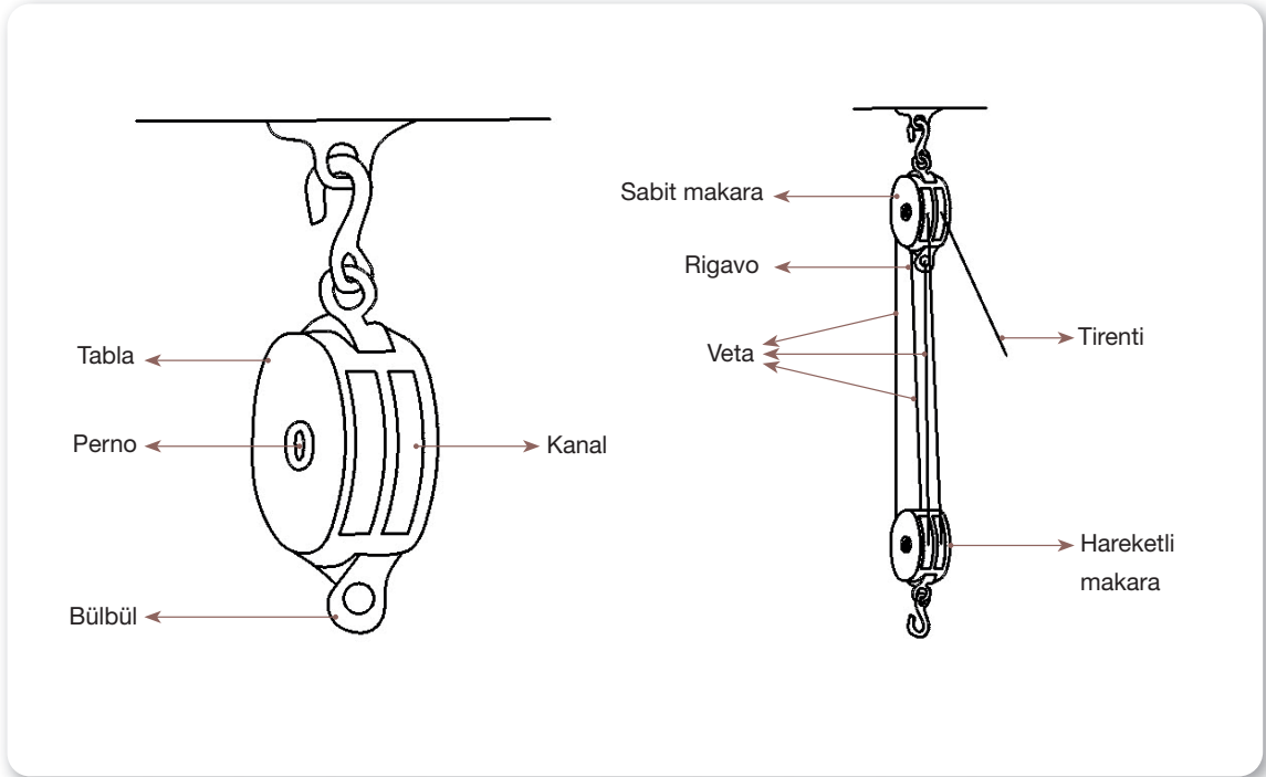
Şekil 4.5: Makara ve palanganın kısımları
