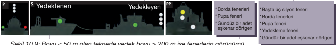
Şekil 10.9: Boyu < 50 m olan teknede yedek boyu >= 200 m ise fenerlerin görünümü
