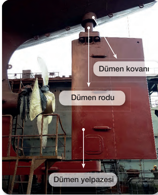
Görsel 6.4: Dümenin kısımları
