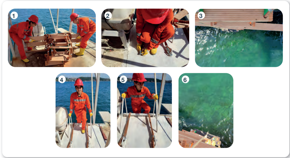
Görsel 3.3: Pilot çarmihını donatma ve istifleme aşamaları
