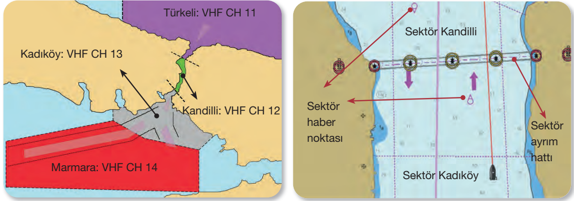
Şekil 10.48: İstanbul Boğazı sektör alanları, VHF kanalları ve sektör haber noktası
