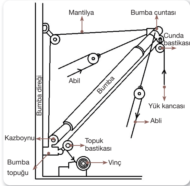
Şekil 4.13: Tek bumba donanımı
