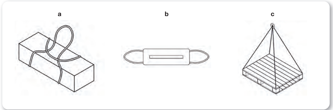
Şekil 4.8: Sapanlar 1
