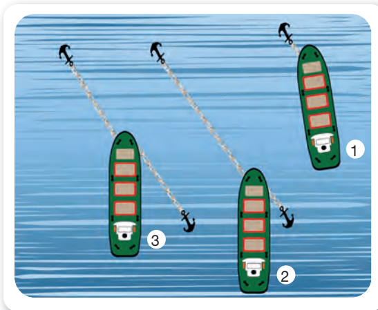
Şekil 8.10: Geriye boyuna demirleme
