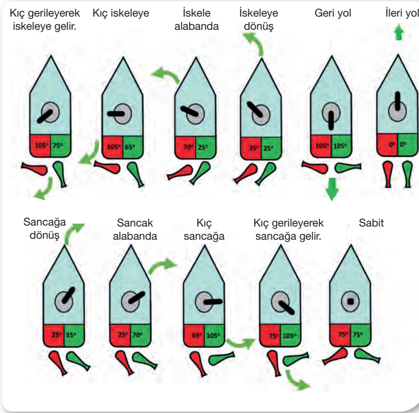
Şekil 6.5: İkiz Schilling dümenli geminin hareketleri
