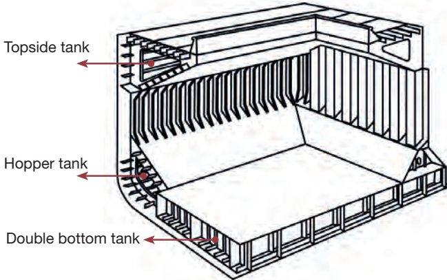
Şekil 5.3: Ambar kesiti
