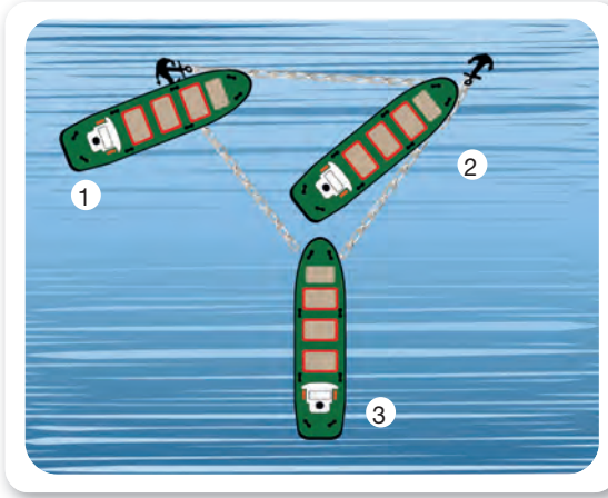
Şekil 8.8: Açık bağlama
