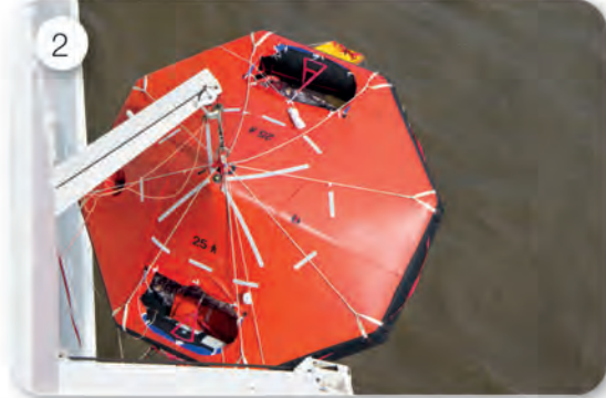
Görsel 5.12: Mataforalı can salını indirme aşamaları
