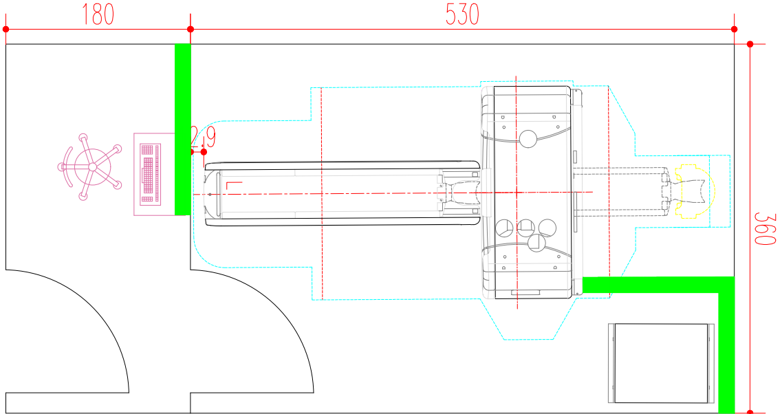
Örnek 4.3: Tomografi odası yerleşim planı şeması
