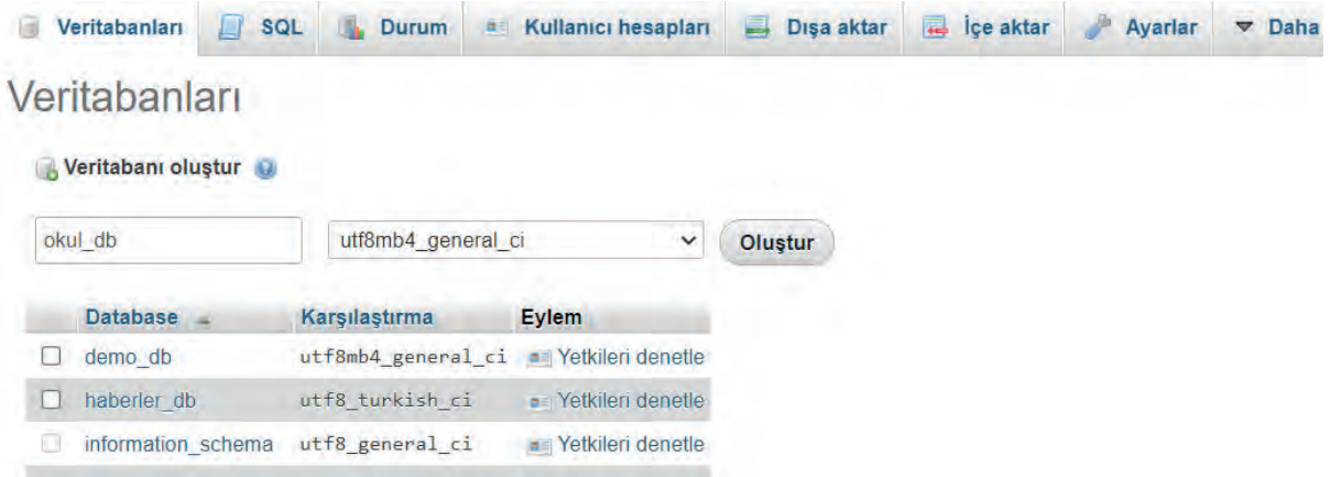
Görsel 9.5: phpMyAdmin ile veri tabanı oluşturma sayfası
