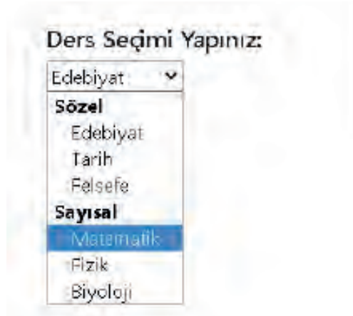
Görsel 5.9: Optgroup özelliği
