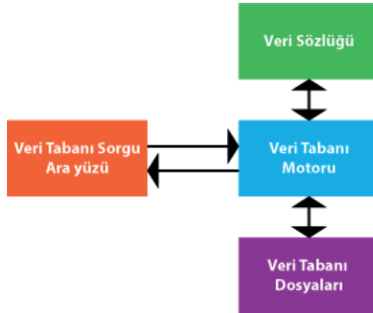
Görsel 9.1: Veri tabanı yönetim sistemi çalışma şeması
