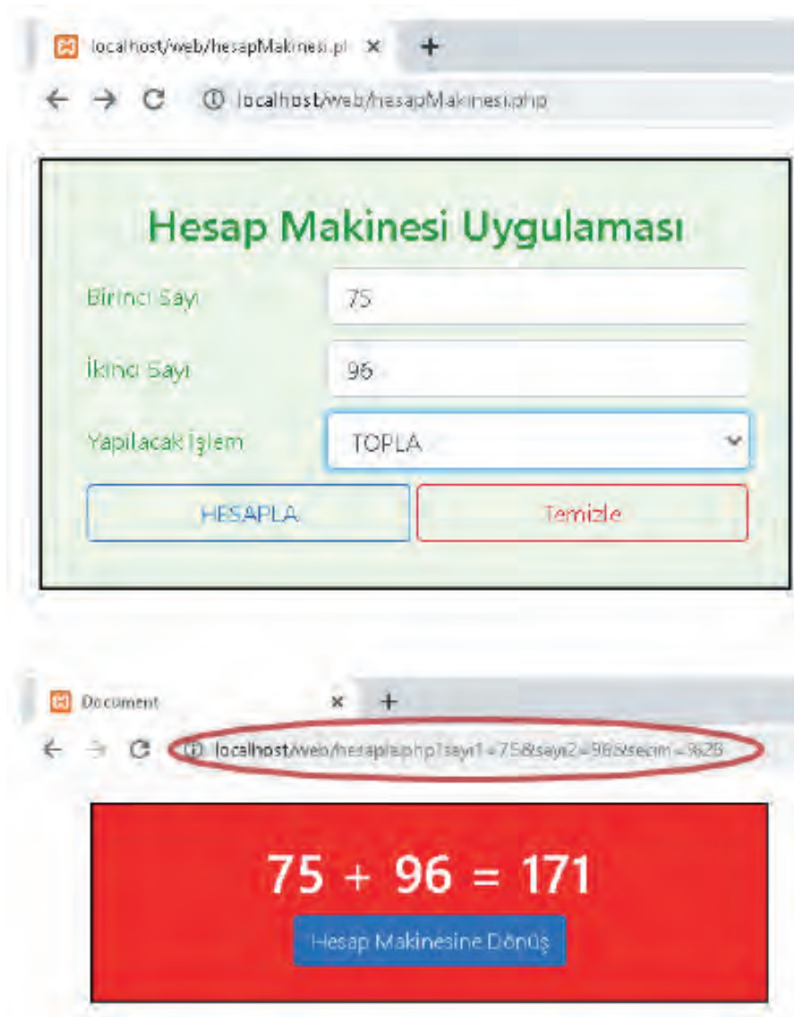
Görsel 5.13: Hesap makinesi
