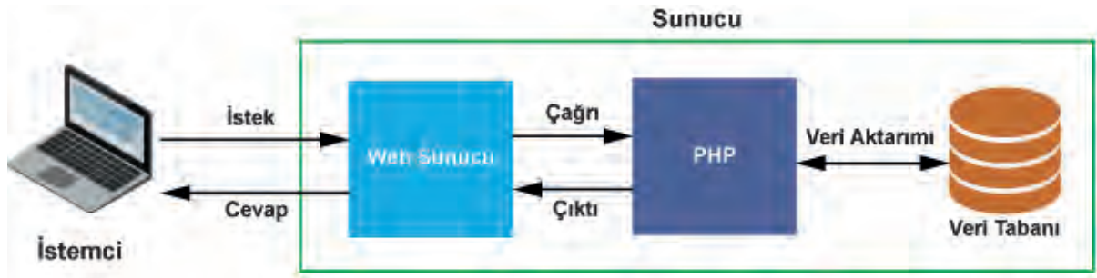
Görsel 1.1: PHP sayfalarının istemci ile sunucu arasındaki iletişimi
