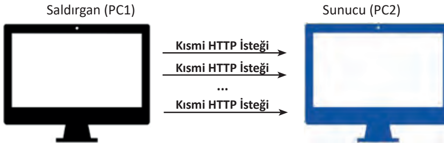
Görsel 7.19: Slowloris aracı ile saldırı davranışı
