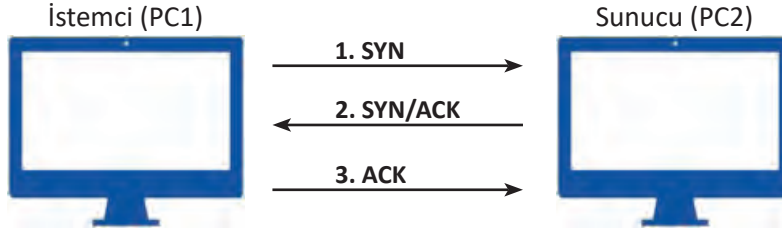
Görsel 7.12: TCP Üç Yollu El Sıkışma modeli
