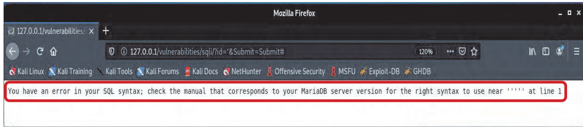
Görsel 8.6: SQL Injection sorgusu sonucu dönen hata bilgisi
