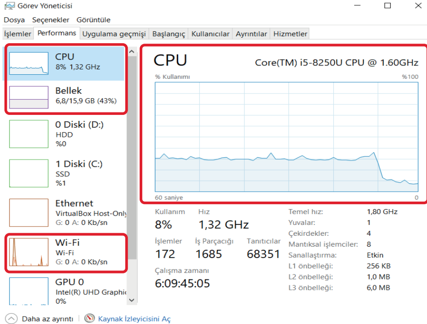
Görsel 7.10: Hulk aracıyla atak sonlandırıldıktan sonra bilgisayar kaynak bilgileri
