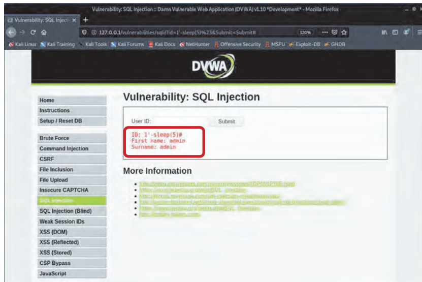
Görşel 8.13: Belirli bir zaman geçtikten sonra verilen sorgu cevabı
