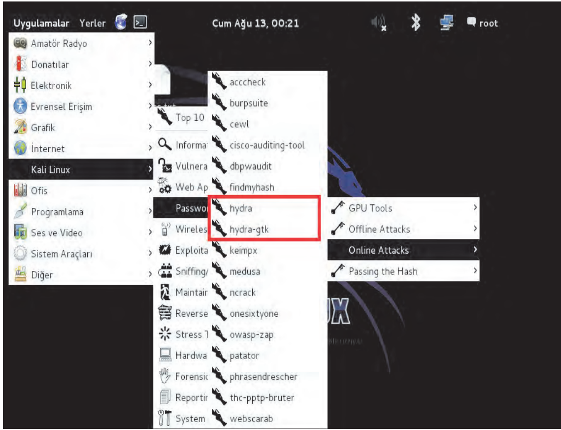
Görsel 6.2: Kali işletim sistemi hydra ve hydra-gtk araçlarına ulaşım
