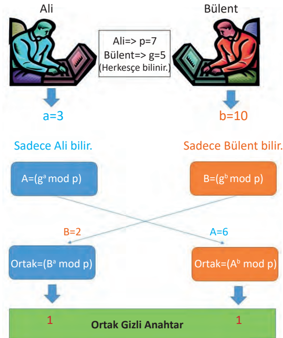
Görsel 5.15: Diffie-Hellman anahtar değişimi prensibi
