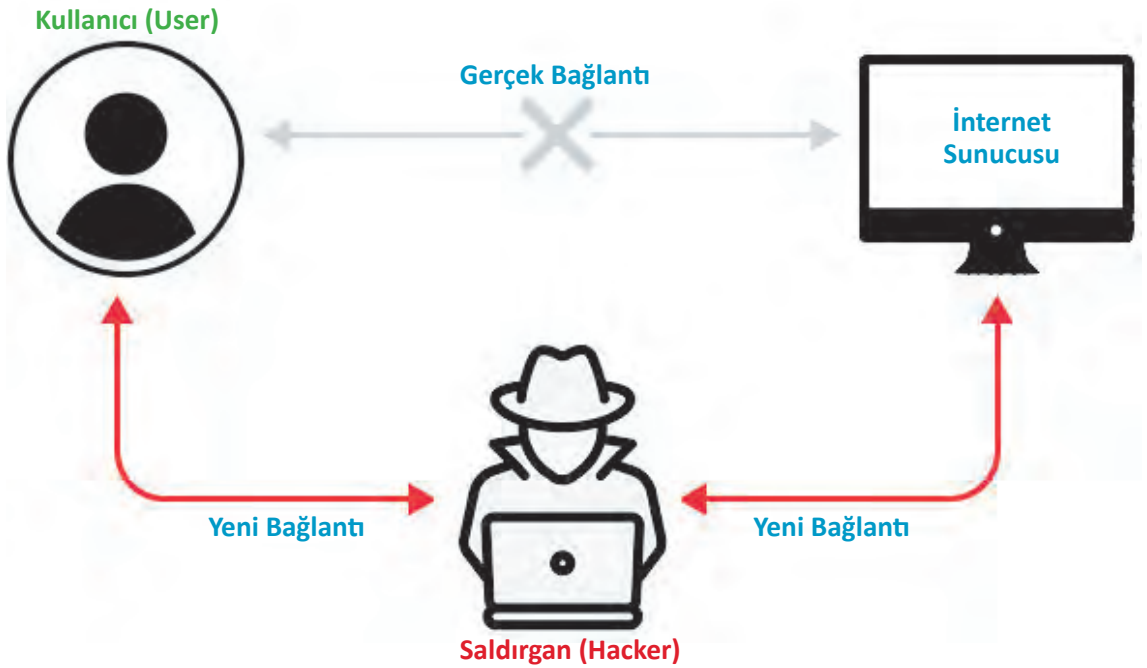
Görsel 4.24: Ortadaki adam saldırısı (MITM)
