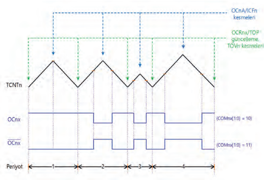
Görsel 4.50: Doğru faz ve frekans PWM modu zamanlama diyagramı
