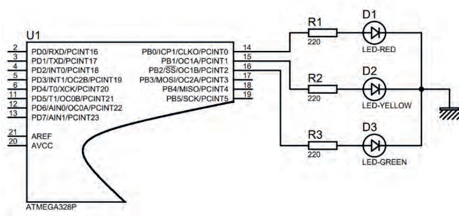
Görsele 2.70: Uygulama devresi
