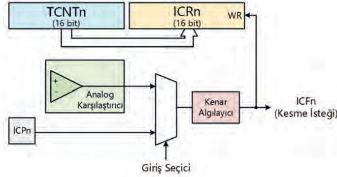
Görşel 4.47: Giriş yakalama birimi basitleştirilmiş blok şeması
