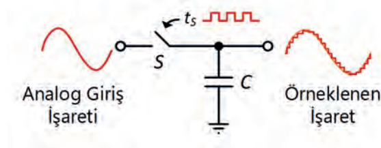
Görsel 4.8: Örnekleme / tutma devresi
