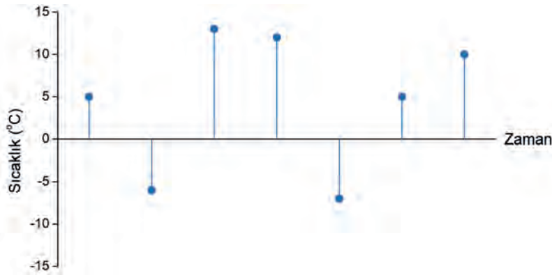
Görsel 4.3: Örneklem periyodu Görsel 4.2’deki işarettten iki kat büyük olan ayırık zamanlı işaret
