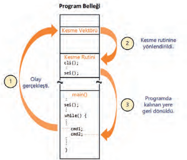
Görsel 4.25: Kesme işleminin adımları
