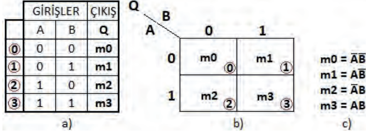
Görsel 1.45: a) Doğruluk tablosu Görsel 1.45: b) Karno haritası Görsel 1.45: c) Lojik ifadeler
