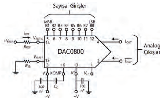
Görsel 4.29: DAC0800 entegresi örnek uygulaması
