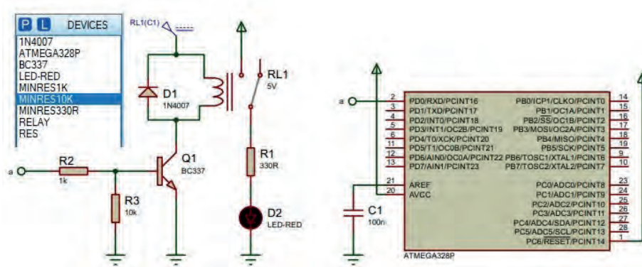
Görsel 3.47: 3.9 No.lu uygulama için simülasyon devre şeması
