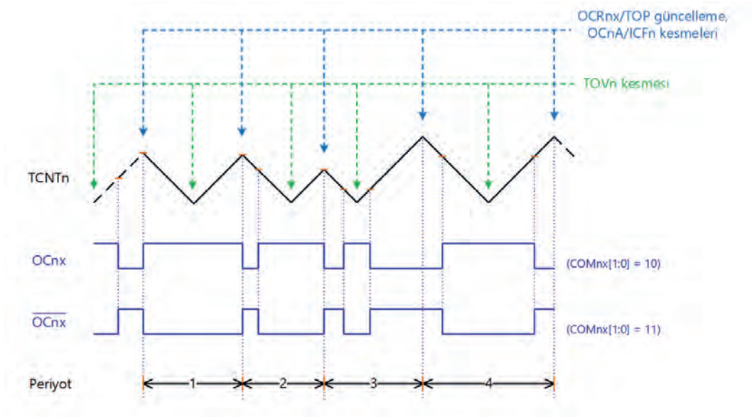
Görsel 4.49: Doğru faz PWM modu zamanlama diyagramı
