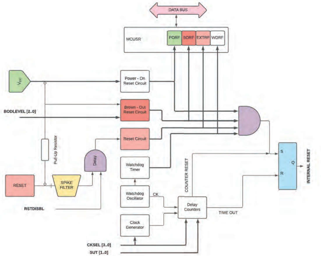
Görsel 2.25: Atmega328P reset devreleri
