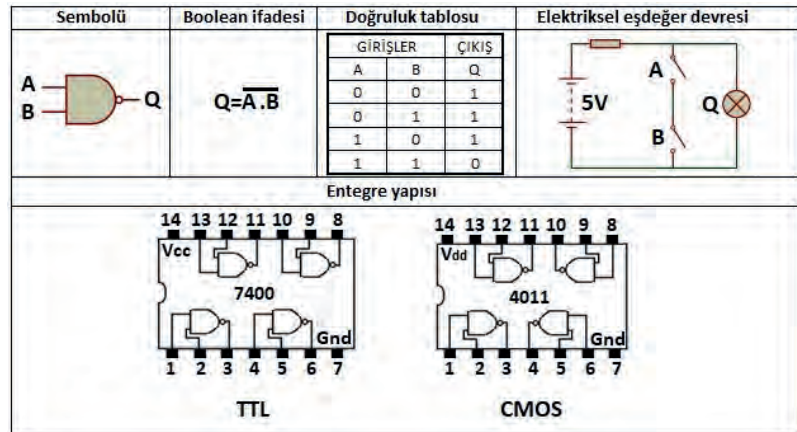
Görsel 1.16: VE DEĞİL kapısı
