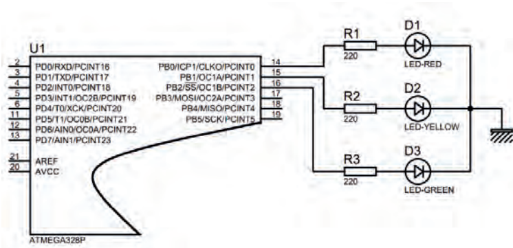
Görsel 2.77: Uygulama devresi
