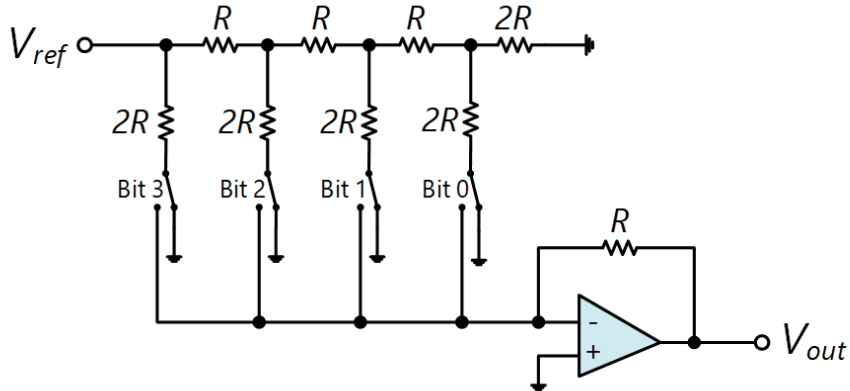
Görsel 4.27: R-2R merdiven direnç tipi DAC devre şeması
