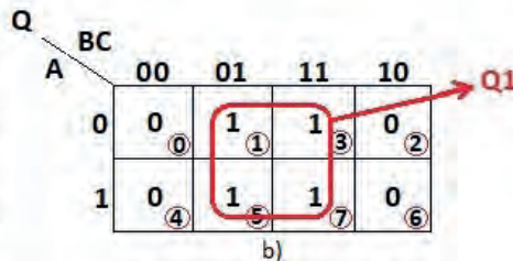
Görsel 1.50: a) Örnek 39'un doğruluk tablosu Görsel 1.50: b) karno haritası
