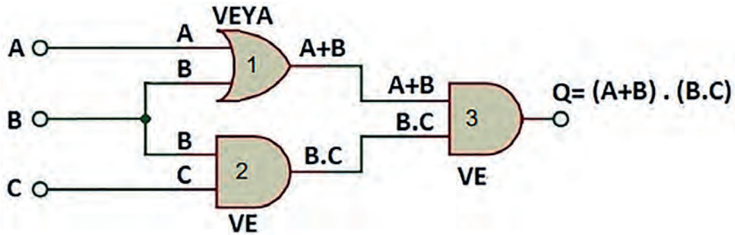
Görsel 1.24: Lojik devrenin lojik ifadesi
