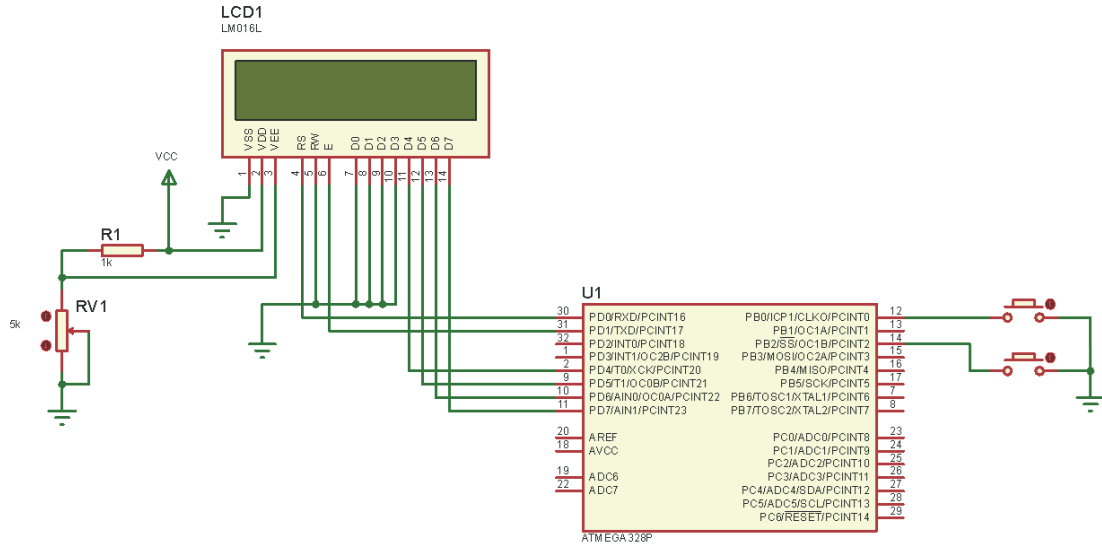
Görsel 4.59: Uygulama 4.7 için simülasyon devre şeması
