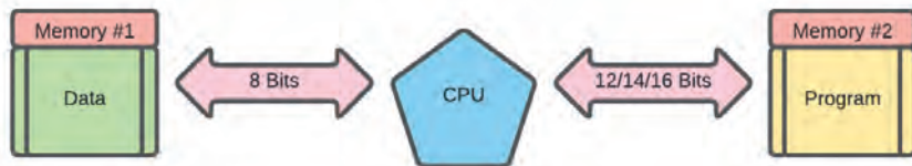
Görsel 2.11: Harvard Mimarisi
