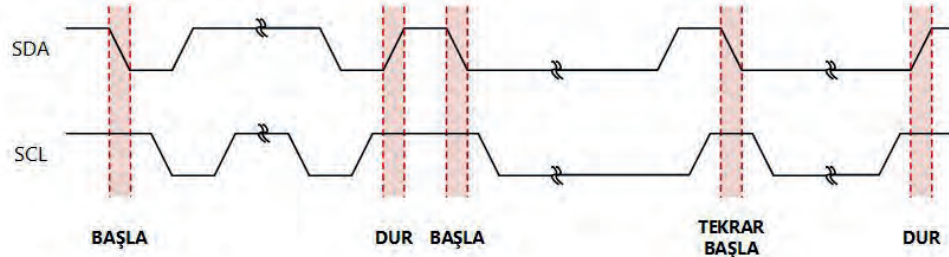
Görsel 3.83: BAŞLA, TEKRAR BAŞLA ve DUR durumları
