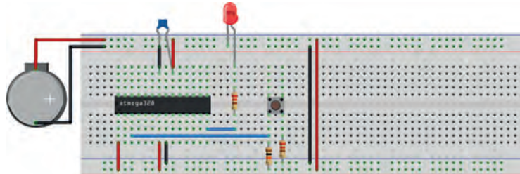
Görsel 2.76: 2.4 No.lu uygulama için breadboard eleman dizilimi
