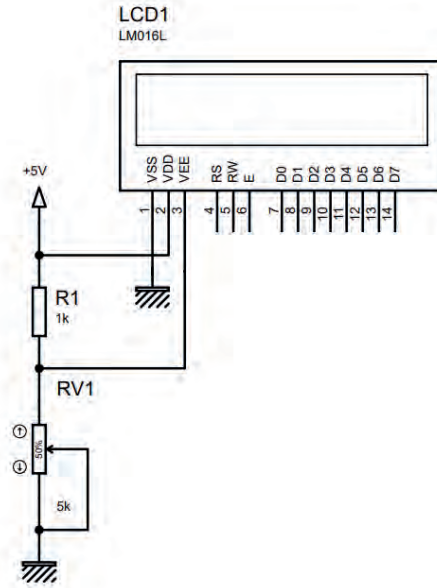
GörSEL 3.25: LCD besleme ve kontrast bağlantısı
