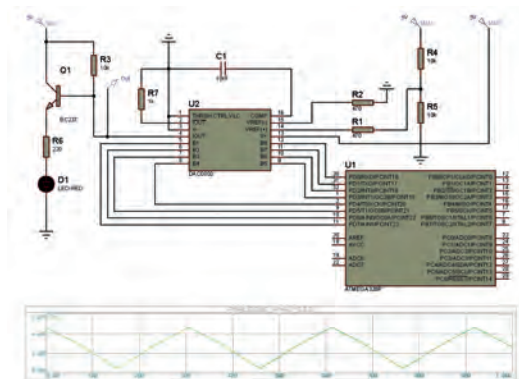
Görsel 4.30: Uygulama 4.4 için simülasyon devresi
