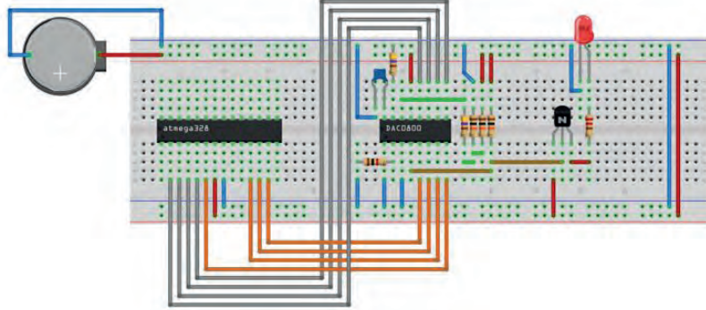
Görsel 4.31: Uygulama 4.4 için breadboard üzerine kurulan devre
