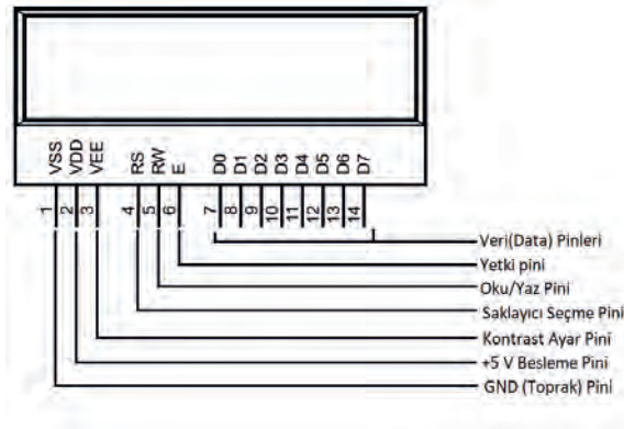
Görsel 3.24: Karakter LCD pin isimleri
