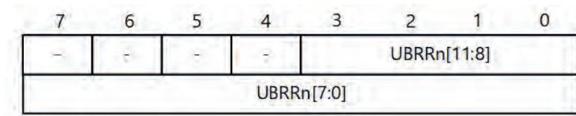
Görsel 3.79: UBRRn kaydedicisi
