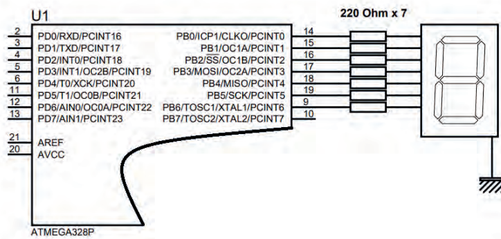
Görsel 3.9: Uygulama devresi
