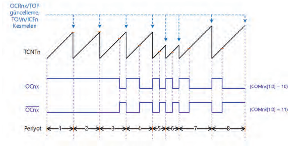
Görsel 4.48: Hızlı PWM modu zamanlama diyagramı
