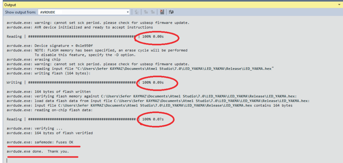
Görsel 2.91: Output penceresi
