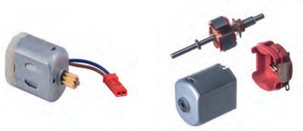
Görsel 3.51: DC motorun dış görünüşü ve iç yapısı
