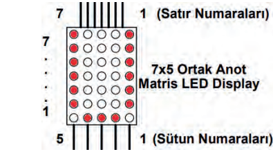
Görsel 3.16: Matris Display LED (U harfi)
