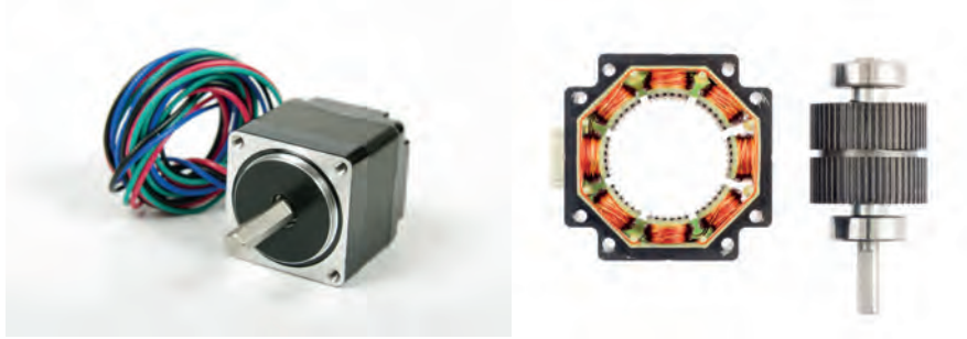
Görsel 3.59: Step Motor dış ve iç görünüşü
