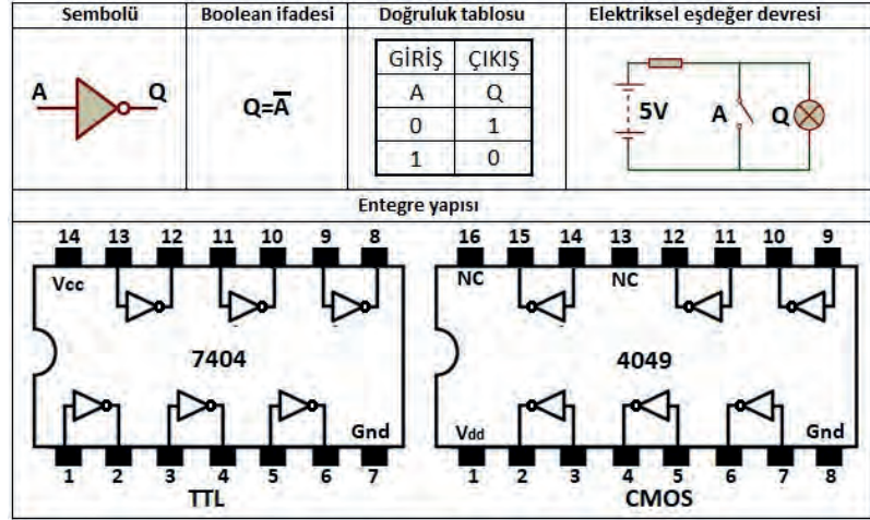
Görsel 1.15: DEĞİL kapısı
