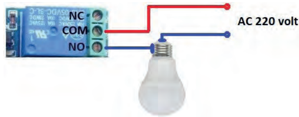
Görsel 3.45: Röle yük bağlantısı
