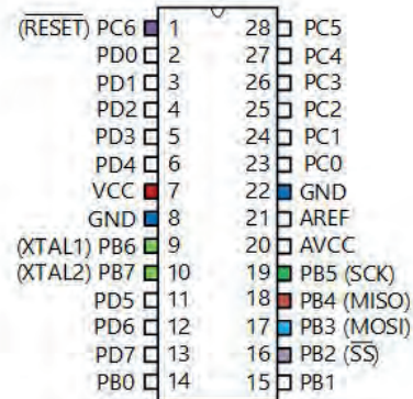
Görsel 3.64: Atmega328P mikrodenetleyicinin SPI modülü ile ilgili pinleri
