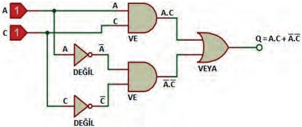
Görsel 1.37: Örnek 36'ya ait lojik devre
