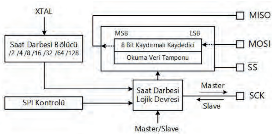
Görsel 3.62: SPI haberleşme modülü basitleştirilmiş blok şeması
