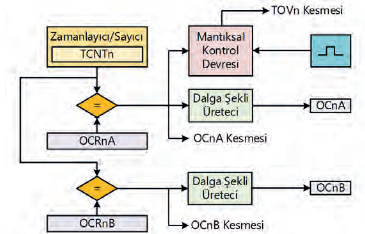
Görsel 4.32: Z/S modülü basitleştirilmiş blok şeması
