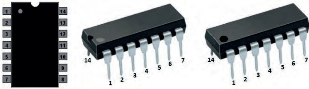
Görsel 1.36: Entegre bacak numaraları ve kılıfları
