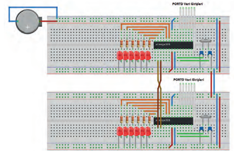
Görsel 3.81: 3.15 No.lu uygulama için breadboard üzerine kurulan devre
