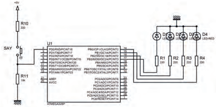
Görsel 2.80: Uygulama devresi
