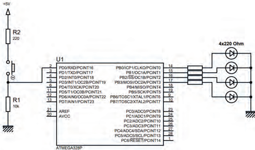
Grsel 2.101: 2.7 No.lu uygulama iin simlasyon devre řeması
