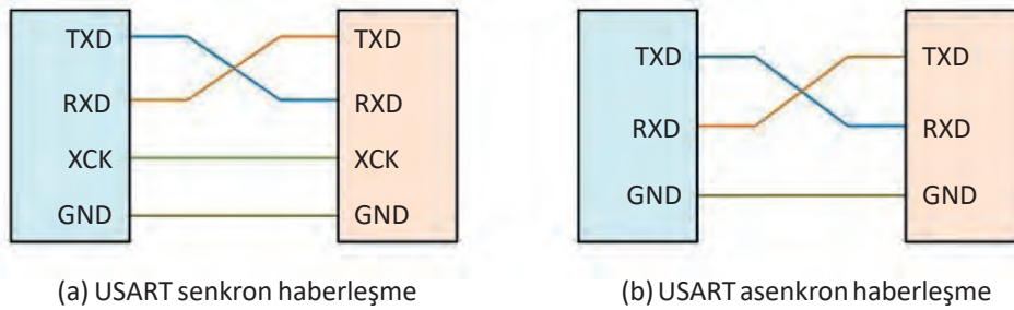
TXGörsel 3.73: USART cihaz bağlantıları
