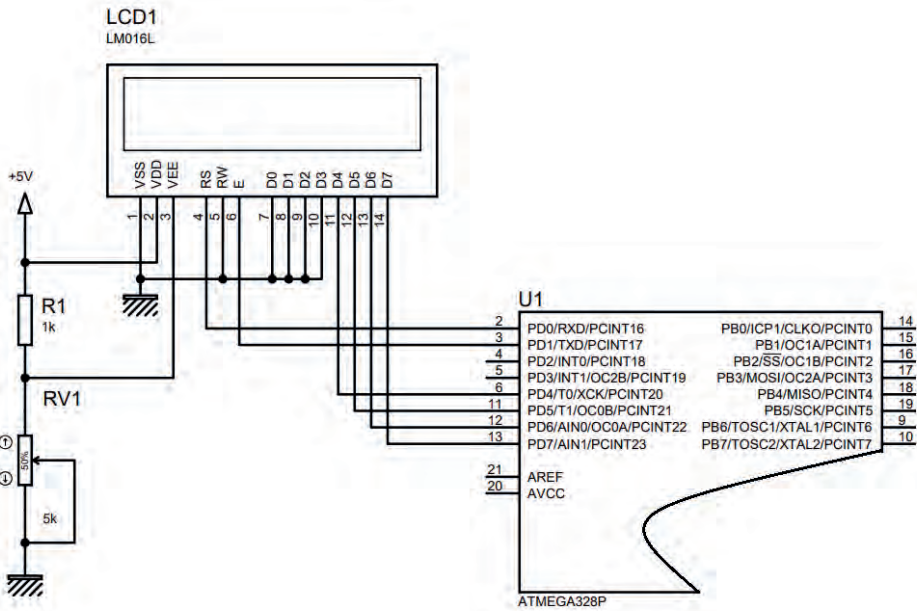
GörSEL 3.26: LCD'nin Denetleyiciye bağlanması
