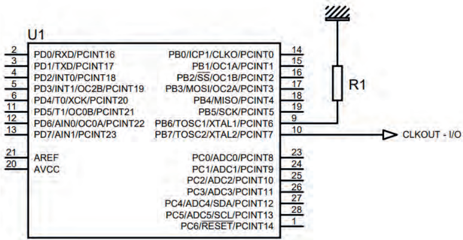
Görsel 2.23: ER osilatör bağlantısı
