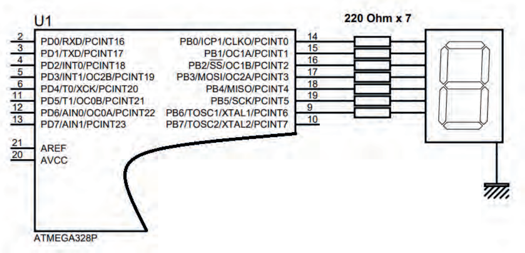
Görsel 3.7: 3.2 No.lu uygulama için simülasyon devre şeması
