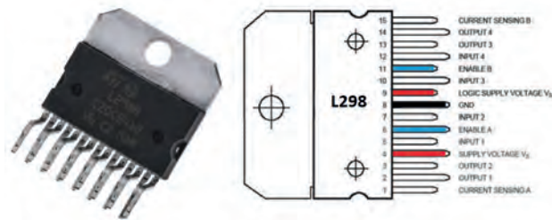
Görsel 3.56: L298 entegresinin dış görünümü ve pin isimleri
