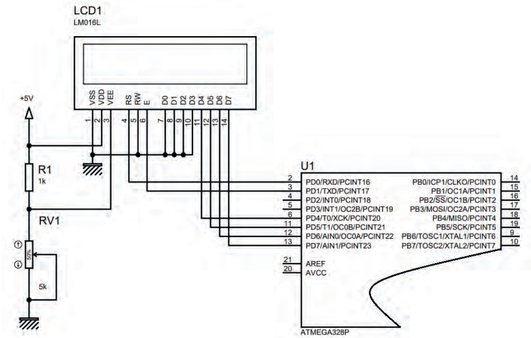
Görsel 3.27: 3.7 No.lu uygulama için simülasyon devre şeması
