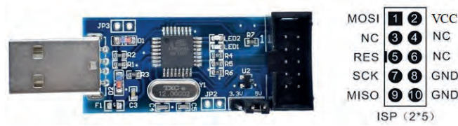
Görsel 2.83: Programlayıcı çıkış pinleri
