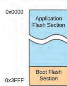
Görsel 2.8: Atmega328P Program belleği haritası
