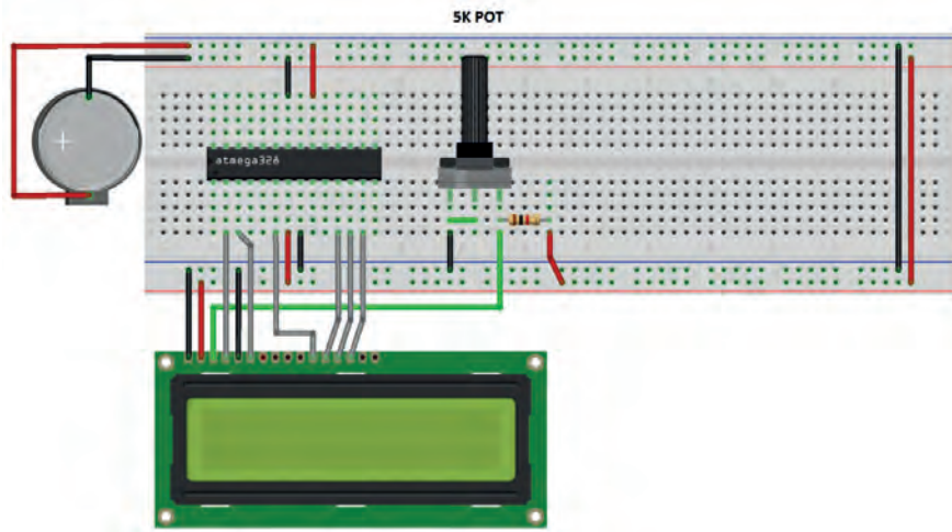
Görsel 3.28: 3.7 No.lu uygulama için breadboard eleman dizilimi
