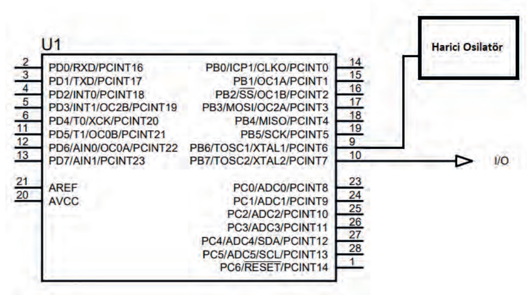
Görsel 2.24: EC osilatör bağlantısı
