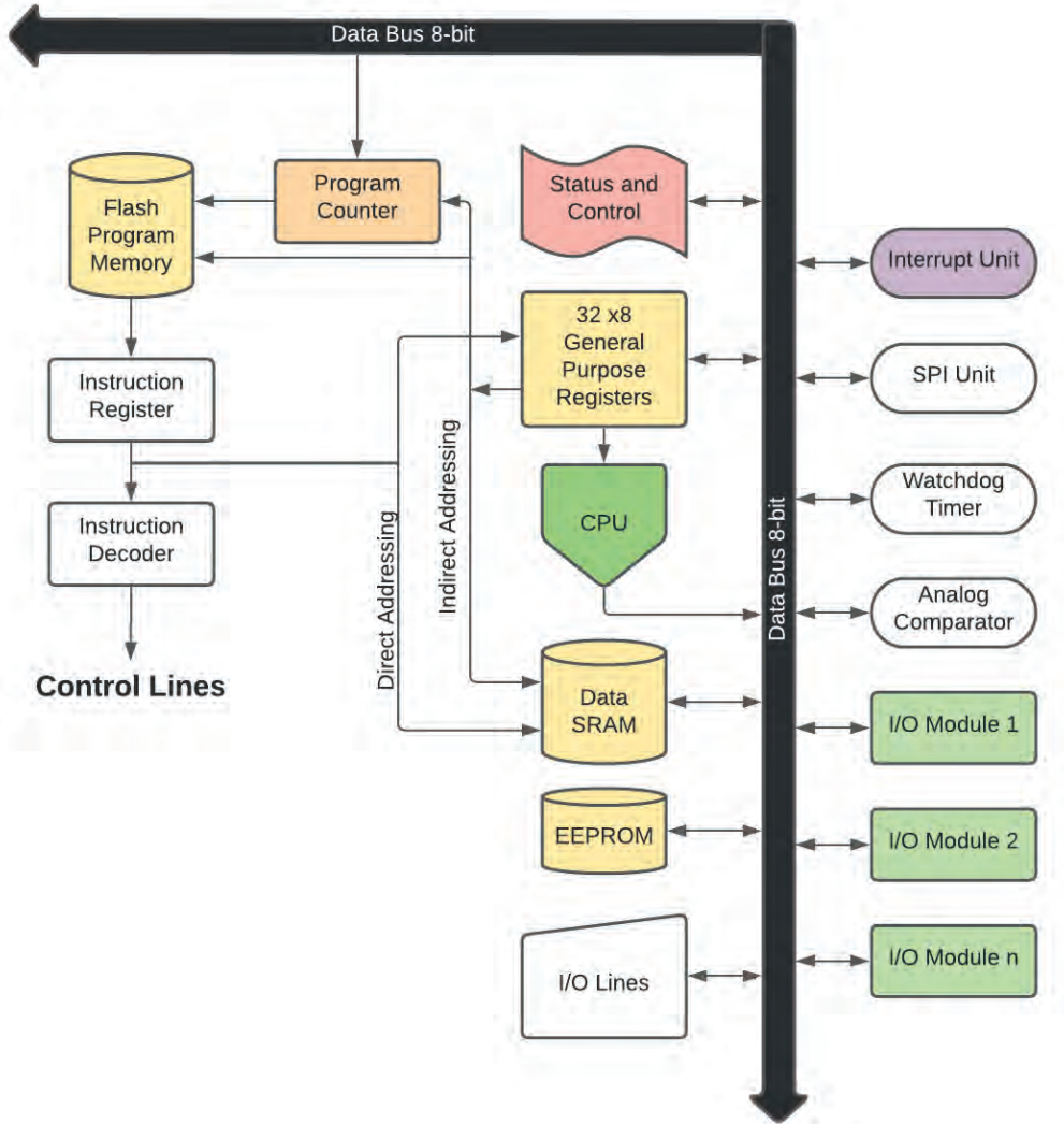
Görsel 2.5: Atmega328P mikrodenetleyicisinin CPU blok diyagramı
