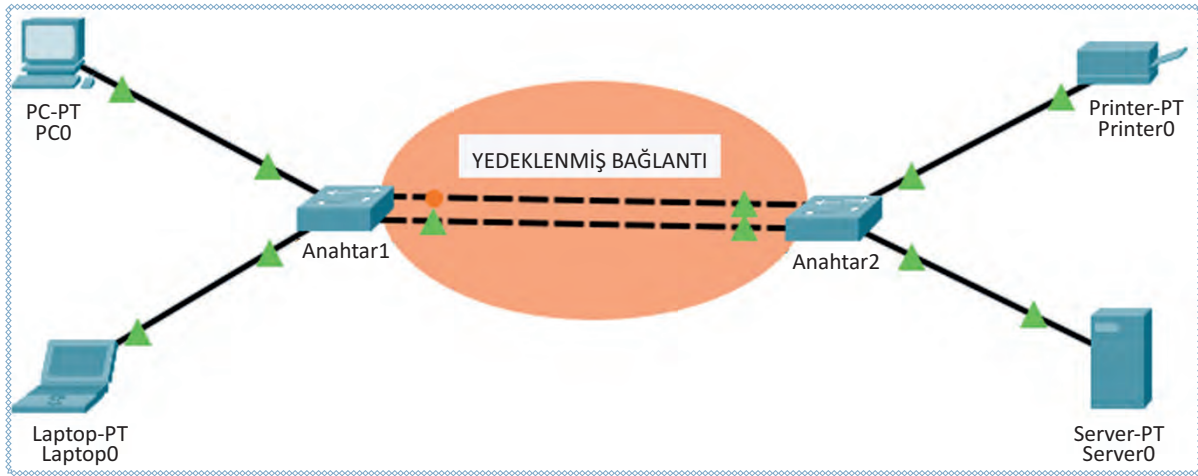
Görsel 8.1: İki anahtar arasında yedeklenmiş bir bağlantı tasarımı
