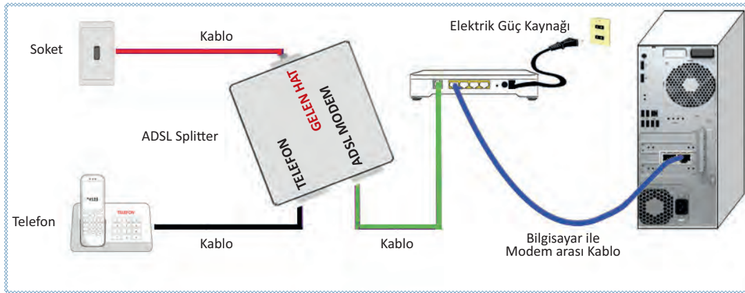
Görsel 2.16: ADSL bağlantı şeması
