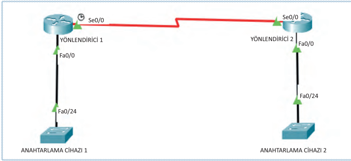
Görsel 11.5: Fast Ethernet arayüzünde düz kablo kullanımı
