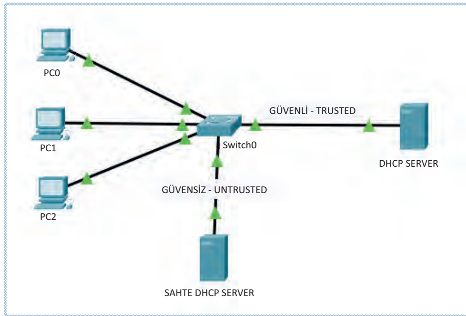
Görsel 10.21: DHCP araya girme topolojisi
