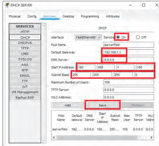
Görsel 10.22: DHCP SERVER yapılandırması
