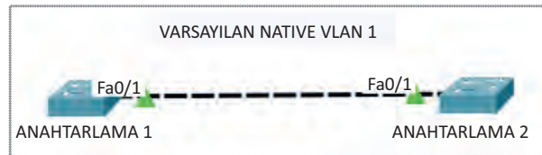
Görsel 10.35: Native VLAN uygulaması
