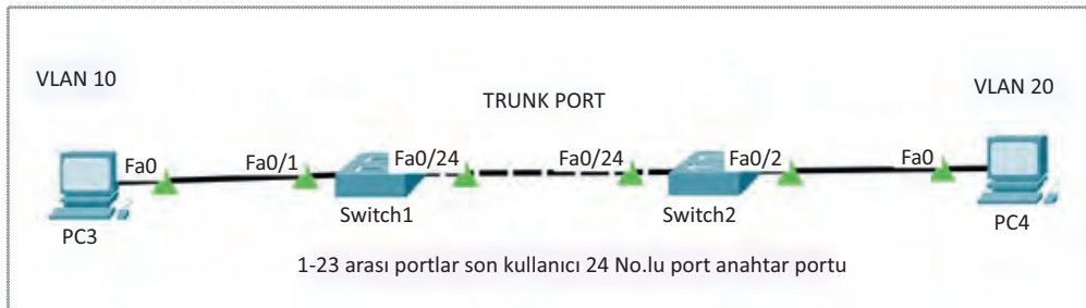
Görsel 10.34: VLAN atlama topolojisi
