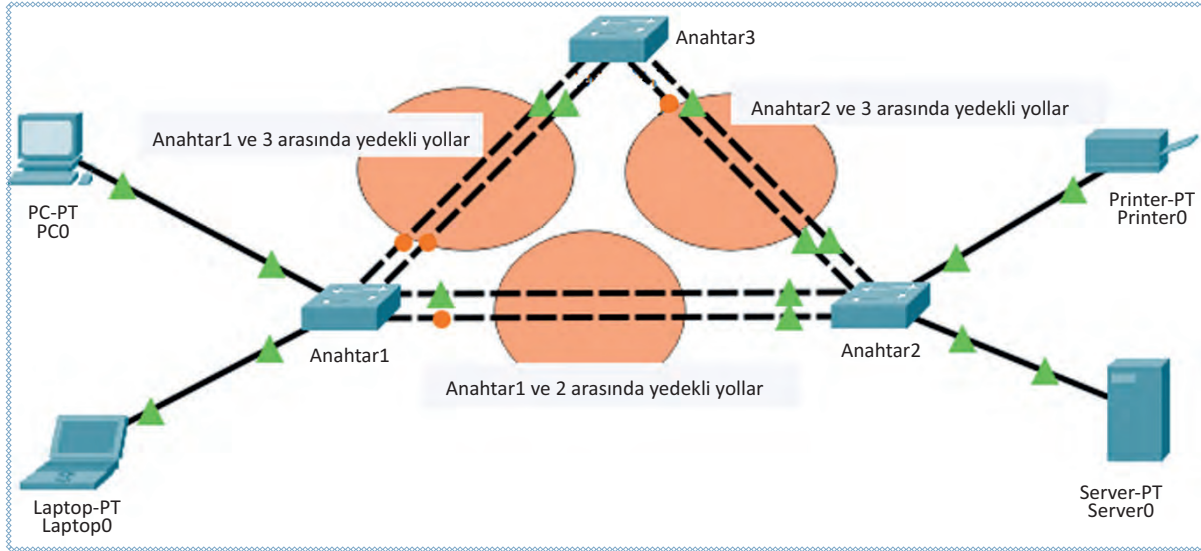
Görsel 8.2: Üç anahtar arasında yedekli bağlantı tasarımı
