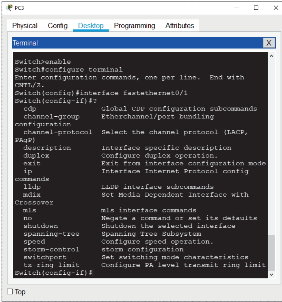
Görsel 6.21: Arayüz konfigürasyon modu
