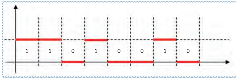
Görsel 1.3: Verinin elektrik sinyalleri sayısal gösterimi
