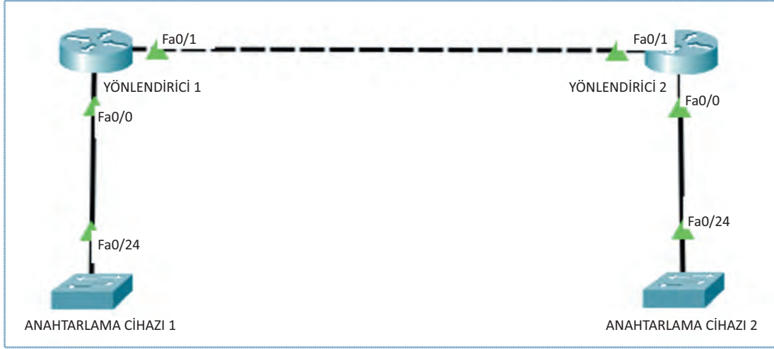
Görsel 11.4: Fast Ethernet arayüzünde çapraz kablo kullanımı
