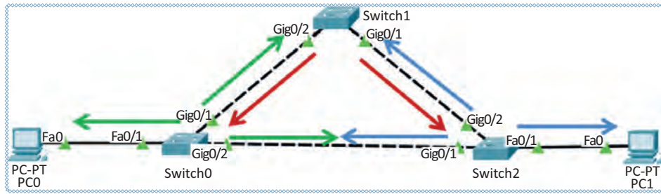
Görsel 8.9: STP algoritması kullanılmadan yayın paketlerinin anahtar cihazlardaki trafiği
