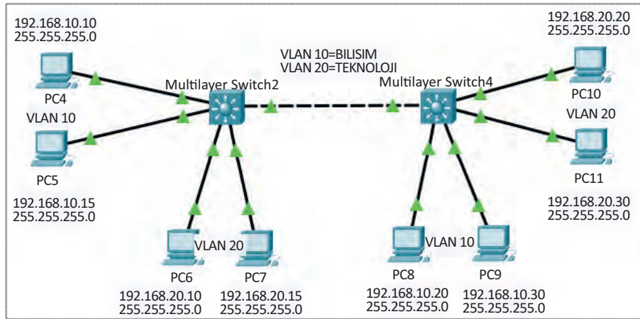
Görsel 9.8: Üçüncü katma anahtarlama VLAN yapılandırma topolojisi
