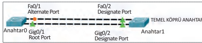
Görsel 8.43: Farklı bağlantı hızlarında STP tercih yolları
