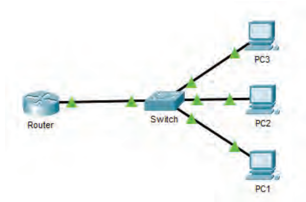
Görsel 3.2: DHCP senaryosu
