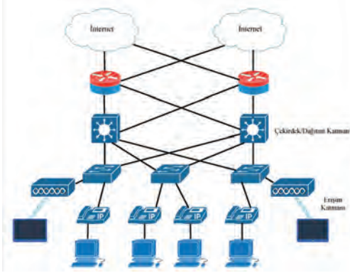
Görsel 2. 1: İki katmanlı model
