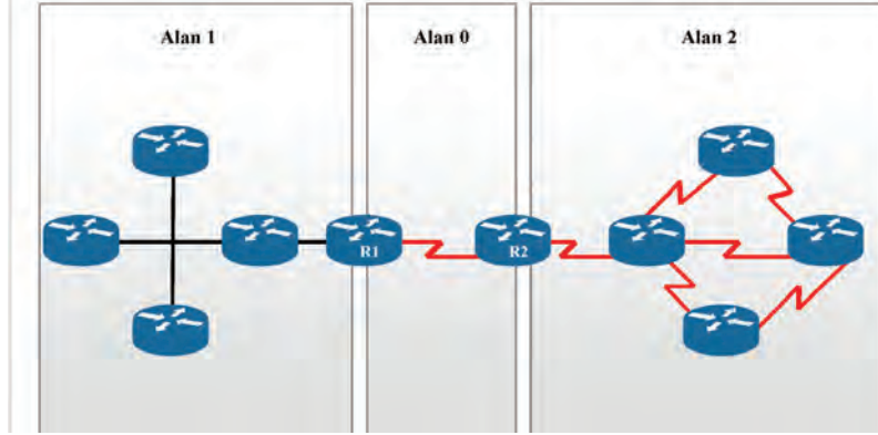
Görsel 2. 7: Çok alanlı OSPF
