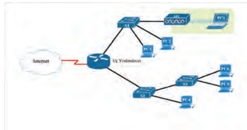
Görsel 2. 5: Kablosuz ağ hata etki alanı
