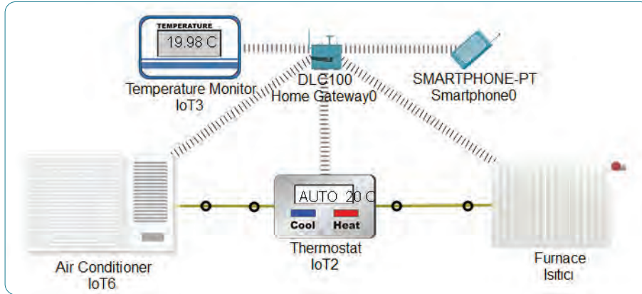
Görsel 2.58: Akıllı ev otomatik ısıtma soğutma sistemi
