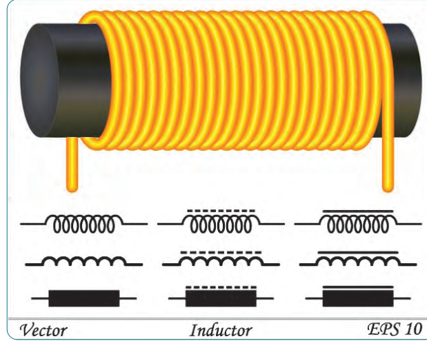
Görsel 2.4: Bobin
