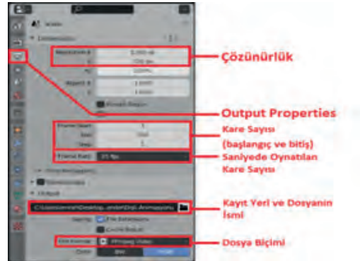
Görsel 3.259: Output Properties parametreleri
