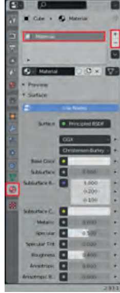
Görsel 3.177: Material Properties menüsü ve parametreleri
