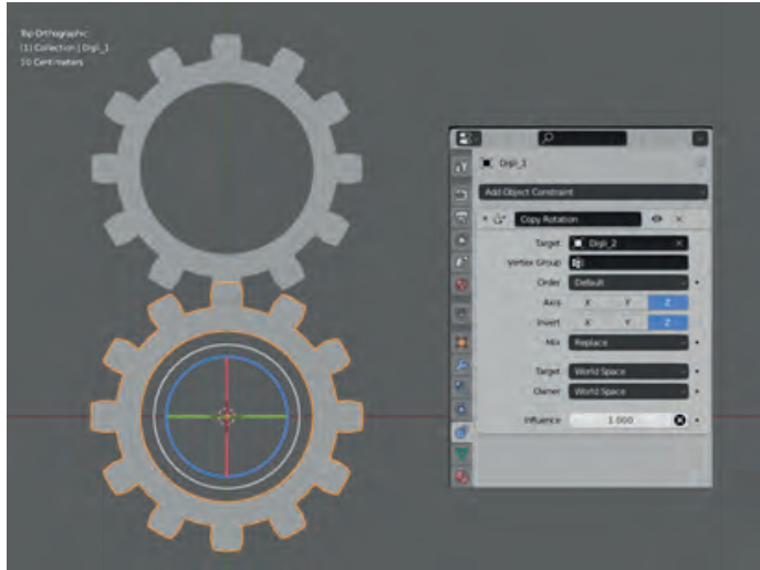
Görsel 3.229: Copy Rotation parametreleri
